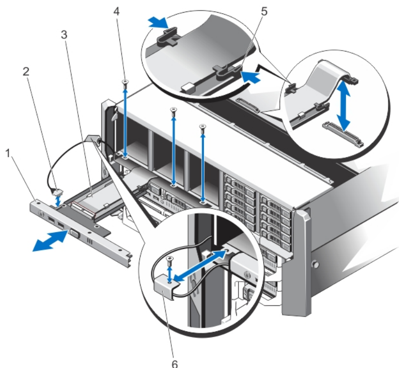
図 81. コントロールパネルの取り外しと取り付け
