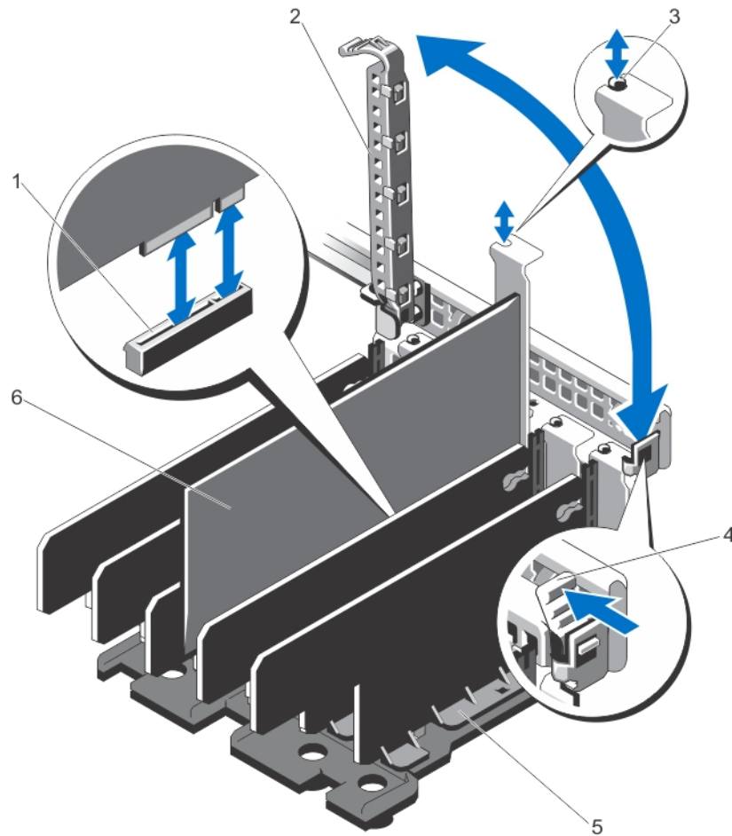
図 64. ロープロファイル拡張カードの取り外しと取り付け
