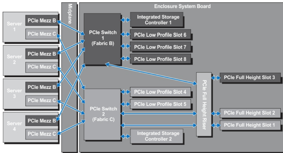
図 27. PCIe 拡張スロットのマッピング — ハーフハイトのサーバーモジュール
