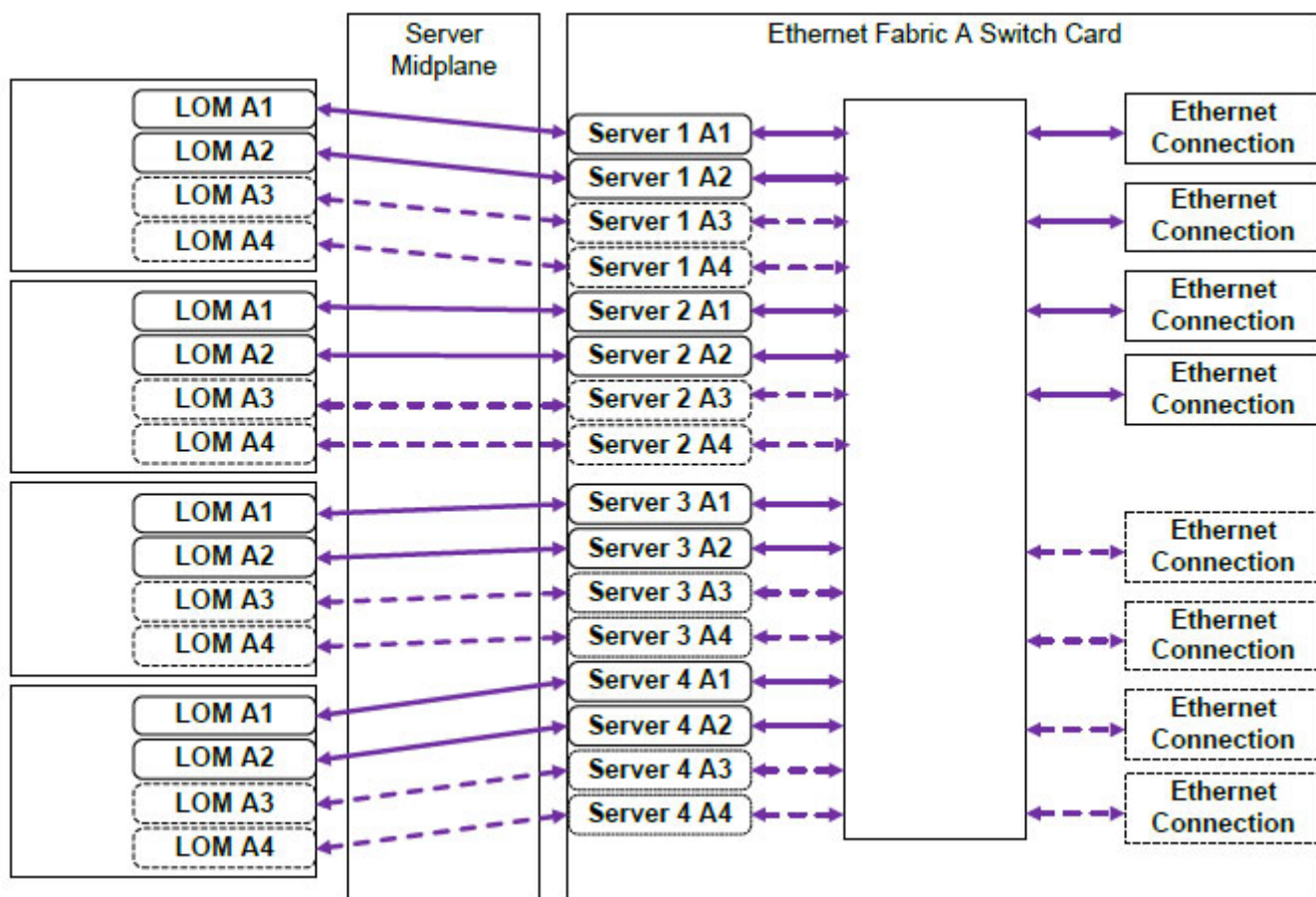
図 25. VRTX ハーフ ハイト ブレード 接続
