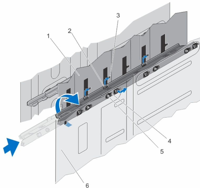
図 47. スロット 2 と 4 の間のサーバーモジュールパーティションの取り付け
