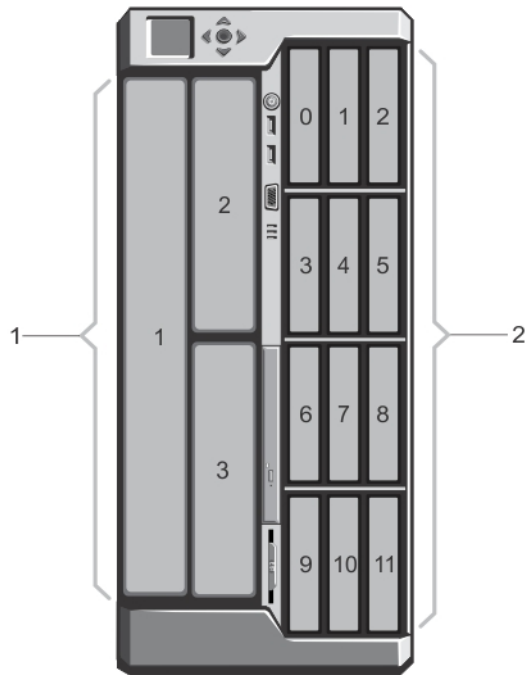
図7. サーバモジュール（ハーフハイトとフルハイトサーバモジュール）とハードドライブの番号付け — 3.5 インチハードドライブシャーシ
