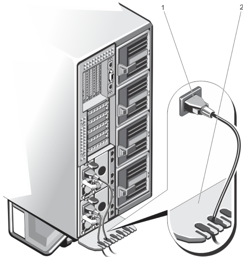
図 51. ホイールアセンブリがある場合の電源ケーブルの固定
