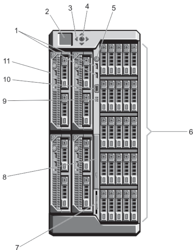
図 14. 前面パネルの機能とインジケータ — 2.5 インチハードドライブシャーシ
