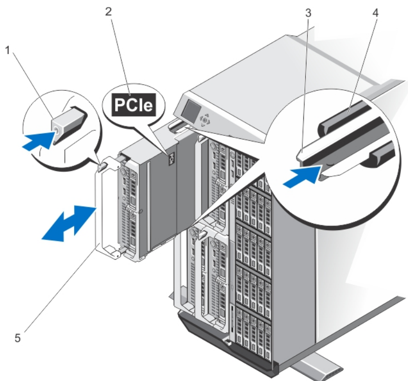
図 42. サーバモジュールの取り外しと取り付け
