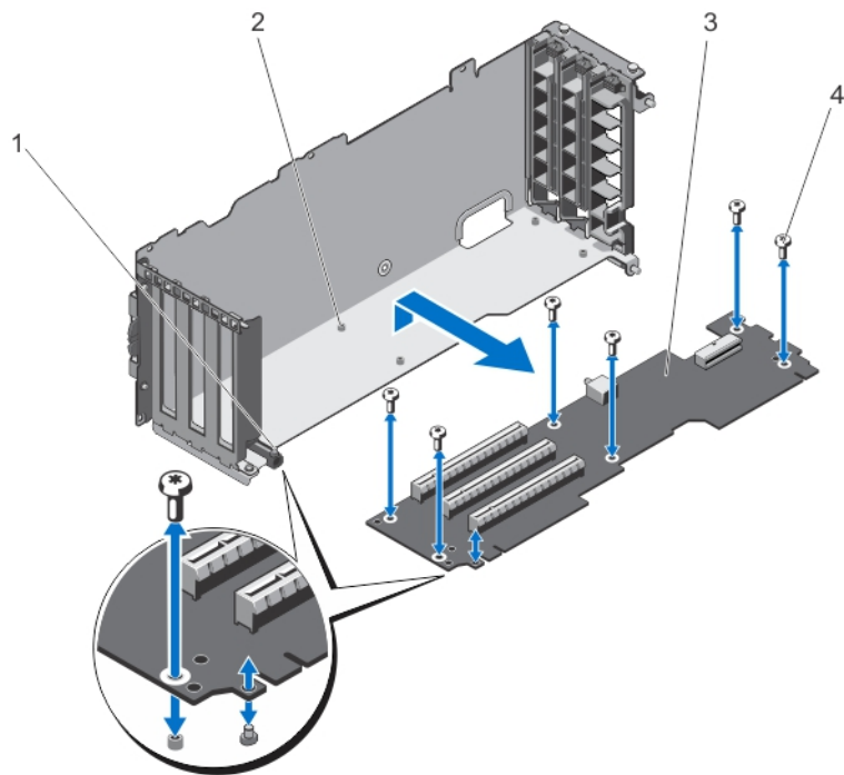
図 69. 拡張カードライザーの取り外しと取り付け
