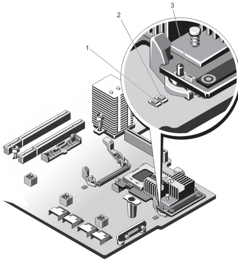
図 75. ストレージコントローラインジケータ
