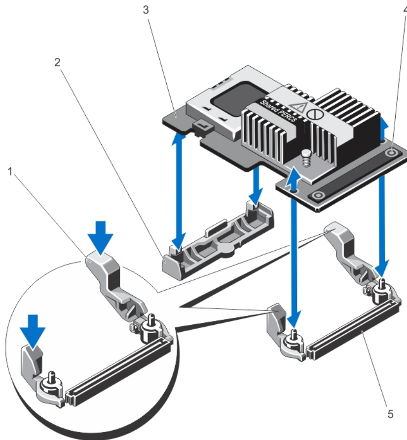
図 76. 内蔵ストレージコントローラカードの取り外しと取り付け
