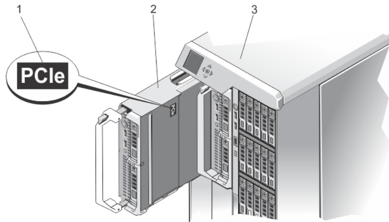
図 1. PowerEdge VRTX エンクロージャ用に構成されたサーバーモジュールの識別
