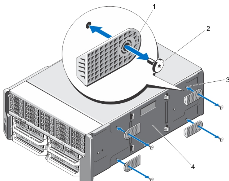
図 30. システムスタビライザーの取り外しと取り付け
