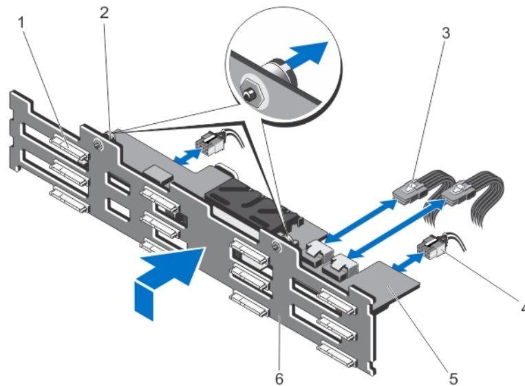
図 86. 3.5 インチ (x12) ハードドライブバックプレーンの取り外しと取り付け
