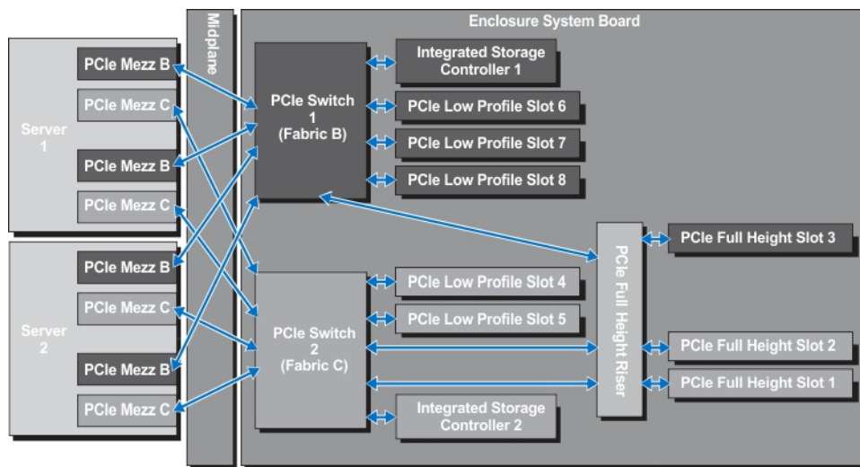
図 28. PCIe 拡張スロットのマッピング — フルハイトのサーバーモジュール
