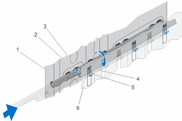
図 46. スロット 1 と 3 の間のサーバーモジュールパーティションの取り付け
