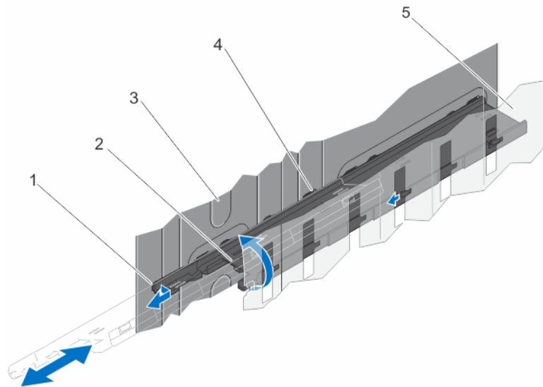
図 44. スロット 1 と 3 の間のサーバーモジュールパーティションの取り外しと取り付け
