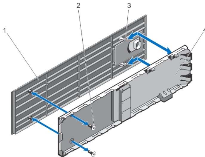
図 96. PCIe ケージドアカバーの取り外しと取り付け
