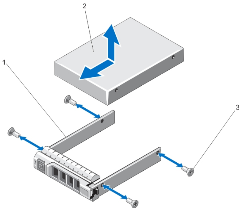
図 38. ハードドライブキャリアに対する 2.5 インチハードドライブの取り外しと取り付け
