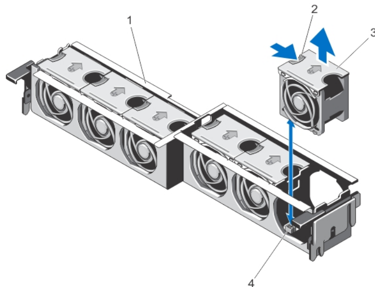
図 53. 冷却ファンの取り外しと取り付け
