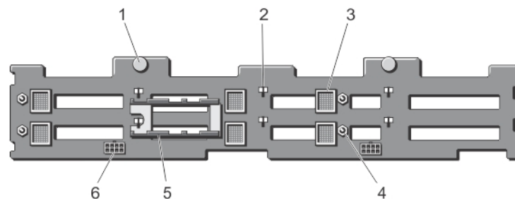
図 87. 3.5 インチ (x12) ハードドライブバックプレーンの背面図
