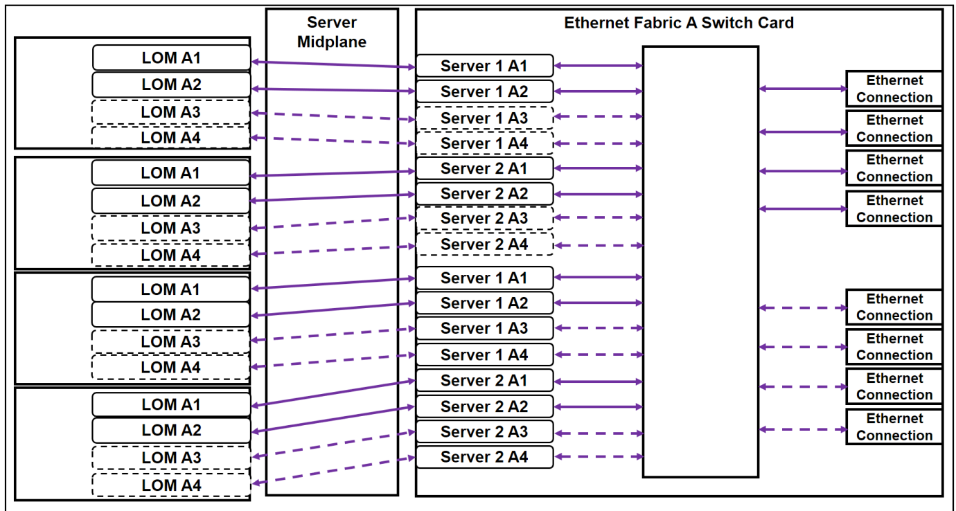
図 26. VRTX フル ハイット ブレード 接続
