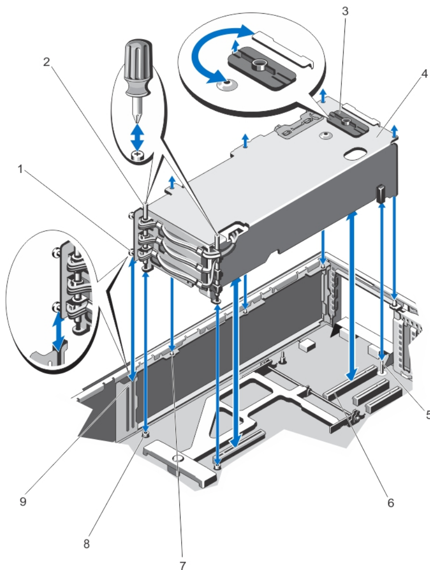
図 62. PCIe ケージの取り外しと取り付け
