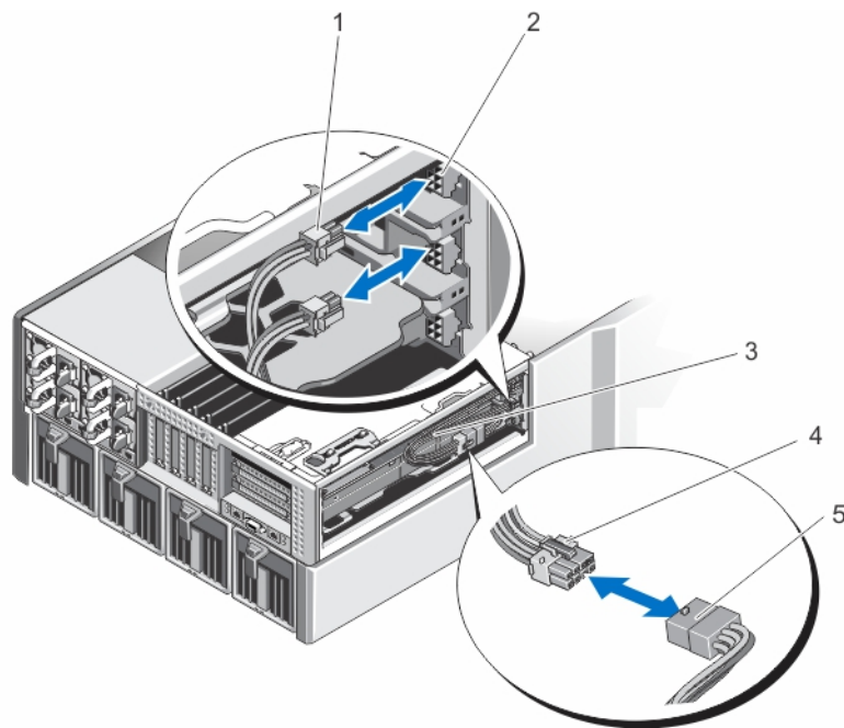
図 74. 補助電源ケーブルの電源ケーブルコネクタへの取り付け
