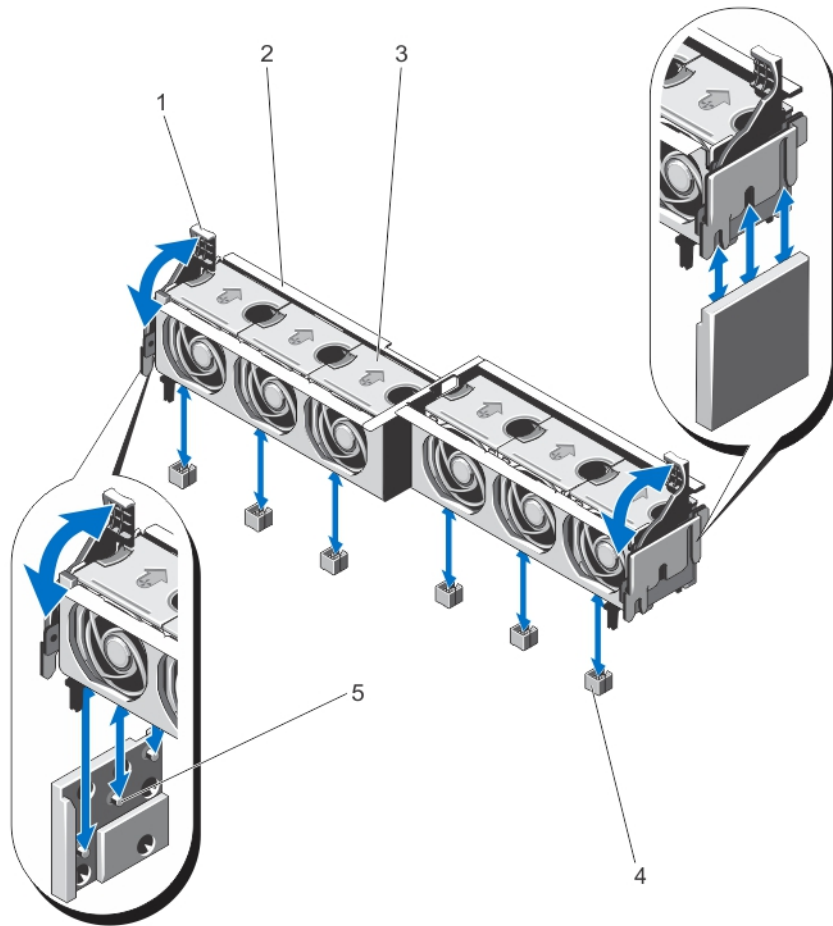
図 54. 冷却ファンアセンブリの取り外しと取り付け
