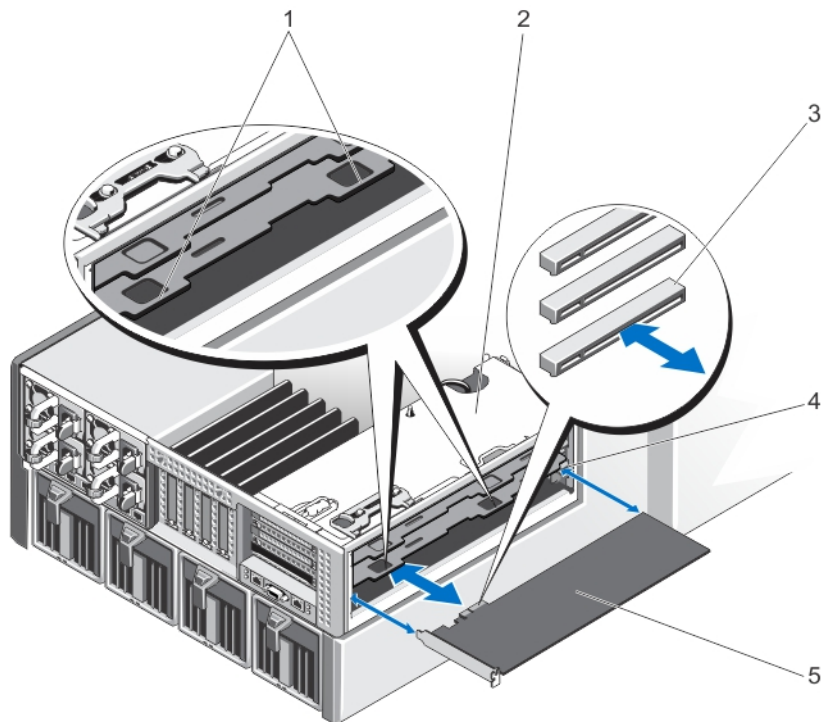
図 67. フルハイト拡張カードの取り外しと取り付け
