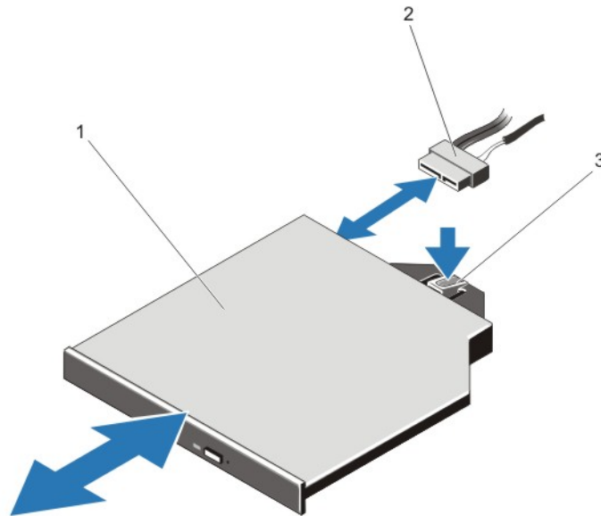
図 58. オプティカルドライブの取り外しと取り付け
