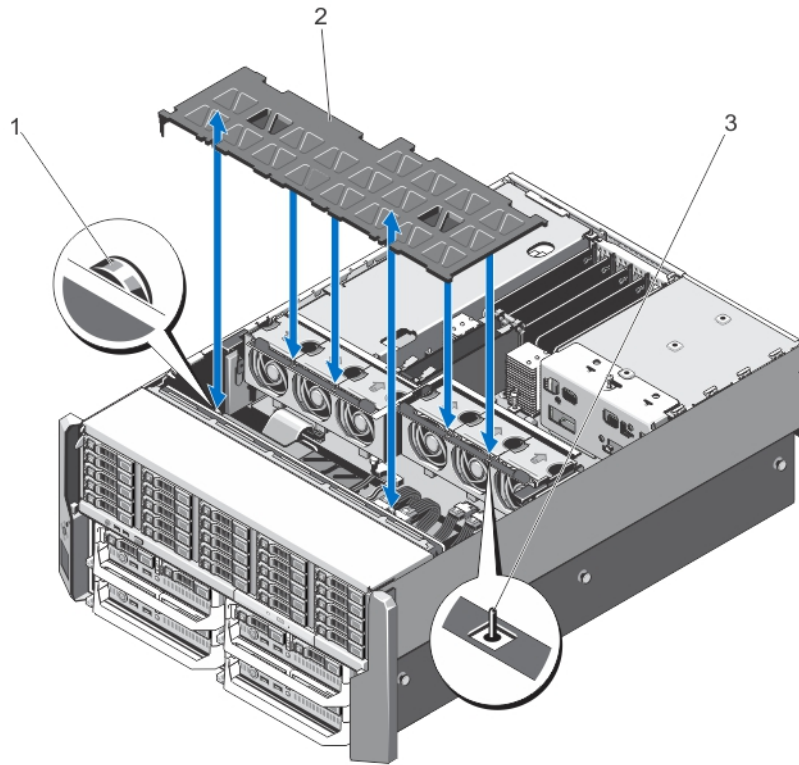
図 52. 冷却エアフローカバーの取り外しと取り付け
