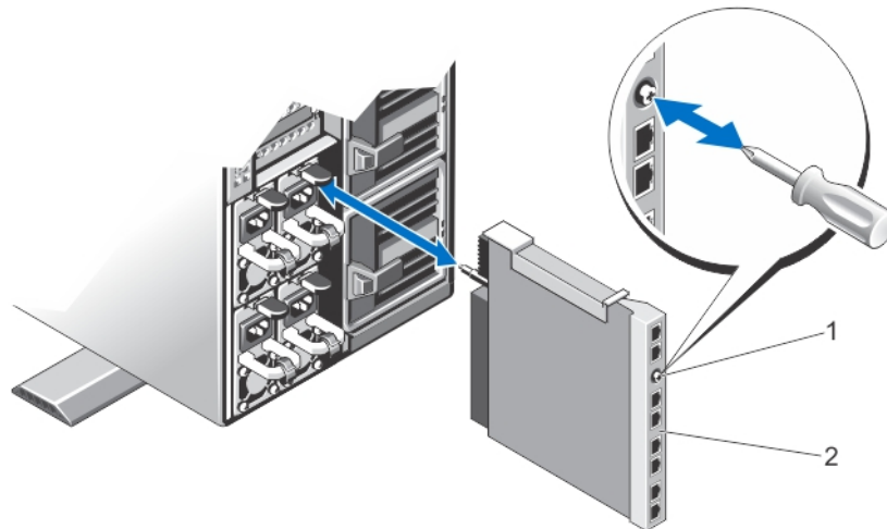
図 57. I/O モジュールの取り外しと取り付け
