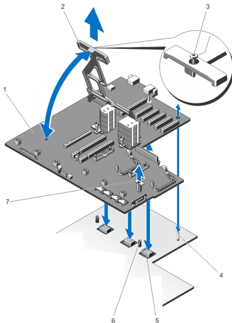
図 90. システム基板の取り外しと取り付け
