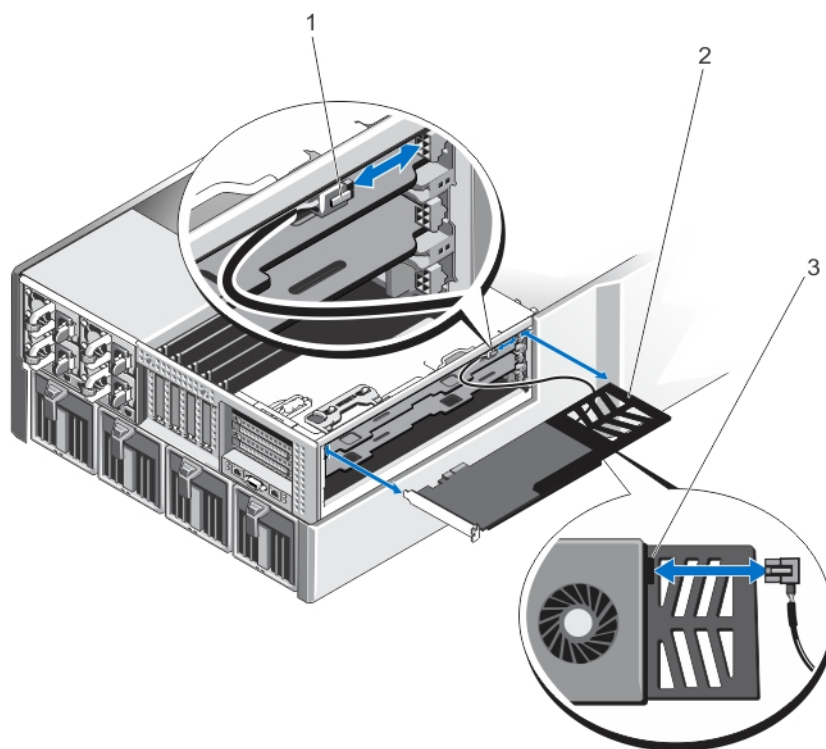
図 66. 拡張カードに対する電源ケーブルの取り外しと取り付け
