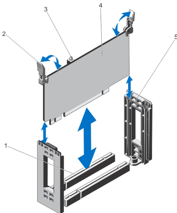
図 60. CMC カードの取り外しと取り付け
