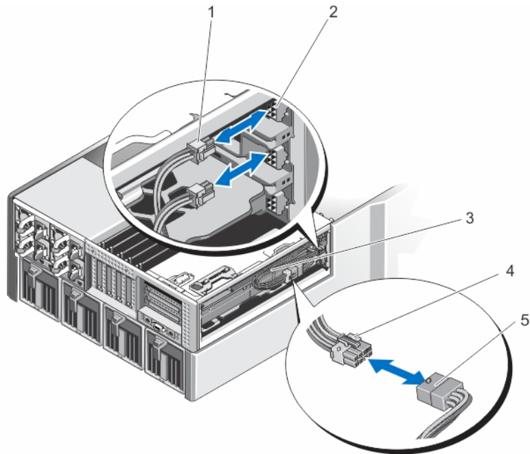
図 71. 補助電源ケーブルの電源ケーブルコネクタに対する取り外しと取り付け
