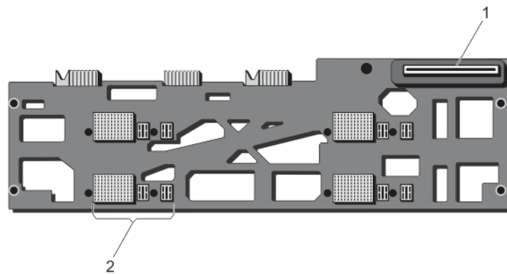
図 92. ミッドプレーンの取り外しと取り付け
