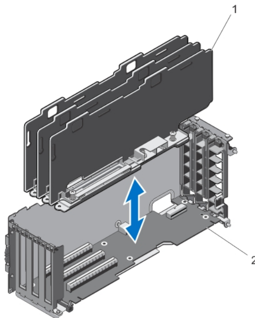
図 68. フルハイト拡張カード分岐ユニットの取り外しと取り付け
