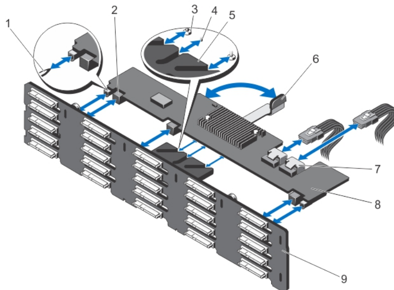
図 83. バックプレーンエキスパンダ基板の取り外しと取り付け
