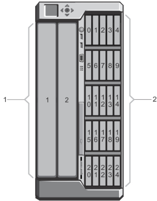
図 3. フルハイトサーバーモジュールとハードドライブの番号付け — 2.5 インチハードドライブシャーシ
