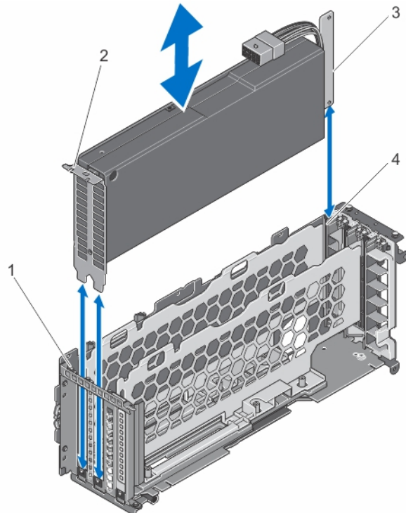
図 72. ダブルワイド GPGPU カードの取り外しと取り付け
