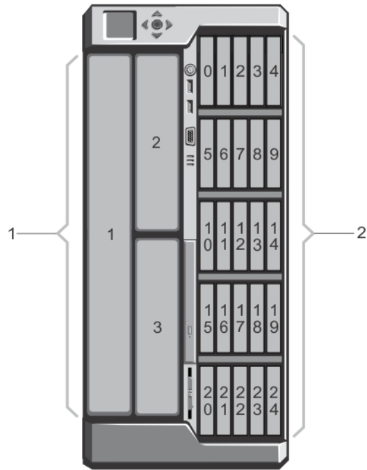
図 4. サーバーモジュール（ハーフハイトとフルハイトサーバーモジュール）とハードドライブの番号付け — 2.5 インチハードドライブシャーシ
