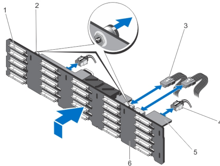
図 84. 2.5 インチ (x25) ハードドライブバックプレーンの取り外しと取り付け
