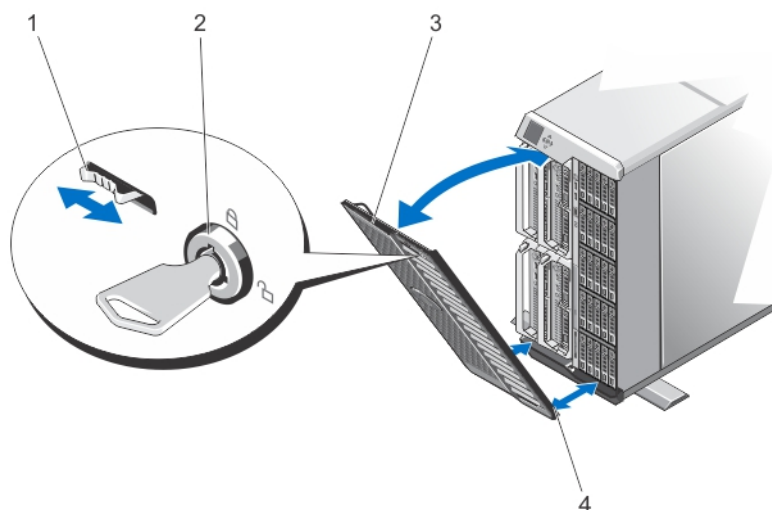
図 29. 前面ベゼルの取り外しと取り付け
