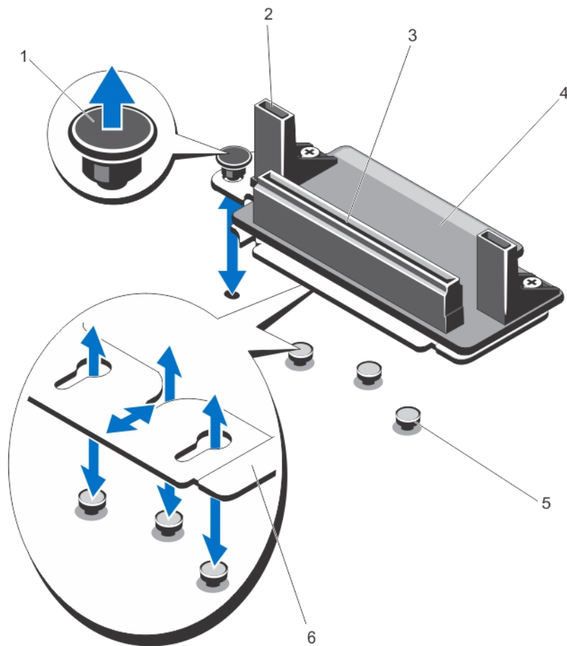
図 91. 電源パススルー基板の取り外しと取り付け
