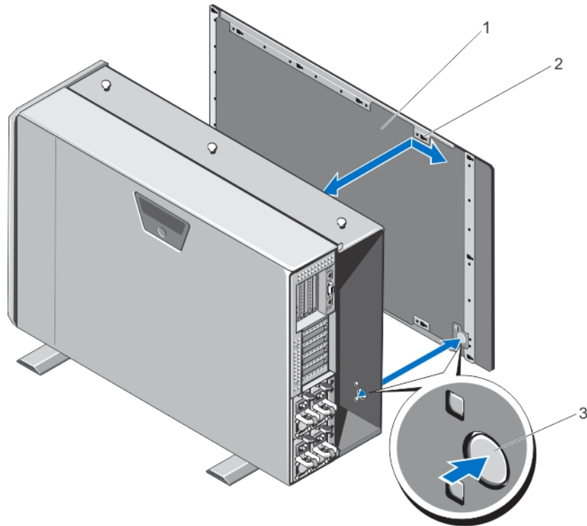
図 95. システム側面カバーの取り外しと取り付け
