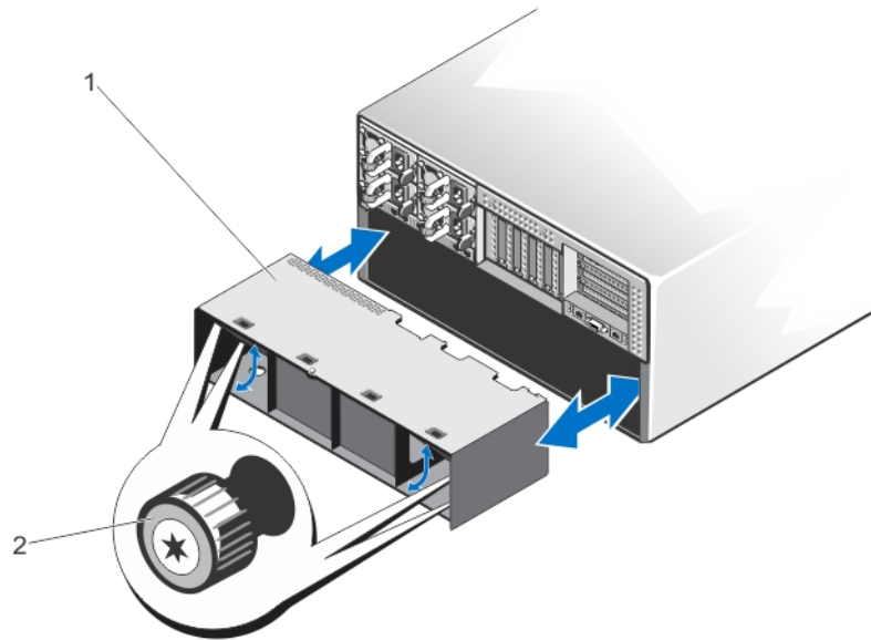
図 56. 送風装置モジュールベイの取り外しと取り付け
