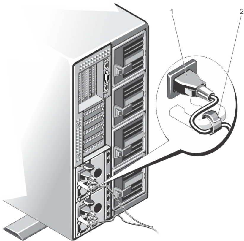
図 50. ホイールアセンブリがない場合の電源ケーブルの固定
