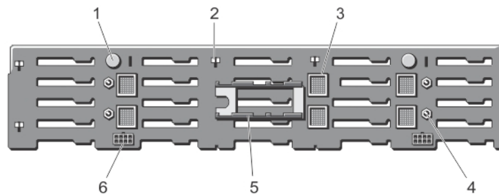
図 85. 2.5 インチ (x25) ハードドライブバックプレーンの背面図
