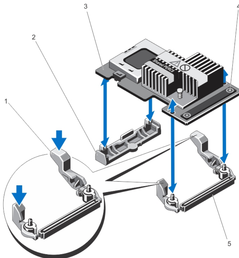
Figure 76. Retrait et installation d'une carte contrôleur de stockage intégré
