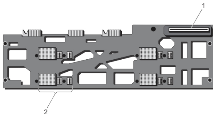
Figure 93. Vue avant du fond de panier central
