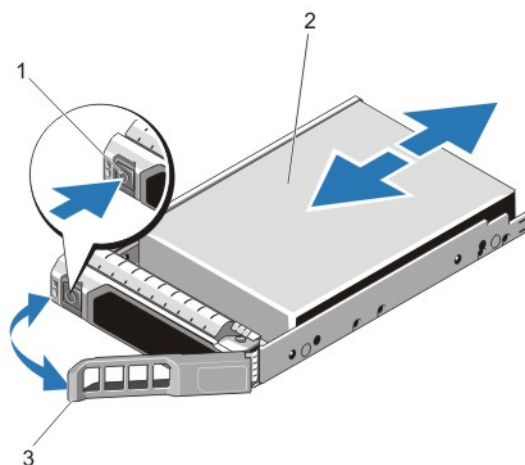
Figure 37. Retrait et installation d'un disque dur remplaçable à chaud
