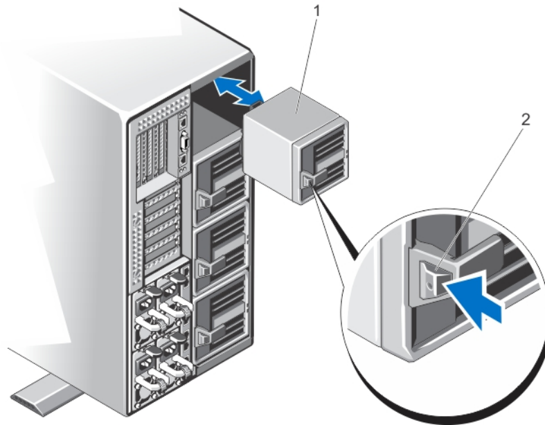
Figure 55. Retrait et installation d'un module de ventilation
