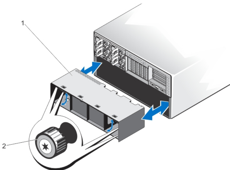
Figure 56. Retrait et installation de la baie du module de ventilation
