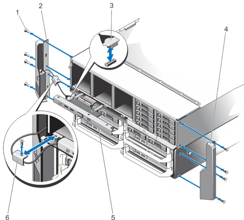
Figure 80. Retrait et installation des équerres de montage
