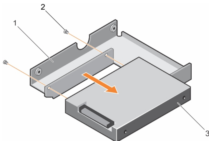
图 35: 将 2.5 英寸热插拔硬盘驱动器从 3.5 英寸硬盘驱动器适配器中卸下
