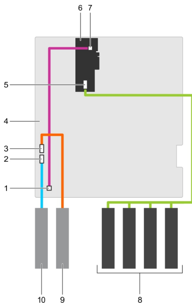
图 44: 布线 — 带有一个 PERC 卡的有线硬盘
