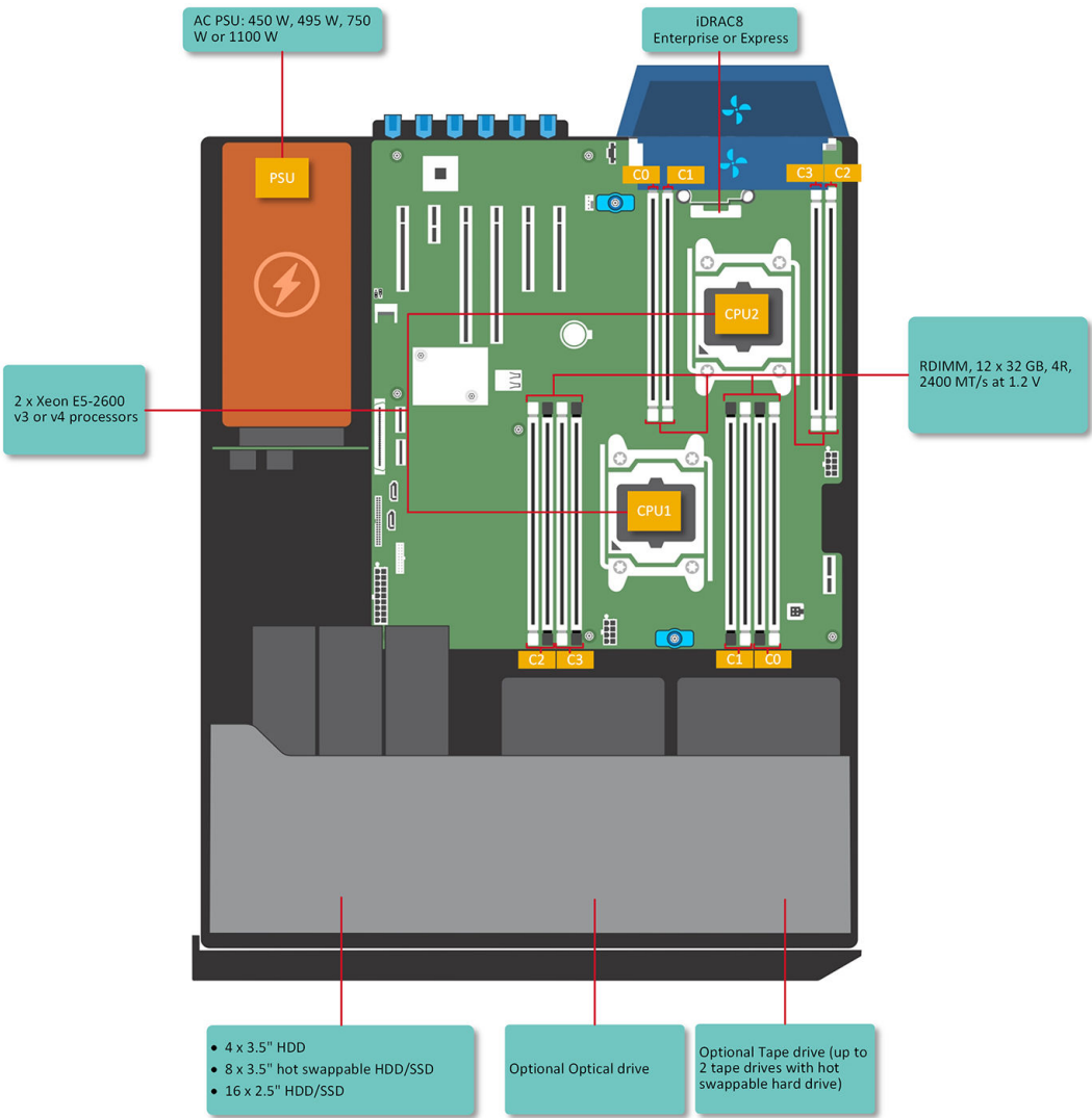
图 1: 所支持配置的系统视图
