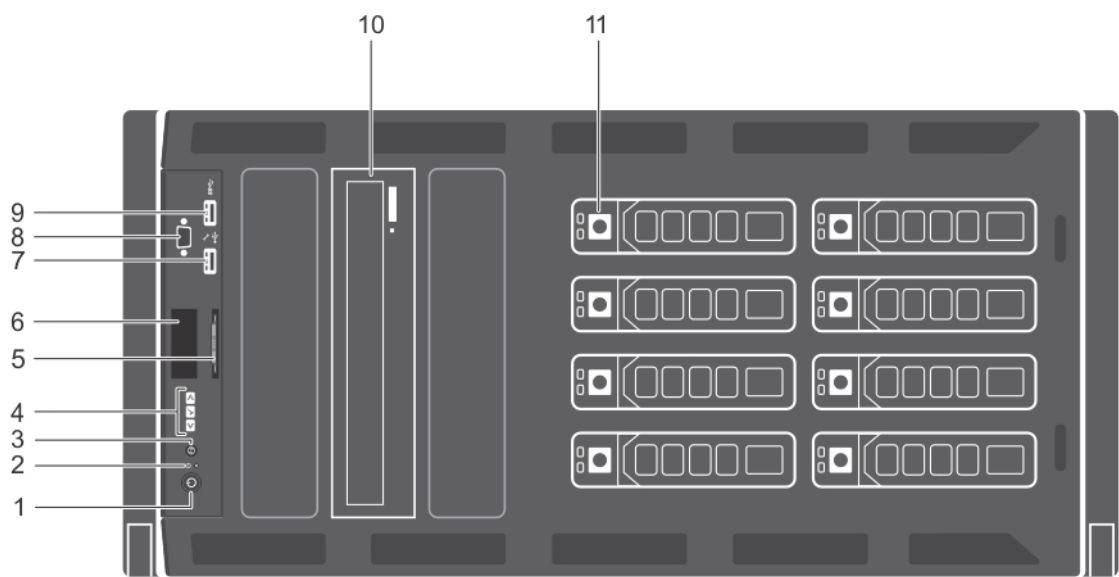
图 4: 前面板功能部件 - 机架模式下的 8 × 3.5 英寸热插拔硬盘机箱
