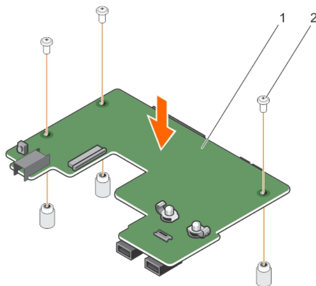
图 103: 为带有热插拔硬盘驱动器的系统安装控制面板线路板
