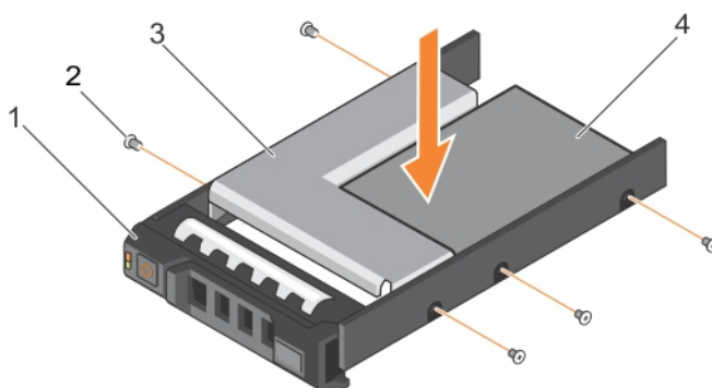
图 37: 将 3.5 英寸硬盘适配器安装到可热插拔硬盘托架中
