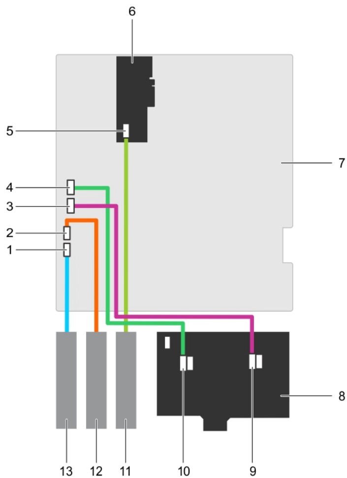
图 49: 布线 - 具有一个 PERC 卡的 x8 硬盘驱动器背板
