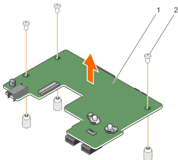
图 101: 从带有热插拔硬盘驱动器的系统卸下控制面板线路板
