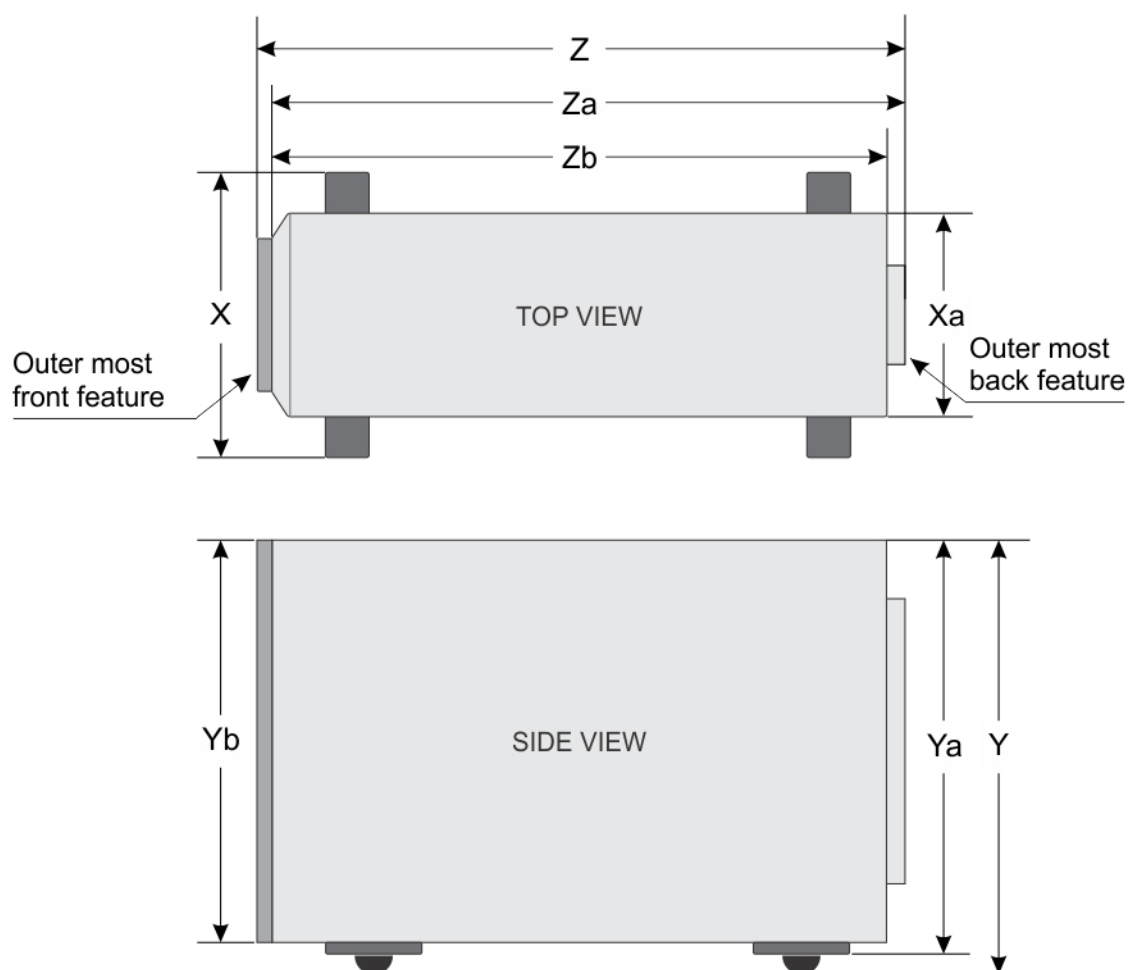
图 14: Dell PowerEdge T430 系统的机箱尺寸
