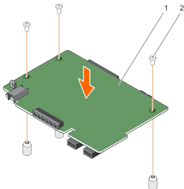
图 104: 为带有有线硬盘驱动器的系统安装控制面板线路板
