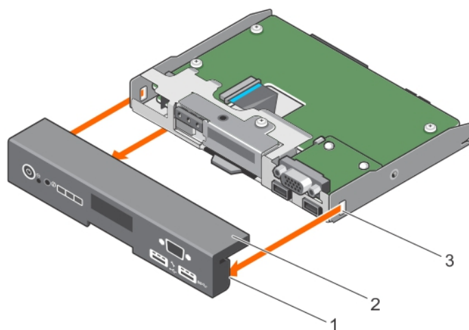
图 97: 从带有 LCD 面板的系统卸下控制面板部件护盖
