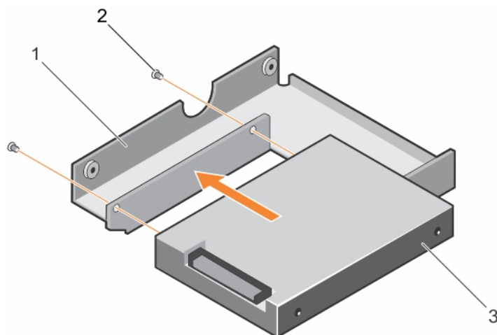
图 36: 将 2.5 英寸热插拔硬盘驱动器安装到 3.5 英寸硬盘驱动器适配器中
