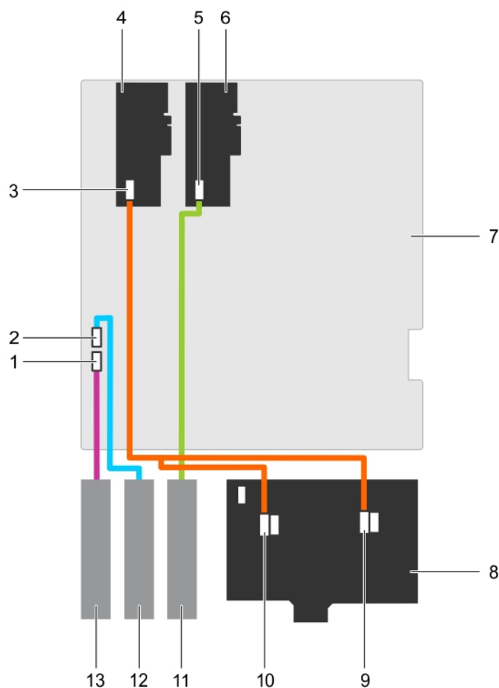
图 50: 布线 - 具有两个 PERC 卡的 x8 硬盘驱动器背板
