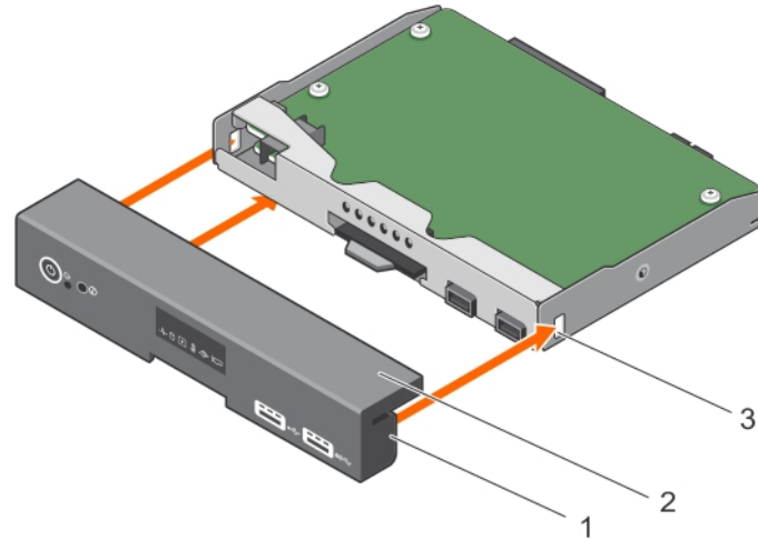
图 100: 为带有 LED 面板的系统安装控制面板部件护盖
