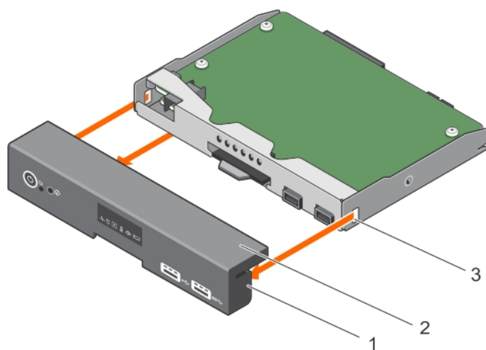
图 98: 从带有 LED 面板的系统卸下控制面板部件护盖
