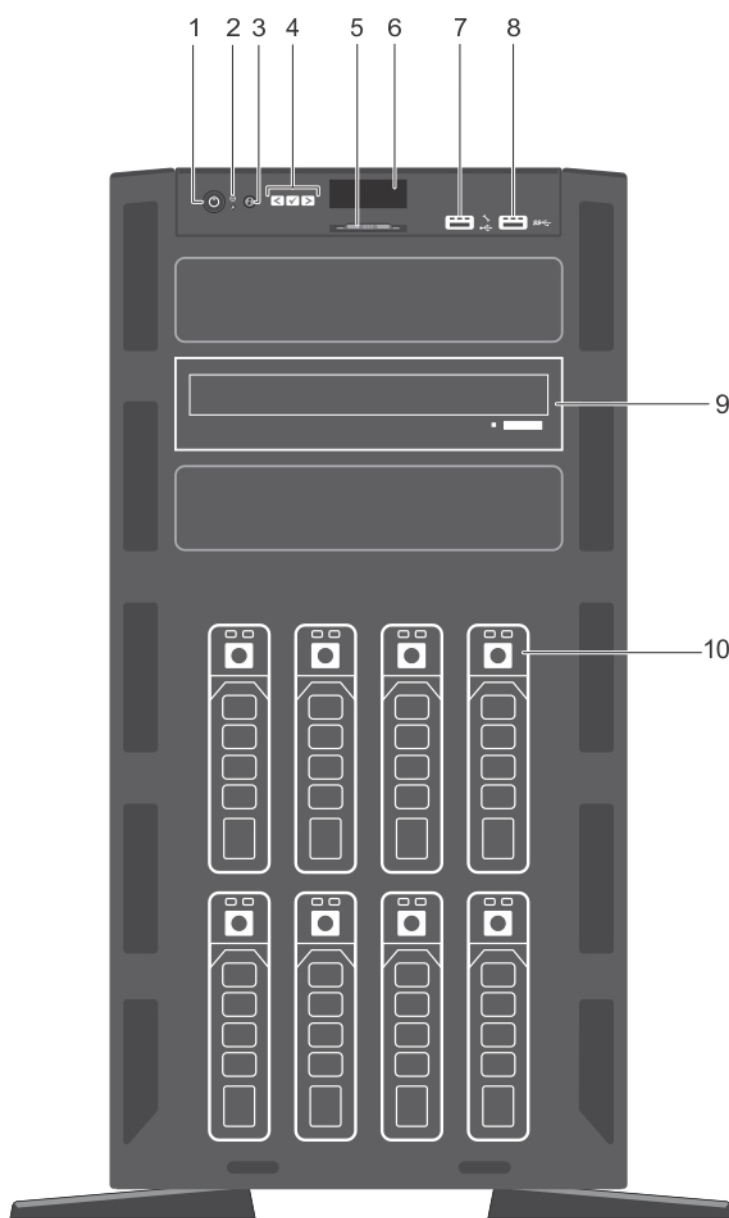
图 3: 8 × 3.5 英寸热插拔硬盘机箱的前面板功能部件
