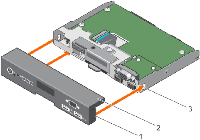
图 99: 为带有 LCD 面板的系统安装控制面板部件护盖
