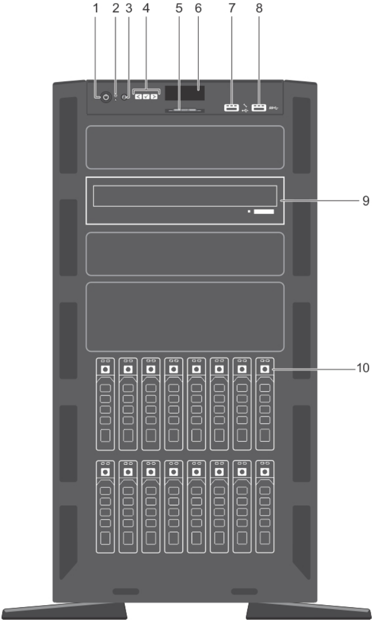
图 2: 16 x 2.5 英寸热插拔硬盘机箱的前面板功能部件
