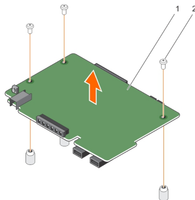
图 102: 此图显示如何为带有线硬盘驱动器的系统卸下和安装控制面板线路板
