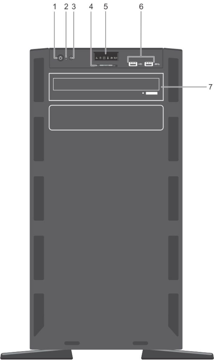
图 5: 前面板功能部件和指示灯 - 4 × 3.5 英寸有线硬盘驱动器机箱
