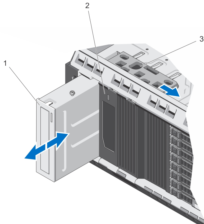
그림 17. 광학 드라이브 또는 테이프 드라이브 분리 및 설치
