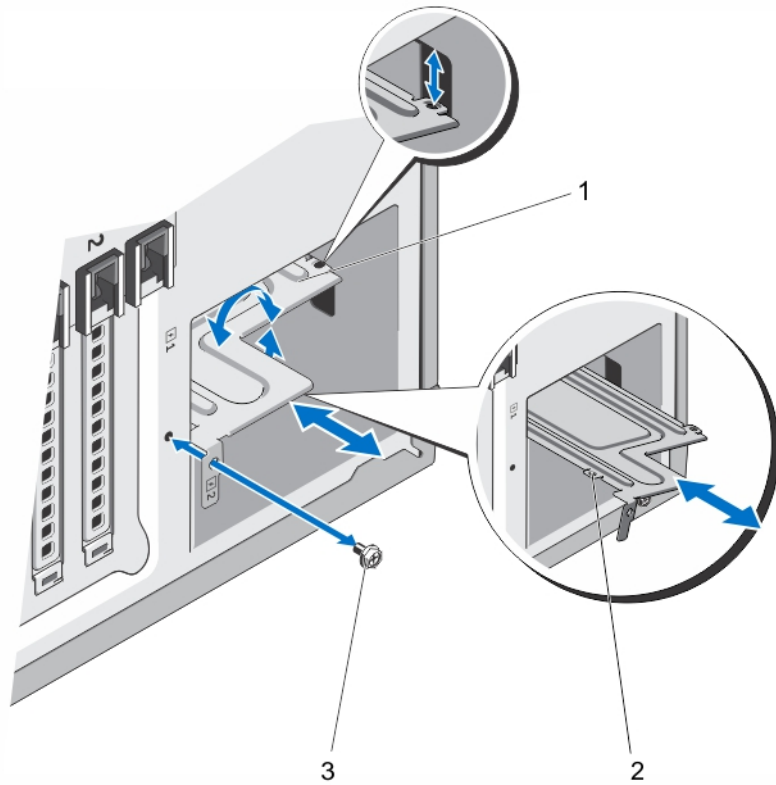
그림 54. 전원 공급 장치 분할기 분리 및 설치
