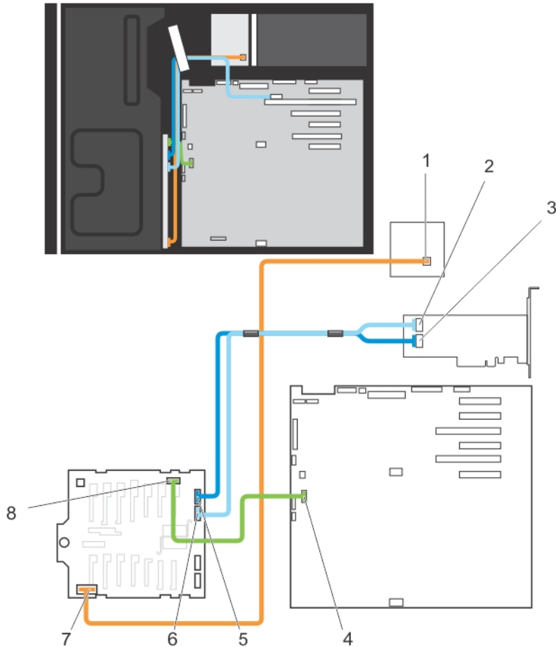
그림 33. 케이블 연결—확장 카드를 포함하는 x16 하드 드라이브 후면판
