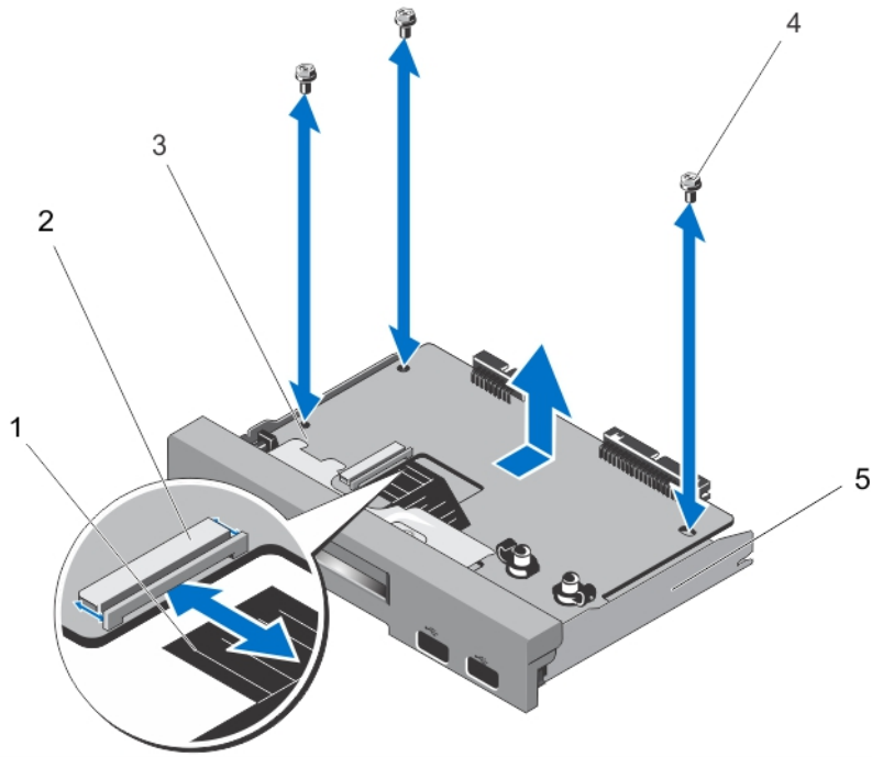
그림 64 . LCD 모듈을 포함하는 콘솔 보드 분리 및 설치
