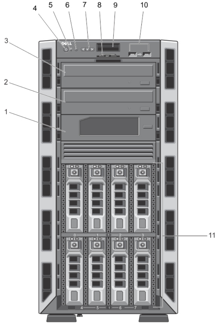
그림 2. 전면 패널 구조 및 표시등—3.5인치 핫 스왑 가능 하드 드라이브 새시
