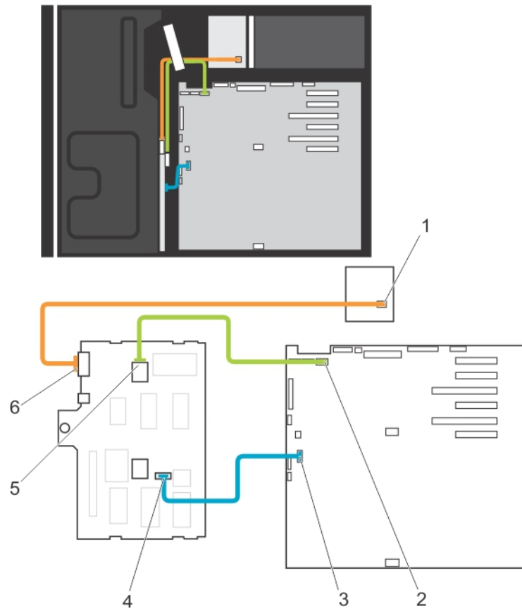
그림 30. 케이블 연결—x8 하드 드라이브 후면판
