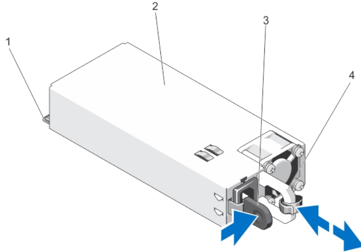
그림 52. 중복 AC 전원 공급 장치 분리 및 설치
