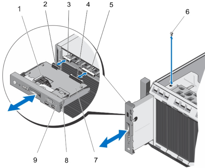
그림 60. 랙 모드 시스템에서 콘솔 조립품의 분리 및 설치
