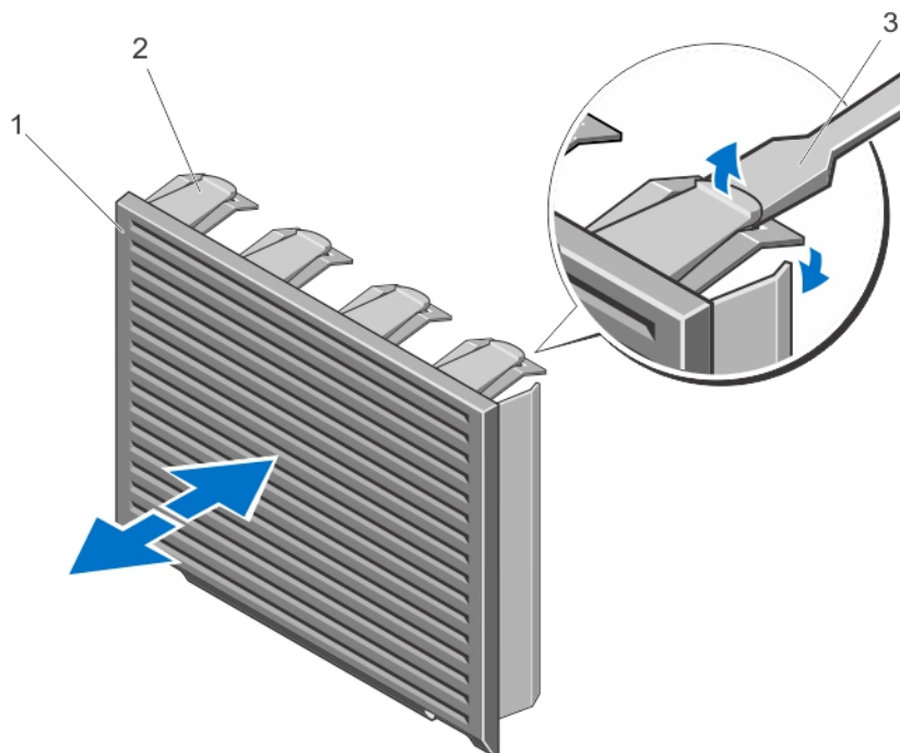
그림 34. 4중 슬롯 하드 드라이브 보호물 설치 및 분리
