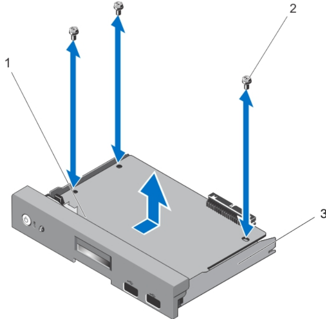
그림 65. 진단 표시등을 포함하는 콘솔 보드의 콘솔 분리 및 설치
