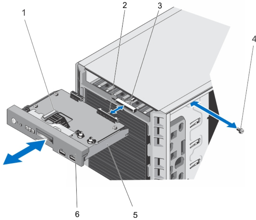
그림 58 . 타워 모드 시스템에서 LCD 모듈을 포함하는 콘솔 조립품의 분리 및 설치
