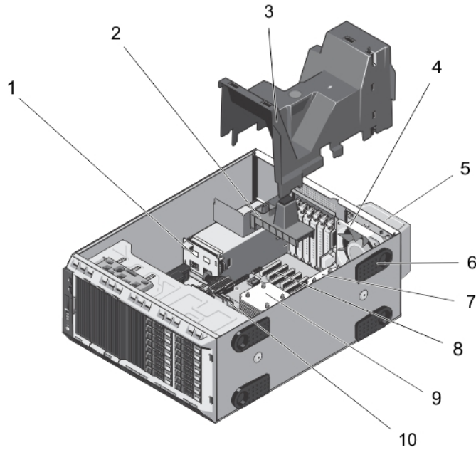
그림 15. 시스템 내부—핫 스왑 가능한 하드 드라이브 포함
