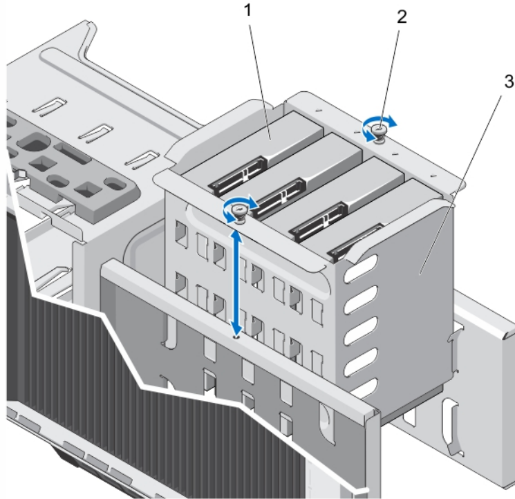
그림 26. 내부 하드 드라이브 베이 설치 및 분리
