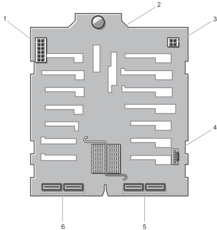
그림 32 . x16 하드 드라이브 후면판의 커넥터
