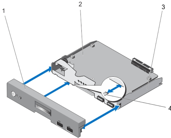
그림 63. 진단 표시등을 포함하는 시스템의 콘솔 분리 및 설치
