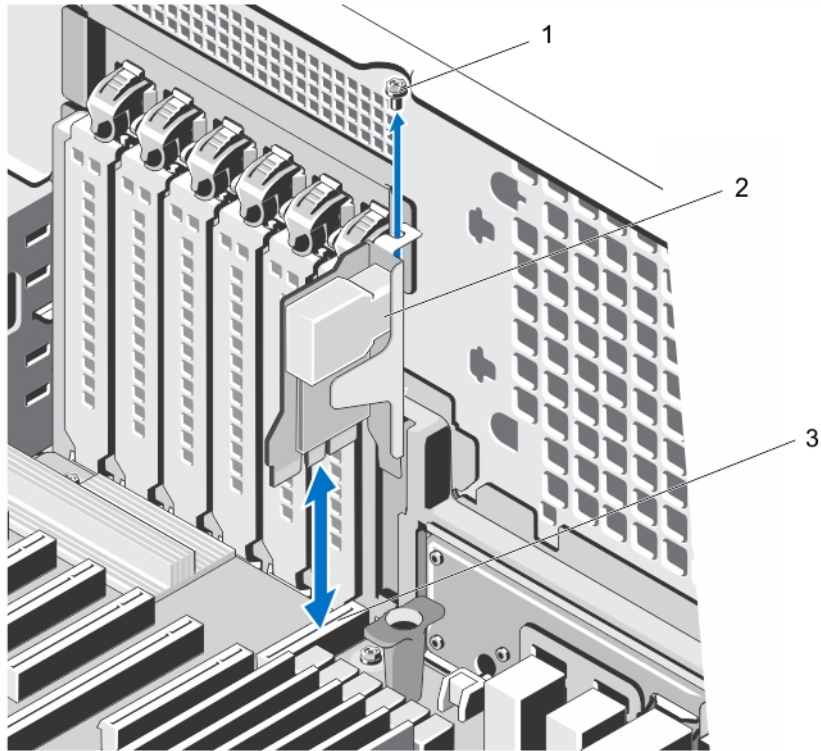
그림 47. iDRAC Ports 카드 분리 및 설치
