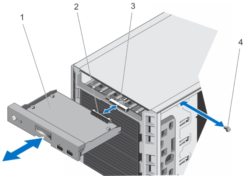
그림 59 . 타워 모드 시스템에서 진단 표시등을 포함하는 콘솔 조립품의 분리 및 설치
