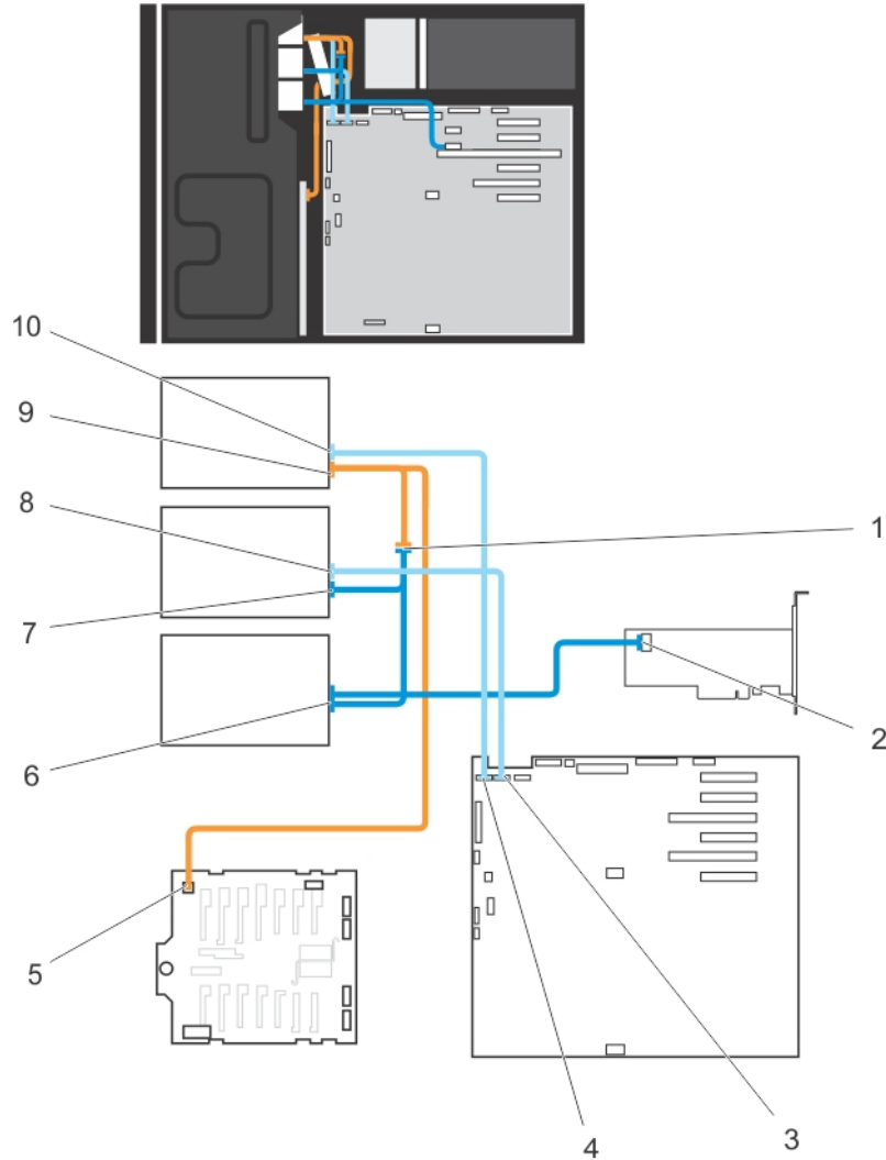
그림 18. 케이블 연결—광학 드라이브 및 테이프 드라이브
