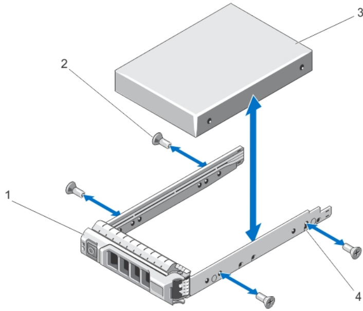
그림 24 . 하드 드라이브 캐리어에서 핫 스왑 하드 드라이브 분리 및 설치
