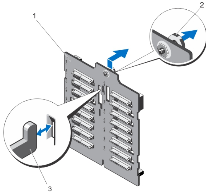
그림 31 . x16 하드 드라이브 후면판 분리 및 설치
