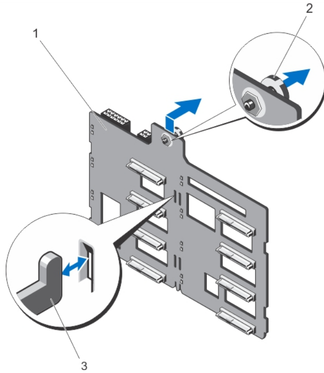
그림 28. x8 하드 드라이브 후면판 분리 및 설치
