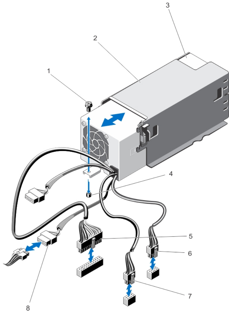
그림 55. 비중복 AC 전원 공급 장치 분리 및 설치
