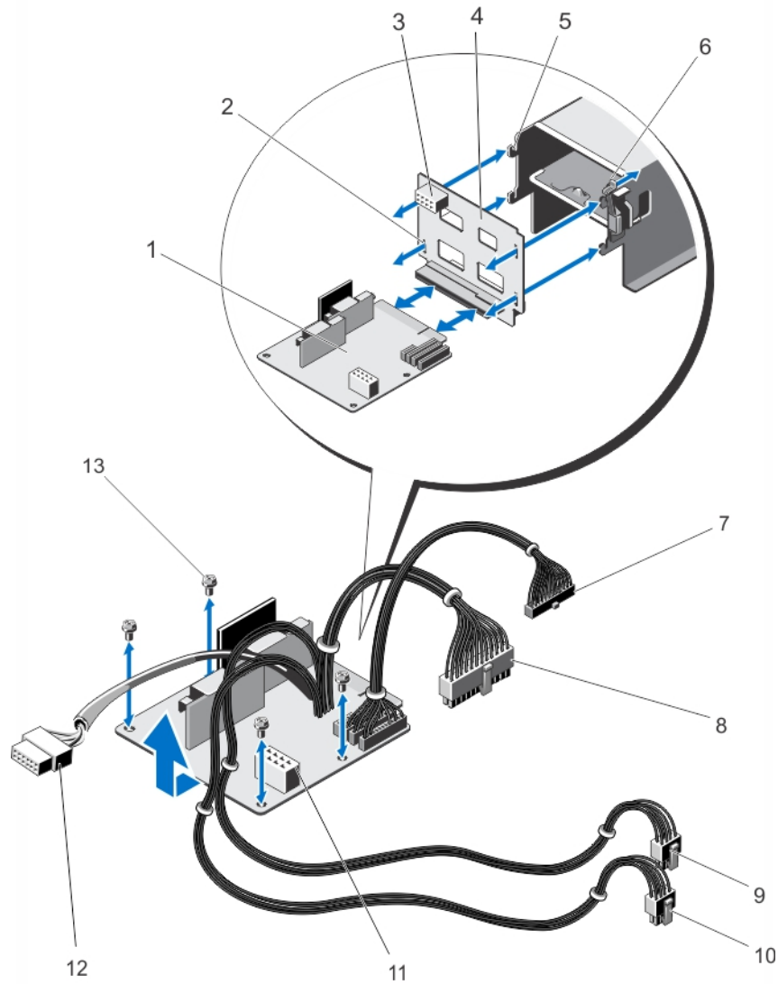
그림 56. 전원 장착 보드와 배전 보드 분리 및 설치
