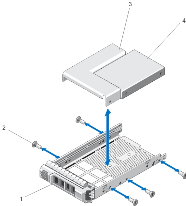
그림 25 . 3.5인치 하드 드라이브 캐리어에서 하드 드라이브 어댑터 분리 및 설치
