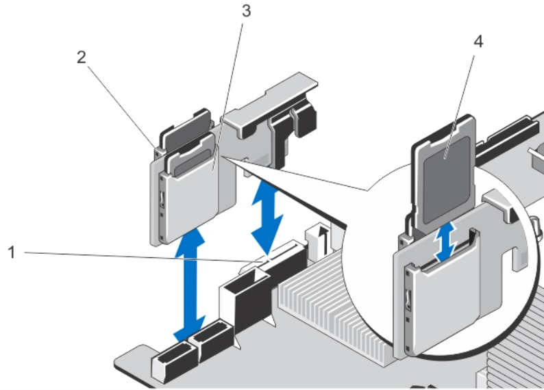
그림 49. 내부 이중 SD 모듈 분리 및 설치
