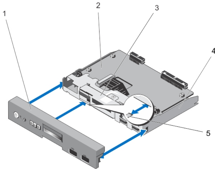
그림 62. LCD 모듈을 포함하는 시스템의 콘솔 분리 및 설치
