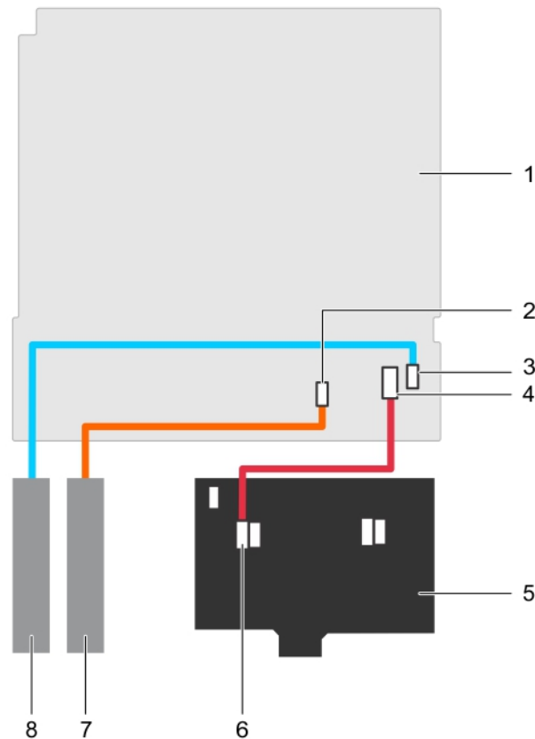
Figure 41. Câblage – fond de panier de disque dur x4
