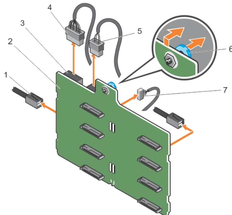
Figure 38. Retrait d'un fond de panier de disques durs x8
