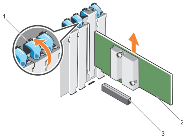
Figure 50. Retrait d'une carte d'extension
