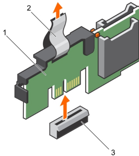
Figure 60. Retrait du module SD interne double (IDSMD)
