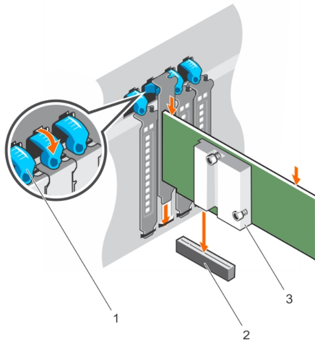
Figure 52. Installation d'une carte d'extension
