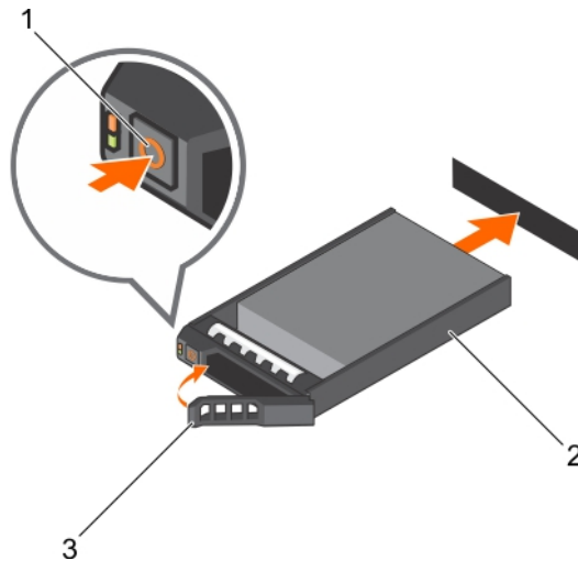
Figure 33. Installation d'un support de disque dur remplaçable à chaud
