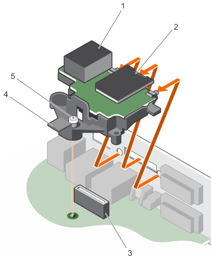
Figure 56. Retrait de la carte des ports iDRAC
