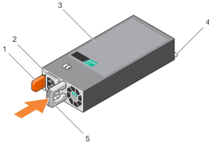
Figure 69. Installation d'un bloc d'alimentation redondant
