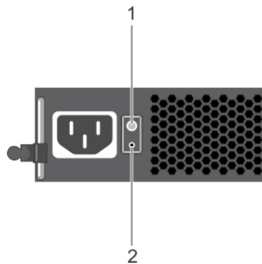
Figure 10. Voyant d'état et bouton d'auto-diagnostic du bloc d'alimentation câblé en CA non redondant
