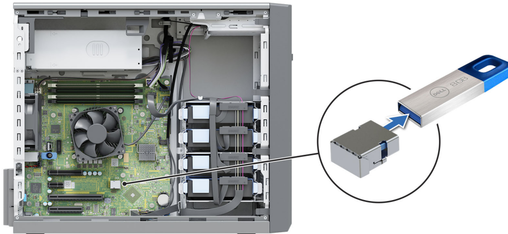
Ilustración 34. Extracción de la llave de memoria USB interna
