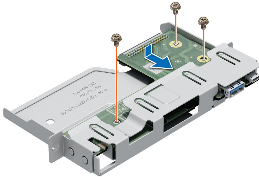
Ilustración 61. Instalación del panel de control
