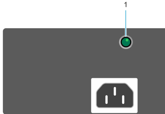
Ilustración 67. Indicador de estado de la fuente de alimentación de CA cableada no redundante
