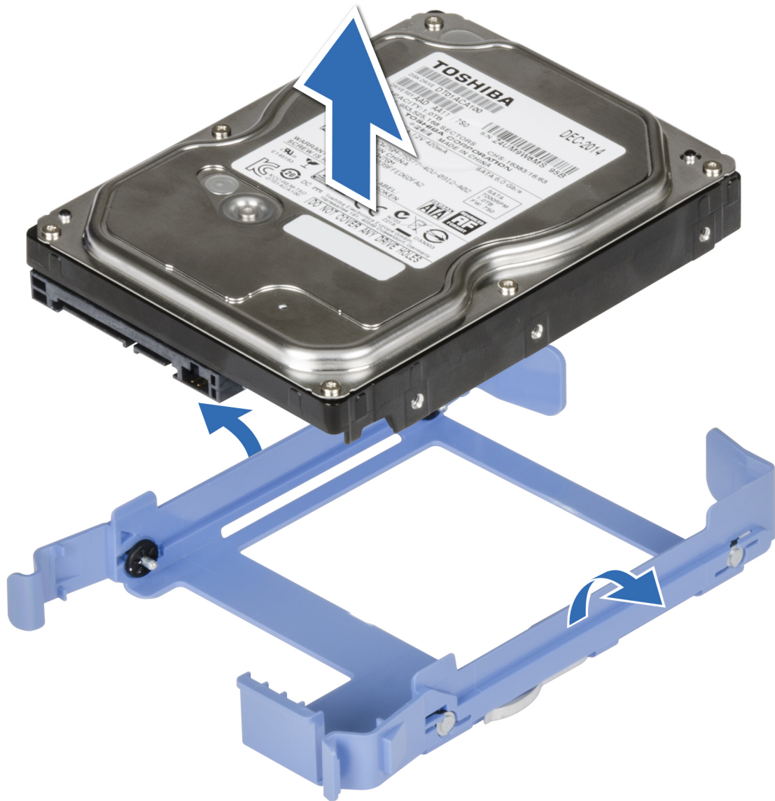
Ilustración 14. Extracción de una unidad del portaunidades
