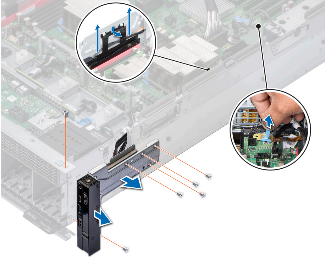
Rakam 106. Sağ kontrol panelini çıkarma
