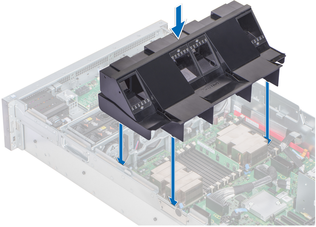
Rakam 29. Hava örtüsünü takma — İki işlemcili sistem
