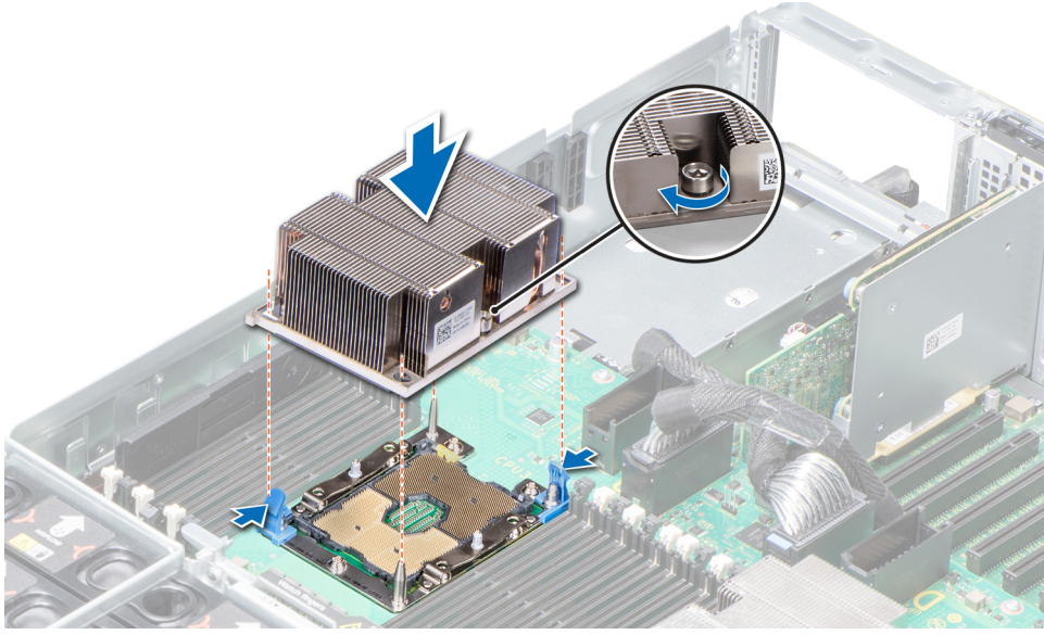
Rakam 67. İşlemciyi ve ısı emici modülünü takma
