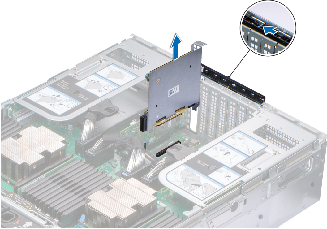
Rakam 84. NDC yükselticisini çıkarma
