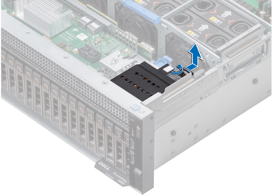
Rakam 98. NVDIMM-N pili çıkarma
