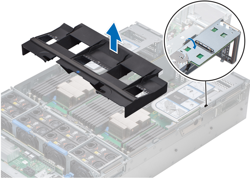
Rakam 28. Hava örtüsünü çıkarma — Dört işlemcili sistem
