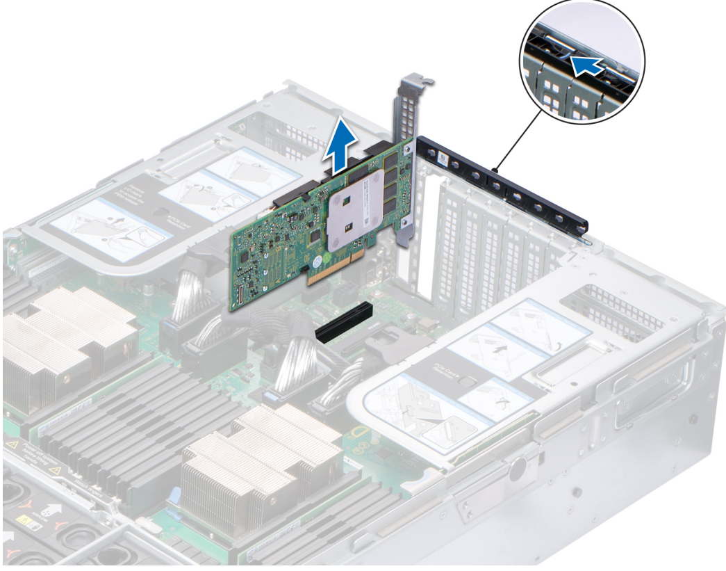
Rakam 88. Depolama denetleyicisi kartını çıkarma
