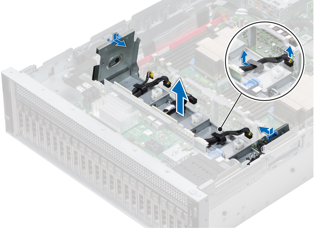
Rakam 35. Fan tepsisini çıkarma
