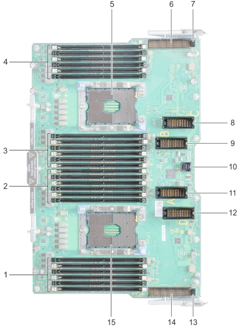
Rakam 111. İşlemci genişletme modülü (PEM) konektörleri
