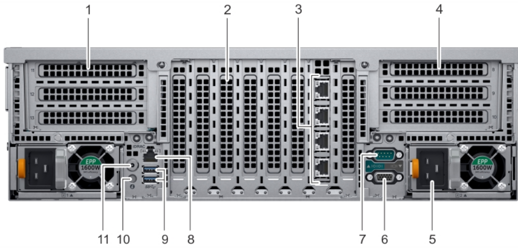
Rakam 8. Arkadan görünüm özellikleri
