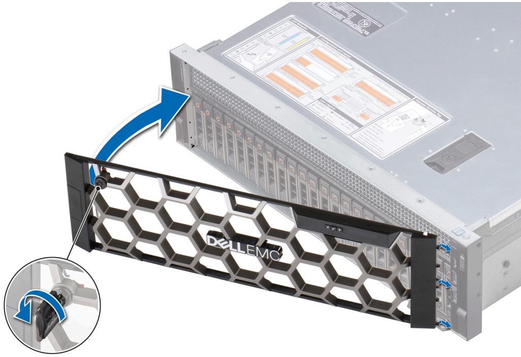
Rakam 22. LCD panelli isteğe bağlı ön çerçeveyi takma
