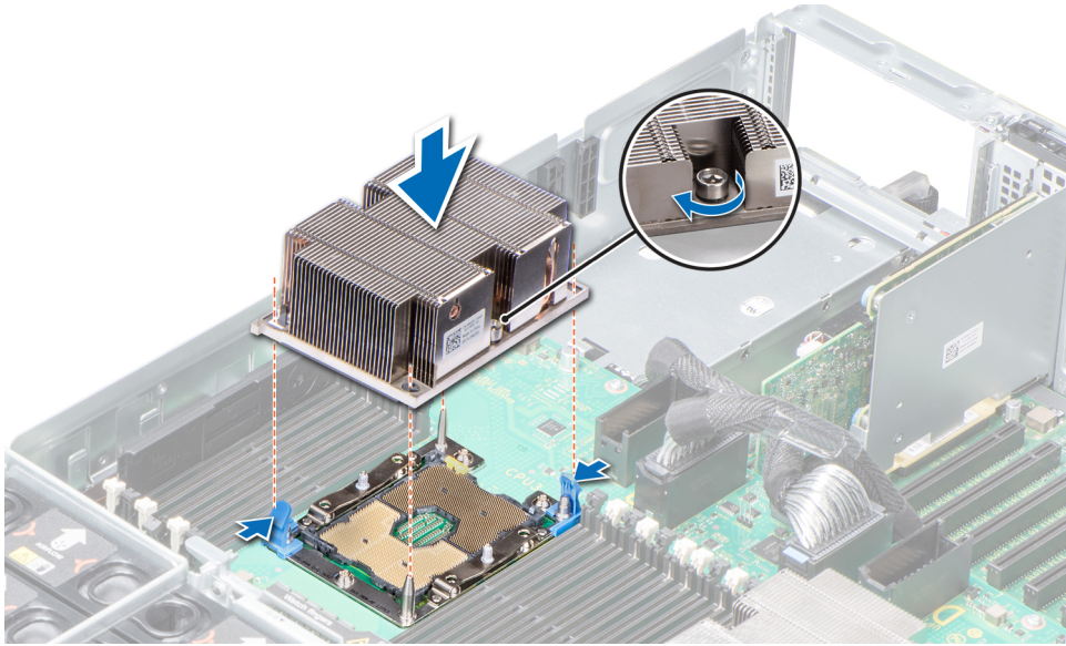
그림 67. 프로세서 및 방열판 모듈 장착
