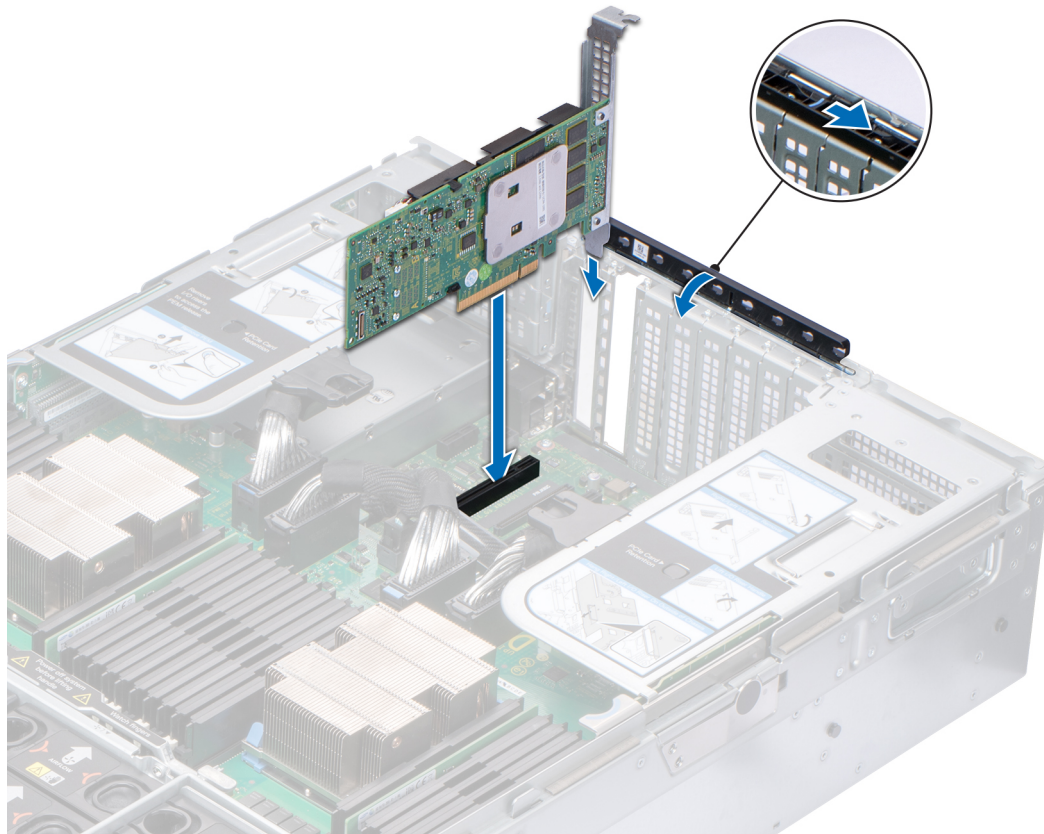
図 89. ストレージコントローラーカードの取り付け
