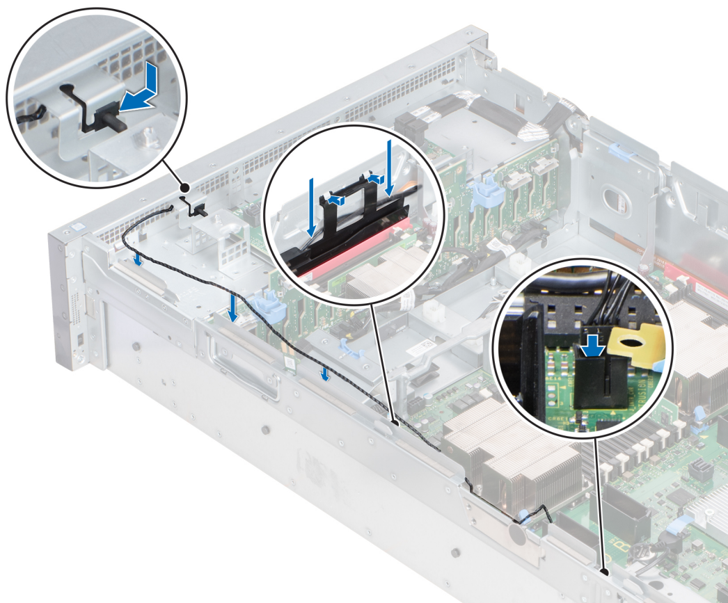
図 38. インテル ジョンスイッチの取り付け
