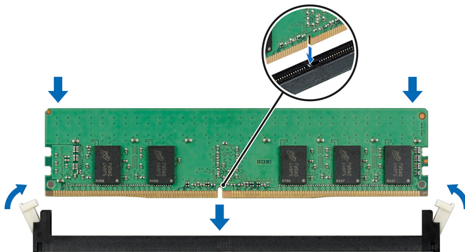
図 60. メモリーモジュールの取り付け
