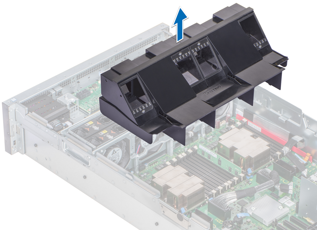
図 27. エアフローカバーの取り外し — 2プロセッサシステム
