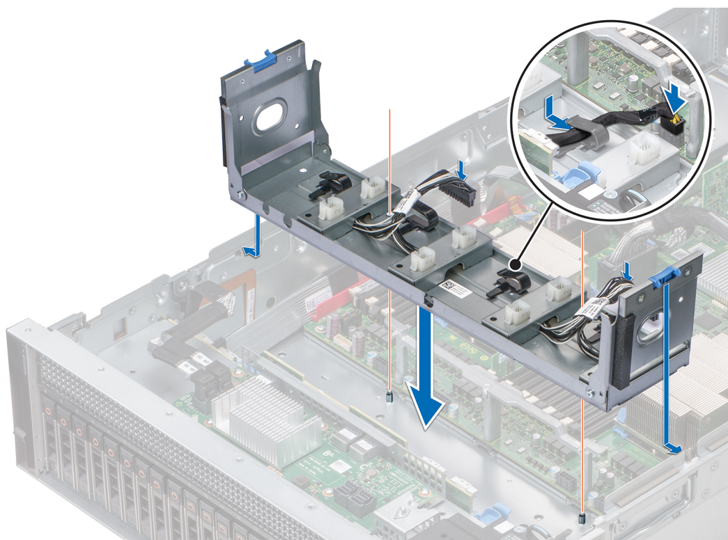
図 36. ファントレイの取り付け
