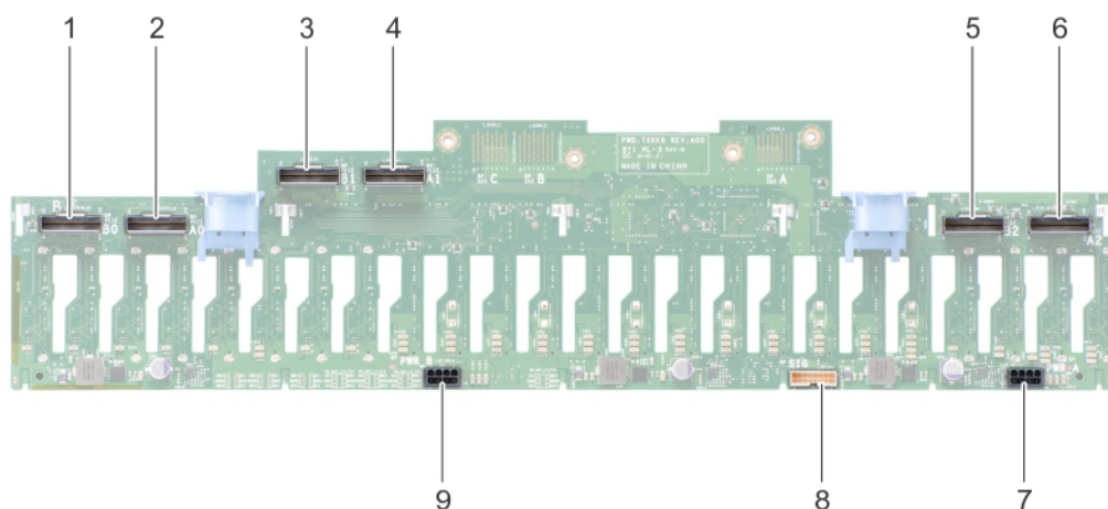
図 45. 24x2.5 インチ ドライブ バックプレーンのコネクタ
