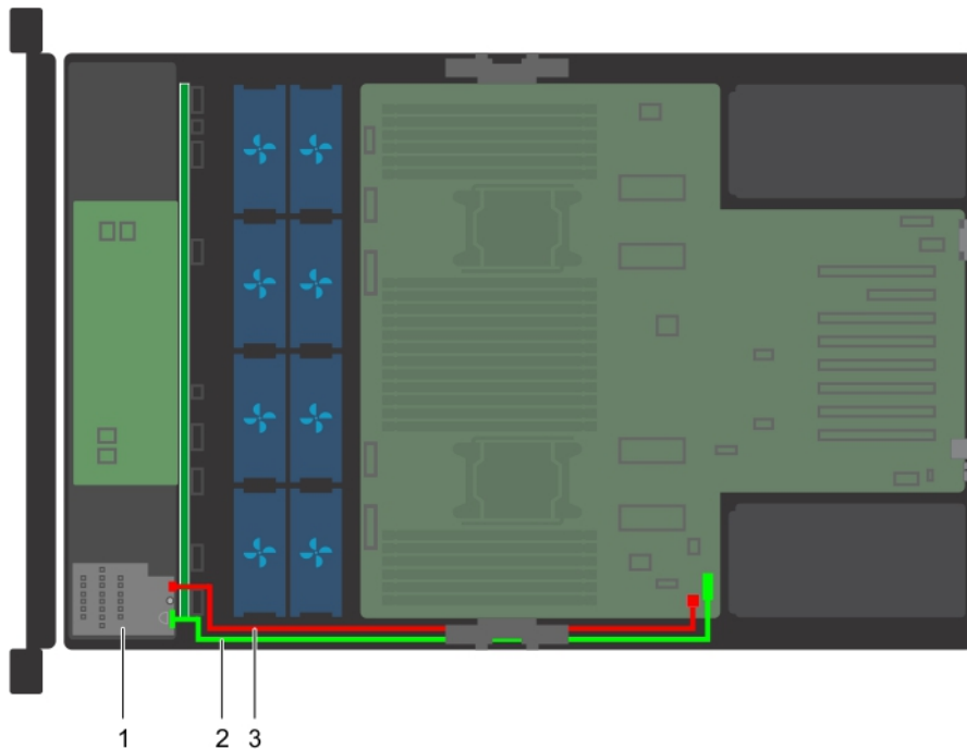
Abbildung 100. Kabelführung – NVDIMM-Batteriekabel
