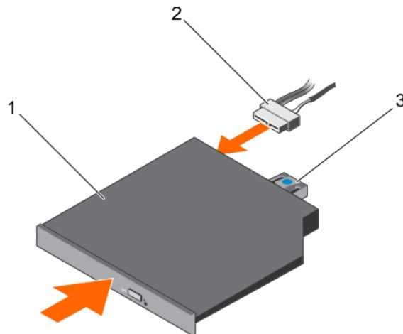
Ilustración 78. Instalación de la unidad óptica opcional
