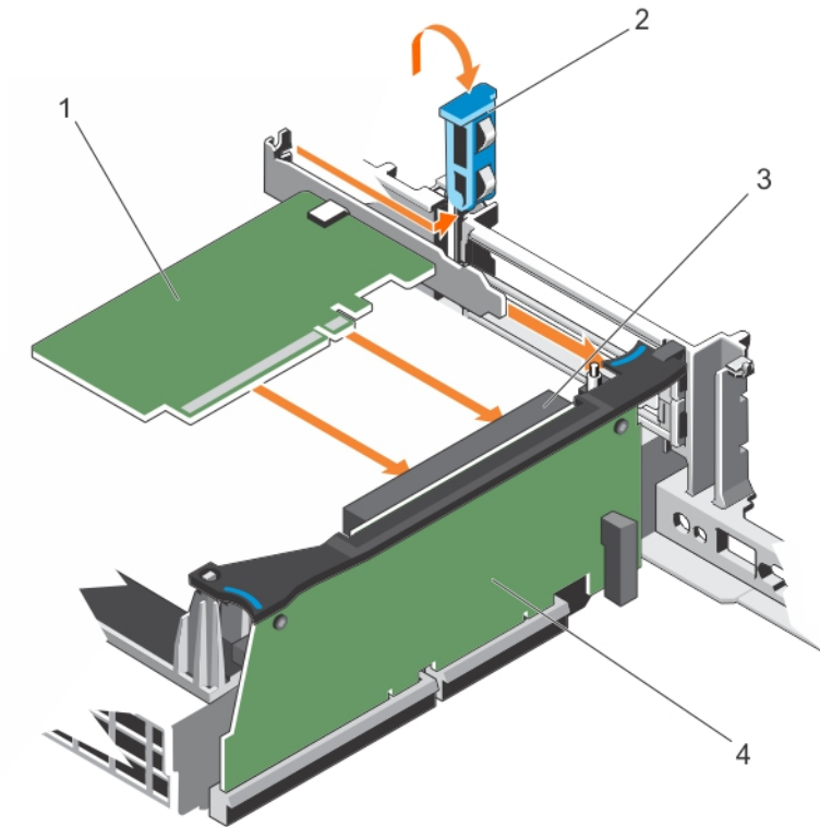
Ilustración 59. Instalación de una tarjeta de expansión de altura media en el soporte vertical para tarjetas de expansión 3
