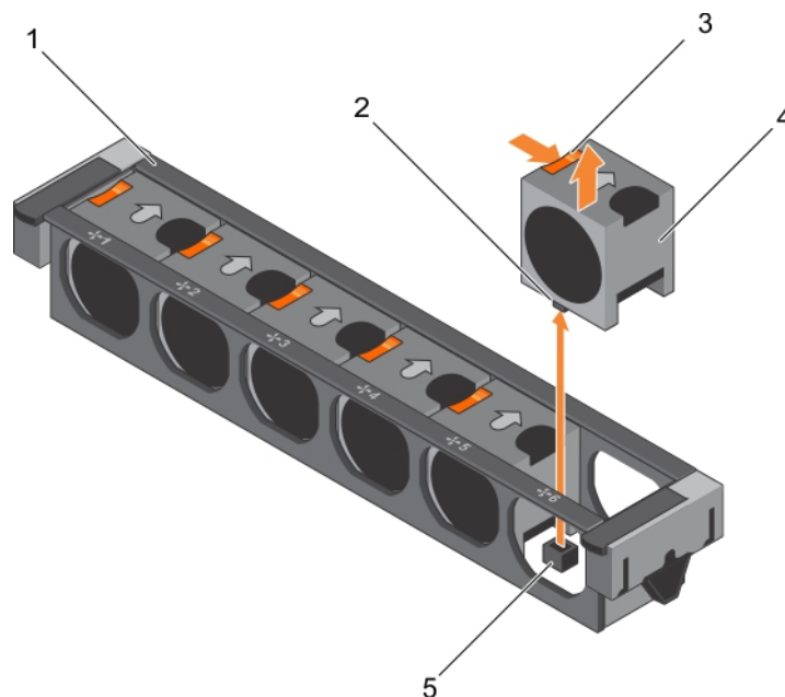
Ilustración 25. Extracción de un ventilador de enfriamiento
