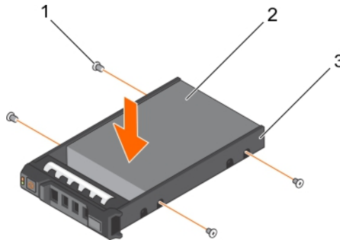
Ilustración 76. Instalación de una unidad de disco duro en un portaunderidades de disco duro
