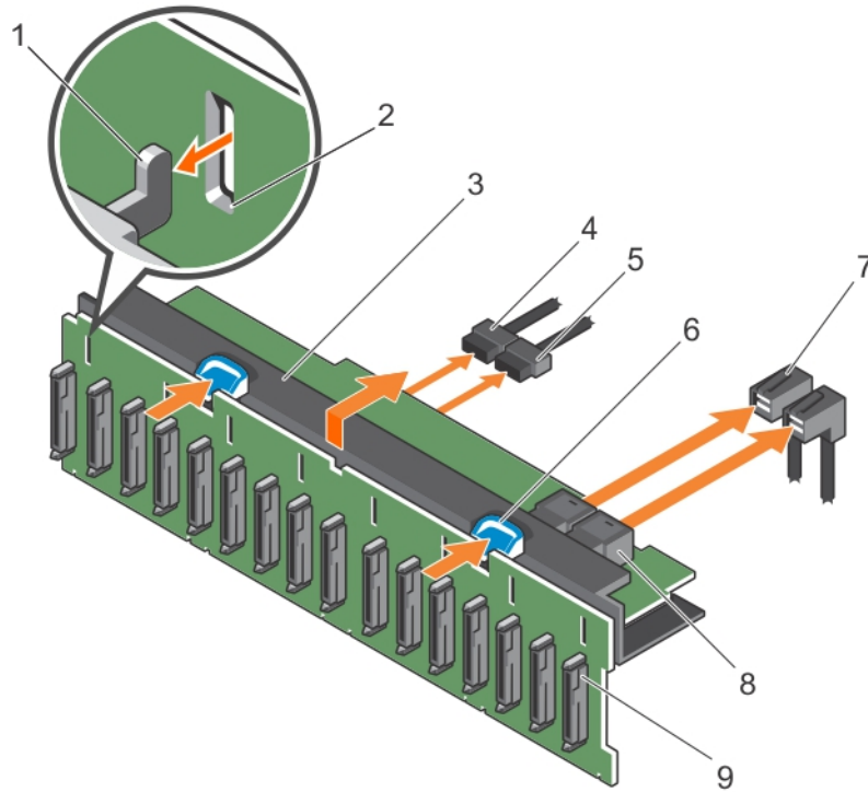
Ilustración 81. Extracción del backplane de SAS/SATA de 2.5 pulgadas (x16)
