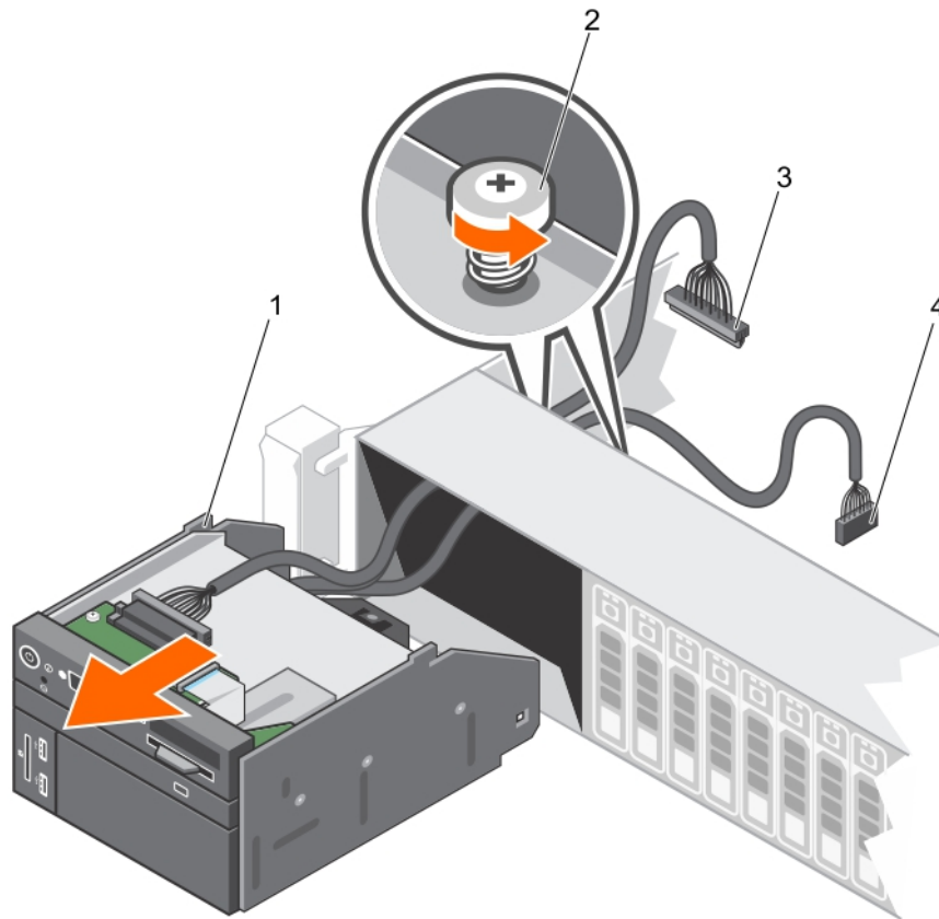
Ilustración 87. Extracción del panel de control
