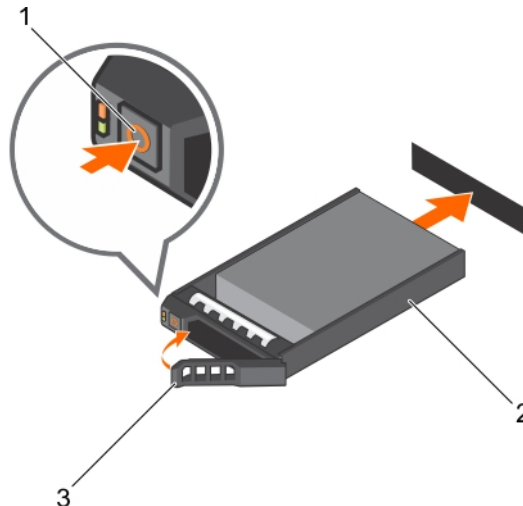
Ilustración 72. Instalación de una SSD o unidad de disco duro de intercambio directo
