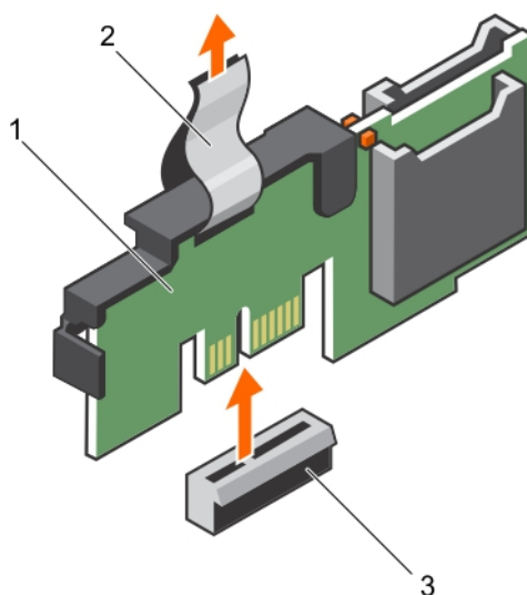
Ilustración 63. Extracción del módulo SD dual interno (IDSDM)
