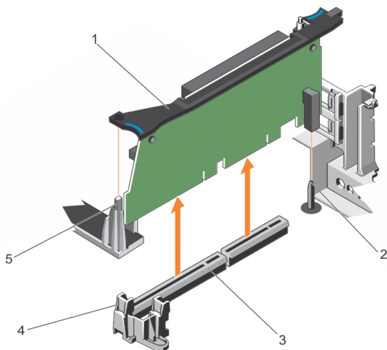
Ilustración 48. Extracción del soporte vertical para tarjetas de expansión 3
