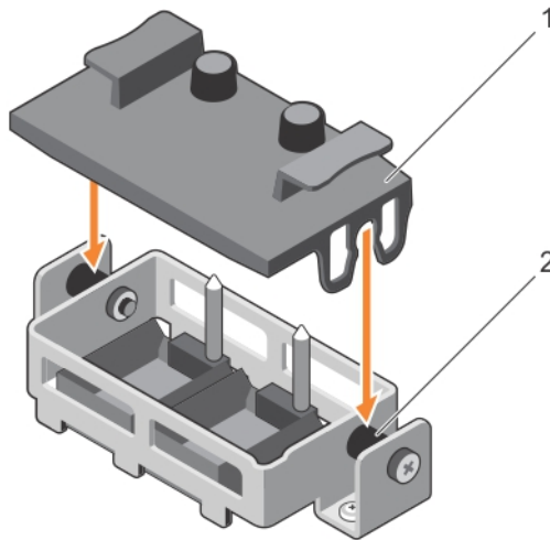
Ilustración 19. Instalación del soporte de relleno en el conector QPI
