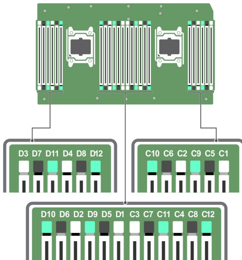
Ilustración 29. Ubicaciones de los zócalos de memoria en el módulo de expansión del procesador
