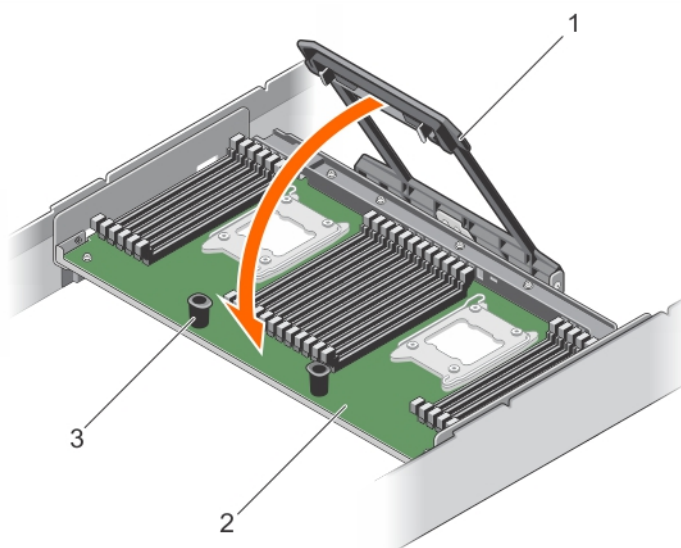
Ilustración 22. Fijar el PEM en el chasis por medio de la palanca de liberación
