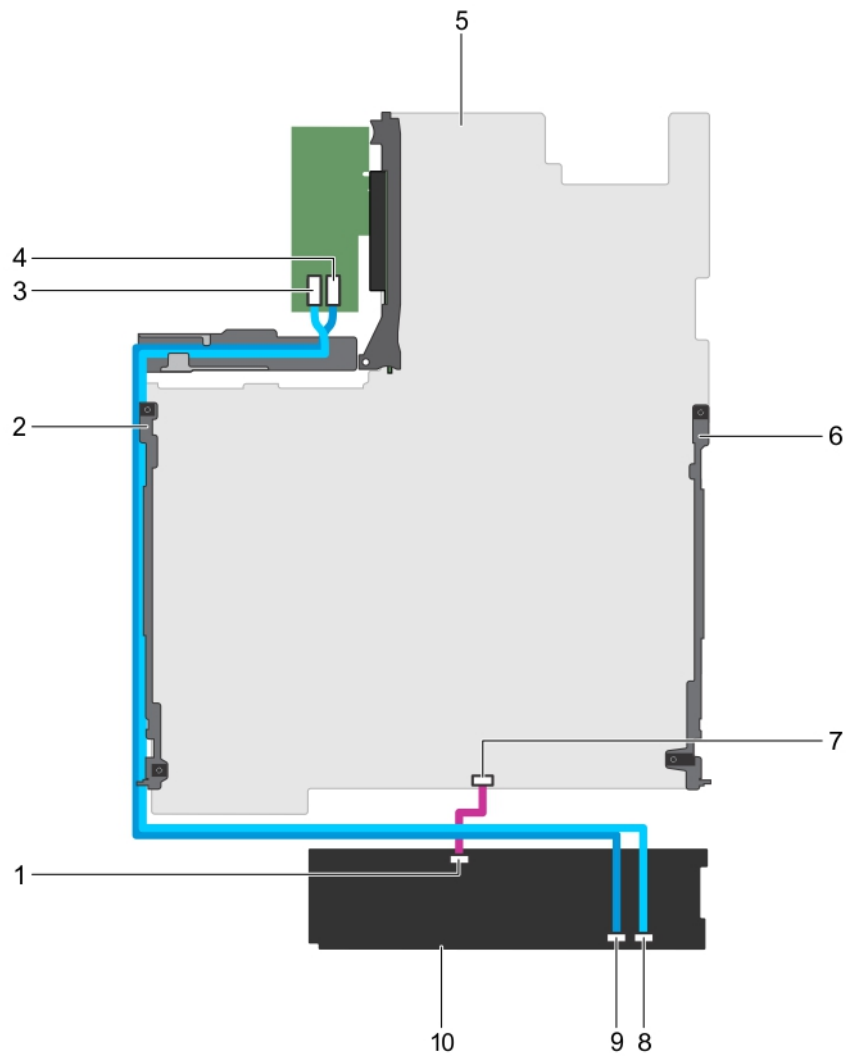
Ilustración 82. Diagrama de cableado: backplane de SAS/SATA de 2.5 pulgadas (x16)
