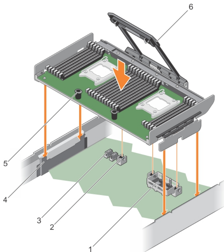
Ilustración 21. Instalación del PEM
