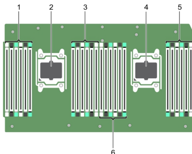
Ilustración 97. Conectores del módulo de expansión del procesador
