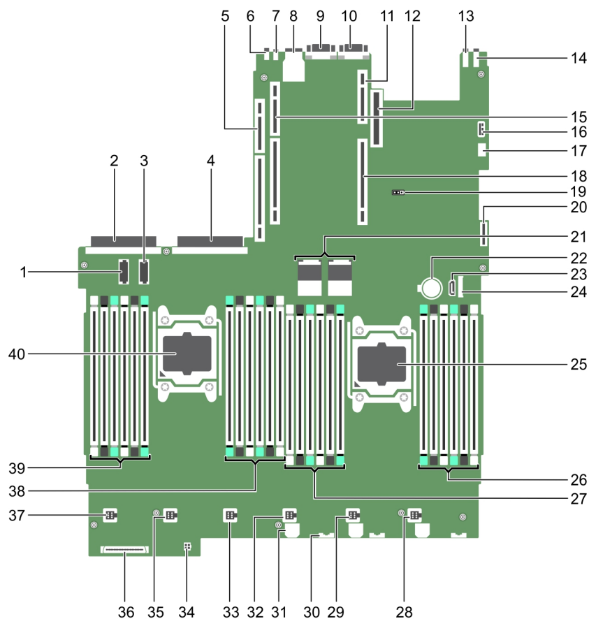
Ilustración 96. Conectores de la tarjeta madre
