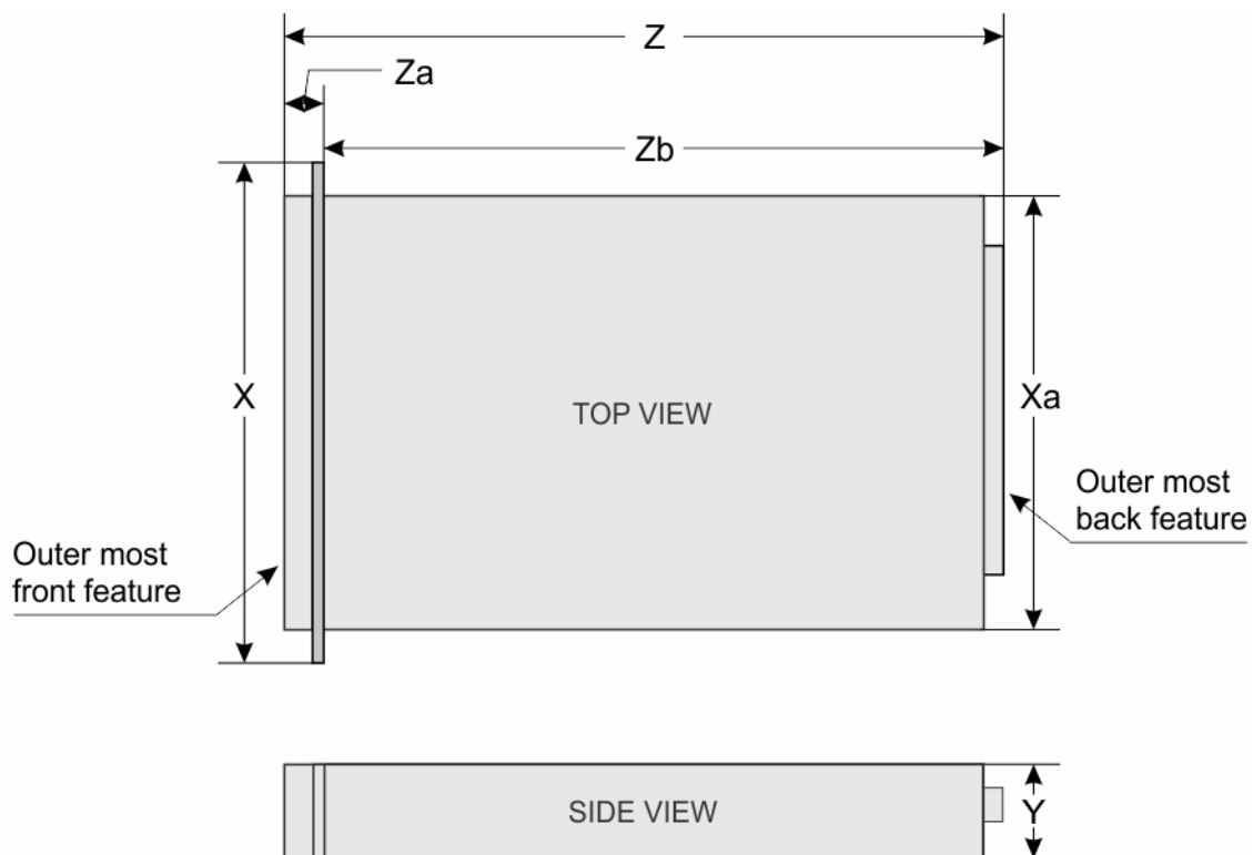
Ilustración 10. Dimensiones del sistema PowerEdge R830
