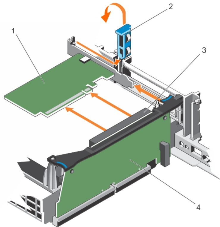
Ilustración 57. Extracción de una tarjeta de expansión de altura media del soporte vertical para tarjetas de expansión 3
