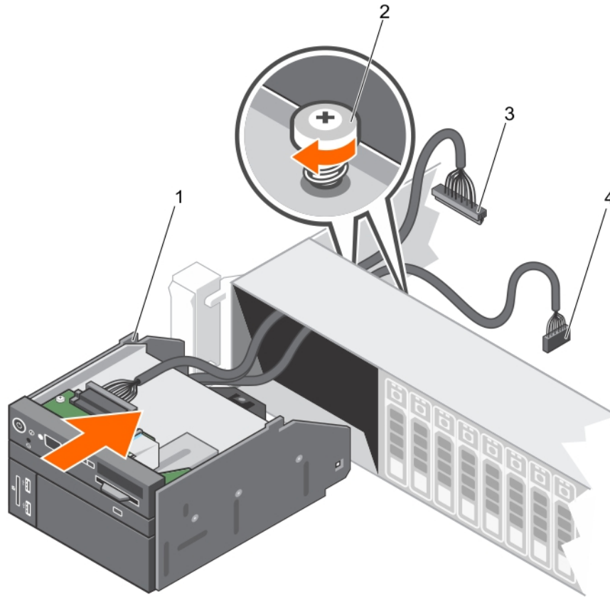
Ilustración 91. Instalación del panel de control
