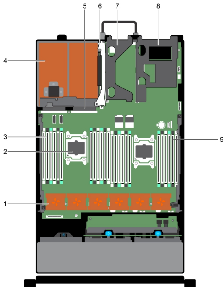
Ilustración 15. Interior del sistema: sistema de procesadores
