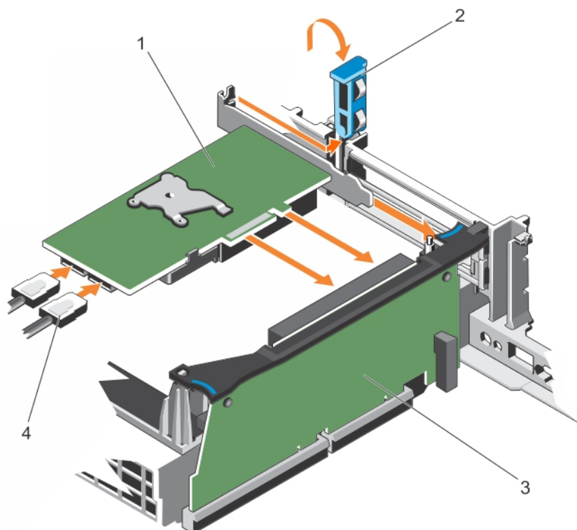
Ilustración 43. Instalación de la tarjeta controladora de almacenamiento integrada
