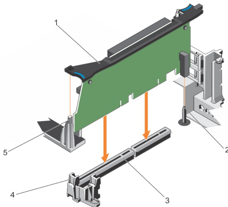
Ilustración 52. Instalación del soporte vertical para tarjetas de expansión 3
