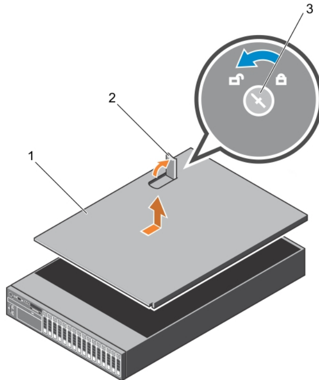
Ilustración 13. Extracción de la cubierta del sistema
