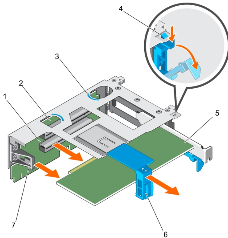
Ilustración 53. Extracción de una tarjeta de expansión del soporte vertical para tarjetas de expansión 1
