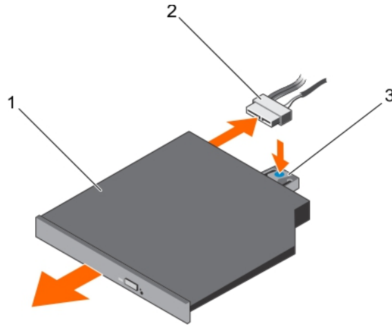
Ilustración 77. Extracción de la unidad óptica opcional
