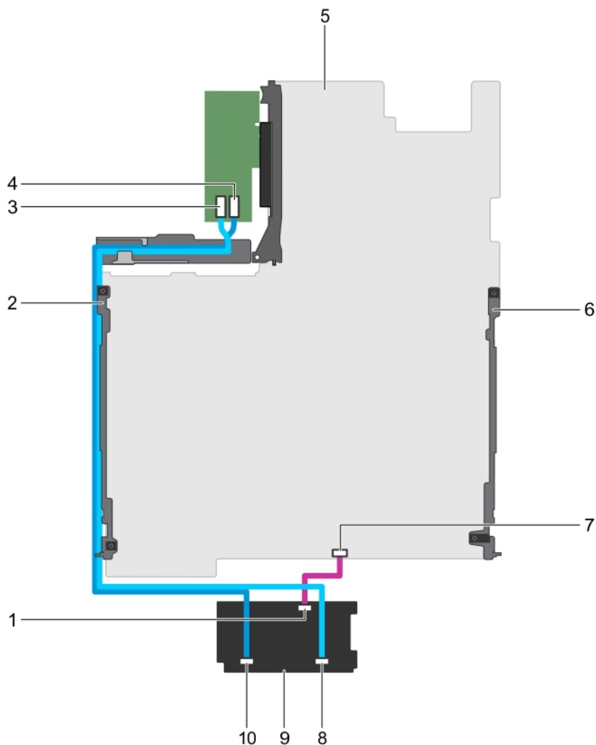
Ilustración 84. Diagrama del cableado: backplane SAS/SATA (x8) de 2,5 pulgadas
