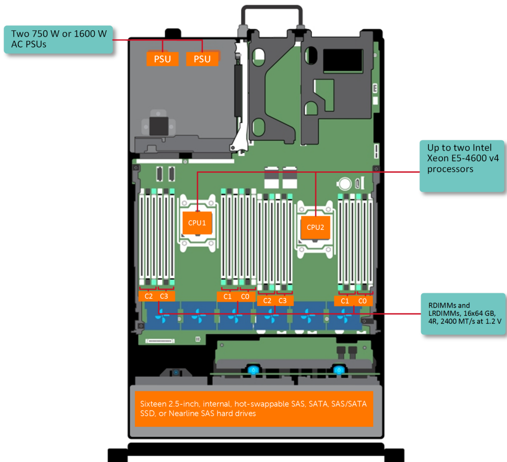
Ilustración 1. Configuraciones admitidas para un sistema PowerEdge R830 de dos procesadores
