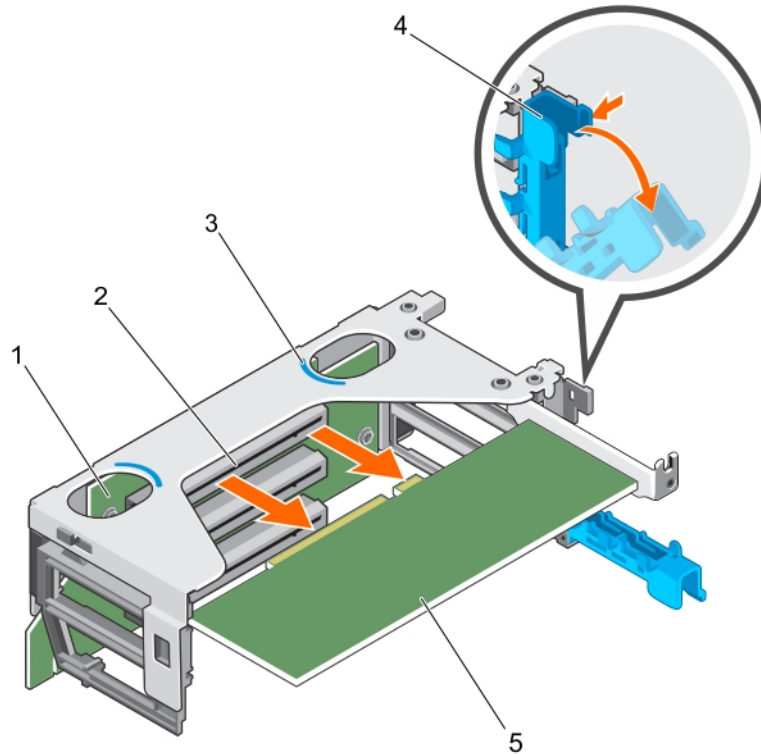
Ilustración 55. Extracción de una tarjeta de expansión del soporte vertical para tarjetas de expansión 2
