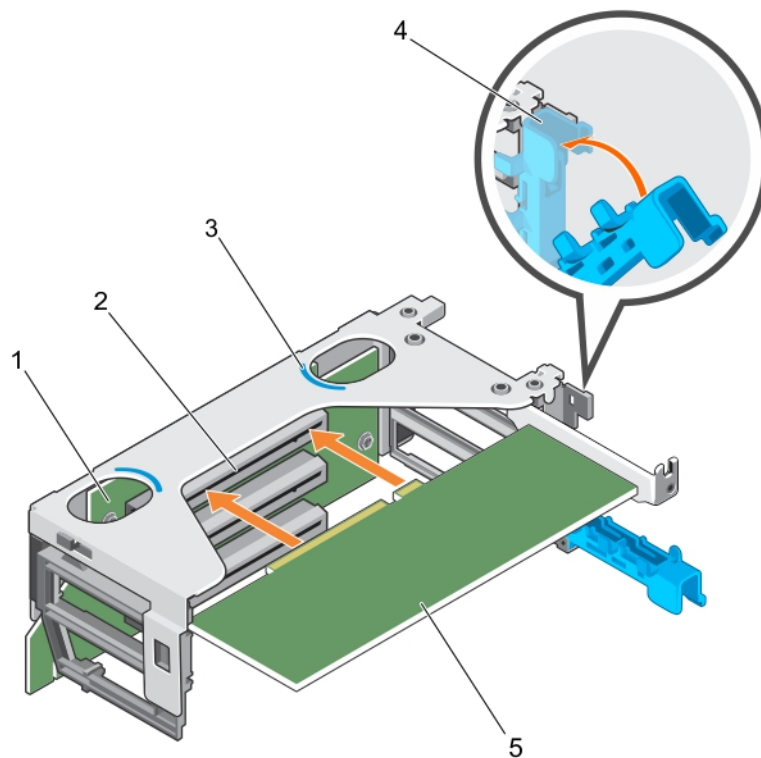
Ilustración 56. Instalación de una tarjeta de expansión en el soporte vertical para tarjetas de expansión 2
