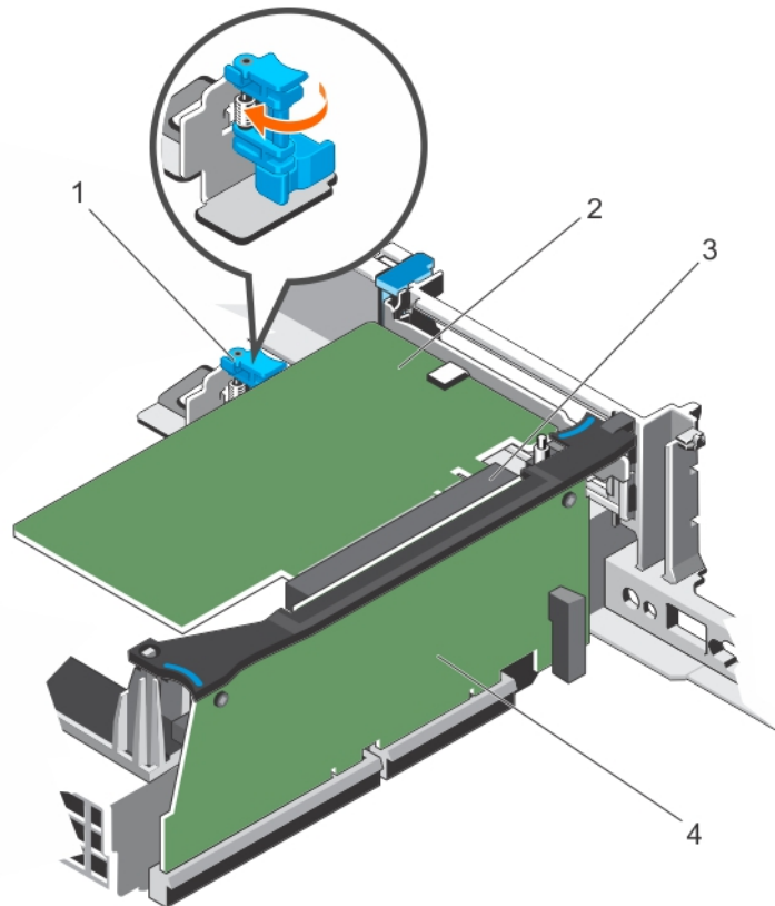
Ilustración 60. Instalación de una tarjeta de expansión de altura completa en el soporte vertical para tarjetas de expansión 3
