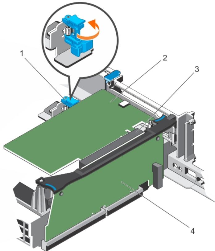
Ilustración 58. Extracción de una tarjeta de expansión de altura completa del soporte vertical para tarjetas de expansión 3
