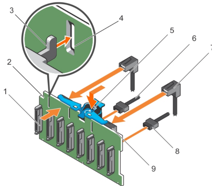
Ilustración 86. Instalación del backplane SAS/SATA (x8) de 2,5 pulgadas
