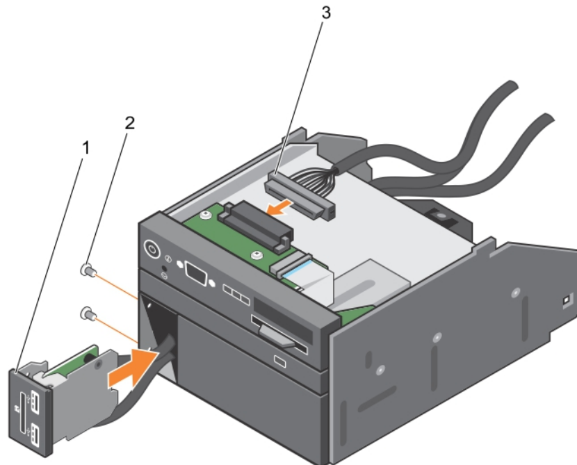
Ilustración 90. Instalación del módulo del conector USB/conector vFlash
