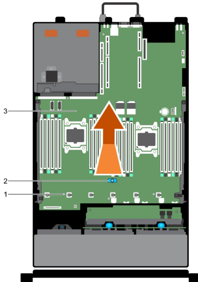
Ilustración 94. Extracción de la tarjeta madre
