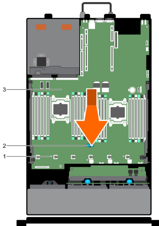
Ilustración 93. Extracción de la tarjeta madre
