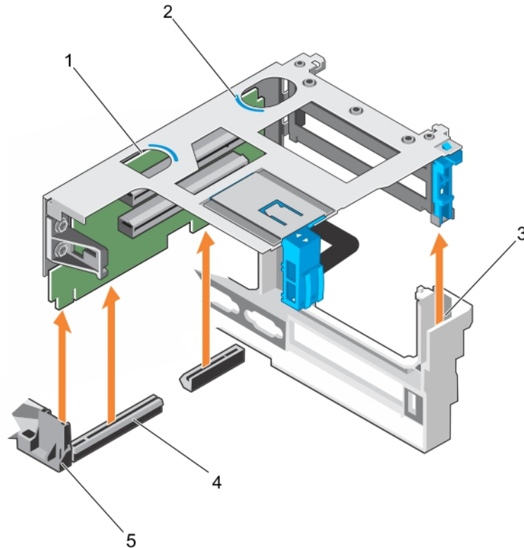
Ilustración 44. Extracción del soporte vertical para tarjetas de expansión 1
