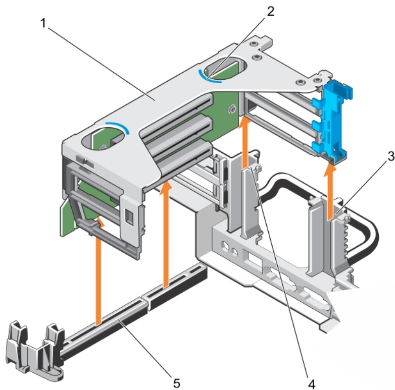
Ilustración 46. Extracción del soporte vertical para tarjetas de expansión 2
