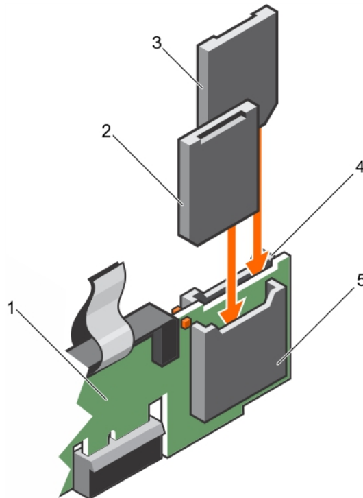
Ilustración 62. Instalación de una tarjeta SD interna
