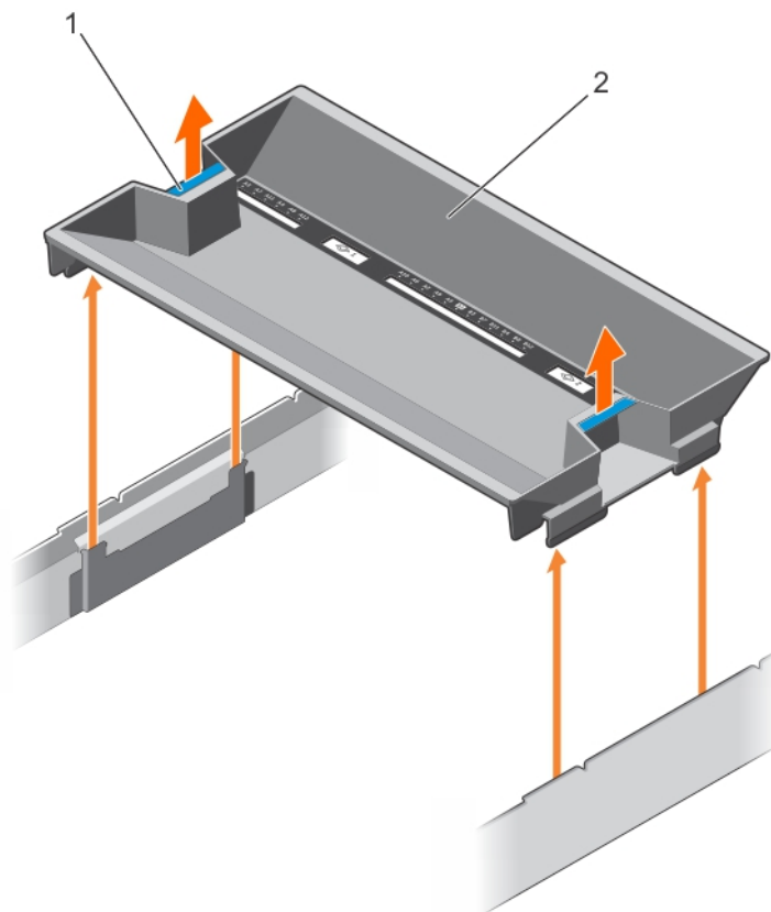
Ilustración 23. Extracción de la cubierta de enfriamiento
