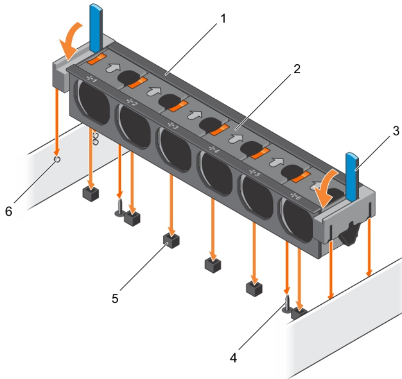
Ilustración 27. Instalación del ensamblaje de ventiladores
