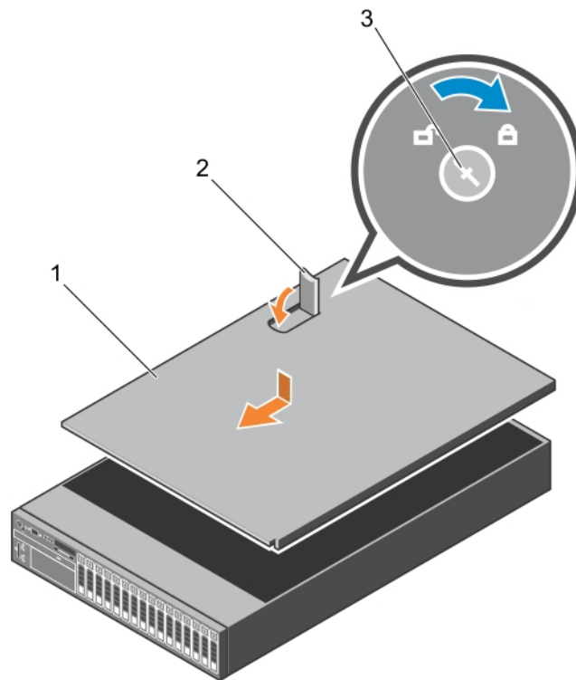
Ilustración 14. Instalación de la cubierta del sistema
