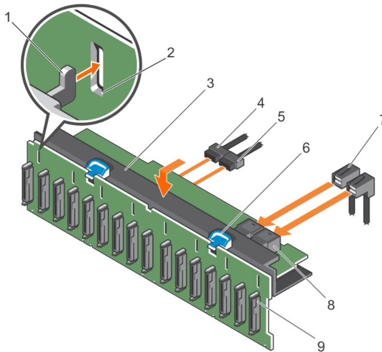
Ilustración 85. Instalación del backplane de SAS/SATA de 2.5 pulgadas (x16)
