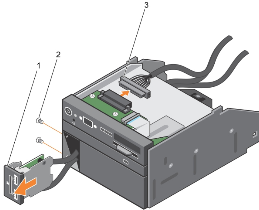
Ilustración 88. Extracción del módulo del conector USB/conector vFlash
