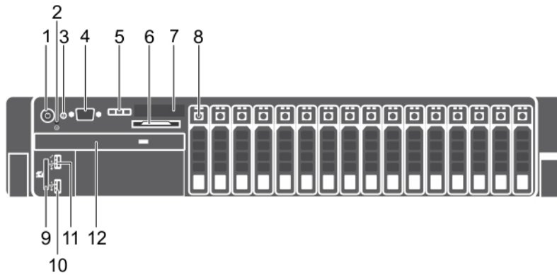
Ilustración 3. Características del panel frontal (chasis de la unidad de disco duro de 2,5 pulgadas)
