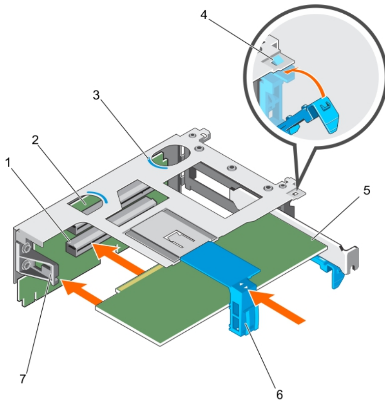
Ilustración 54. Instalación de una tarjeta de expansión en el soporte vertical 1 para tarjetas de expansión
