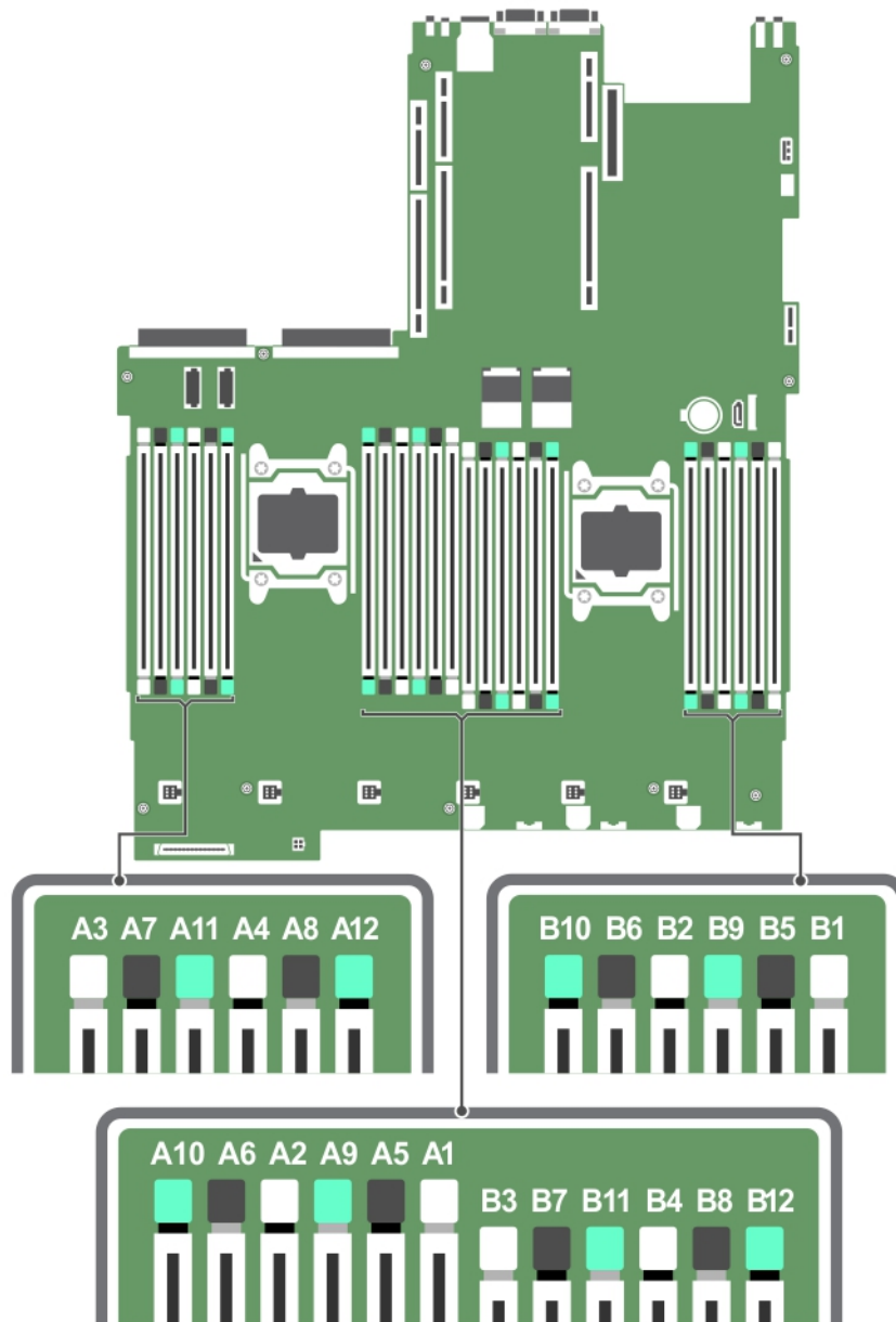
Ilustración 28. Ubicaciones de los sockets de memoria
