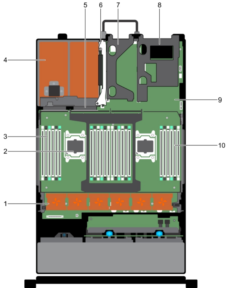
Ilustración 16. Interior del sistema: sistema con cuatro procesadores con módulo de expansión del procesador (PEM)
