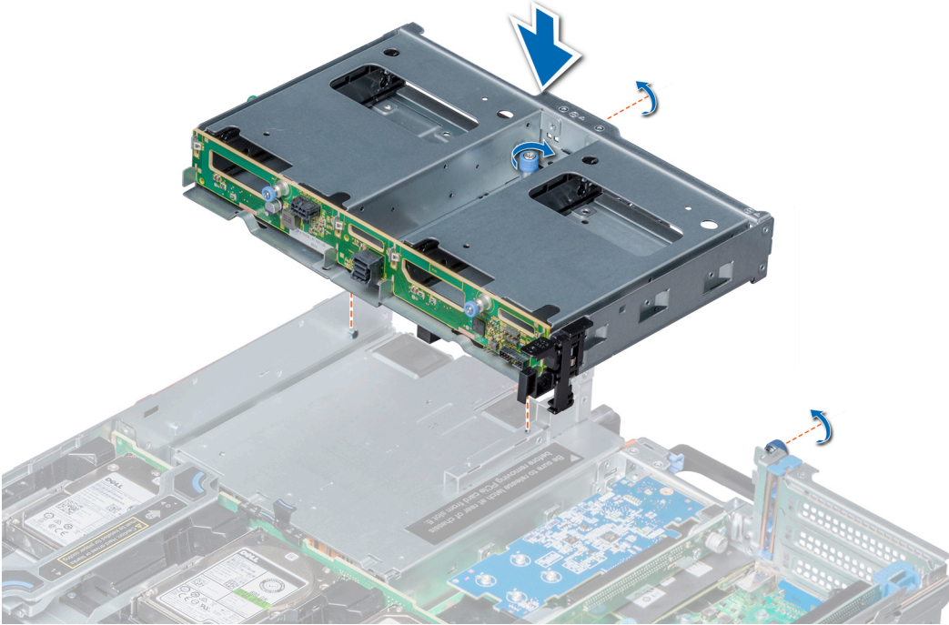
Rakam 68. 2 x 3,5 inç arka sürücü kafesini takma
