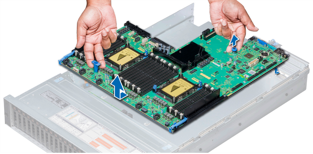
Rakam 171. Sistem kartını çıkarma
