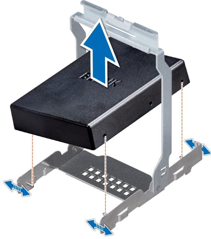
Rakam 47. Orta sürücü taşıyıcısından sürücü kasasını çıkarma
