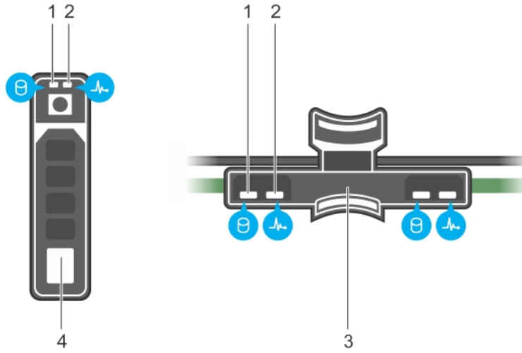
Rakam 13. Sürücü ve orta sürücü tepsisi arka paneli üzerindeki sürücü göstergeleri
