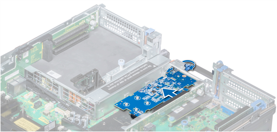
Rakam 83. Genişletme kartını genişletme kartı yükselticisi 2B'den çıkarma
