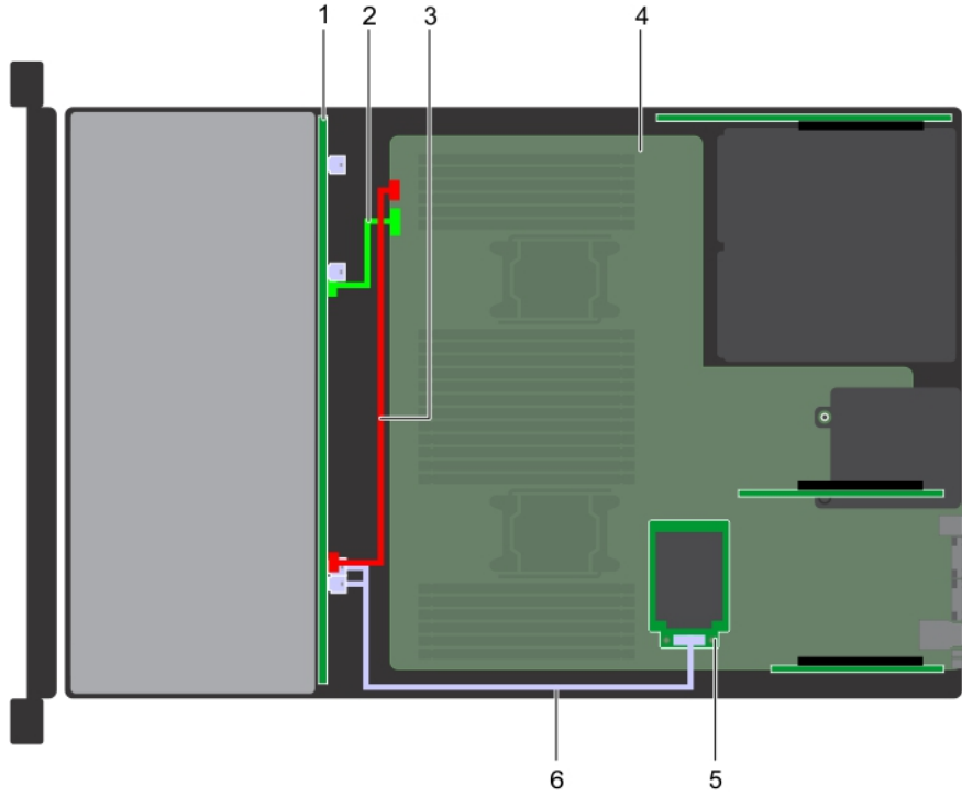
Rakam 155. Kablo yerleşimi - mini PERC'li 12 x 3,5 inç sürücü arka paneli
