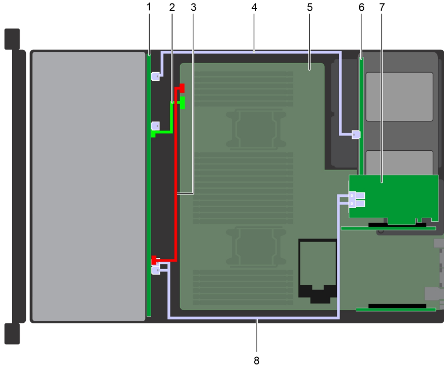
Rakam 145. Kablo yerleşimi – Adaptör PERC11/HBA'lı 4 x 2,5 inç arka sürücü arka paneli ile 12 x 3,5 inç sürücü arka paneli
