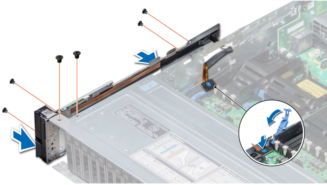
Rakam 175. Sol kontrol panelini takma
