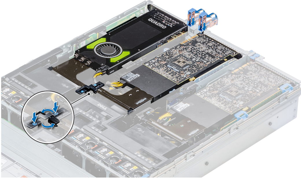
Rakam 111. GPU 2 ve 3'ü sabitleme
