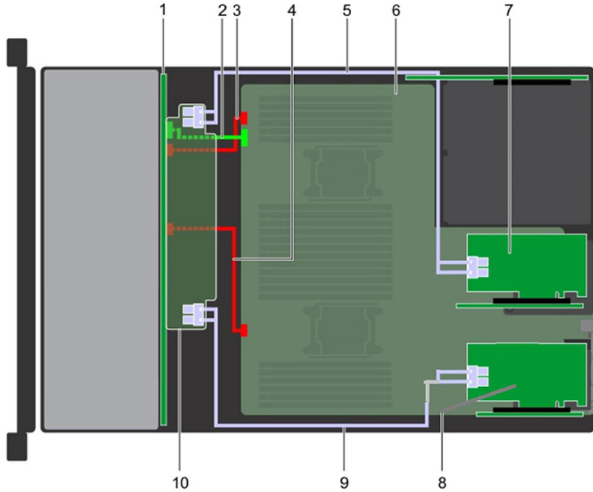
Rakam 139. Kablo yerleşimi - çift adaptör PERC11/HBA'lı 24 x 2,5 inç sürücü arka paneli
