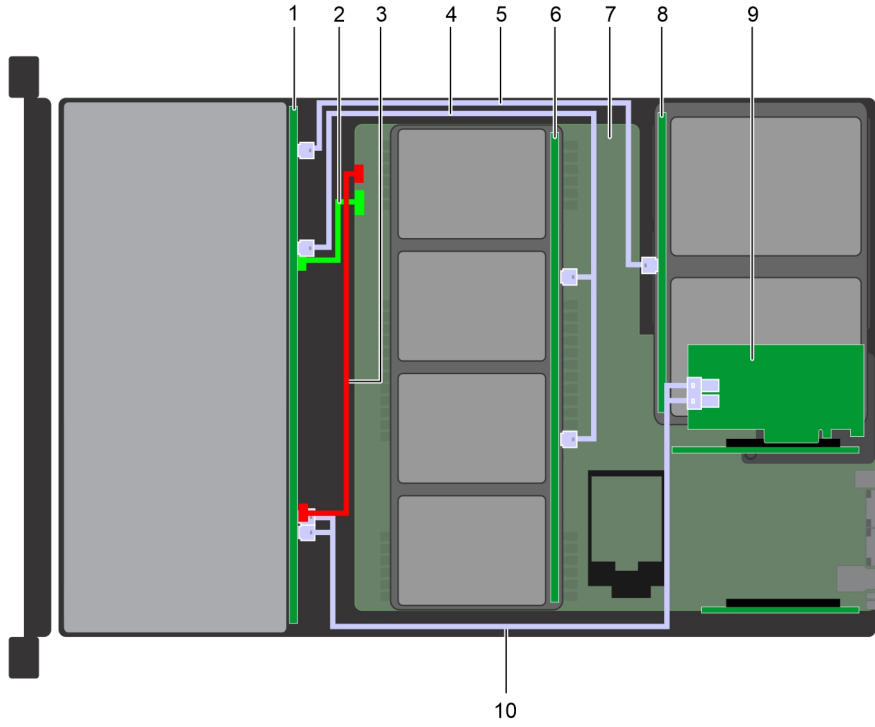
Rakam 144. Kablo yerleşimi – 4 x 3,5 inç (4 x 2,5 inç adaptör) orta sürücü tepsisi arka paneli ve adaptör PERC11/HBA'lı 2 x 3,5 inç arka sürücü arka paneliyle 12 x 3,5 inç sürücü arka paneli
