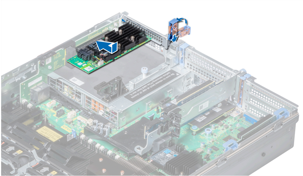
Rakam 89. Genişletme kartını genişletme kartı yükselticisi 3'e takma
