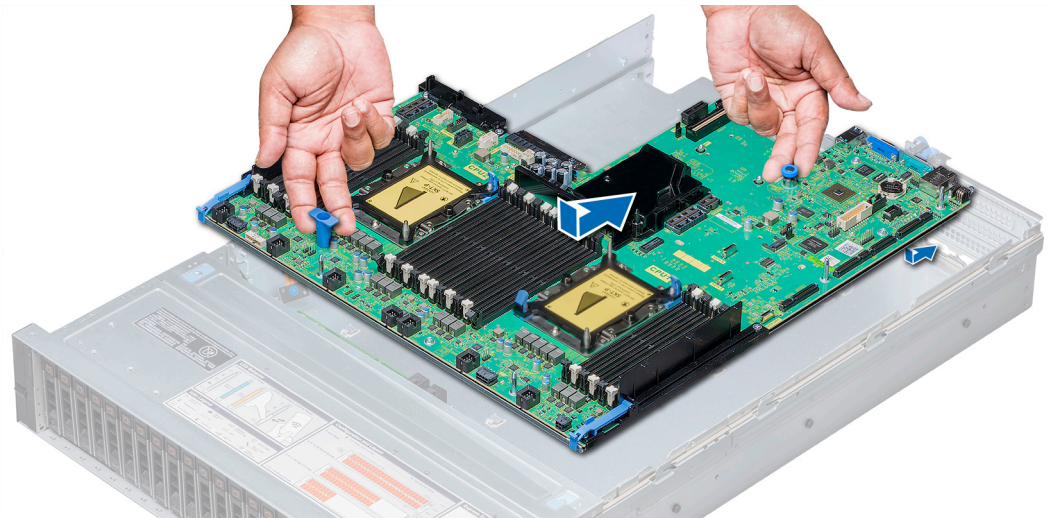
Rakam 172. Sistem kartını takma
