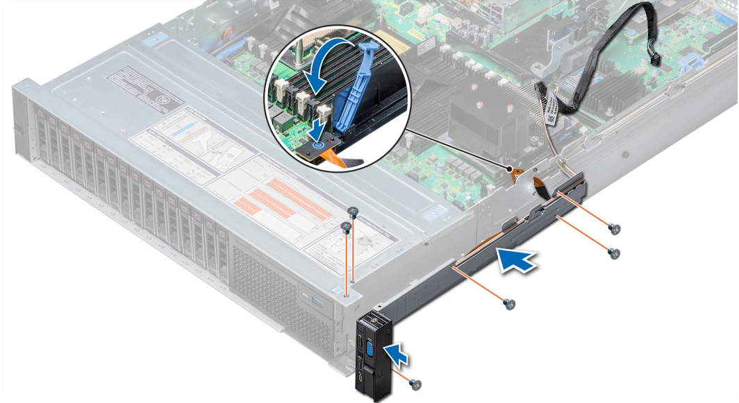
Rakam 177. Sađ kontrol panelini takma
