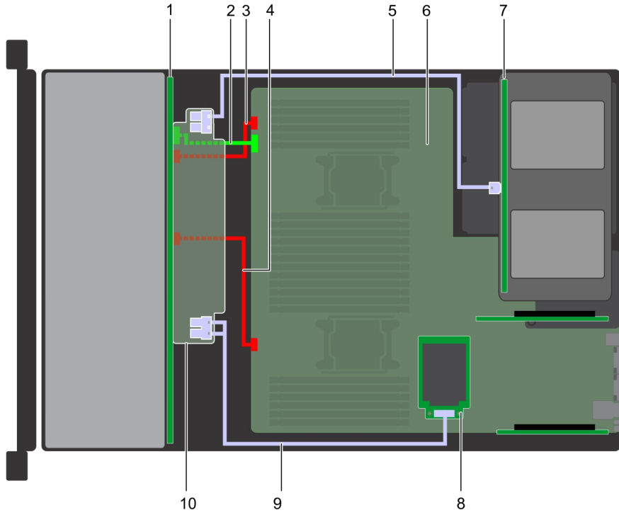
Rakam 151. Kablo yerleşimi - 4 x 2,5 inç arka sürücü arka paneli ile 24 x 2,5 inç sürücü arka paneli
