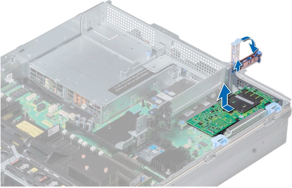
Rakam 82. Genişletme kartını genişletme kartı yükselticisi 1'den çıkarma
