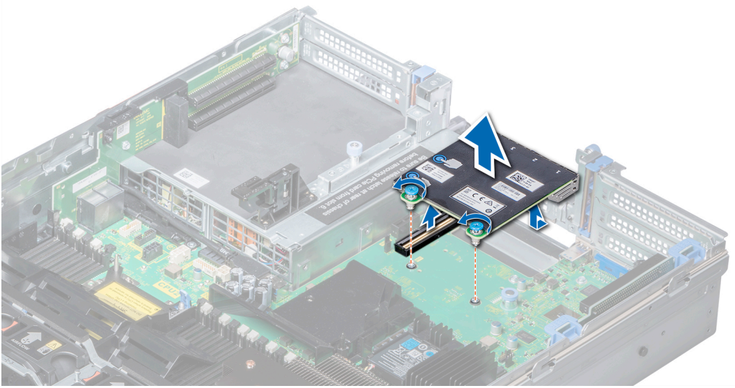
Rakam 118. Ağ ek kartını çıkarma
