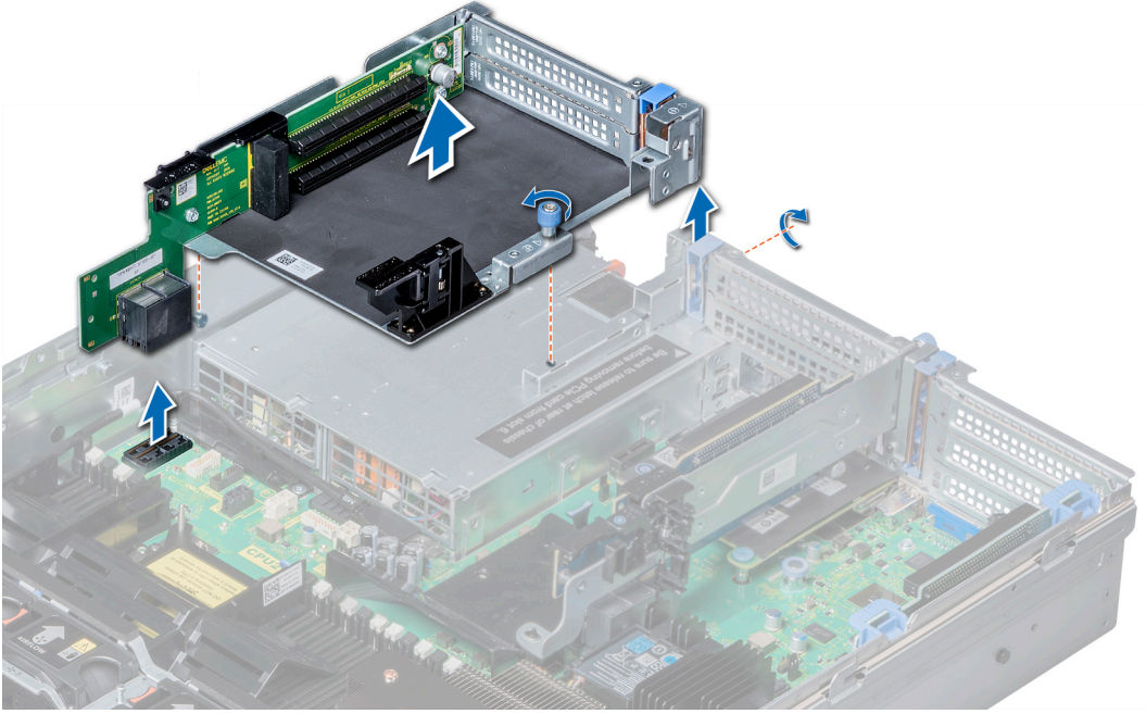
Rakam 100. Geniřletme kartı yükselticisi 3'ü çıkarma
