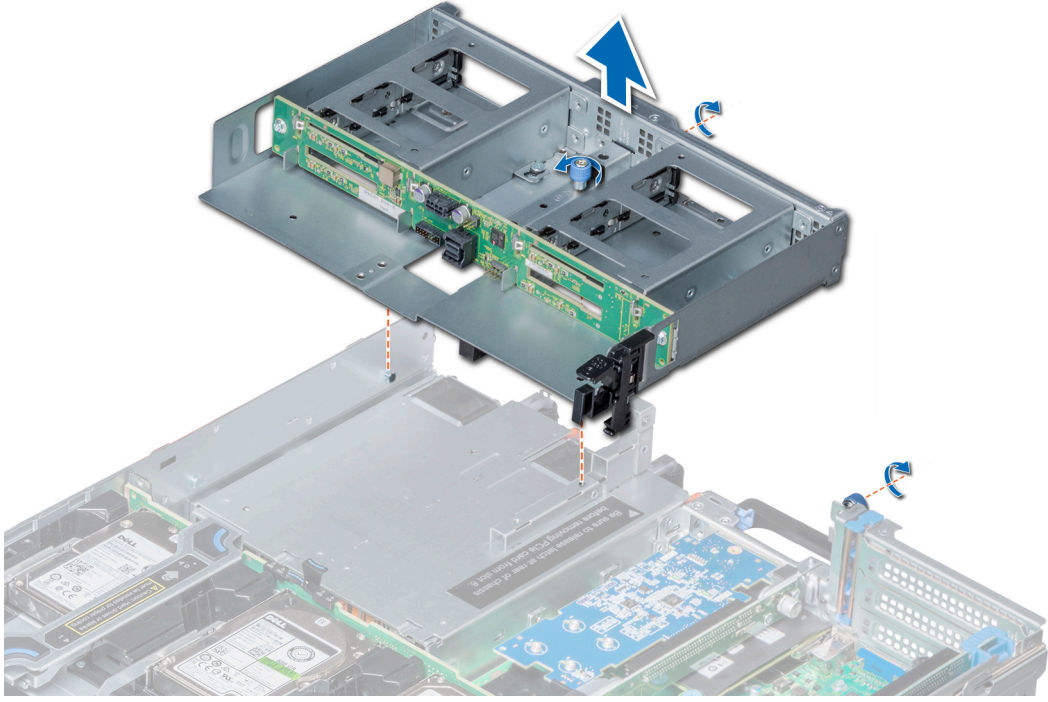
Rakam 65. 4x 2,5 inç arka sürücü kafesini çıkarma
