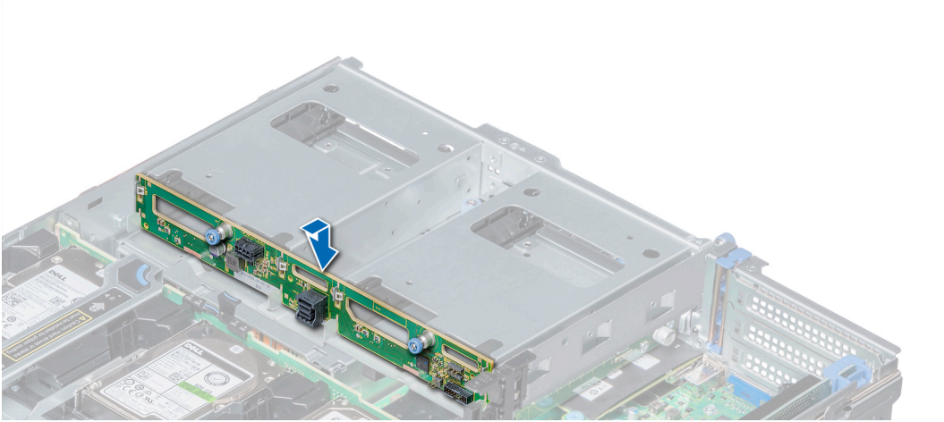
Rakam 136. 3,5 inç sürücü arka panelini takma
