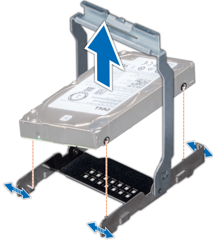
Rakam 51. 3,5 inç sürücüyü sürücü taşıyıcısından çıkarma
