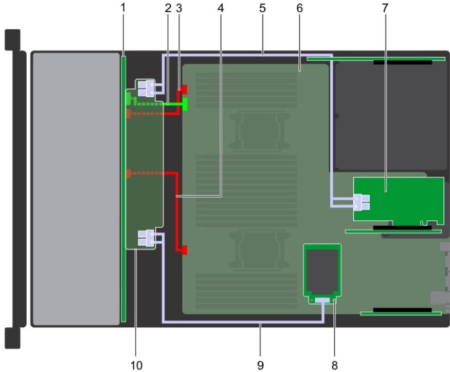
Rakam 149. Kablo yönlendirmesi - mini PERC/HBA'lı ve adaptör PERC/HBA'lı 24 x 2,5 inç sürücü arka paneli
