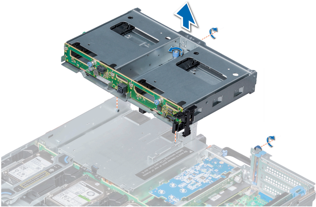
Rakam 66. 2 x 3,5 inç sürücü arka kafesini çıkarma
