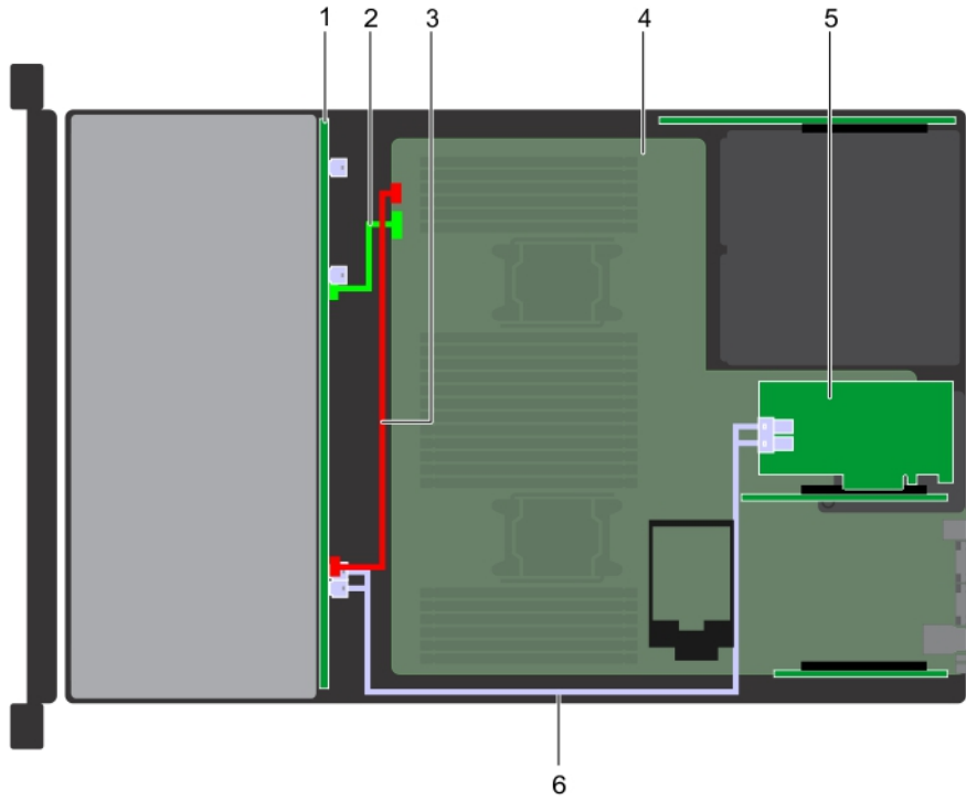
Rakam 156. adaptör PERC'li 12 x 3,5 inç sürücü arka paneli
