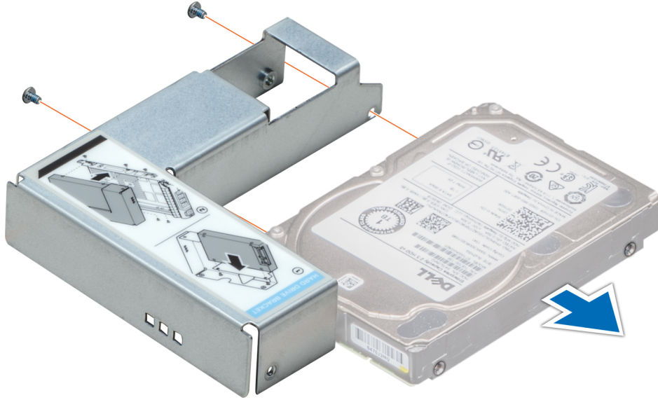
Rakam 59. 2,5 inç sürücüyü 3,5 inç sürücü adaptöründen çıkarma
