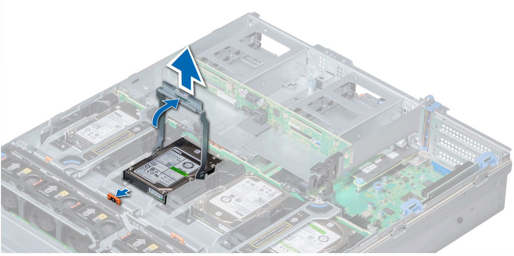
Rakam 49. Sürücü taşıyıcısını orta sürücü tepsisinden çıkarma
