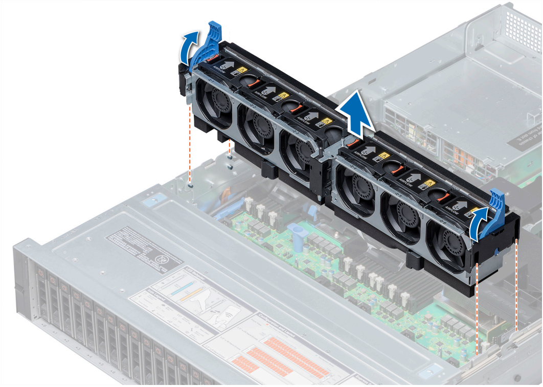
Rakam 33. Soğutma fanı aksamını çıkarma
