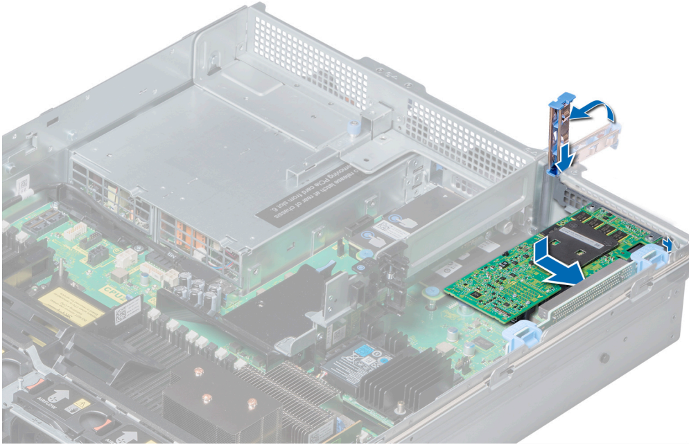
Rakam 86. Genişletme kartını genişletme kartı yükselticisi 1'e takma
