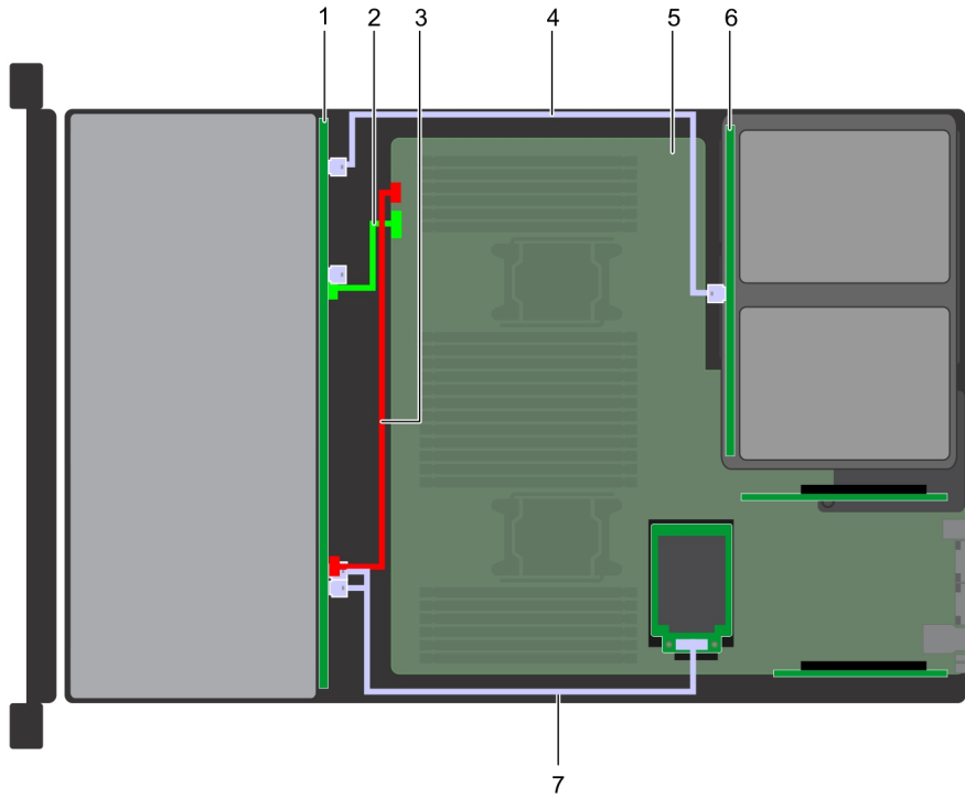
Rakam 159. Kablo yerleşimi - 2 x 3,5 inç arka sürücü arka paneli ile 12 x 3,5 inç sürücü arka paneli
