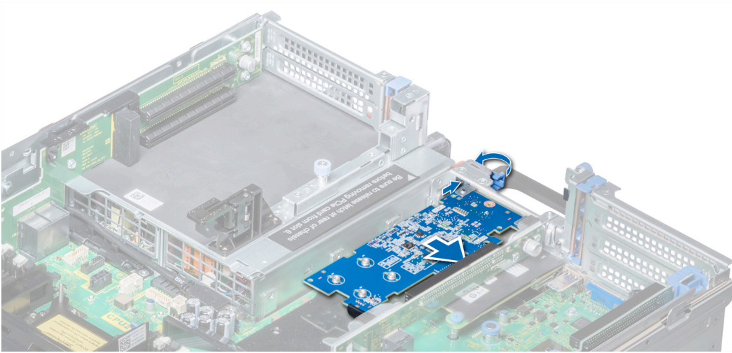
Rakam 87. Genişletme kartını genişletme kartı yükselticisi 2B'ye takma
