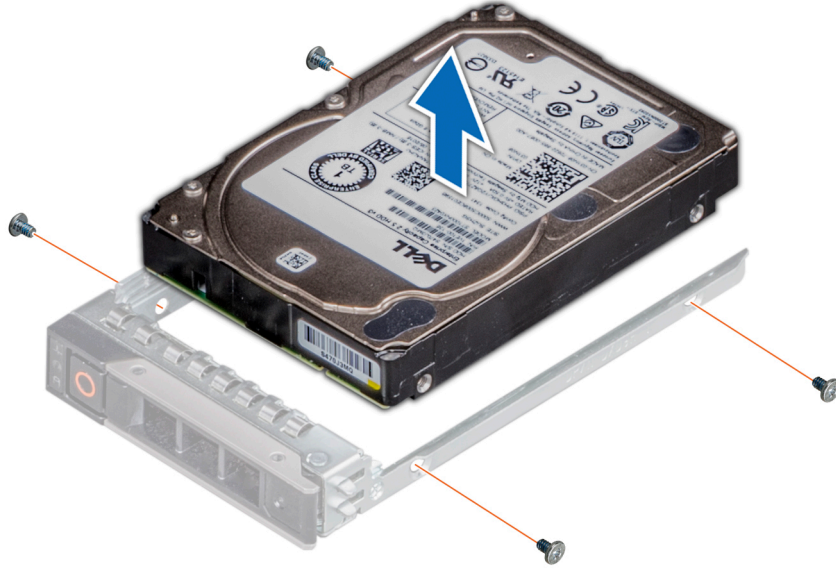
Rakam 63. Sürücü kutusundan sürücüyü çıkarma
