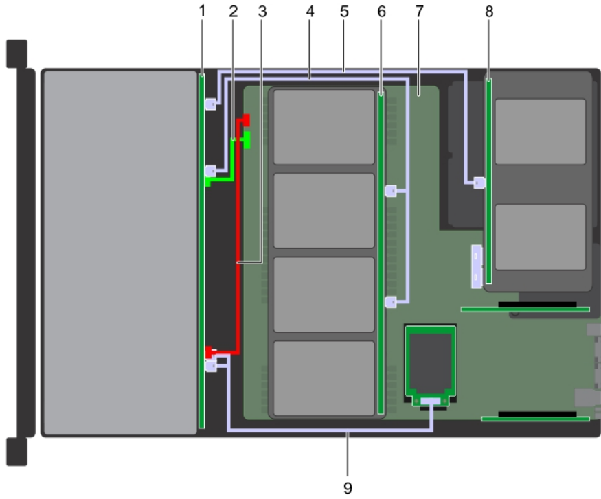
Rakam 158. Kablo yerleşimi – 4 x 3,5 inç (4 x 2,5 inç adaptör) orta sürücü tepsisi arka paneli ve 4 x 2,5 inç arka sürücü arka paneliyle 12 x 3,5 inç sürücü arka paneli
