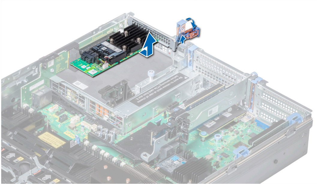
Rakam 85. Genişletme kartını genişletme kartı yükselticisi 3'ten çıkarma
