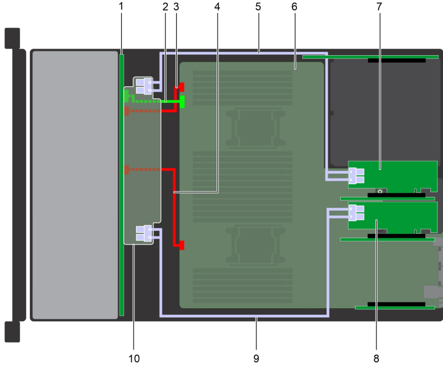
Rakam 140. Kablo yerleşimi - çift adaptör PERC11/HBA'lı 24 x 2,5 inç sürücü arka paneli
