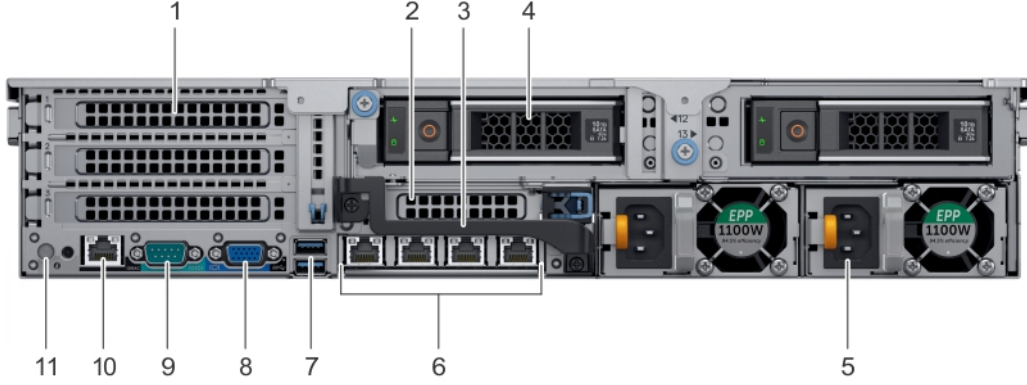
Rakam 9. 2 x 3,5 inç sürücü sisteminin arkadan görünümü
