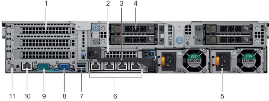
Rakam 8. 4 x 2,5 inç sürücü sisteminin arkadan görünümü
