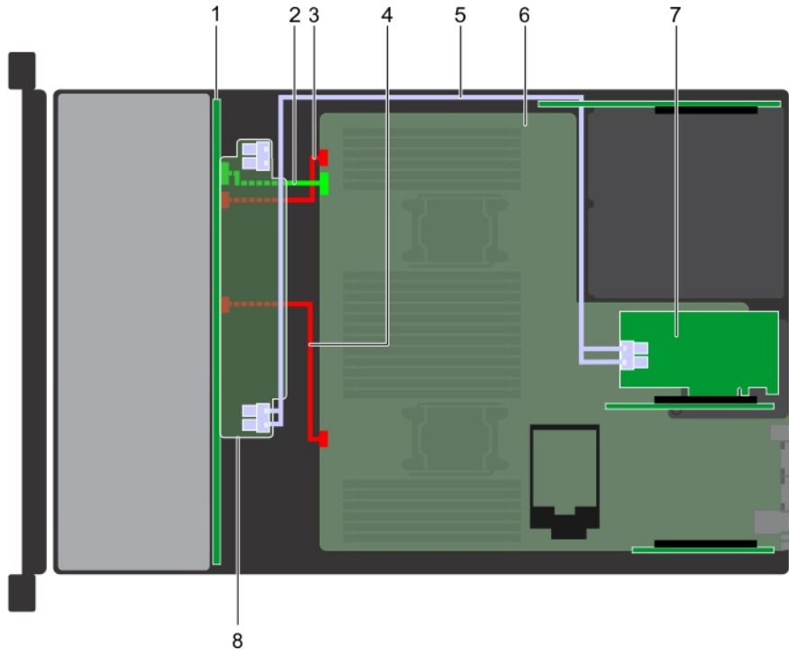
Rakam 148. Kablo yerleşimi - adaptör PERC'li 24 x 2,5 inç sürücü arka paneli
