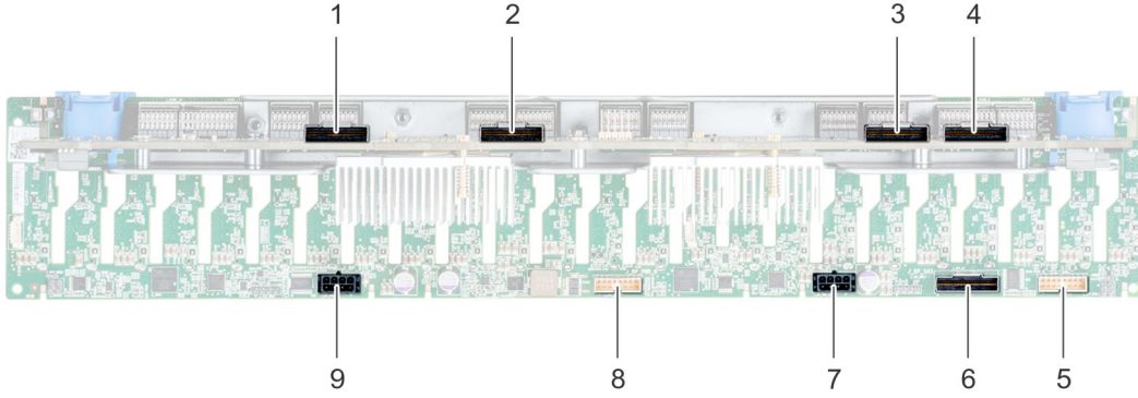
Rakam 125. 24 x 2,5 inç (24 NVMe) arka panelin arkadan görünümü
