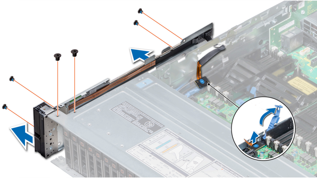
Rakam 174. Sol kontrol panelini çıkarma
