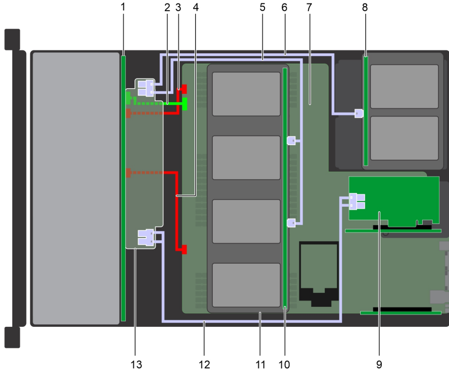
Rakam 141. Kablo yerleşimi - 4 x 2,5 inç adaptör orta sürücü tepsi arka paneli ve adaptör PERC11/HBA'lı 4 x 2,5 inç arka sürücü arka paneli ile 24 x 2,5 inç sürücü arka paneli
