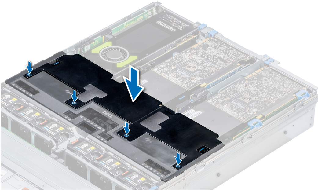
Rakam 112. GPU hava örtüsünün üst kapağını takma
