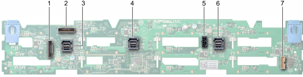
Rakam 130. 3,5 inç Çalışırken Takılabilen sürücülü (SATA ve SAS) karma arka panelin NVMe U.2 SSD ile arkadan görünümü
