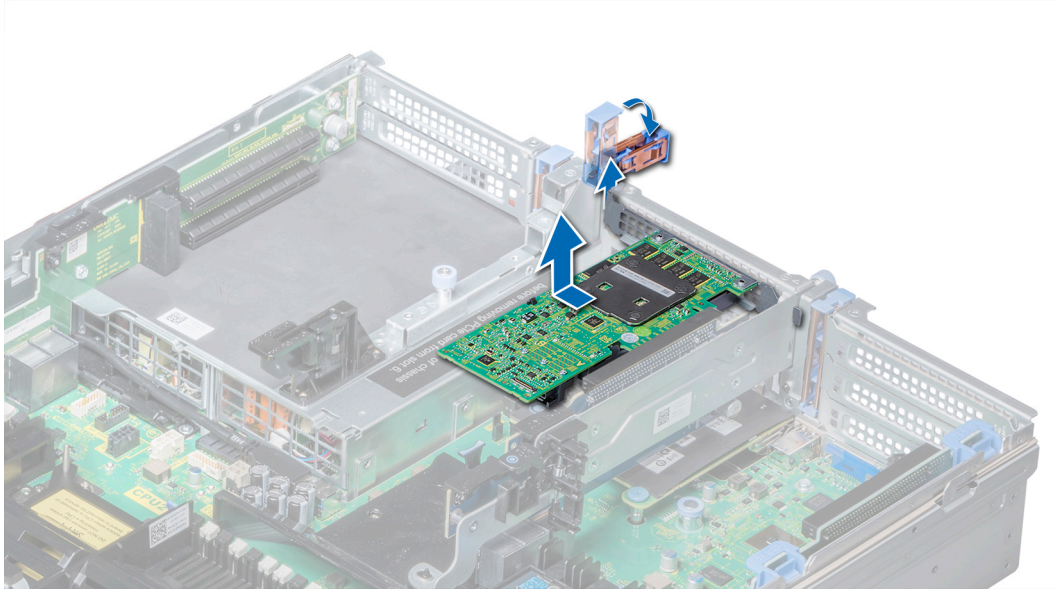
Rakam 84. Genişletme kartını genişletme kartı yükselticisi 2'den çıkarma
