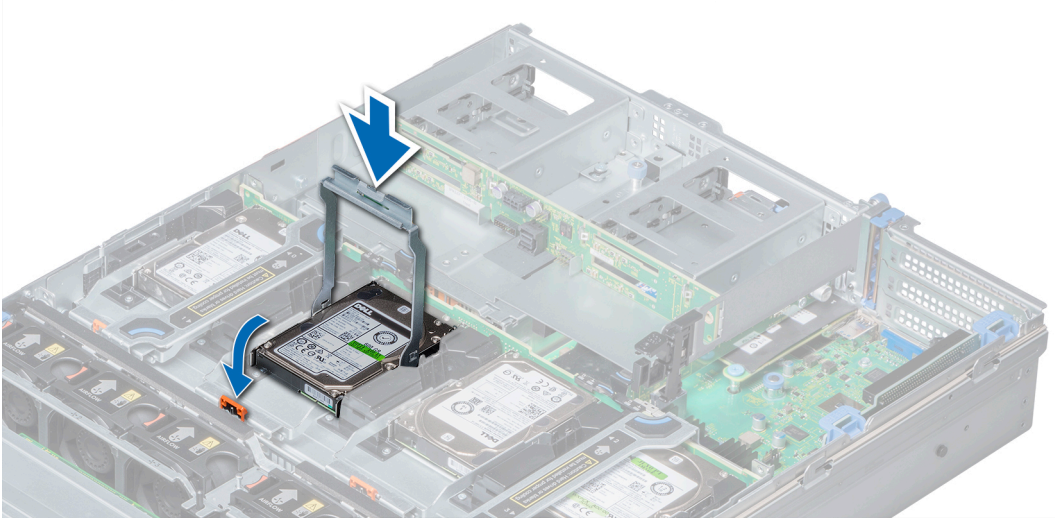
Rakam 50. Sürücü taşıyıcısını orta sürücü tepsisine takma
