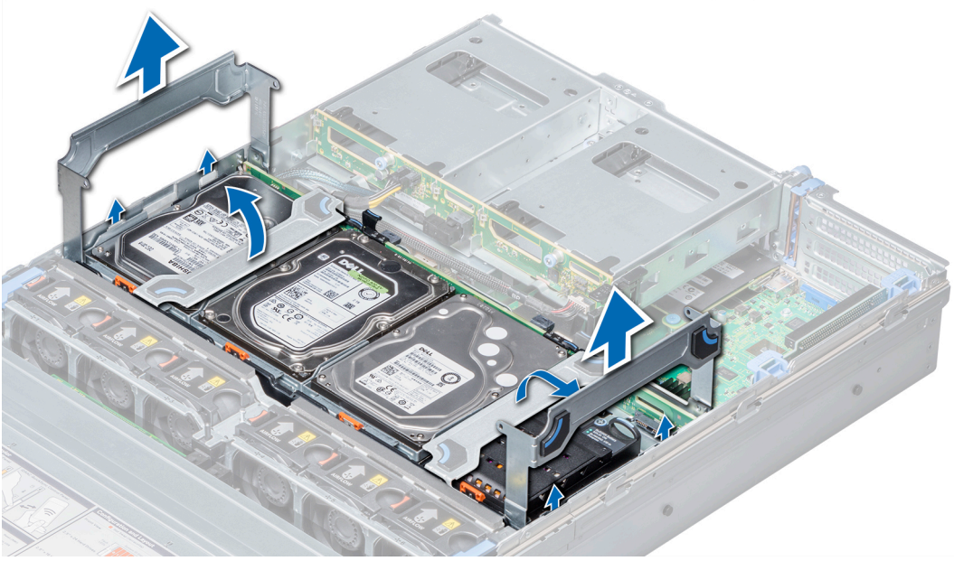
Rakam 45. Orta sürücü tepsisini çıkarma
