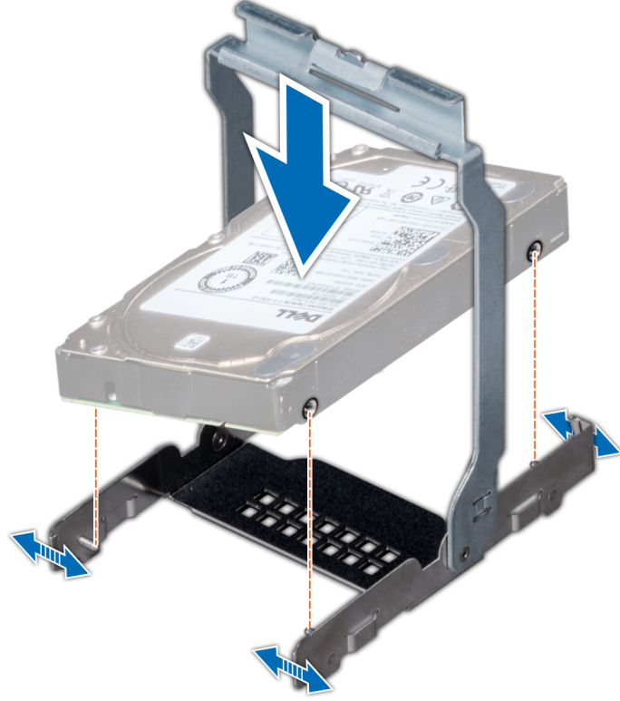
Rakam 52. Sürücü taşıyıcısına 3,5 inç sürücüyü takma
