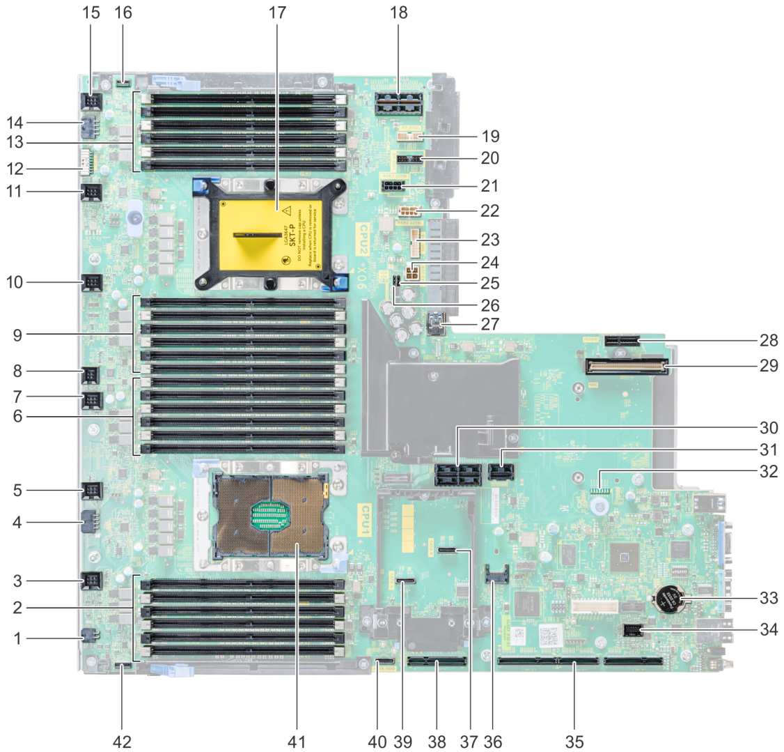
Rakam 178. Sistem kartı atlama telleri ve konektörleri
