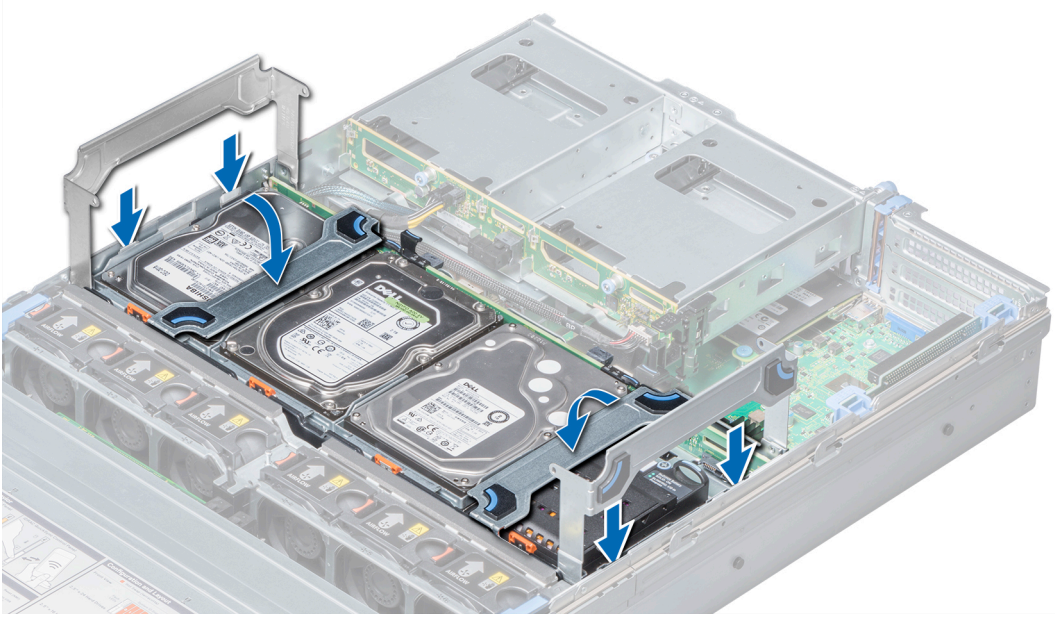
Rakam 46. Orta sürücü tepsisini takma
