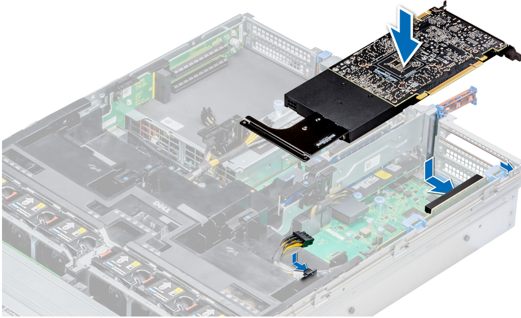
Rakam 108. GPU 1'i takma
