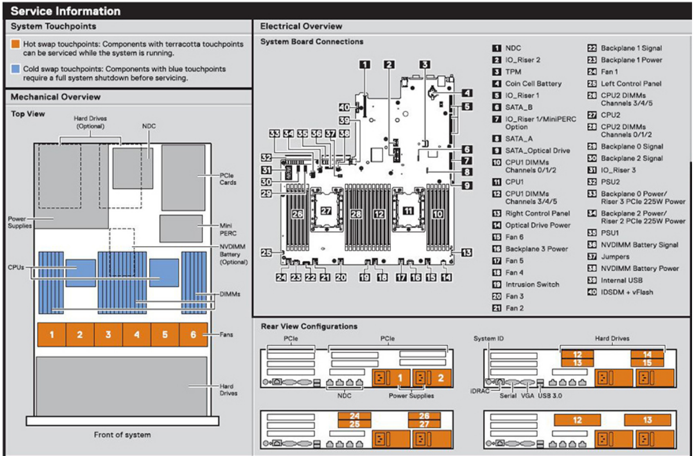
Rakam 19. Servis Bilgileri
