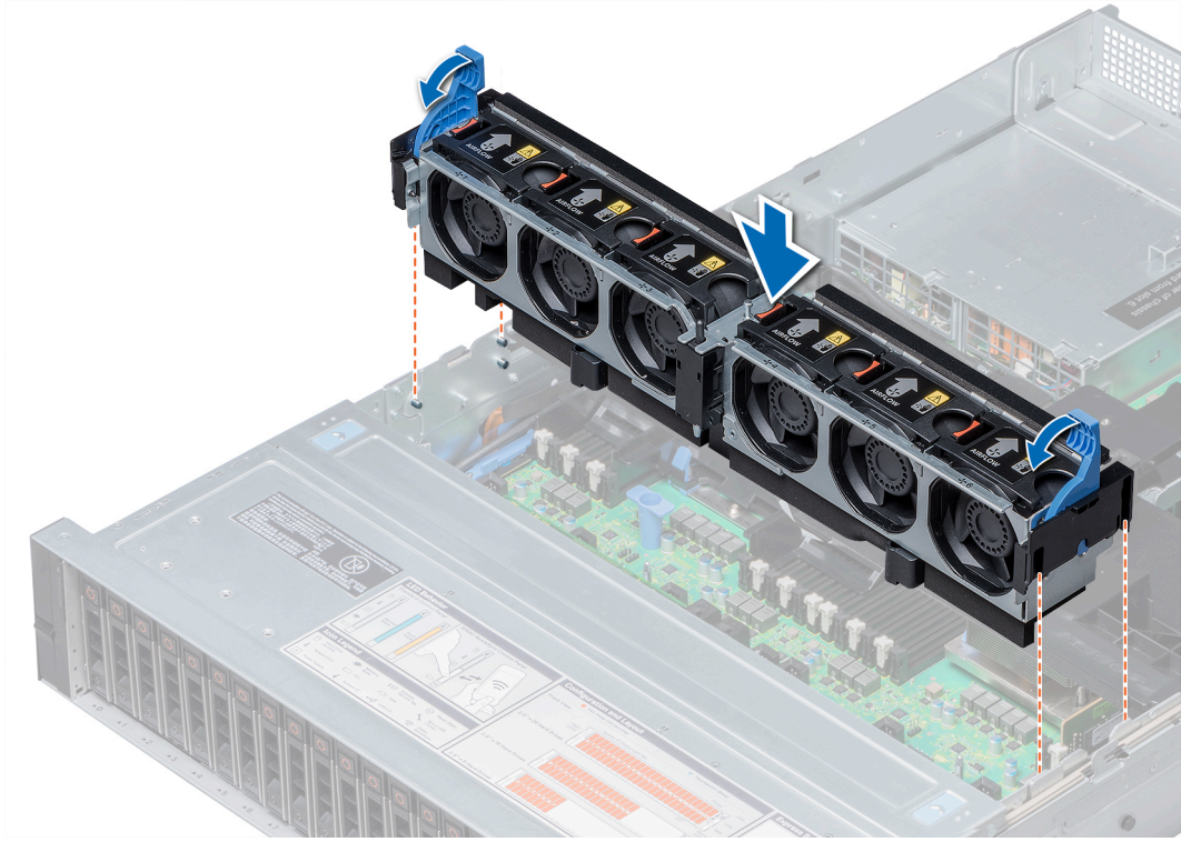
Rakam 34. Soğutma fanı aksamını takma
