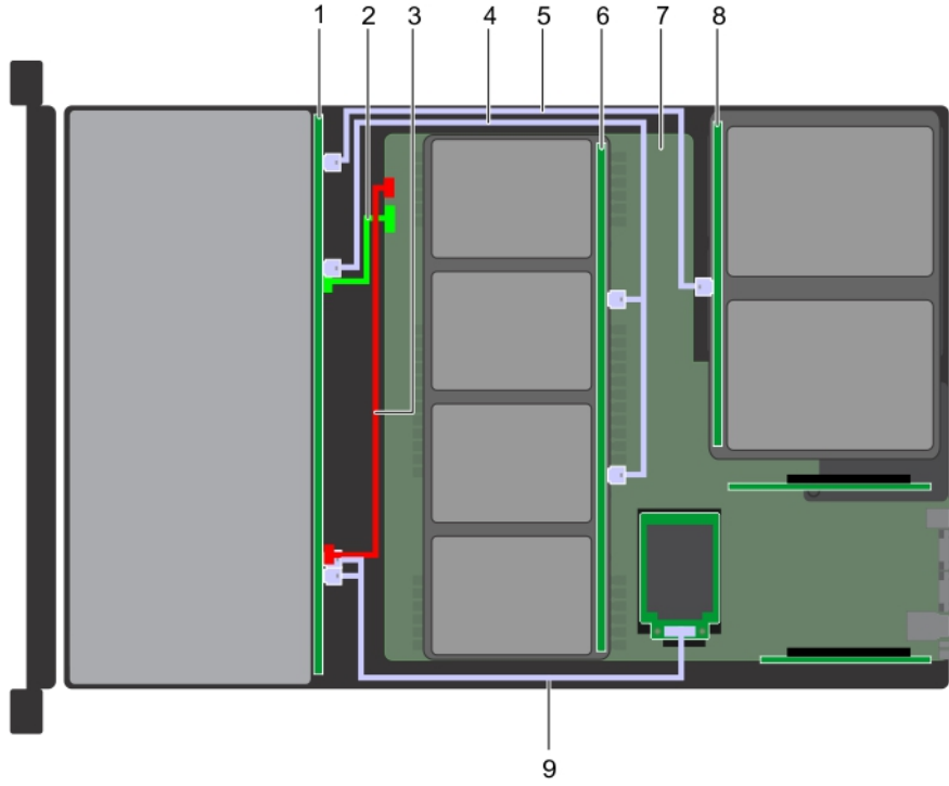
Rakam 157. Kablo yerleşimi – 4 x 3,5 inç (4 x 2,5 inç adaptör) orta sürücü tepsisi arka paneli ve 2 x 3,5 inç arka sürücü arka paneliyle 12 x 3,5 inç sürücü arka paneli
