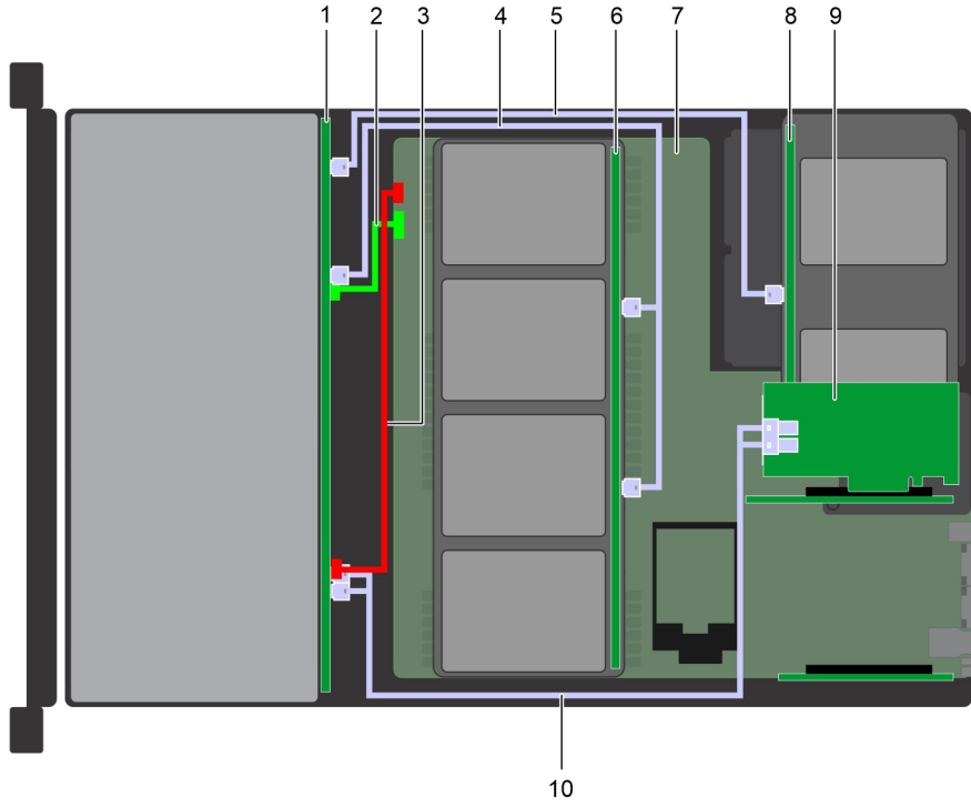
Rakam 143. Kablo yerleşimi – 4 x 3,5 inç (4 x 2,5 inç adaptör) orta sürücü tepsisi arka paneli ve adaptör PERC11/HBA'lı 4 x 2,5 inç arka sürücü arka paneliyle 12 x 3,5 inç sürücü arka paneli
