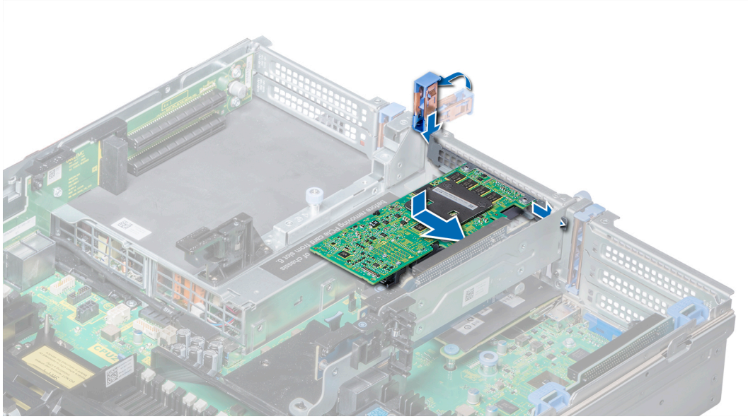
Rakam 88. Genişletme kartını genişletme kartı yükselticisi 2'ye takma
