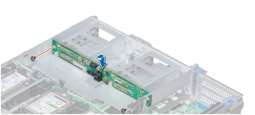
Rakam 138. 2,5 inç sürücü arka panelini takma
