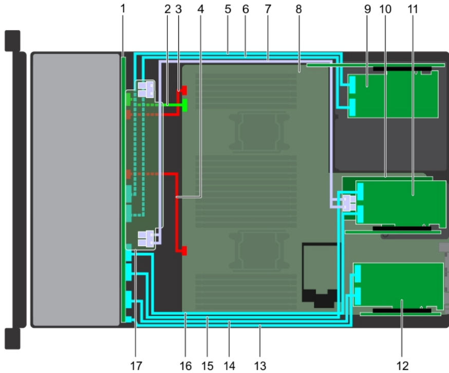
Rakam 152. Kablo yerleşimi - 12 SAS artı 12 PCIe ve adaptör PERC'li 24 x 2,5 inç sürücü arka paneli
