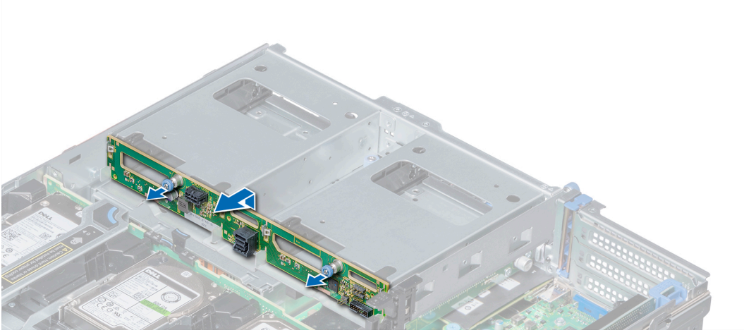
Rakam 135. 3,5 inç sürücü arka panelini çıkarma
