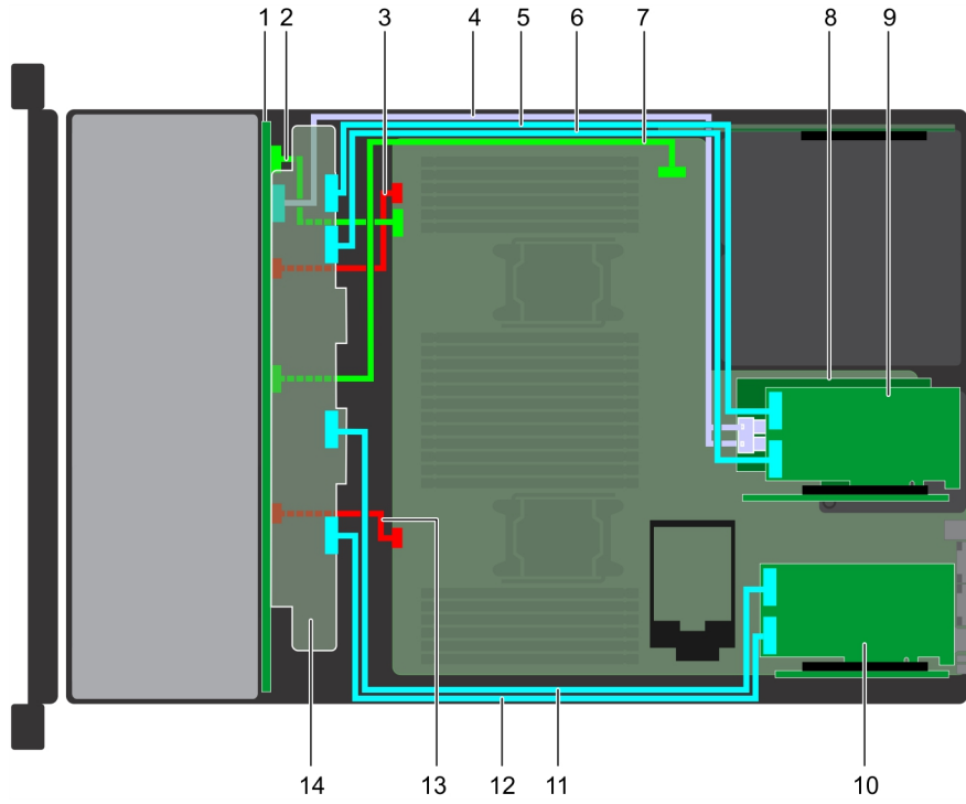
Rakam 154. Kablo yerleşimi – en çok 24 NVMe veya NVMe'li en çok 8 SAS/SATA sürücülü 24 x 2,5 inç sürücü arka paneli
