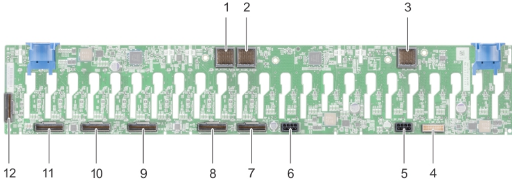
Rakam 124. 24 x 2,5 inç arka panelin arkadan görünümü
