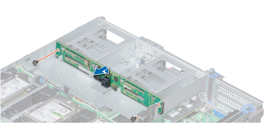
Rakam 137. 2,5 inç sürücü arka panelini çıkarma
