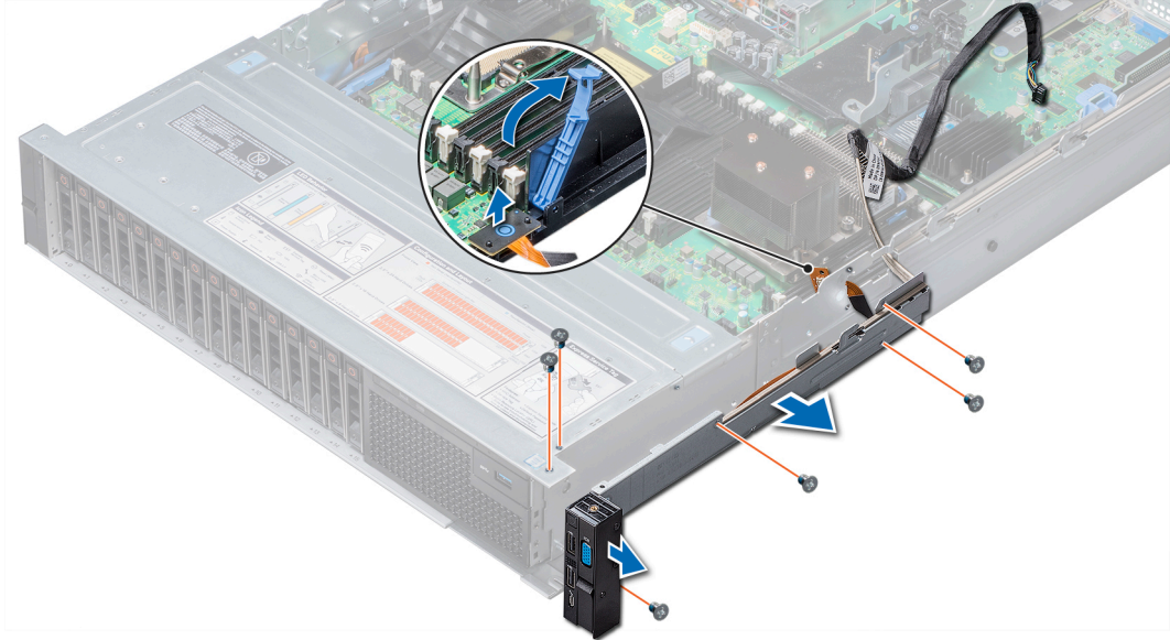
Rakam 176. Sağ kontrol panelini çıkarma
