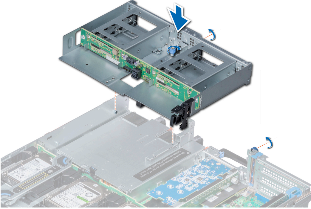
Rakam 67. 4x 2,5 inç arka sürücü kafesini takma
