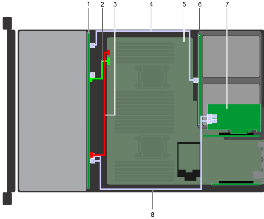
Rakam 146. Kablo yerleşimi – Adaptör PERC11/HBA'lı 2 x 3,5 inç arka sürücü arka paneli ile 12 x 3,5 inç sürücü arka paneli
