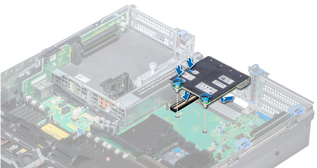
Rakam 119. Ağ çekme kartını takma
