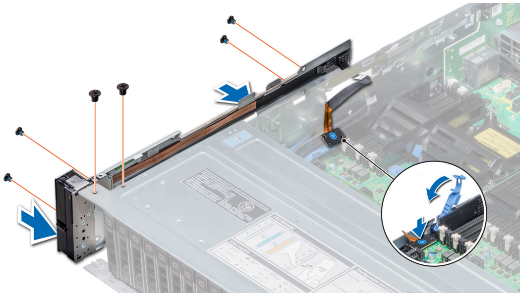
Figure 175. Installation du panneau de commande gauche
