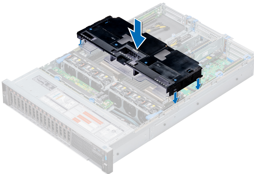
Figure 105. Installation du carénage d'aération du processeur graphique
