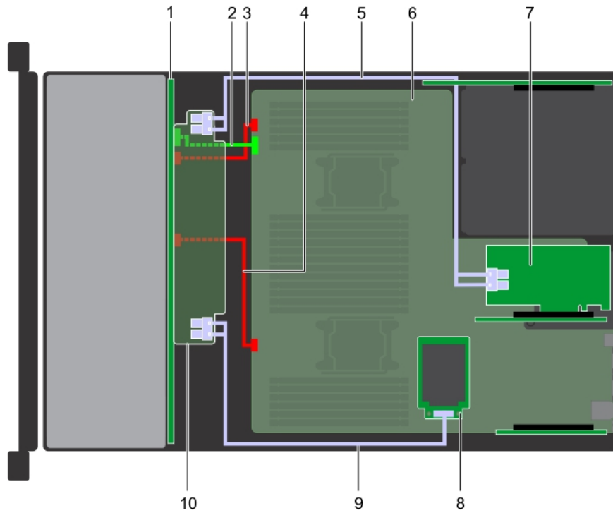
Figure 149. Acheminement des câbles - Fond de panier de 24 disques de 2,5 pouces avec carte mini PERC/HBA et adaptateur PERC/HBA
