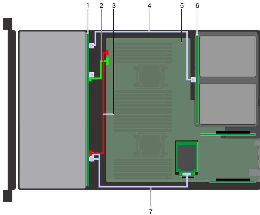
Figure 159. Acheminement des câbles - Fond de panier de 12 disques de 3,5 pouces avec fond de panier de 2 disques arrière de 3,5 pouces
