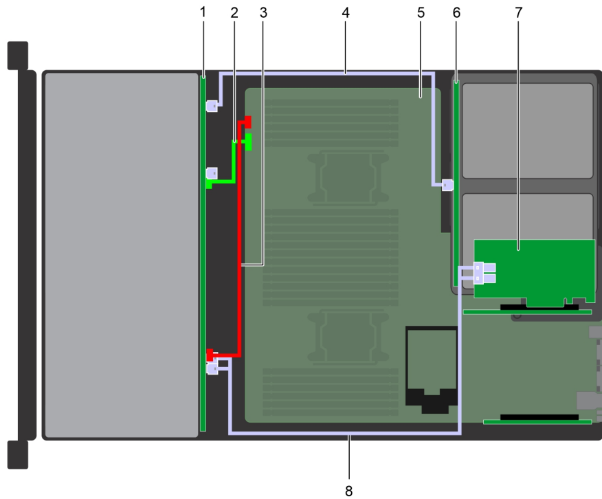
Figure 146. Acheminement des câbles - Fond de panier de 12 disques de 3,5 pouces avec fond de panier de disque arrière de 3,5 pouces (x 2) avec adaptateur PERC11/HBA
