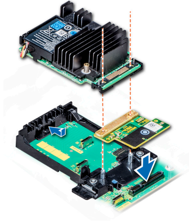
Figure 122. Installation de la carte de contrôleur de stockage intégré
