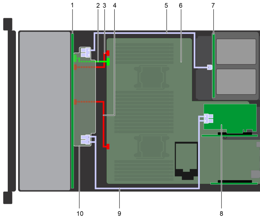
Figure 142. Acheminement des câbles - Fond de panier de 24 disques de 2,5 pouces avec fond de panier de disque arrière de 2,5 pouces (x 4) avec adaptateur PERC11/HBA
