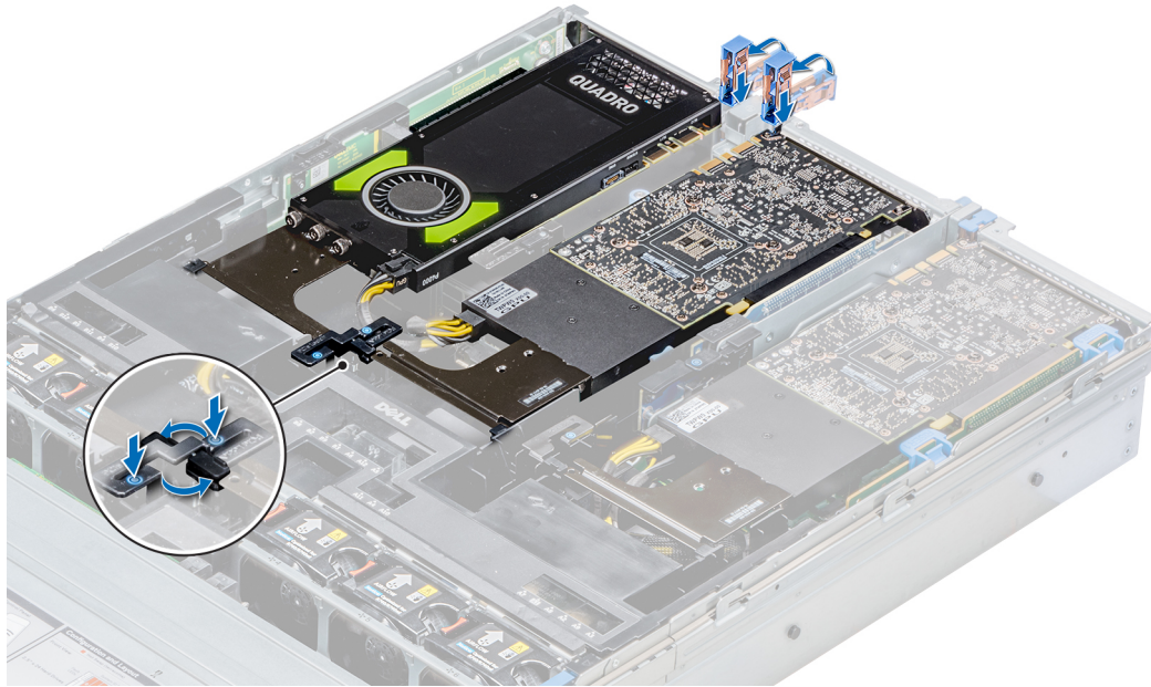
Figure 111. Fixation des processeurs graphiques 2 et 3
