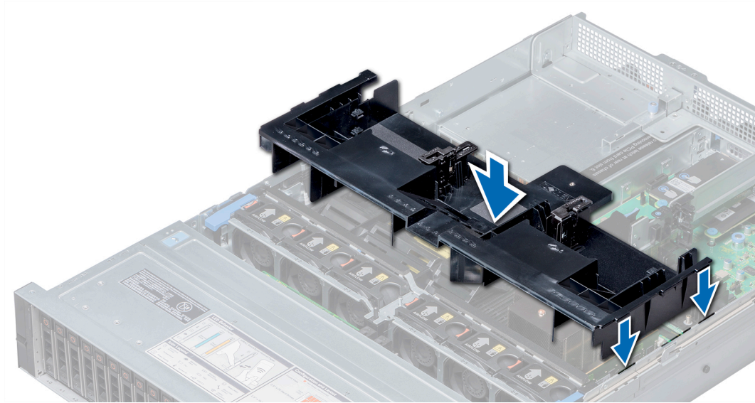
Figure 32. Installation du carénage à air
