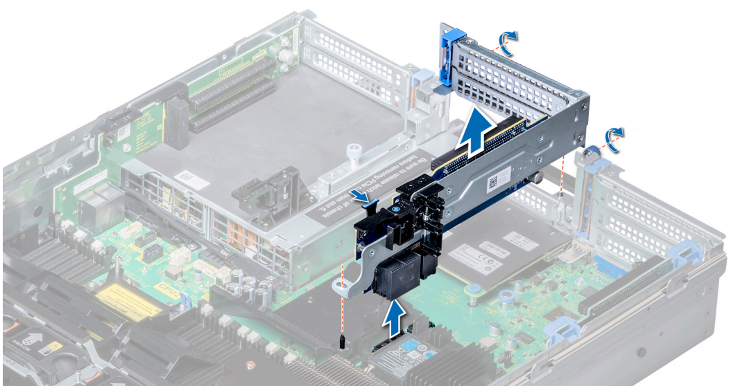
Figure 96. Retrait de la carte de montage pour carte d'extension 2A
