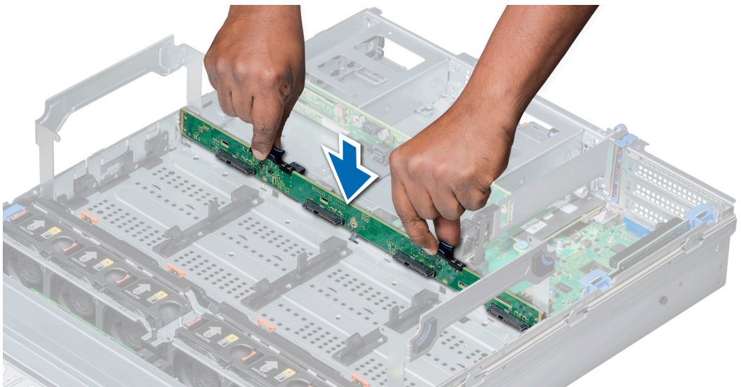
Figure 134. Installation du backplane du plateau de disques intermédiaire
