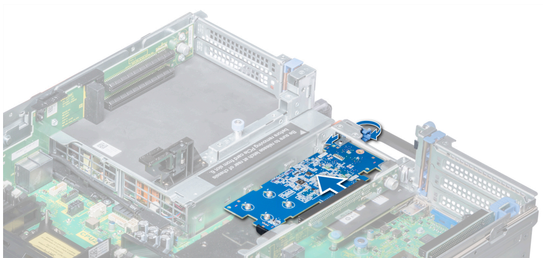
Figure 83. Retrait de la carte d'extension de la carte de montage pour carte d'extension 2B
