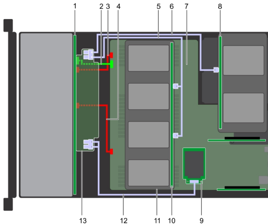
Figure 150. Acheminement des câbles - Fond de panier de 24 disques de 2,5 pouces avec fond de panier de 4 disques de plateau intermédiaire d'adaptateur de 2,5 pouces et fond de panier de 4 disques arrière de 2,5 pouces
