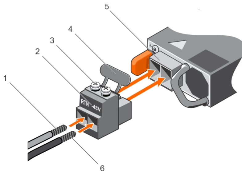
Figure 169. Assemblage des câbles d'alimentation d'entrée CC
