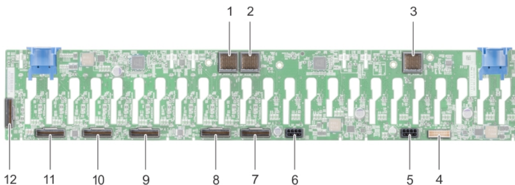
Figure 124. Vue arrière du backplane de 24 disques de 2,5 pouces
