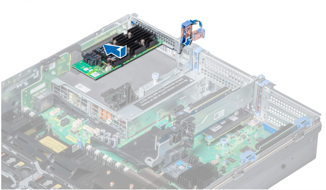
Figure 89. Installation d'une carte d'extension dans la carte de montage pour carte d'extension 3
