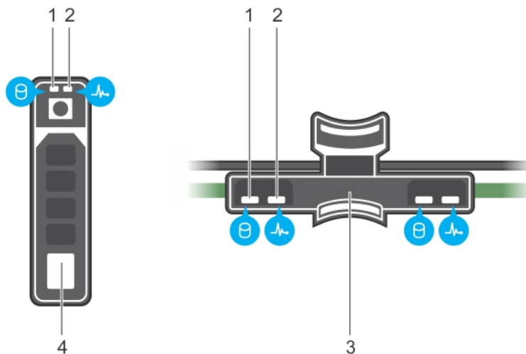
Figure 13. Voyants présents sur le disque et sur le backplane de plateau de disques intermédiaire
