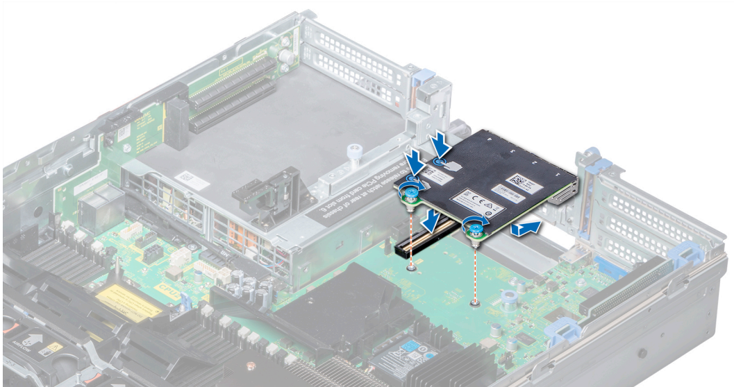
Figure 119. Installation de la carte fille réseau
