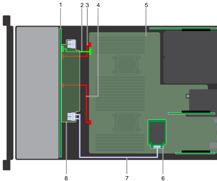
Figure 147. Acheminement des câbles - Fond de panier de 24 disques de 2,5 pouces avec mini PERC
