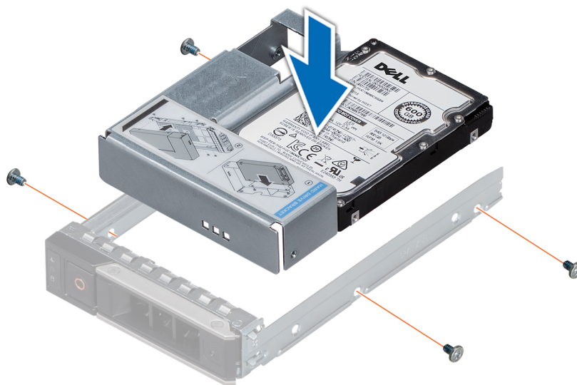
Figure 62. Installation d'un adaptateur de 3,5 pouces dans un support de disque de 3,5 pouces
