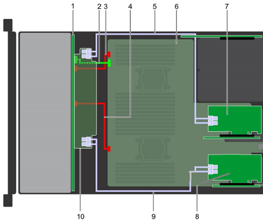
Figure 139. Acheminement des câbles - Fond de panier de 24 disques de 2,5 pouces avec double adaptateur PERC/HBA
