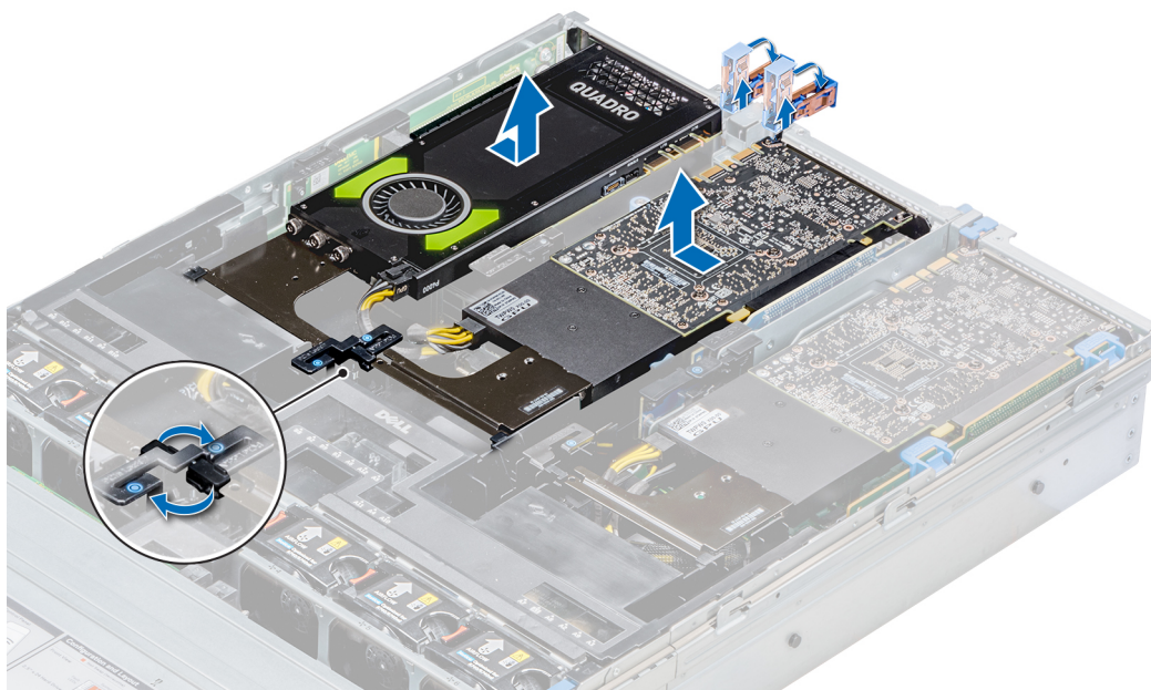
Figure 104. Retrait des processeurs graphiques 2 et 3
