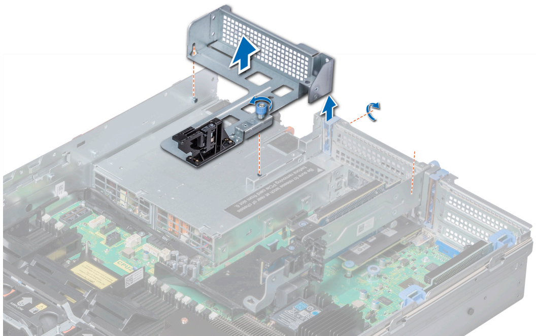
Figure 92. Retrait du cache de la carte de montage 3
