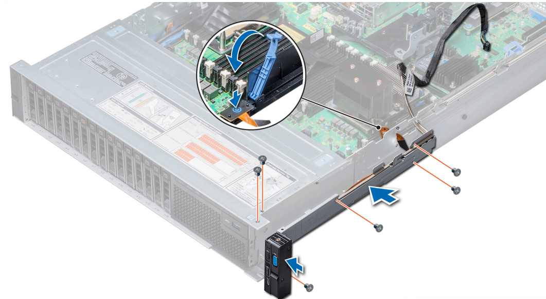
Figure 177. Installation du panneau de commande droit
