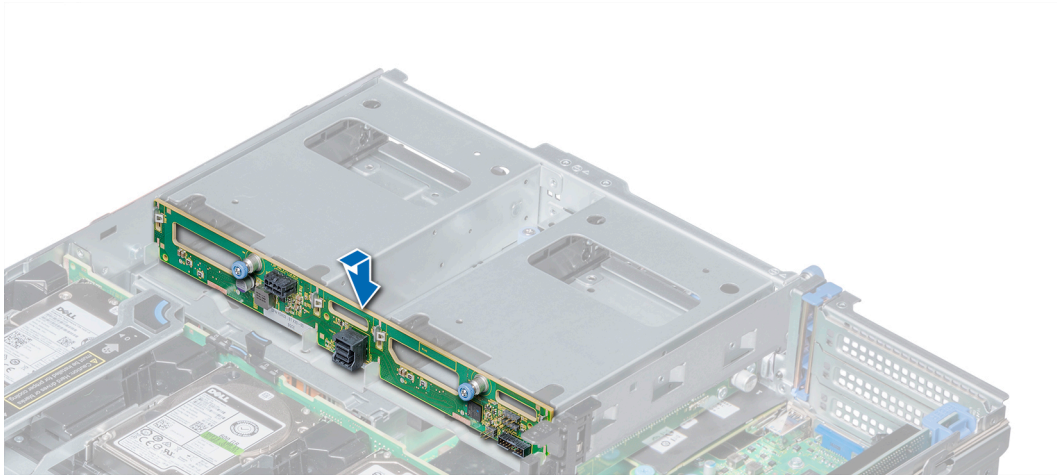
Figure 136. Installation du backplane arrière des disques de 3,5 pouces
