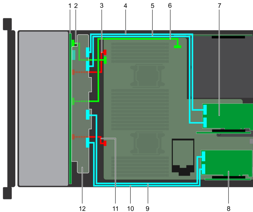
Figure 153. Acheminement des câbles - Fond de panier de 24 disques NVMe de 2,5 pouces
