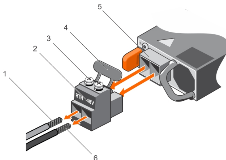
Figure 170. Retrait des câbles d'alimentation d'entrée en CC
