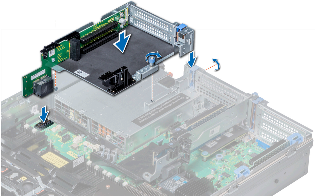
Figure 101. Installation de la carte de montage pour carte d'extension 3
