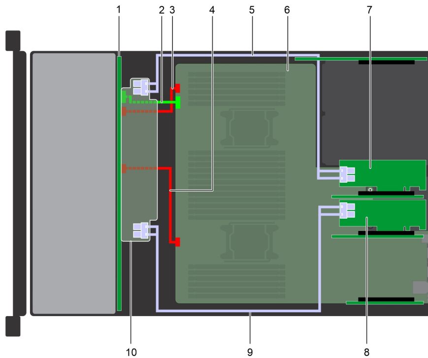
Figure 140. Acheminement des câbles - Fond de panier de 24 disques de 2,5 pouces avec double adaptateur PERC/HBA
