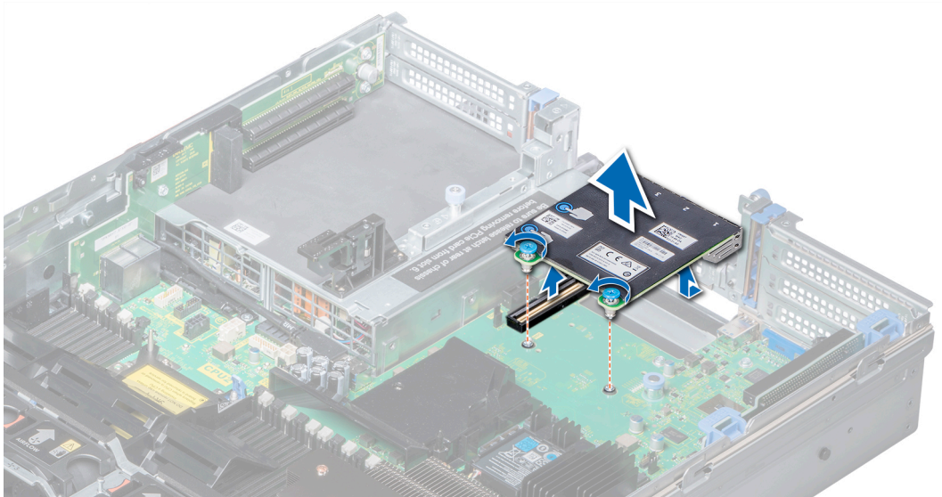
Figure 118. Retrait de la carte fille réseau
