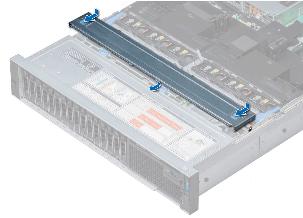
Figure 28. Installation du cache de fond de panier
