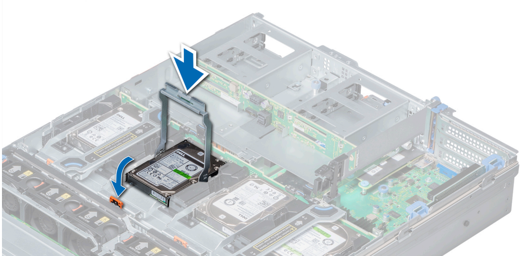
Figure 50. Installation d'un support de disque dans un plateau de disque demi-hauteur
