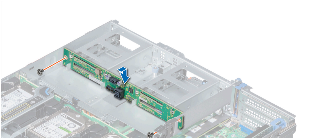
Figure 138. Installation du backplane de disques 2,5 pouces arrière
