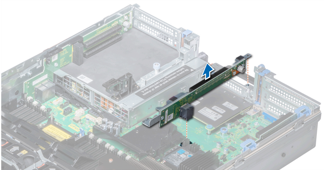
Figure 97. Retrait de la carte de montage 2 pour carte d'extension
