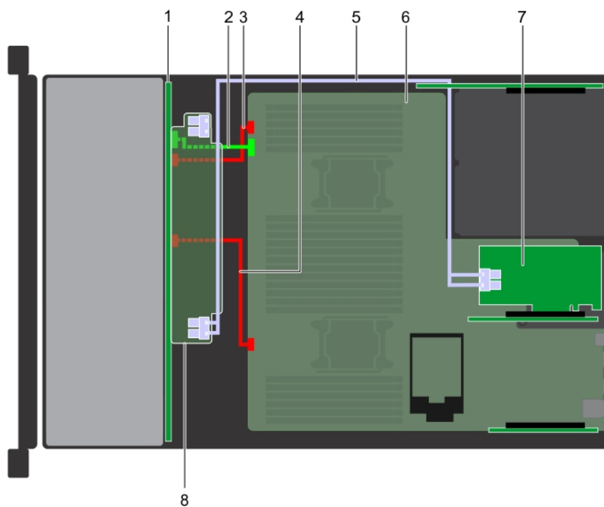
Figure 148. Acheminement des câbles - Fond de panier de 24 disques de 2,5 pouces avec adaptateur PERC
