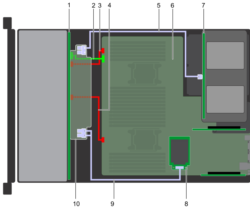
Figure 151. Acheminement des câbles - Fond de panier de 24 disques de 2,5 pouces avec fond de panier de disque arrière de 2,5 pouces (x 4)
