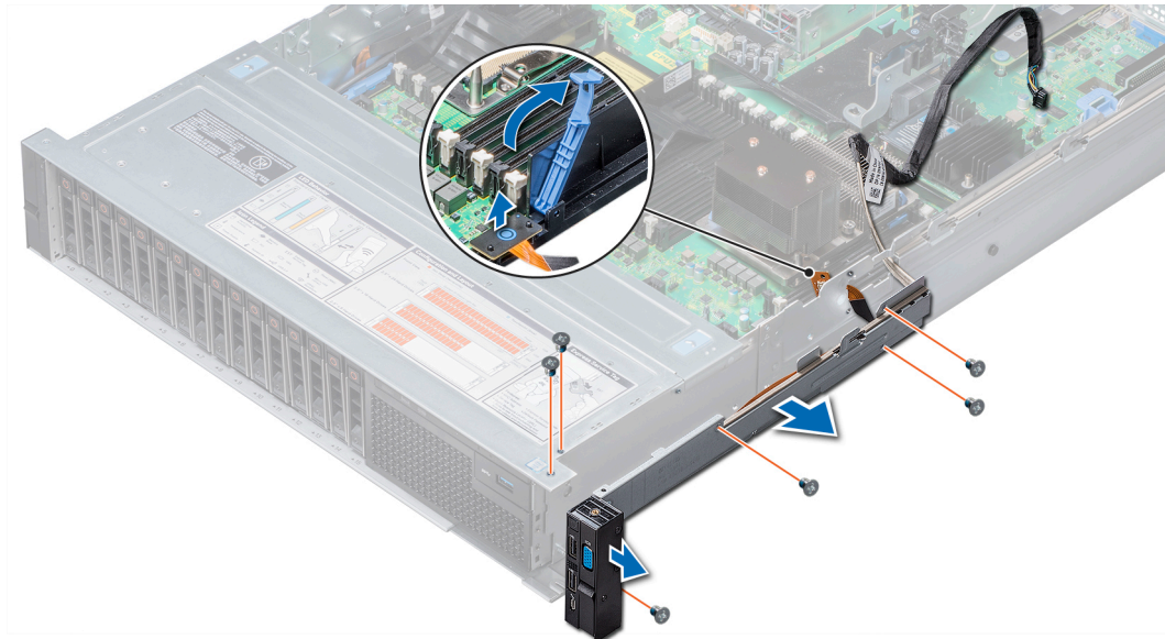
Figure 176. Retrait du panneau de commande droit
