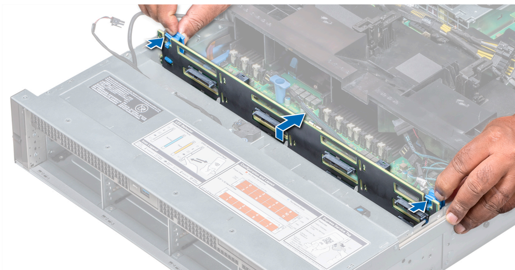
Figure 131. Retrait du fond de panier
