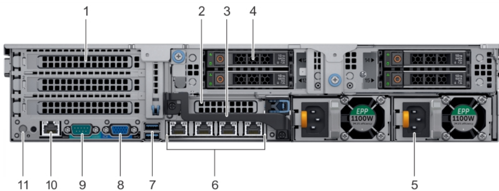
Figure 8. Vue arrière du système à 4 disques de 2,5 pouces
