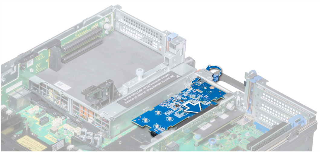
Figure 87. Installation d'une carte d'extension dans la carte de montage pour carte d'extension 2B
