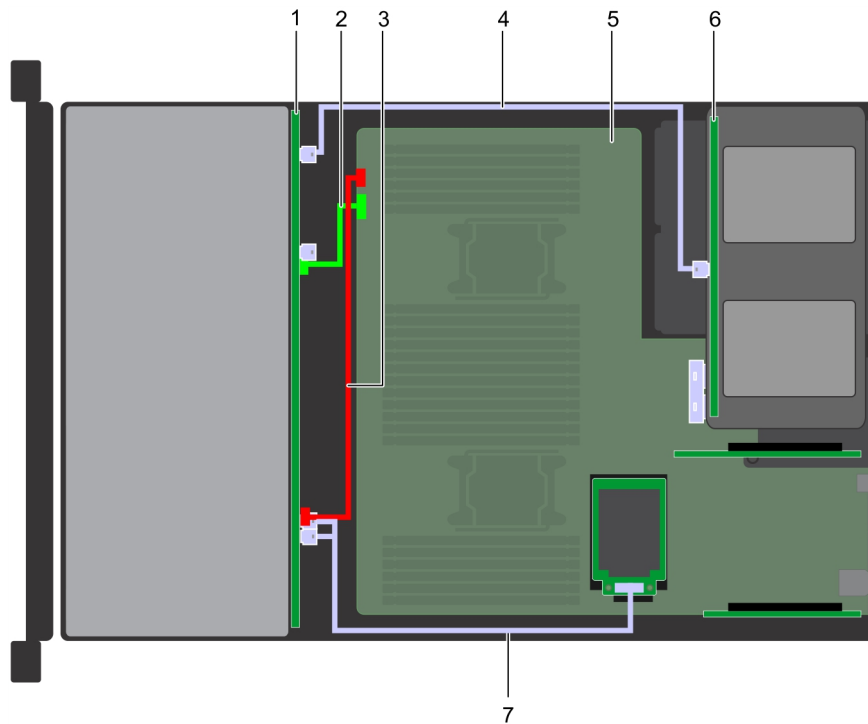
Figure 160. Acheminement des câbles - Fond de panier de 12 disques de 3,5 pouces avec fond de panier de 4 disques arrière de 2,5 pouces
