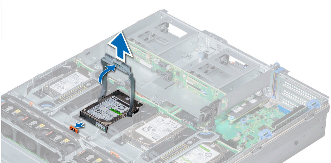
Figure 49. Retrait d'un disque dur installé dans un plateau de disque dur
