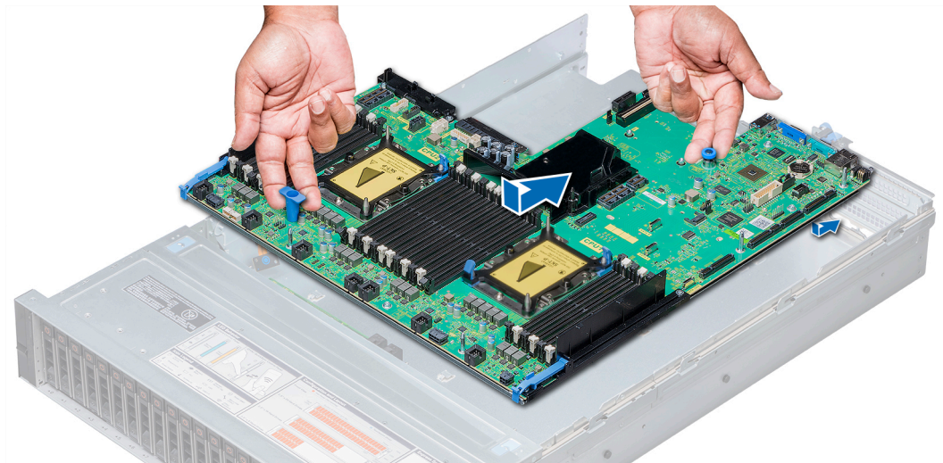
Figure 172. Installation de la carte système
