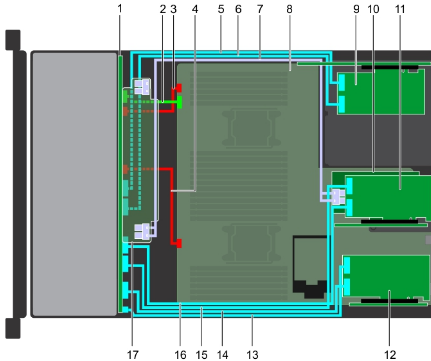
Figure 152. Acheminement des câbles - Fond de panier de 24 disques de 2,5 pouces avec 12 disques SAS plus 12 PCIe et adaptateur PERC
