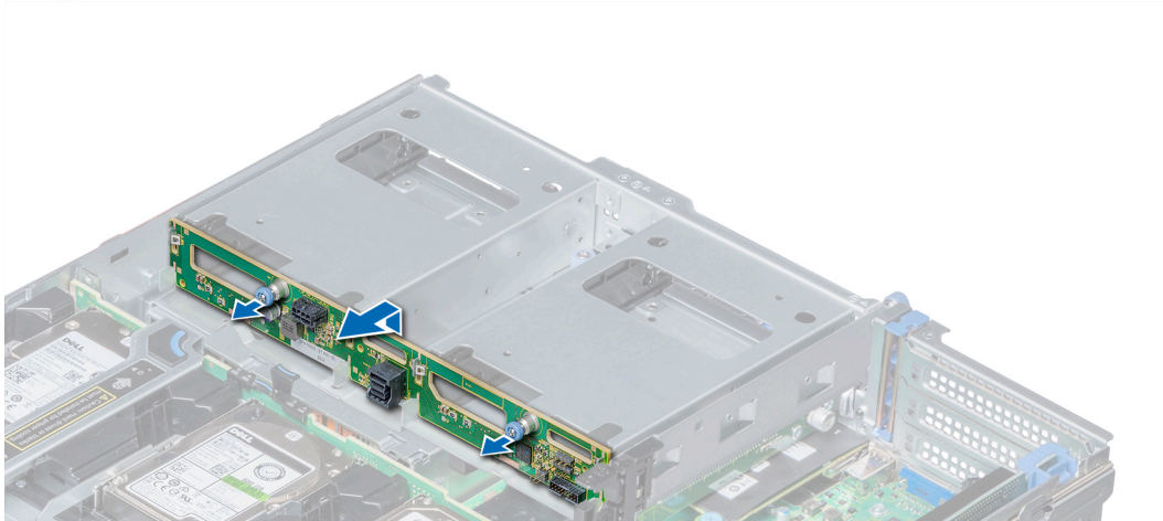
Figure 135. Retrait du backplane de disques 3,5 pouces arrière
