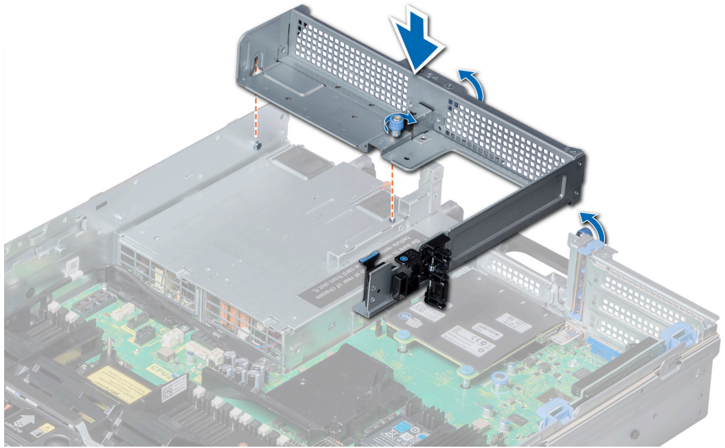
Figure 91. Installation du cache des cartes de montage 2 et 3
