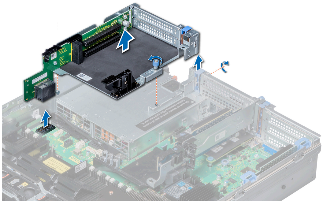
Figure 100. Retrait de la carte de montage pour carte d'extension 3
