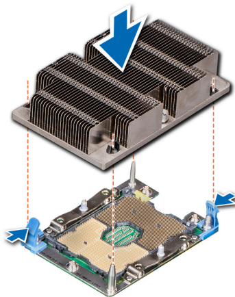
Figure 79. Installation du module processeur et dissipateur de chaleur (1U)
