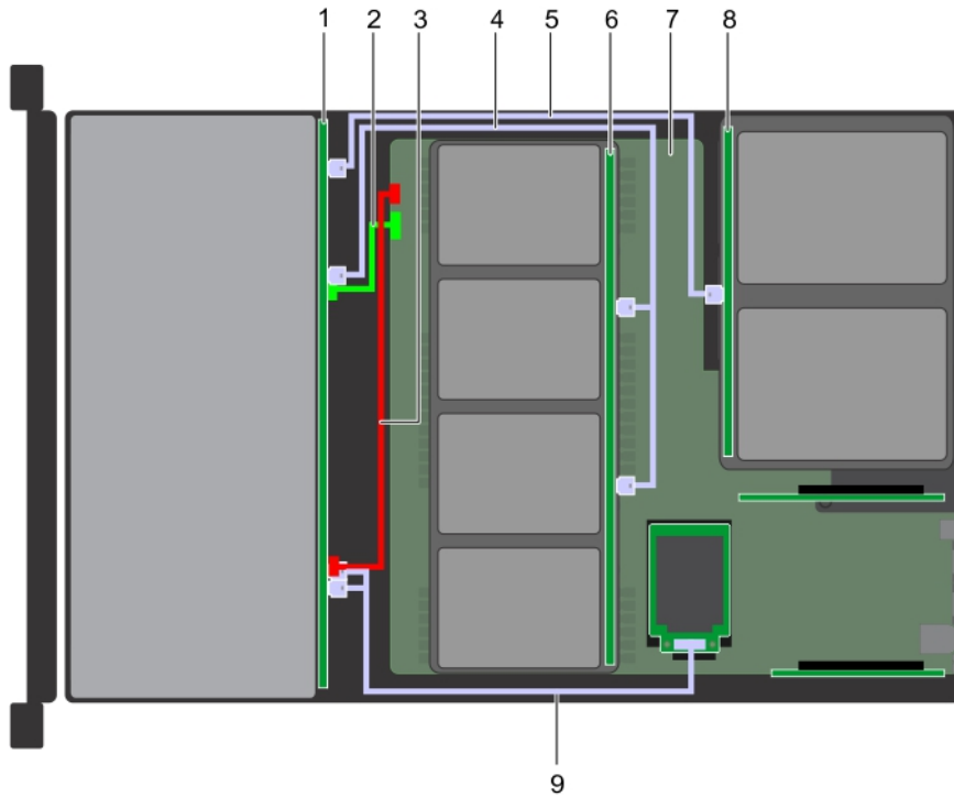
Figure 157. Acheminement des câbles - Fond de panier de 12 disques de 3,5 pouces avec fond de panier de plateau de disque central de 4 x 3,5 pouces (adaptateur de 4 x 2,5 pouces) et fond de panier de disque arrière de 2 x 2,5 pouces
