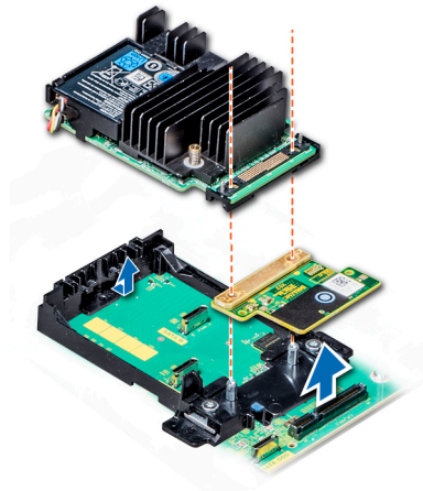
Figure 121. Retrait de la carte de contrôleur de stockage intégré
