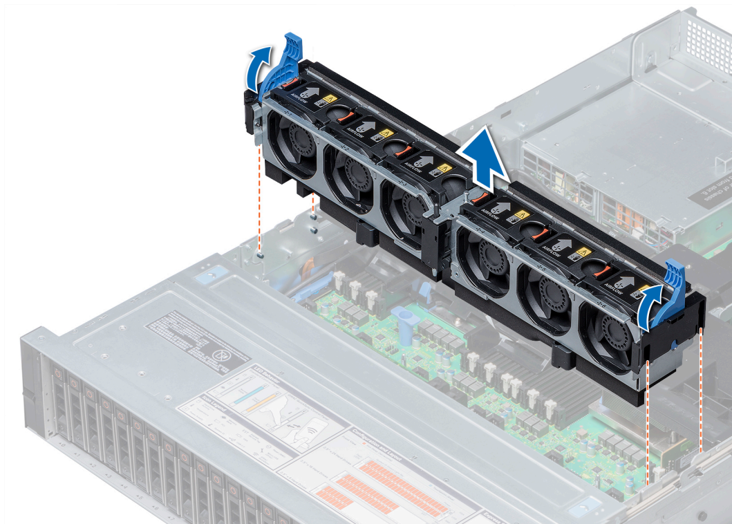
Figure 33. Retrait de l'assemblage de ventilation
