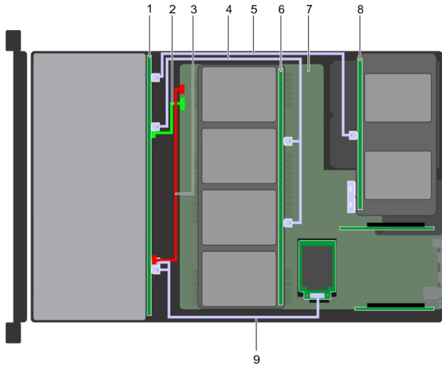
Figure 158. Acheminement des câbles - Fond de panier de 12 disques de 3,5 pouces avec fond de panier de plateau de disque central de 4 x 3,5 pouces (adaptateur de 4 x 2,5 pouces) et fond de panier de disque arrière de 4 x 2,5 pouces
