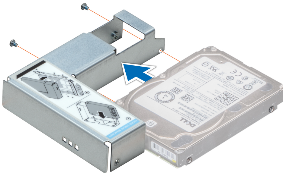
Figure 60. Installation d'un disque de 2,5 pouces dans un adaptateur de disque de 3,5 pouces
