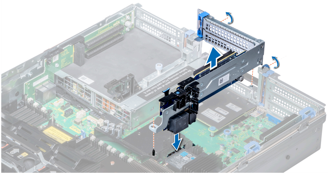
Figure 98. Installation de la carte de montage pour carte d'extension 2A
