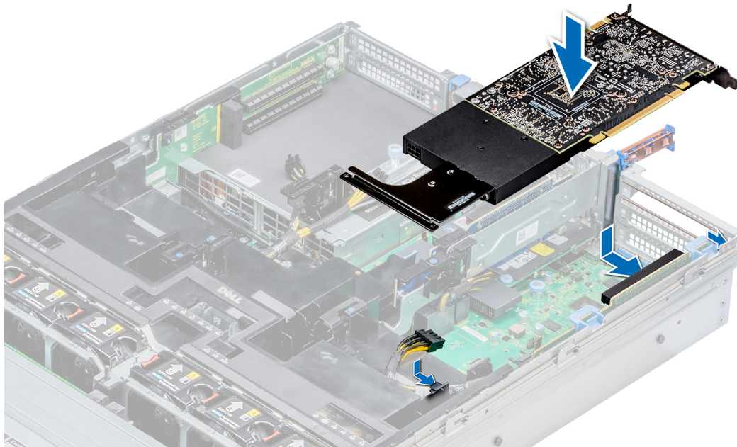
Figure 108. Installation du processeur graphique 1
