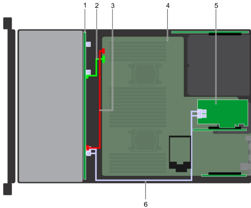
Figure 156. Fond de panier de 12 disques de 3,5 pouces avec adaptateur PERC
