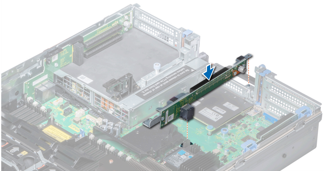
Figure 99. Installation de la carte de montage pour carte d'extension 2
