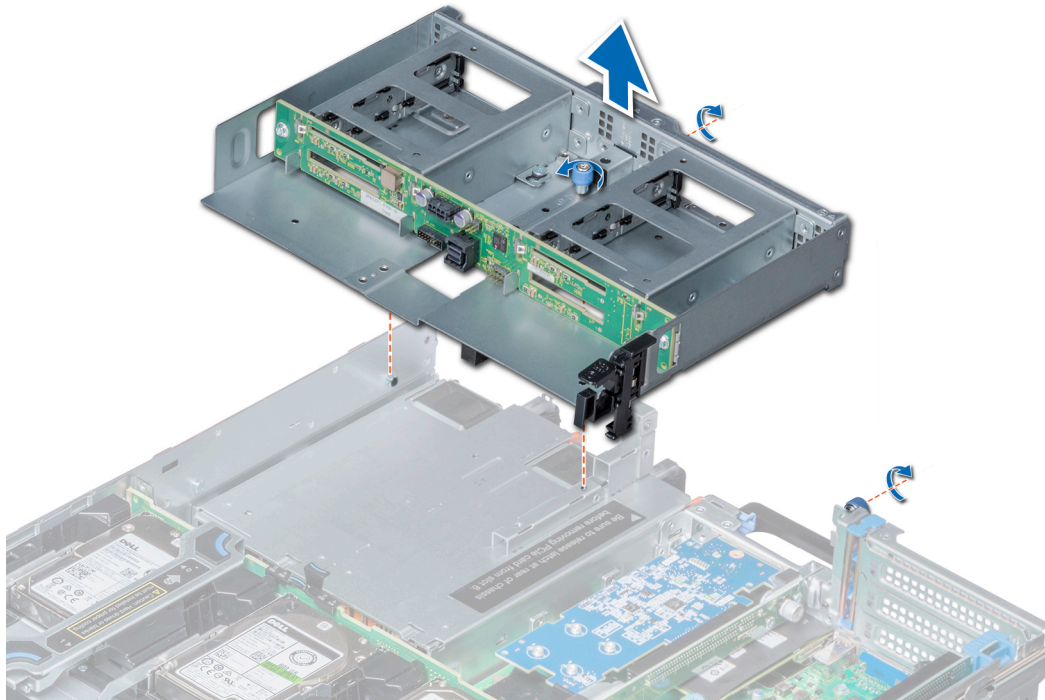
Figure 65. Retrait du bâti des disques arrière 4 x 2,5 pouces
