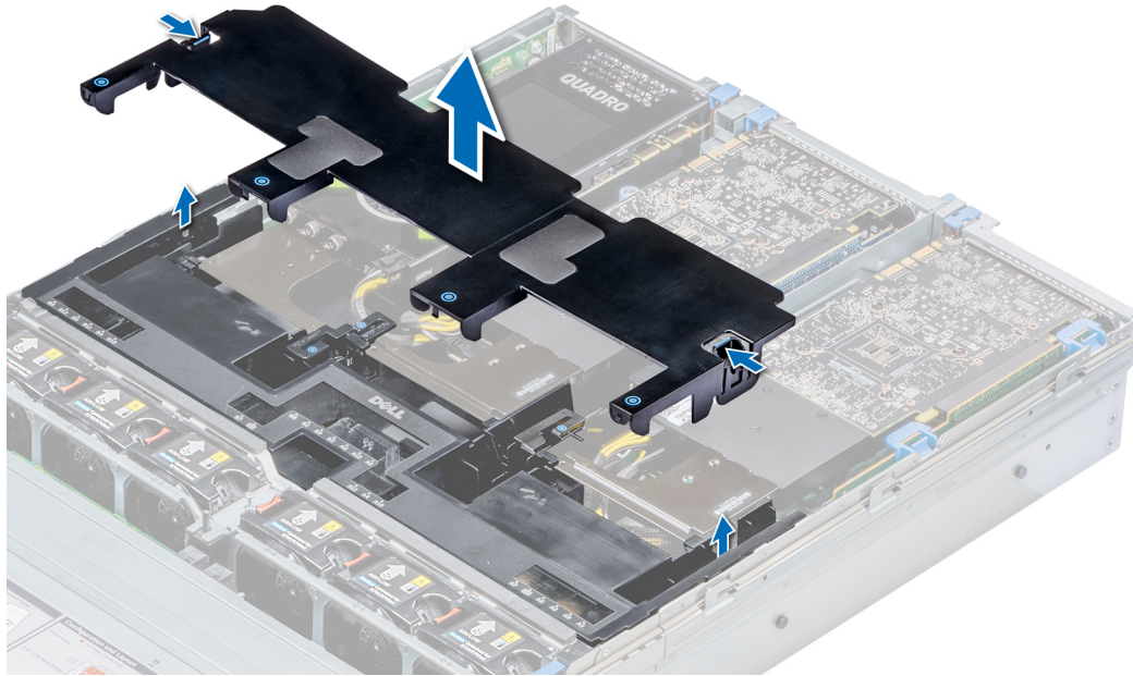
Figure 106. Retrait du capot supérieur du carénage
