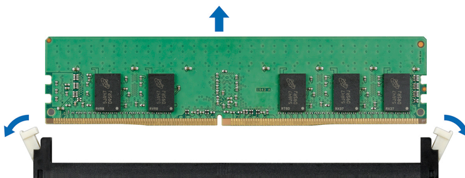
Figure 70. Retrait d'un module de mémoire
