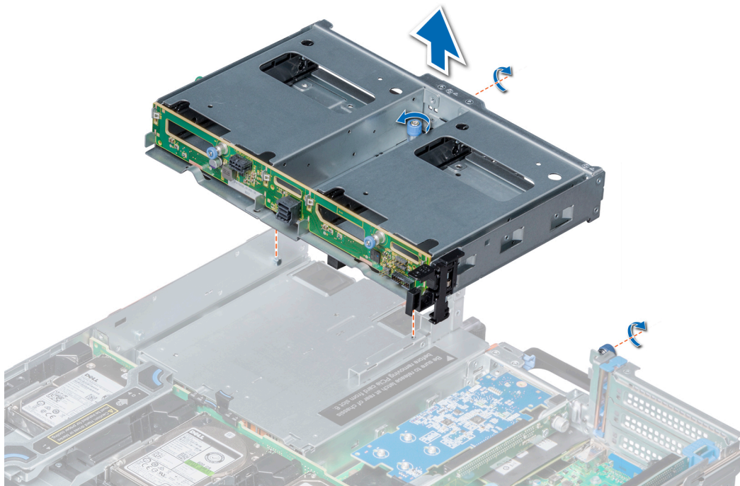
Figure 66. Retrait du bâti des disques arrière 2 x 3,5 pouces
