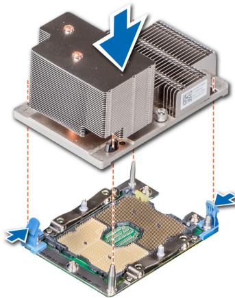
Figure 78. Installation du module processeur et dissipateur de chaleur (2U)
