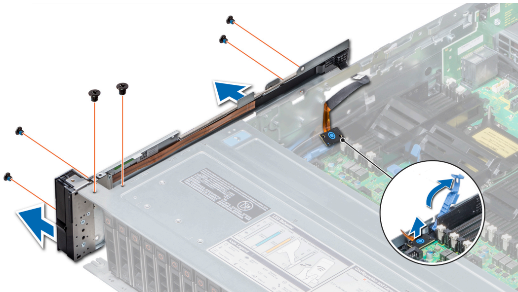
Figure 174. Retrait du panneau de commande de gauche
