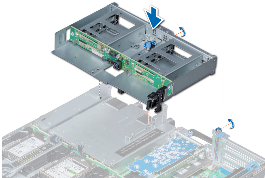
Figure 67. Installation du bâti des disques arrière 4 x 2,5 pouces
