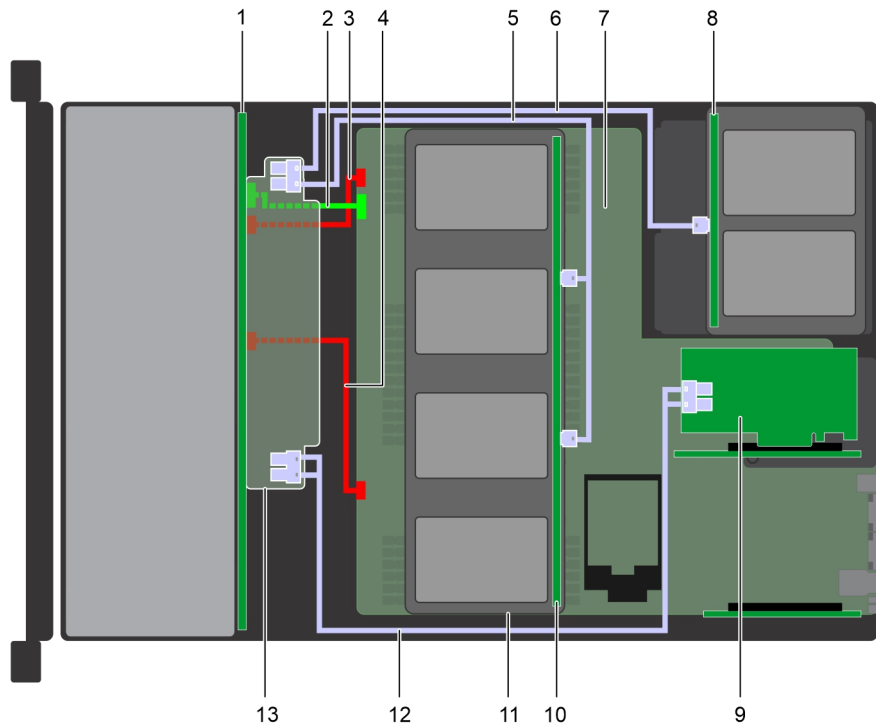
Figure 141. Acheminement des câbles - Fond de panier de 24 disques de 2,5 pouces avec fond de panier de 4 disques de plateau intermédiaire d'adaptateur de 2,5 pouces et fond de panier de 4 disques arrière de 2,5 pouces
