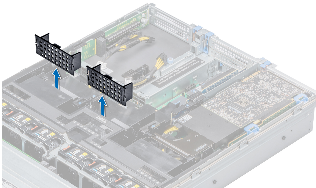
Figure 107. Retrait des panneaux de remplissage situés dans les logements du carénage d'aération du processeur graphique
