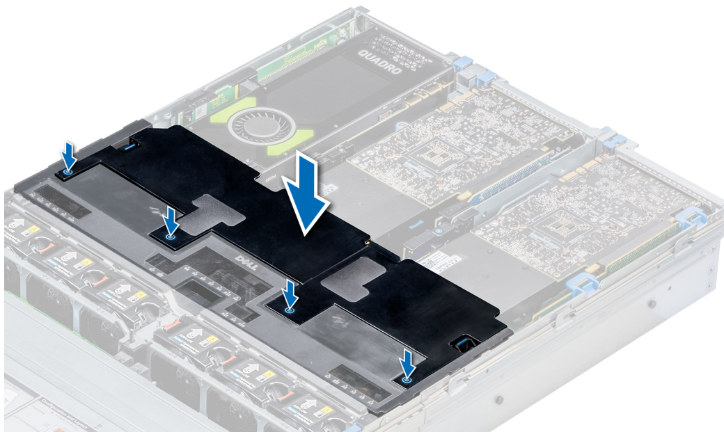
Figure 112. Installation du capot supérieur du carénage d'aération du processeur graphique
