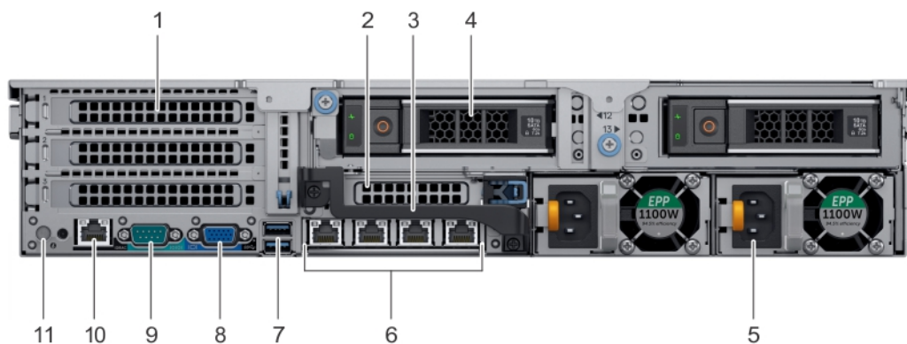
Figure 9. Vue arrière du système à 2 disques de 3,5 pouces
