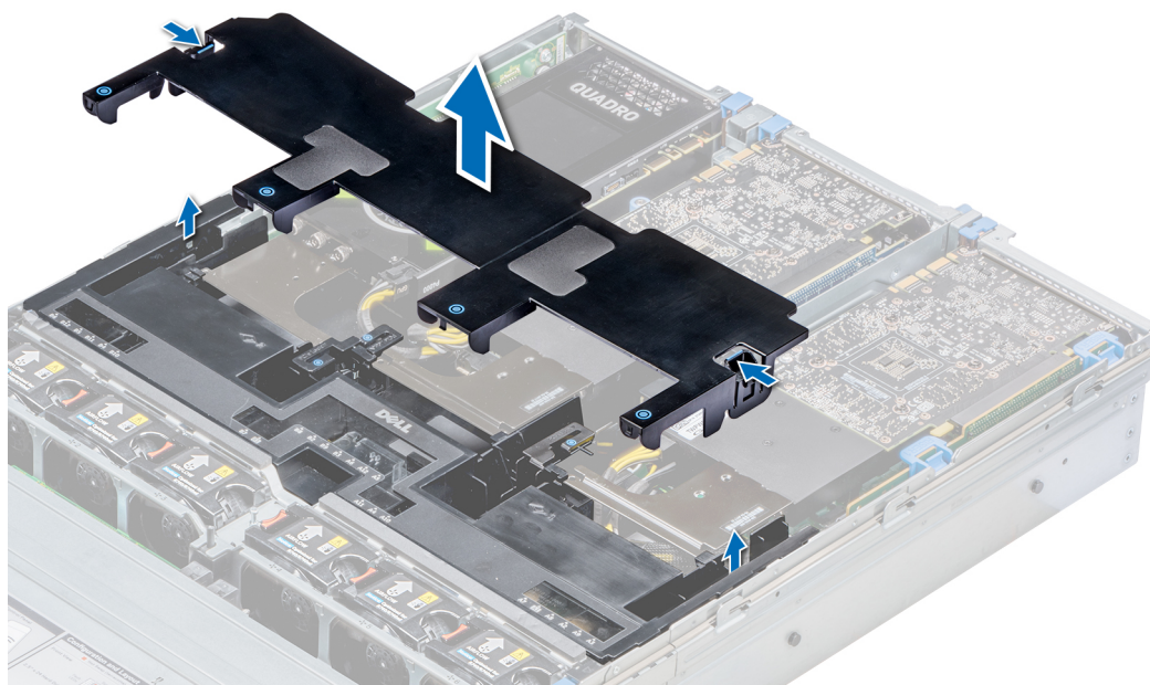
Figure 102. Retrait du capot supérieur du carénage d'aération du processeur graphique
