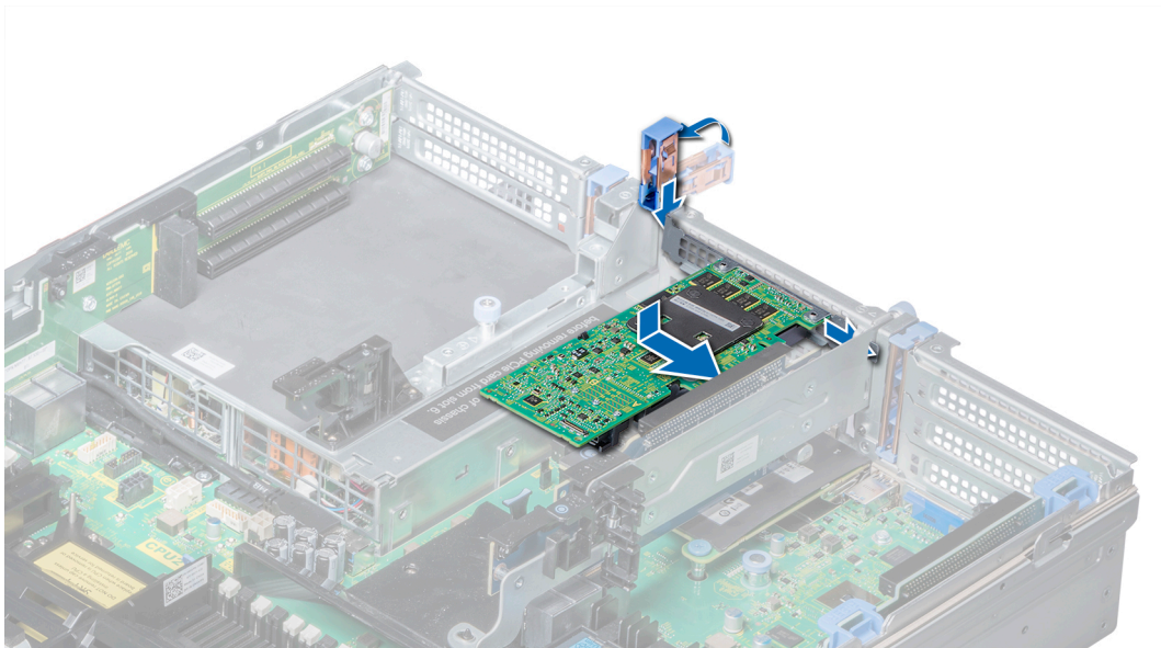
Figure 88. Installation d'une carte d'extension dans la carte de montage pour carte d'extension 2
