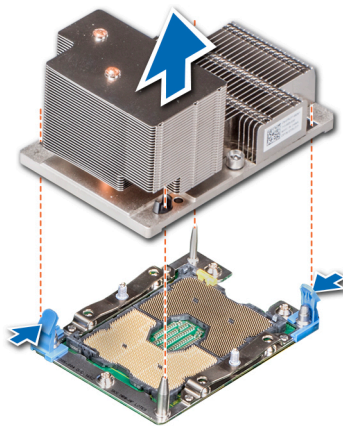
Figure 71. Retrait du module du processeur et du dissipateur de chaleur (2U)
