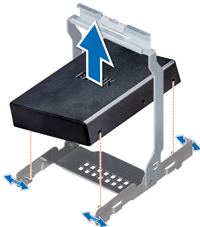
Figure 47. Retrait du cache de disque du support de disque demi-hauteur
