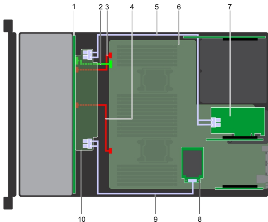
Ilustración 149. Enrutamiento de cables: backplane de unidad de 24 x 2,5 pulgadas con miniPERC/HBA y PERC/HBA del adaptador
