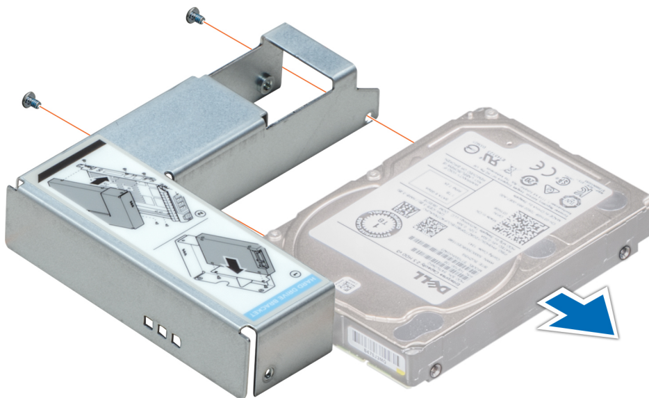
Ilustración 59. Extracción de una unidad de 2,5 pulgadas del adaptador de unidad de 3,5 pulgadas
