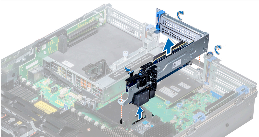
Ilustración 96. Extracción del soporte vertical para tarjetas de expansión 2A
