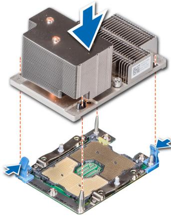
Ilustración 78. Instalación del módulo del disipador de calor y el procesador (2U)
