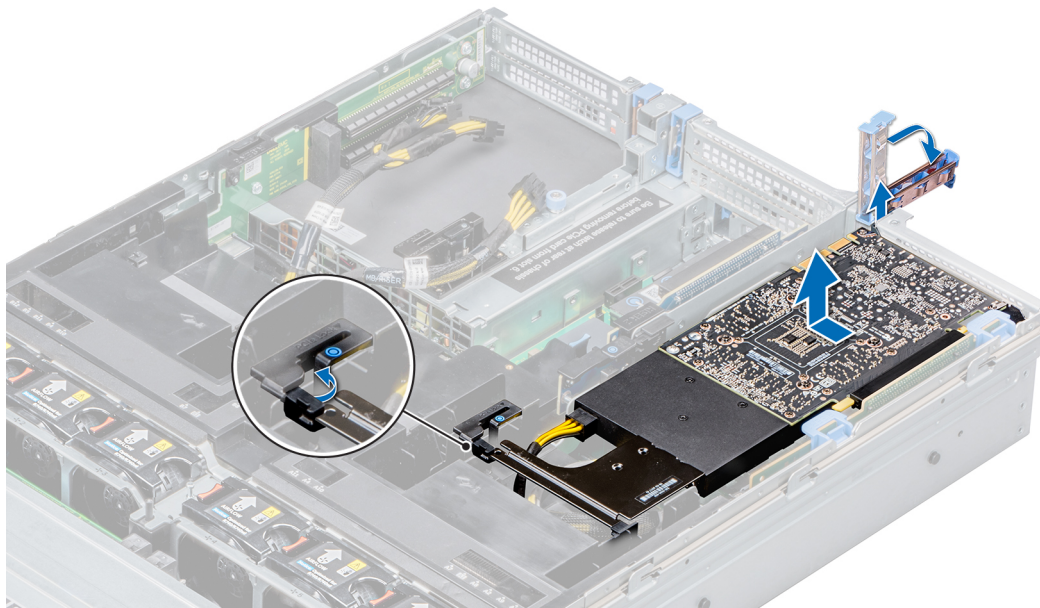
Ilustración 103. Extracción de la GPU 1
