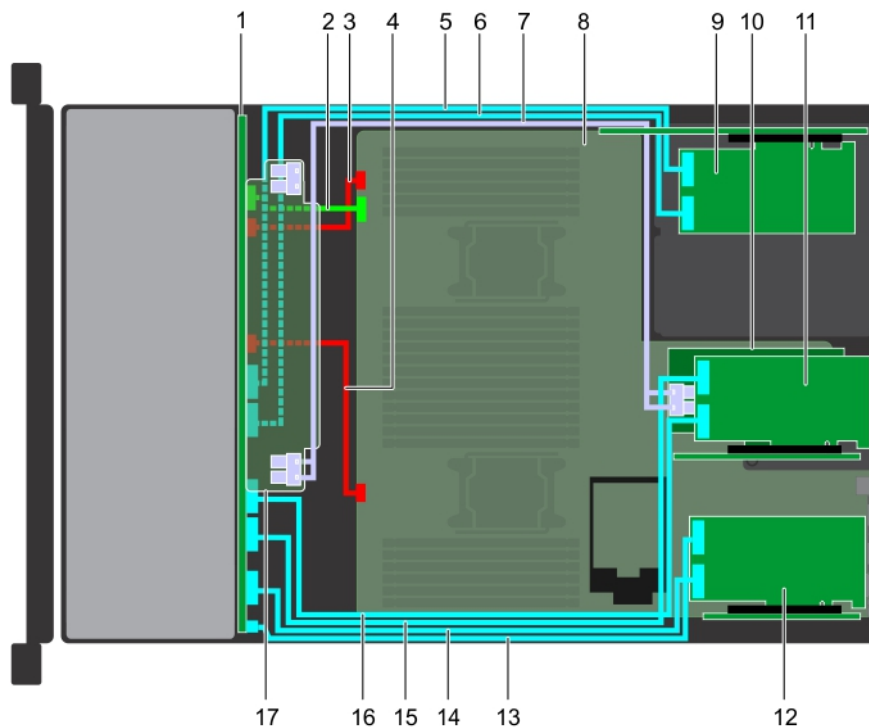
Ilustración 152. Enrutamiento de los cables: backplane de unidad de 24 x 2.5 pulgadas con 12 SAS más 12 PCIe y PERC adaptadora
