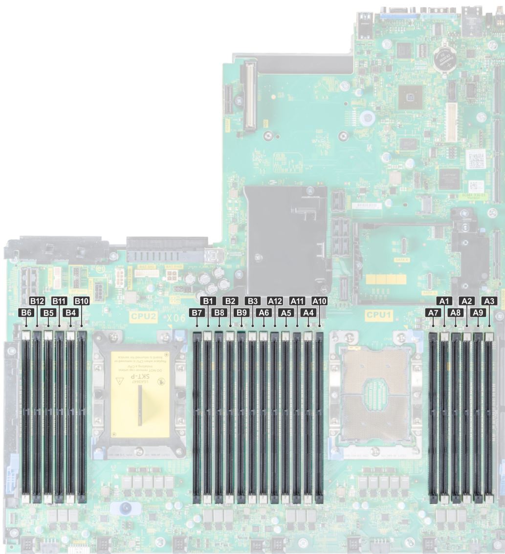
Ilustración 69. Ubicaciones de los sockets de memoria
