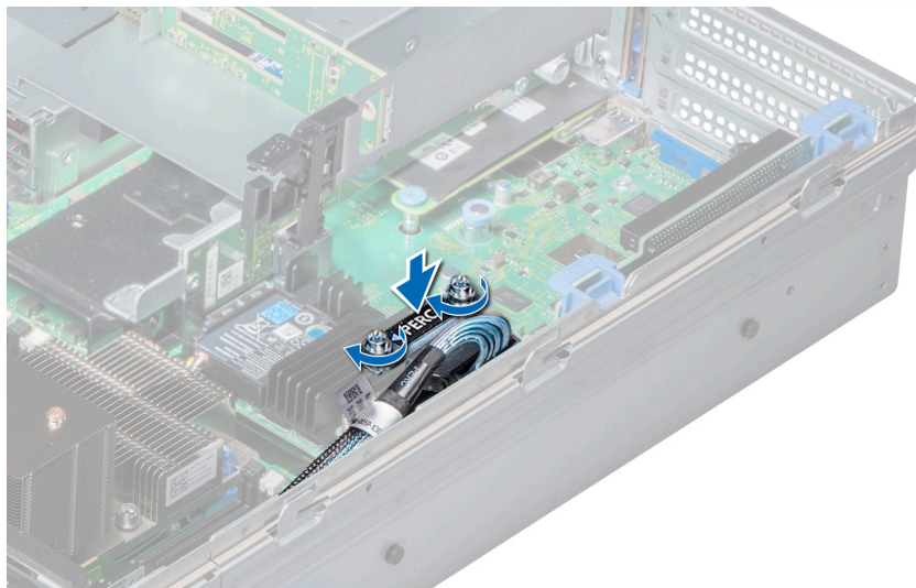
Ilustración 123. Instalación del cable de la tarjeta controladora de almacenamiento integrada
