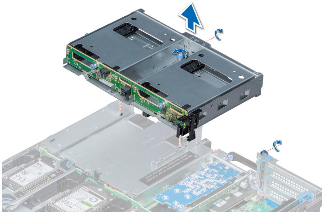
Ilustración 66. Extracción de la canastilla para unidades de 2 x 3.5 pulgadas posterior
