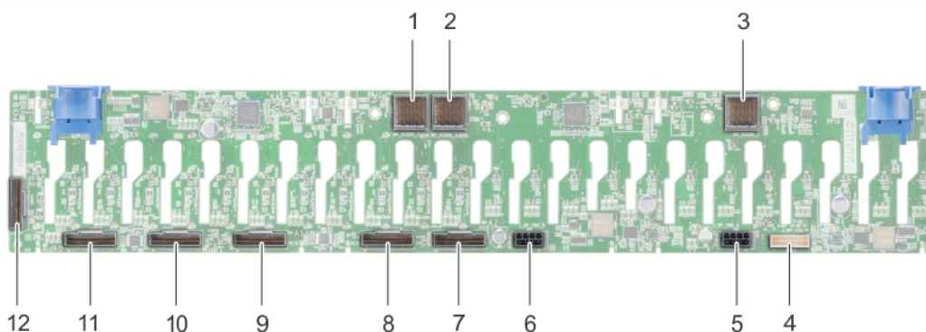
Ilustración 124. Vista posterior del backplane de 24 x 2,5 pulgadas
