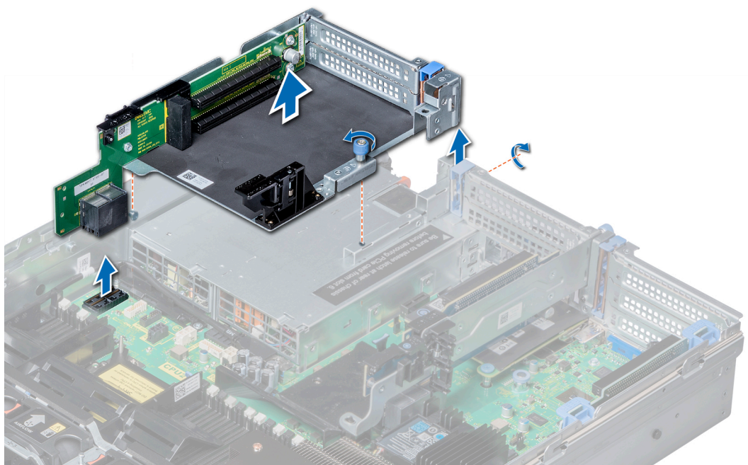
Ilustración 100. Extracción del soporte vertical para tarjetas de expansión 3
