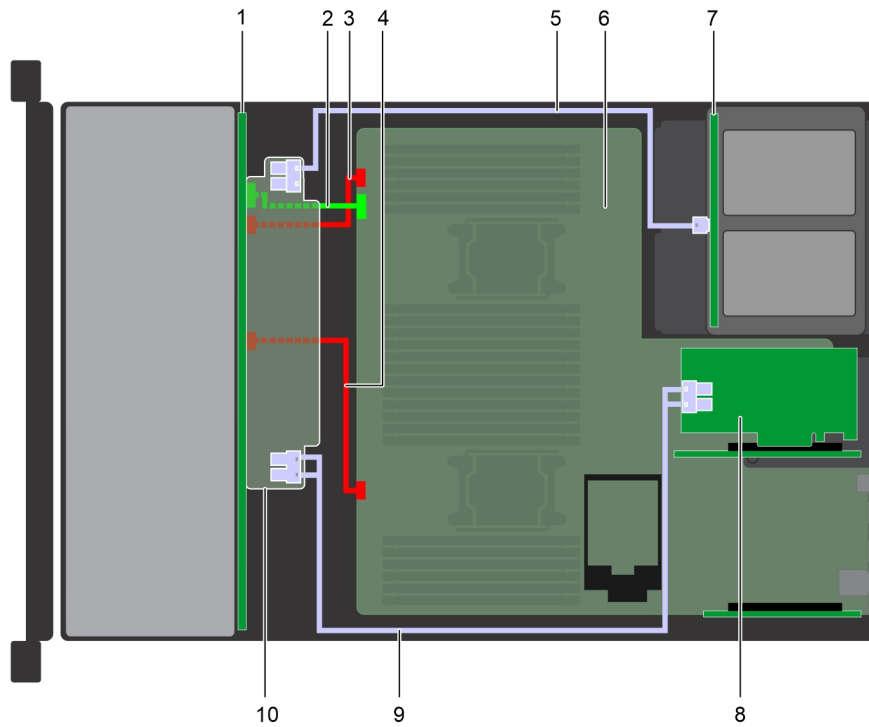
Ilustración 142. Enrutamiento de cables: backplane para 24 unidades de 2,5 pulgadas con backplane para 4 unidades posteriores de 2,5 pulgadas con adaptador de PERC11/HBA
