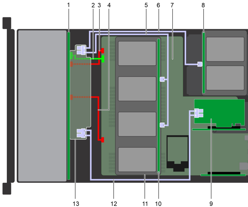
Ilustración 141. Enrutamiento de cables: backplane para 24 unidades de 2,5 pulgadas con backplane para bandeja adaptadora de 4 unidades intermedias de 2,5 pulgadas y backplane para 4 unidades posteriores de 2,5 pulgadas con adaptador de PERC11/HBA
