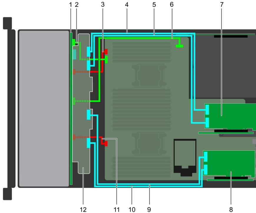
Ilustración 153. Enrutamiento de cables: backplane de unidad NVMe de 24 x 2.5 pulgadas
