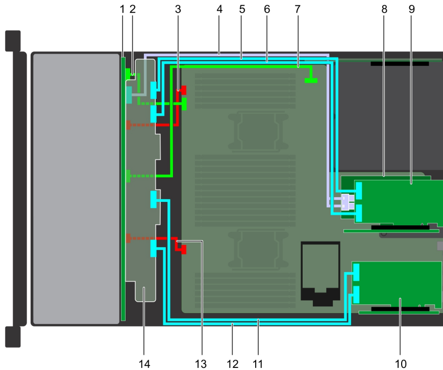
Ilustración 154. Enrutamiento de los cables: backplane de unidad de 24 x 2.5 pulgadas con hasta 24 NVMe o hasta 8 unidades SAS/SATA con NVMe
