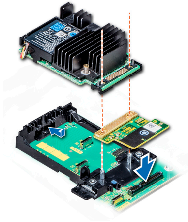
Ilustración 122. Instalación de la tarjeta controladora de almacenamiento integrada
