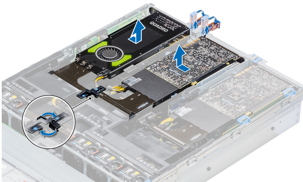
Ilustración 104. Extracción de la GPU 2 y 3
