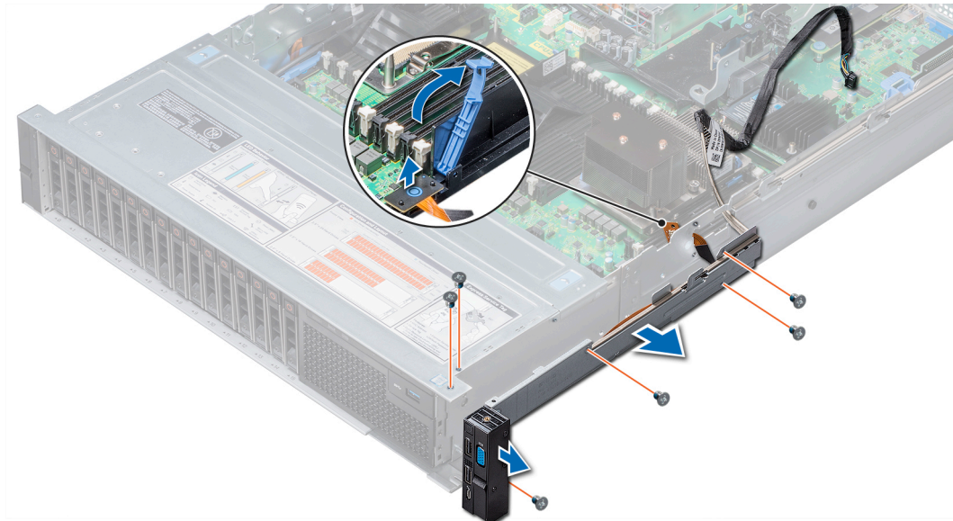
Ilustración 176. Desmontaje del panel de control derecho
