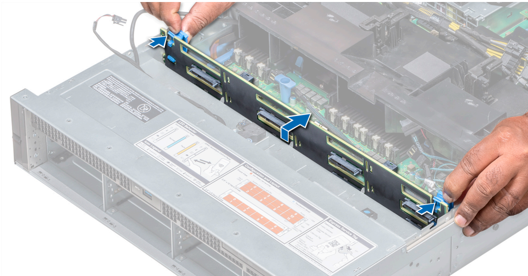
Ilustración 131. Extracción del plano posterior
