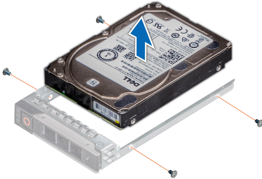
Ilustración 63. Extracción de una unidad del portaunidades
