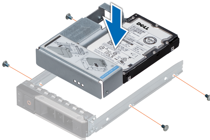
Ilustración 62. Instalación de un adaptador de unidad de 3,5 pulgadas en un portaunidades de 3,5 pulgadas
