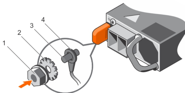
Ilustración 167. Ensamblaje y conexión del cable de toma de tierra de seguridad
