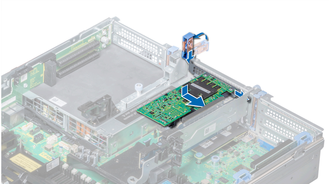
Ilustración 88. Instalación de una tarjeta de expansión en el soporte vertical para tarjetas de expansión 2
