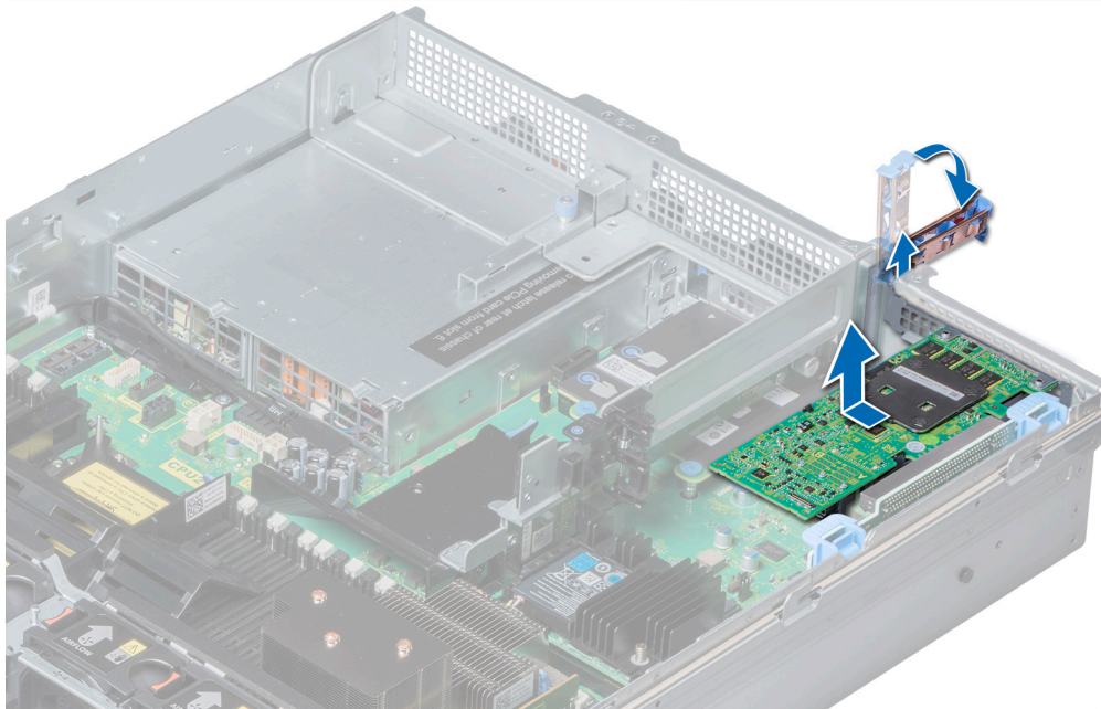
Ilustración 82. Extracción de una tarjeta de expansión del soporte vertical para tarjetas de expansión 1
