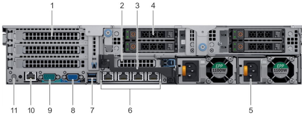
Ilustración 8. Vista posterior de 4 sistemas de unidad de disco de 2,5 pulgadas
