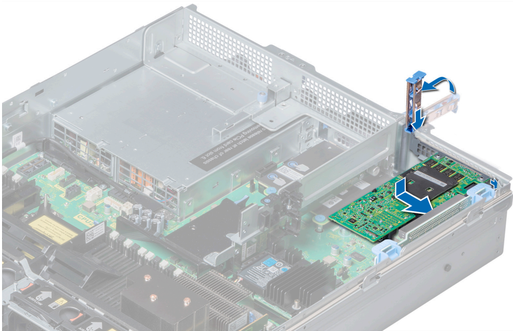
Ilustración 86. Instalación de una tarjeta de expansión en el soporte vertical para tarjetas de expansión 1
