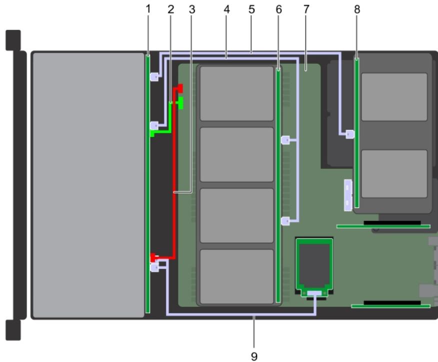
Ilustración 158. Enrutamiento de los cables: backplane de unidad de 12 x 3.5 pulgadas con backplane de bandeja de unidad intermedia de 4 x 3.5 pulgadas (adaptador de 4 x 2.5 pulgadas) y backplane de unidad posterior de 4 x 2.5 pulgadas
