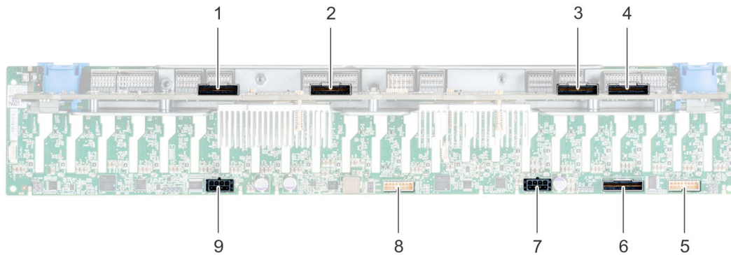
Ilustración 125. Vista posterior del backplane de 24 x 2,5 pulgadas (24 NVMe)
