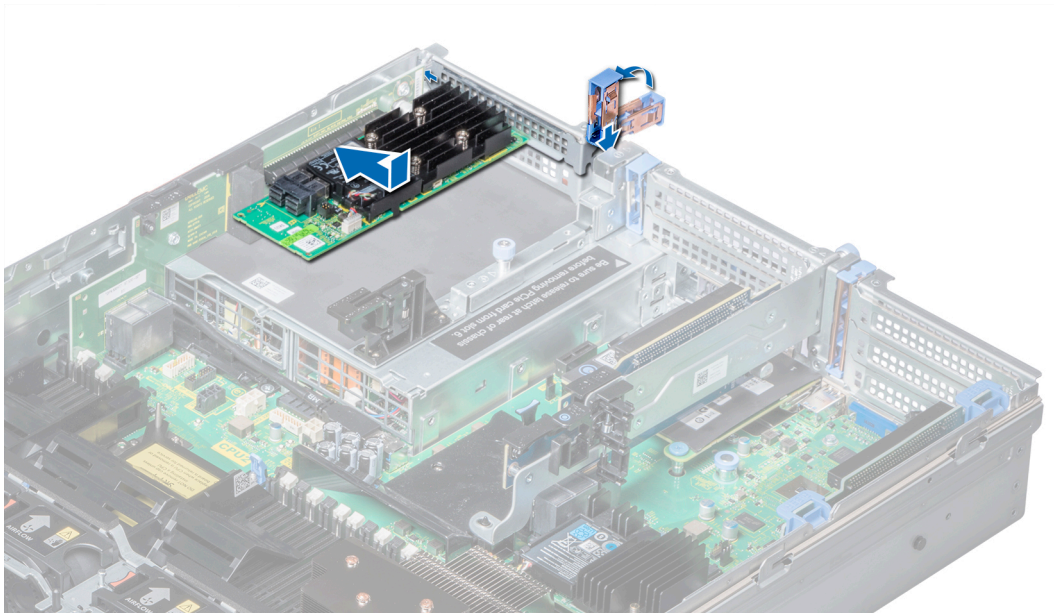
Ilustración 89. Instalación de una tarjeta de expansión en el soporte vertical para tarjetas de expansión 3
