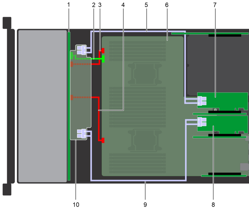
Ilustración 140. Enrutamiento de cables: backplane para 24 unidades de 2,5 pulgadas con adaptador doble de PERC11/HBA
