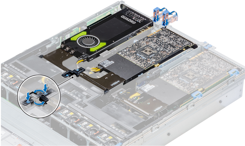
Ilustración 111. Asegurar las GPU 2 y 3
