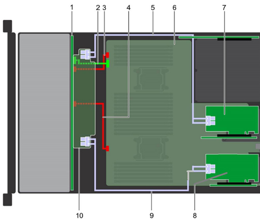
Ilustración 139. Enrutamiento de cables: backplane para 24 unidades de 2,5 pulgadas con adaptador doble de PERC11/HBA
