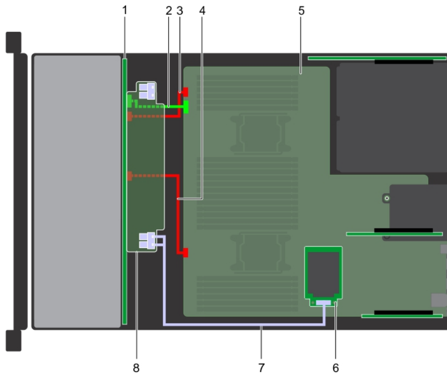
Ilustración 147. Enrutamiento de cables: backplane de 24 x 2.5 pulgadas con miniPERC
