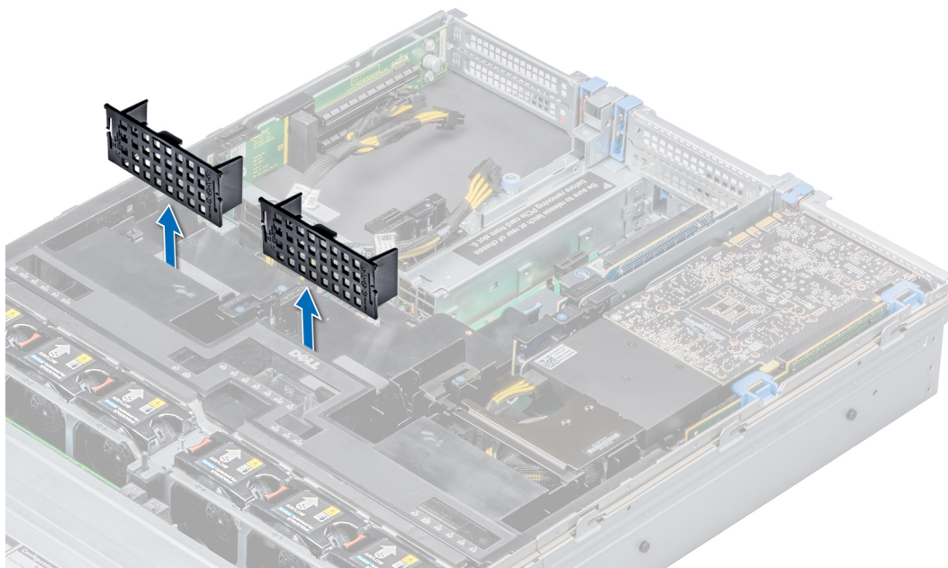
Ilustración 107. Extracción de la cubierta de relleno de las ranuras en la cubierta para flujo de aire de la GPU
