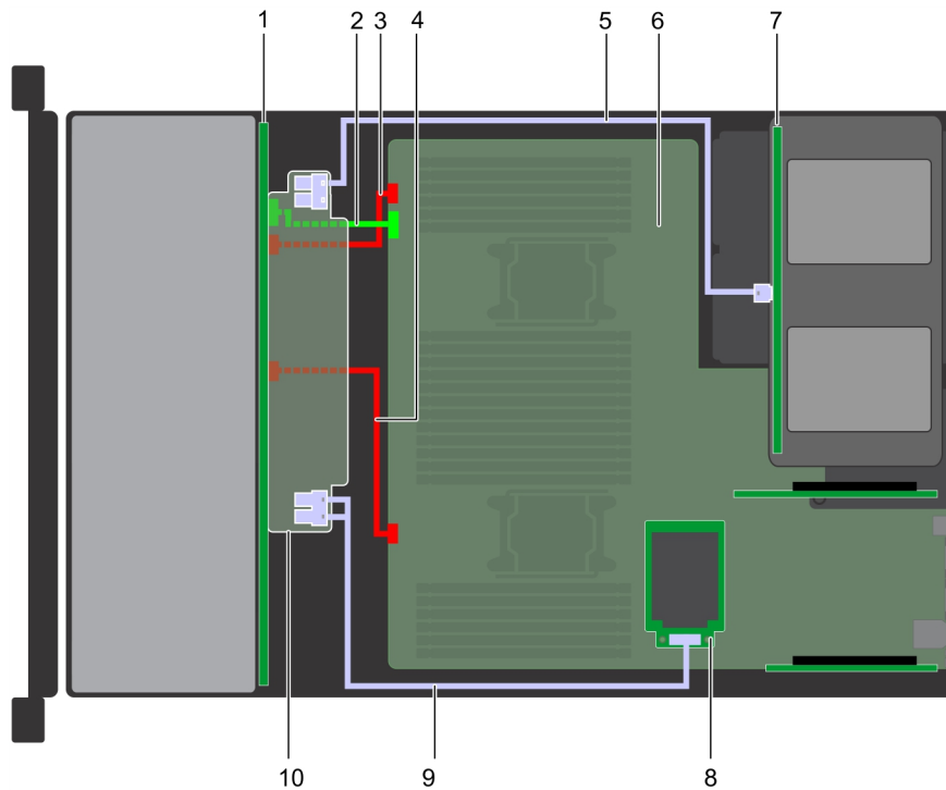
Ilustración 151. Enrutamiento de los cables: backplane de unidad de 24 x 2.5 pulgadas con backplane de unidad posterior de 4 x 2.5 pulgadas
