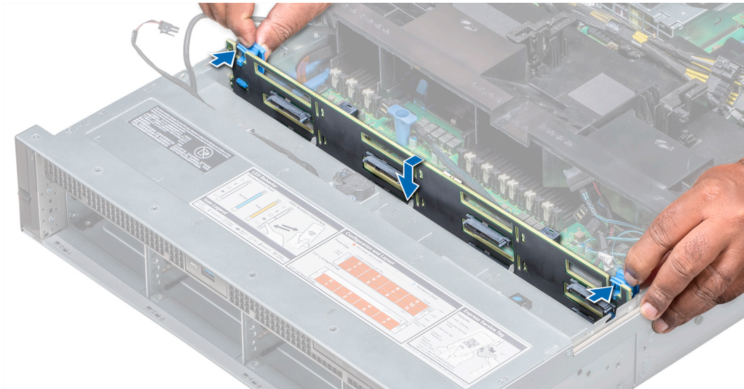
Ilustración 132. Instalación del plano posterior
