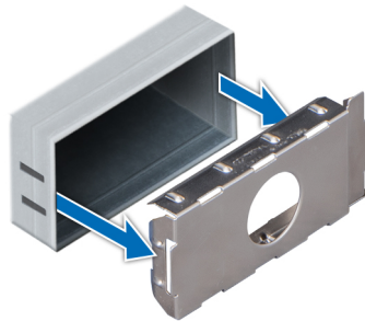
Ilustración 163. Extracción de la unidad de suministro de energía de relleno
