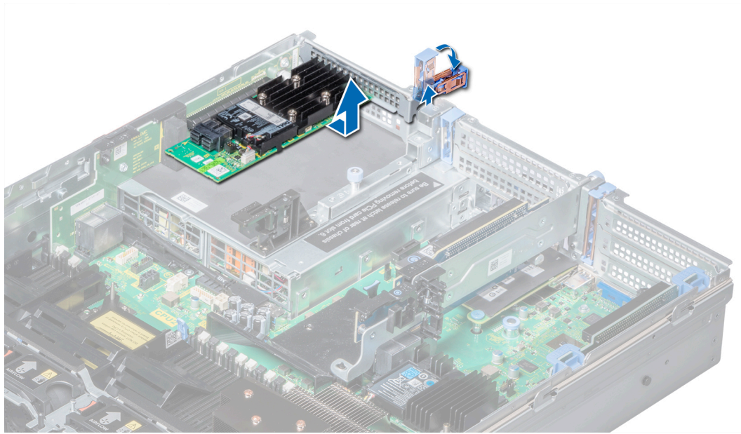
Ilustración 85. Extracción de una tarjeta de expansión del soporte vertical para tarjetas de expansión 3
