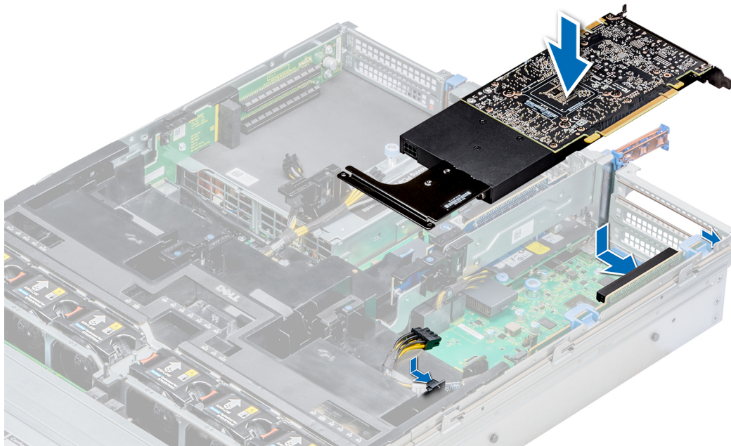
Ilustración 108. Instalación de la GPU 1
