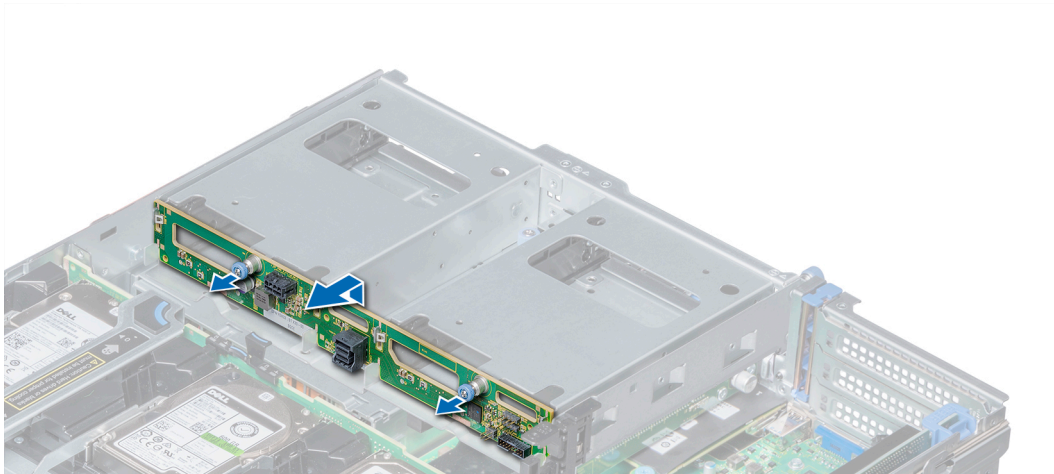
Ilustración 135. Extracción del backplane de unidad de 3.5 pulgadas posterior
