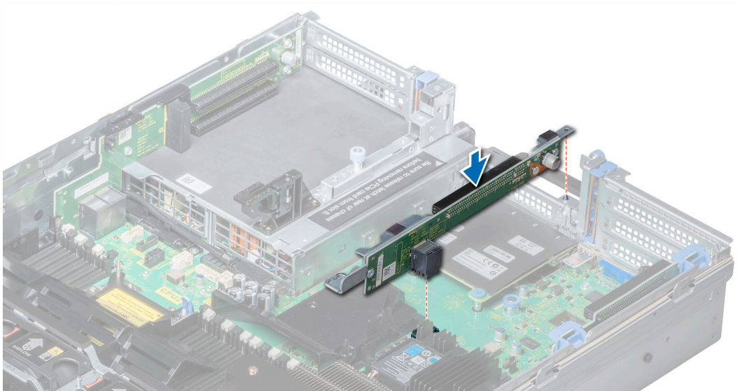
Ilustración 99. Instalación del soporte vertical para tarjetas de expansión 2
