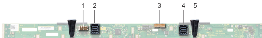
Ilustración 127. Vista posterior del backplane de 3,5 pulgadas (bandeja de unidad intermedia)
