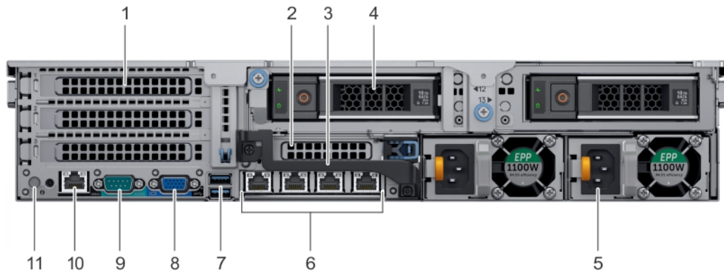
Ilustración 9. Vista posterior de 2 sistemas de unidad de disco de 3,5 pulgadas
