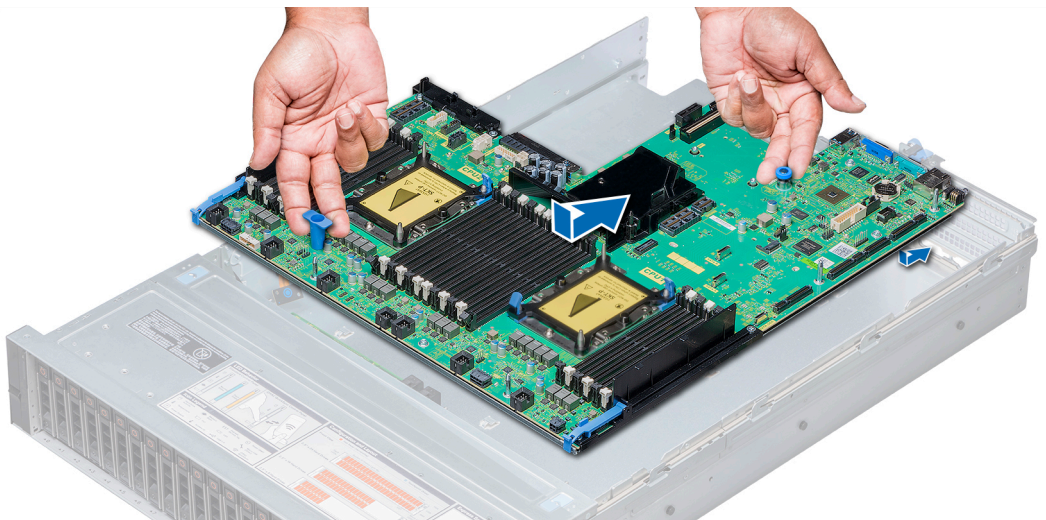
Ilustración 172. Instalación de la tarjeta madre del sistema
