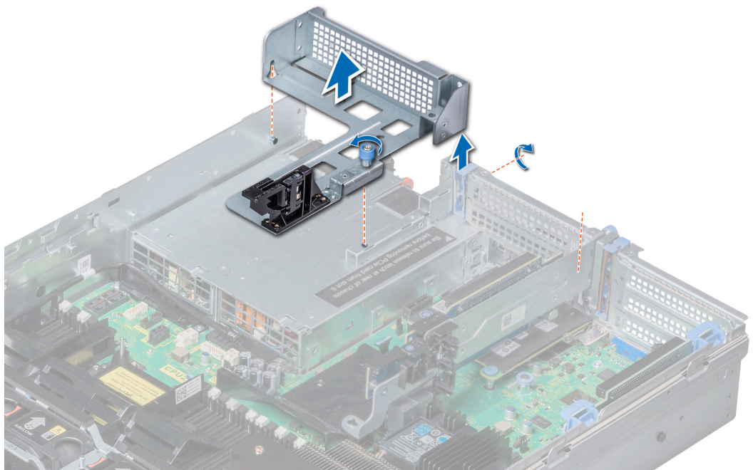
Ilustración 92. Extracción del soporte vertical de relleno 3
