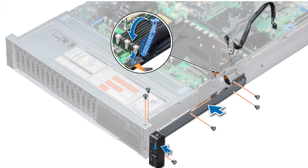
Ilustración 177. Instalación del panel de control derecho
