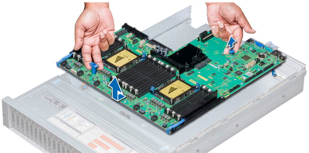
Ilustración 171. Extracción de la tarjeta madre del sistema
