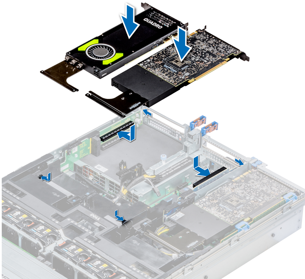
Ilustración 110. Instalación de las GPU 2 y 3
