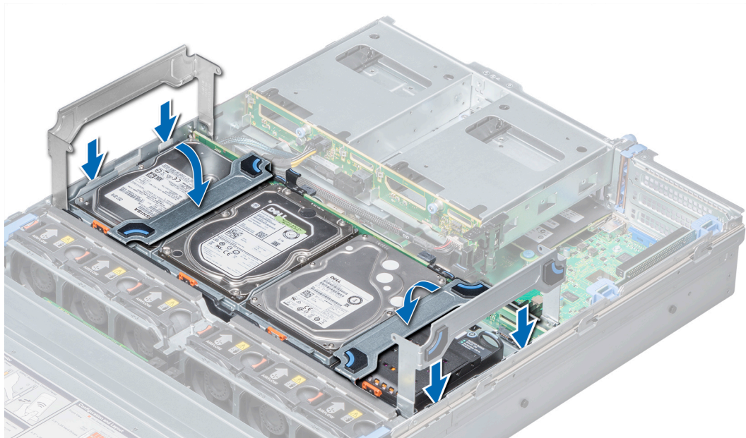
Ilustración 46. Instalación de la bandeja de unidad intermedia
