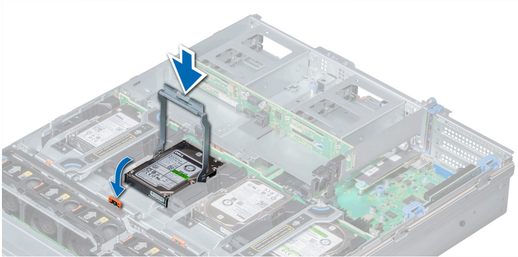
Ilustración 50. Instalación de un portaunidades en la bandeja de unidad intermedia
