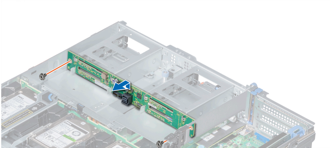
Ilustración 137. Extracción del backplane de unidad de 2.5 pulgadas posterior
