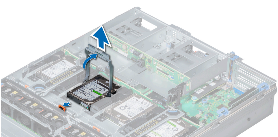
Ilustración 49. Extracción de un portaunidades de la bandeja de unidad intermedia
