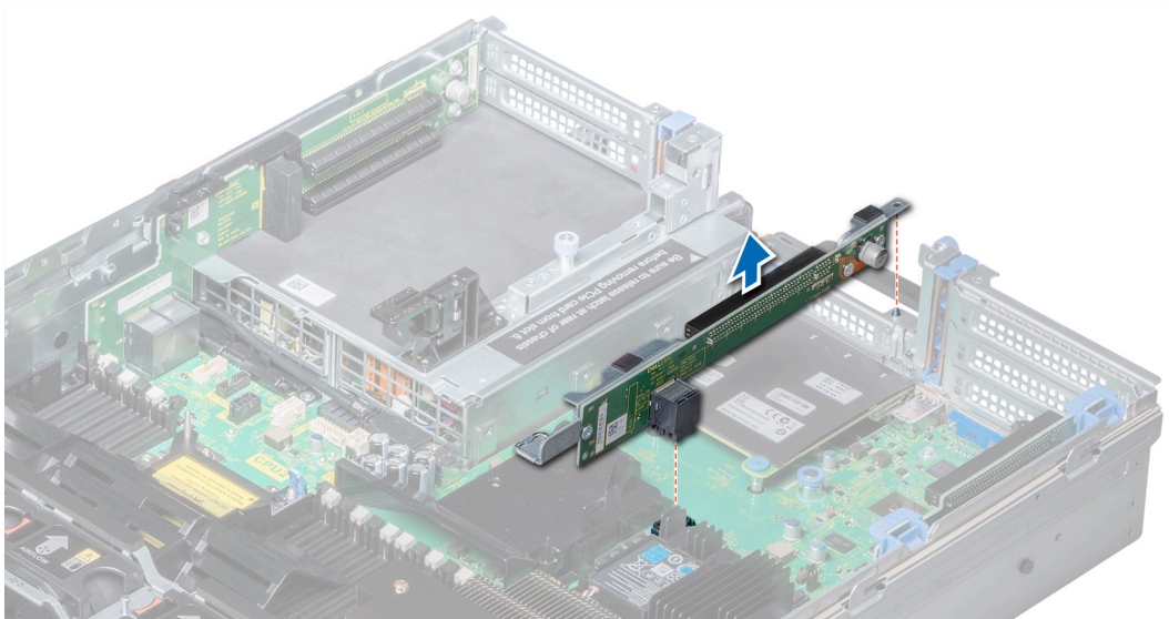
Ilustración 97. Extracción del soporte vertical para tarjetas de expansión 2
