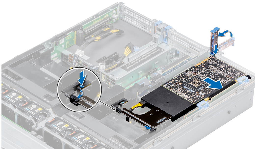
Ilustración 109. Asegurar la GPU 1
