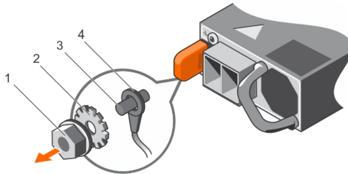
Ilustración 168. Extracción del cable de conexión a tierra de seguridad
