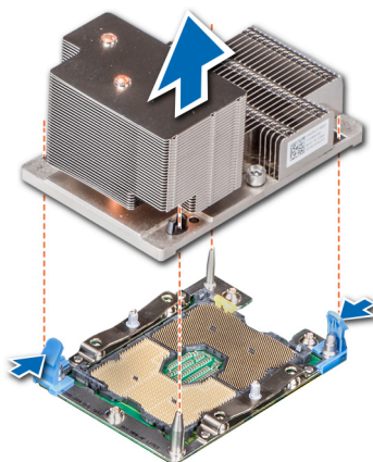
Ilustración 71. Extracción de un módulo del disipador de calor y procesador (2U)
