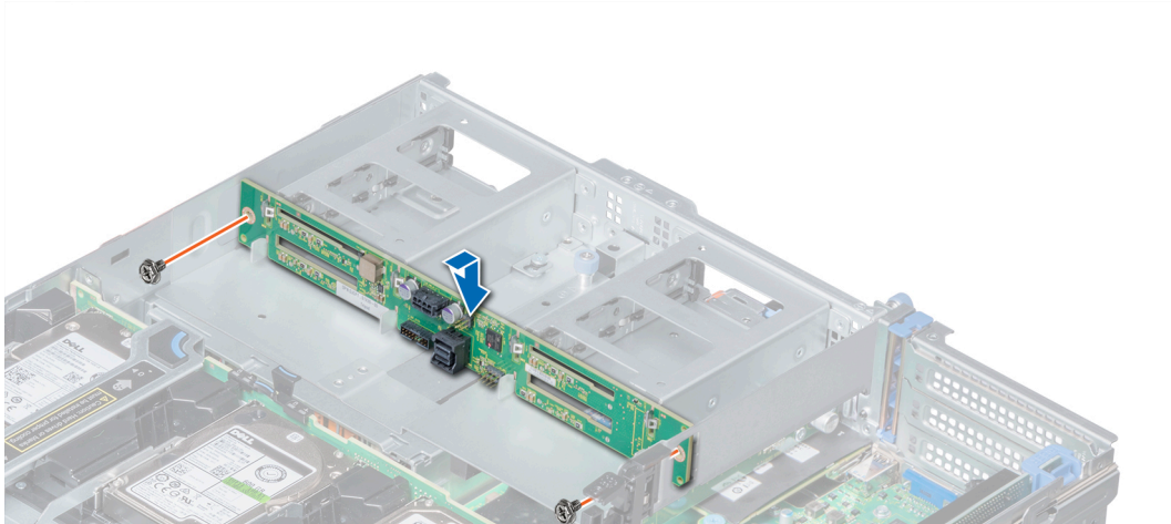
Ilustración 138. Instalación del backplane de la unidad de 2.5 pulgadas posterior
