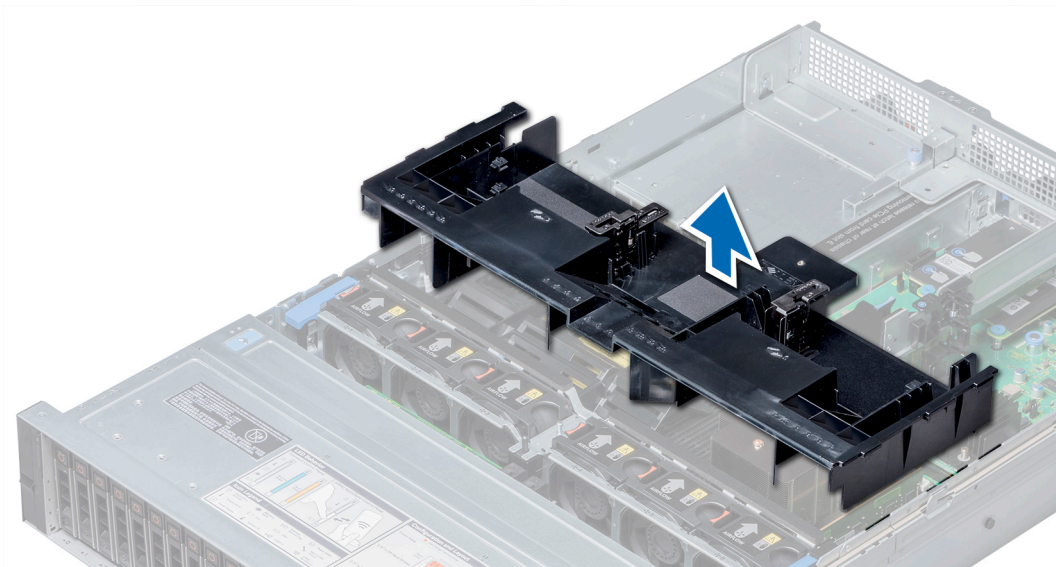
Ilustración 31. Extracción de la cubierta para aire
