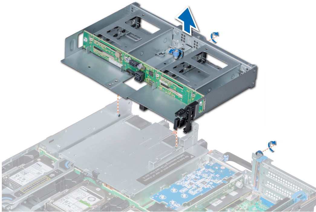
Ilustración 65. Extracción de la canastilla para unidades de 4 x 2.5 pulgadas posterior
