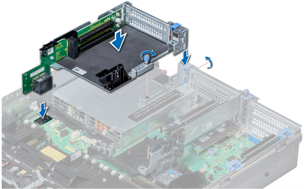
Ilustración 101. Instalación de soportes verticales para tarjetas de expansión
