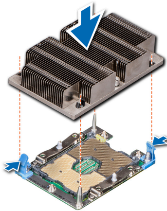
Ilustración 79. Instalación del módulo del disipador de calor y el procesador (1U)
