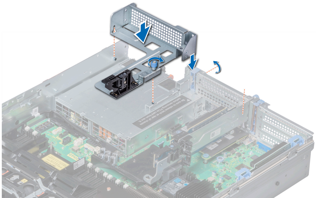
Ilustración 93. Instalación del soporte vertical de relleno 3
