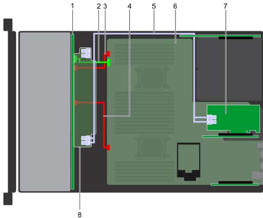
Ilustración 148. Enrutamiento de los cables: backplane de unidad de 24 x 2.5 pulgadas con PERC adaptadora
