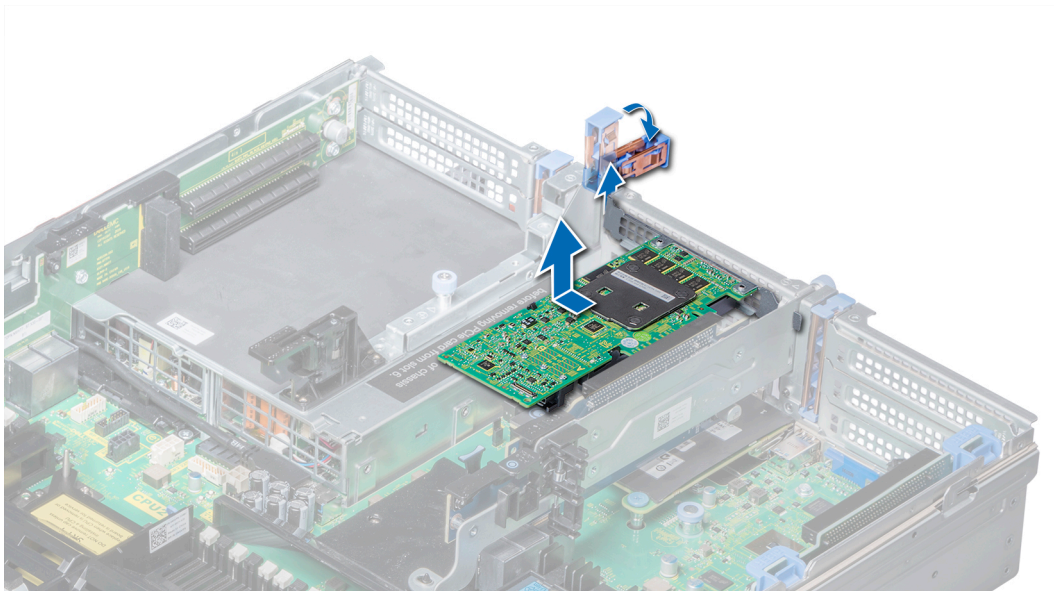
Ilustración 84. Extracción de una tarjeta de expansión del soporte vertical para tarjetas de expansión 2
