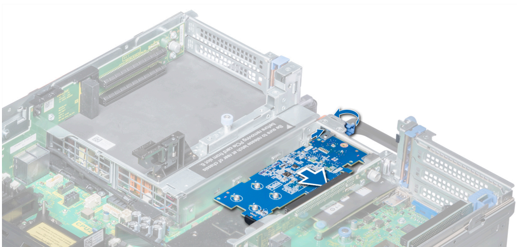
Ilustración 87. Instalación de una tarjeta de expansión en el soporte vertical para tarjetas de expansión 2B
