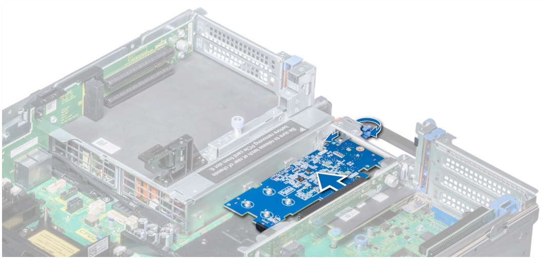
Ilustración 83. Extracción de una tarjeta de expansión del soporte vertical para tarjetas de expansión 2B
