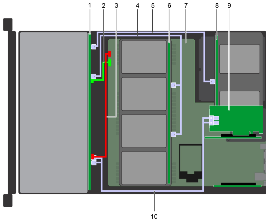
Ilustración 143. Enrutamiento de cables: backplane para 12 unidades de 3,5 pulgadas con backplane para bandeja (adaptadora para 4 de 2,5 pulgadas) de 4 unidades intermedias de 3,5 pulgadas y backplane para 4 unidades posteriores de 2,5 pulgadas con adaptador de PERC11/HBA
