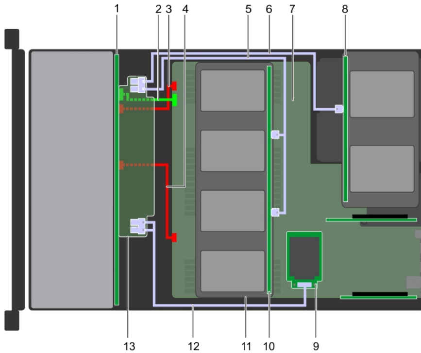
Ilustración 150. Enrutamiento de los cables: backplane de unidad de 24 x 2.5 pulgadas con backplane de bandeja de unidad intermedia adaptadora de 4 x 2.5 pulgadas y backplane de unidad posterior de 4 x 2.5 pulgadas
