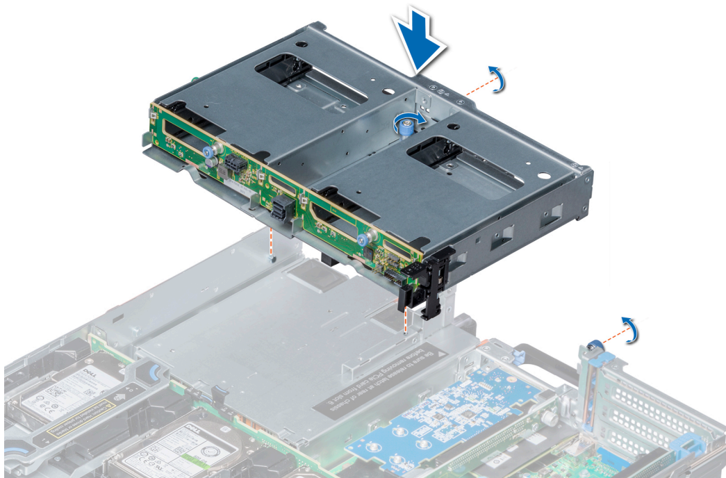
Ilustración 68. Instalación de una canastilla para unidades posterior de 2 x 3.5 pulgadas
