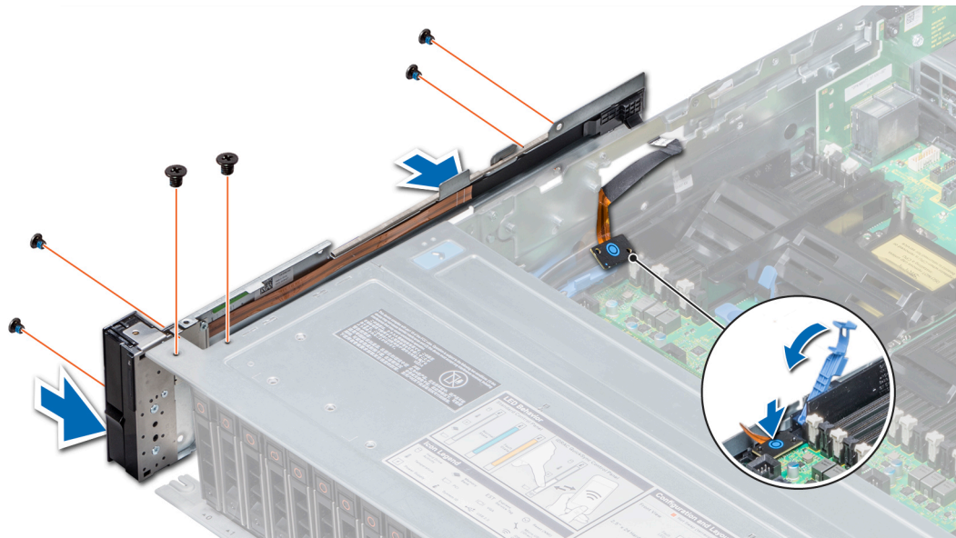
Ilustración 175. Instalación del panel de control izquierdo
