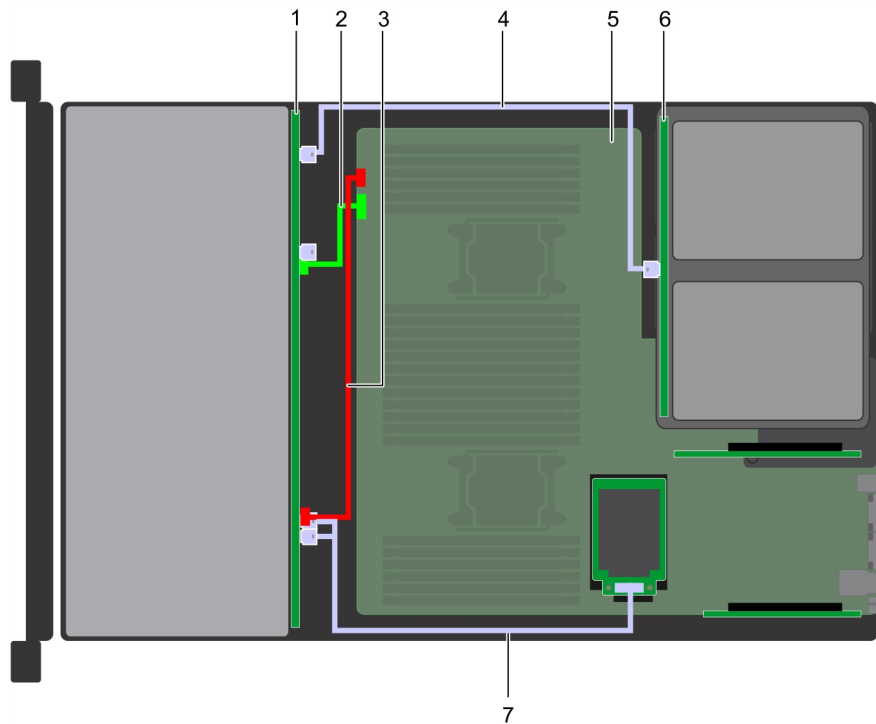
Ilustración 159. Enrutamiento de los cables: backplane de unidad de 12 x 3.5 pulgadas con backplane de unidad posterior de 2 x 3.5 pulgadas
