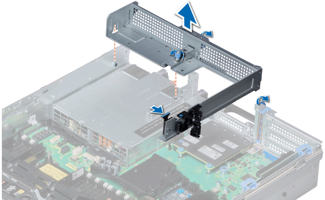
Ilustración 90. Extracción de los soportes verticales de relleno 2 y 3
