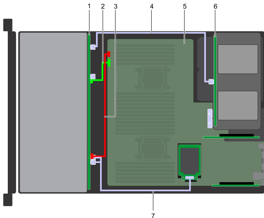
Ilustración 160. Enrutamiento de los cables: backplane de unidad de 12 x 3.5 pulgadas con backplane de unidad posterior de 4 x 2.5 pulgadas
