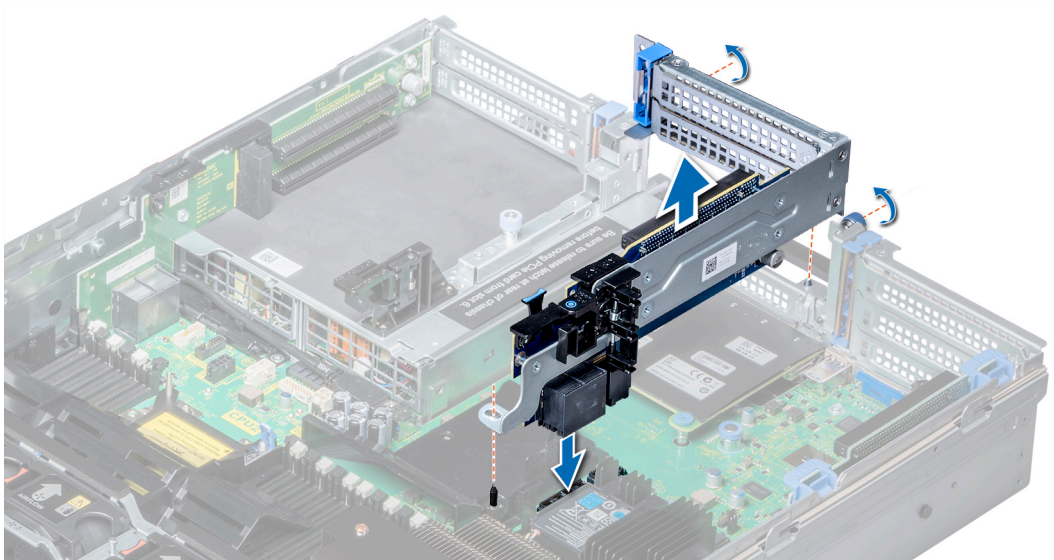
Ilustración 98. Instalación del soporte vertical para tarjetas de expansión 2A
