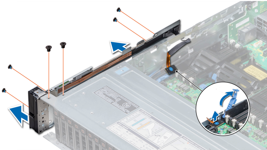
Ilustración 174. Extracción del panel de control izquierdo
