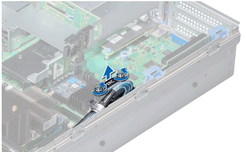
Ilustración 120. Extracción del cable de la controladora de almacenamiento integrada
