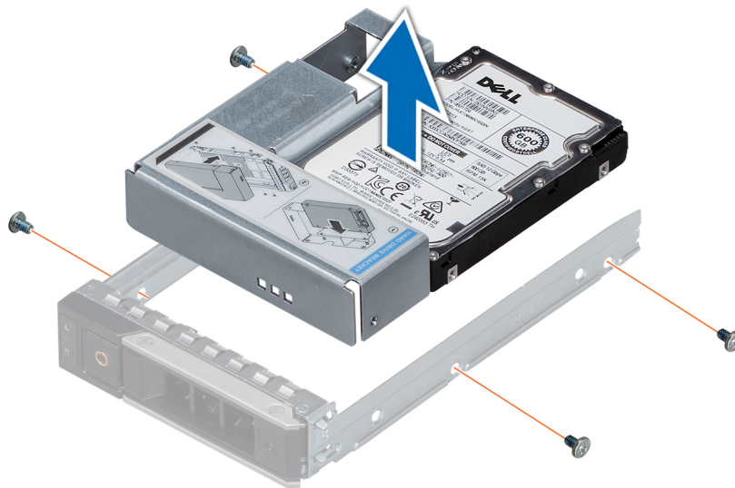
Ilustración 61. Extracción de un adaptador de 3,5 pulgadas de un portaunidades de 3,5 pulgadas
