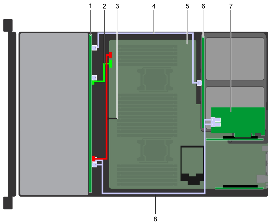
Ilustración 146. Enrutamiento de cables: backplane para 12 unidades de 3,5 pulgadas con backplane para 2 unidades posteriores de 3,5 pulgadas con adaptador de PERC11/HBA
