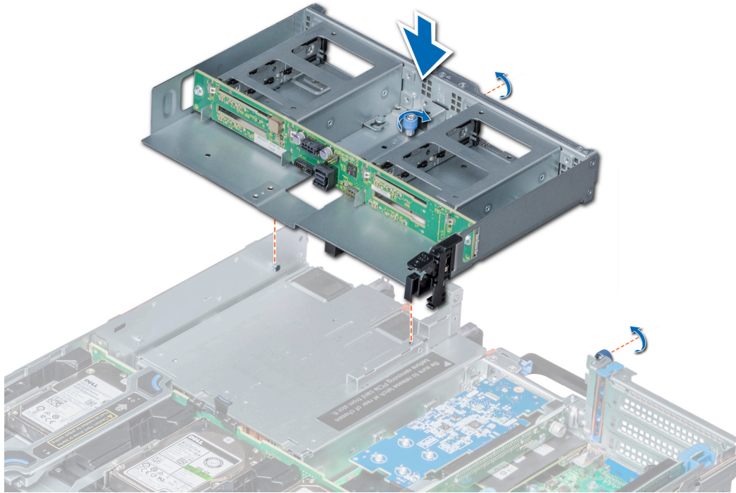
Ilustración 67. Instalación de una canastilla para unidades posterior de 4 x 2.5 pulgadas
