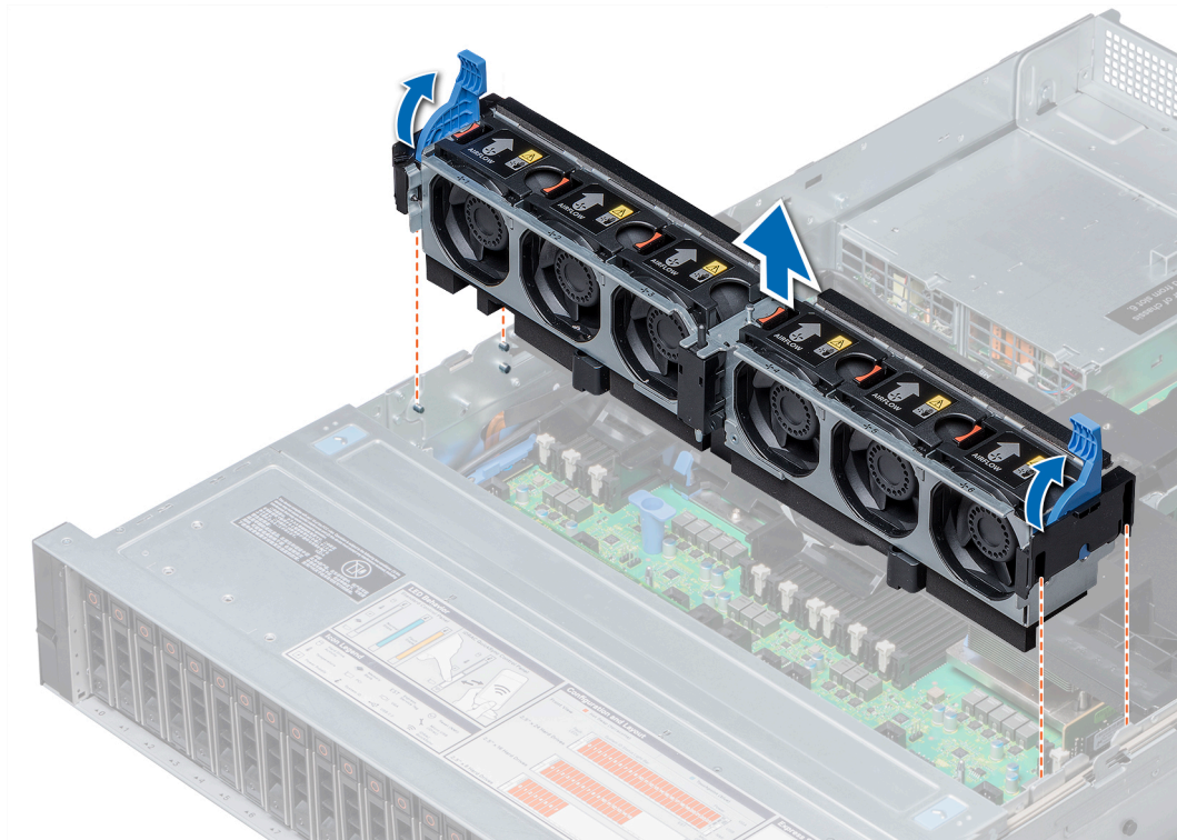
Ilustración 33. Extracción del ensamblaje del ventilador de refrigeración
