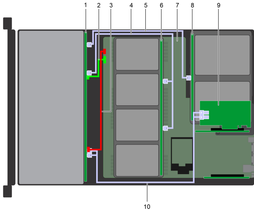
Ilustración 144. Enrutamiento de cables: backplane para 12 unidades de 3,5 pulgadas con backplane para bandeja (adaptadora para 4 de 2,5 pulgadas) de 4 unidades intermedias de 3,5 pulgadas y backplane para 2 unidades posteriores de 3,5 pulgadas con adaptador de PERC11/HBA
