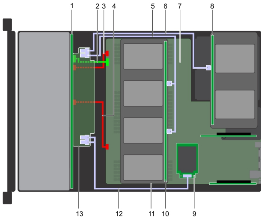
Abbildung 150. Kabelführung – 24 x 2,5-Zoll-Laufwerk-Rückwandplatine mit 4 x 2,5-Zoll-Adapter-Rückwandplatte des mittleren Laufwerkfachs und hintere 4 x 2,5-Zoll-Laufwerk-Rückwandplatine
