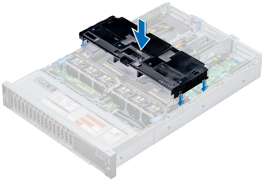
Abbildung 105. Installieren des GPU-Kühlgehäuses
