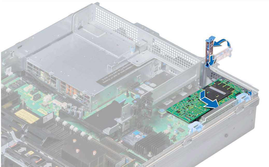
Abbildung 86. Installieren einer Erweiterungskarte in Erweiterungskarten-Riser 1
