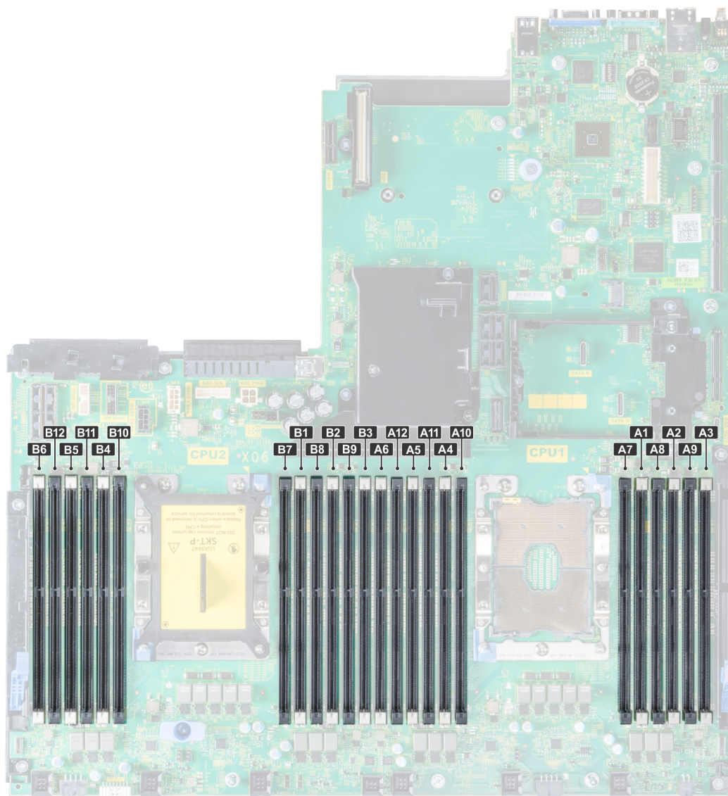
Abbildung 69. Positionen der Speichersockel
