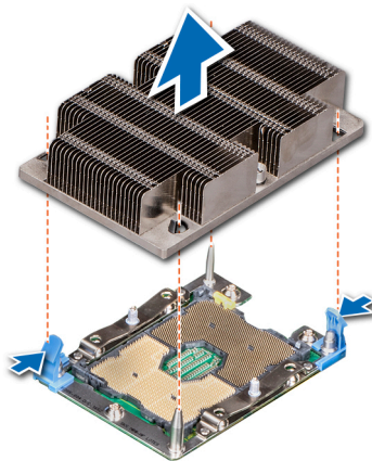
Abbildung 72. Entfernen eines Prozessor- und Kühlkörpermoduls (1HE)
