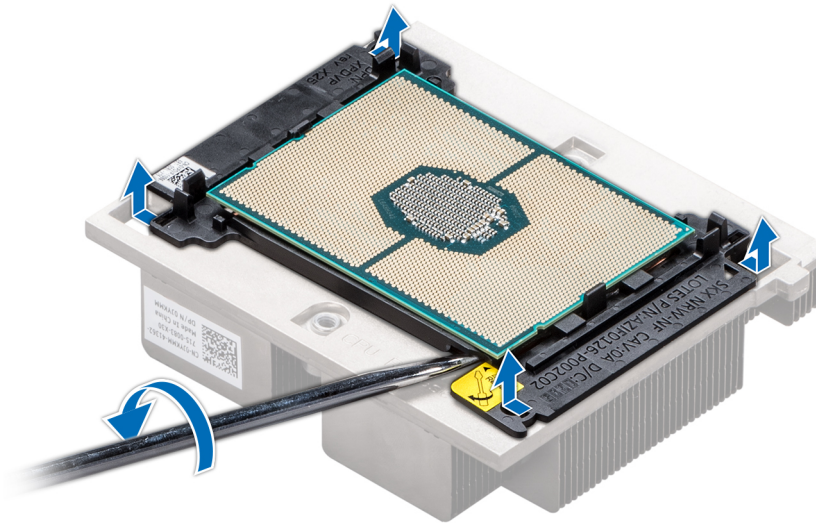
Abbildung 73. Das Lösen der Prozessorhalterung
