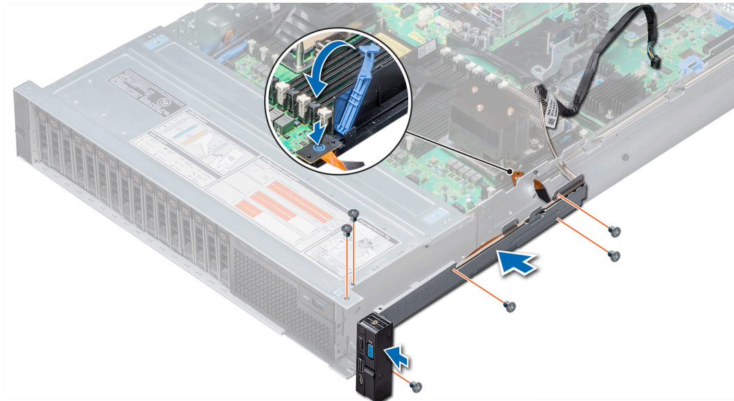
Abbildung 177. Installieren des rechten Bedienfelds
