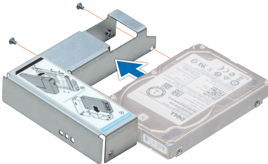
Abbildung 60. Installieren eines 2,5-Zoll-Laufwerks in einem 3,5-Zoll-Laufwerkadapter
