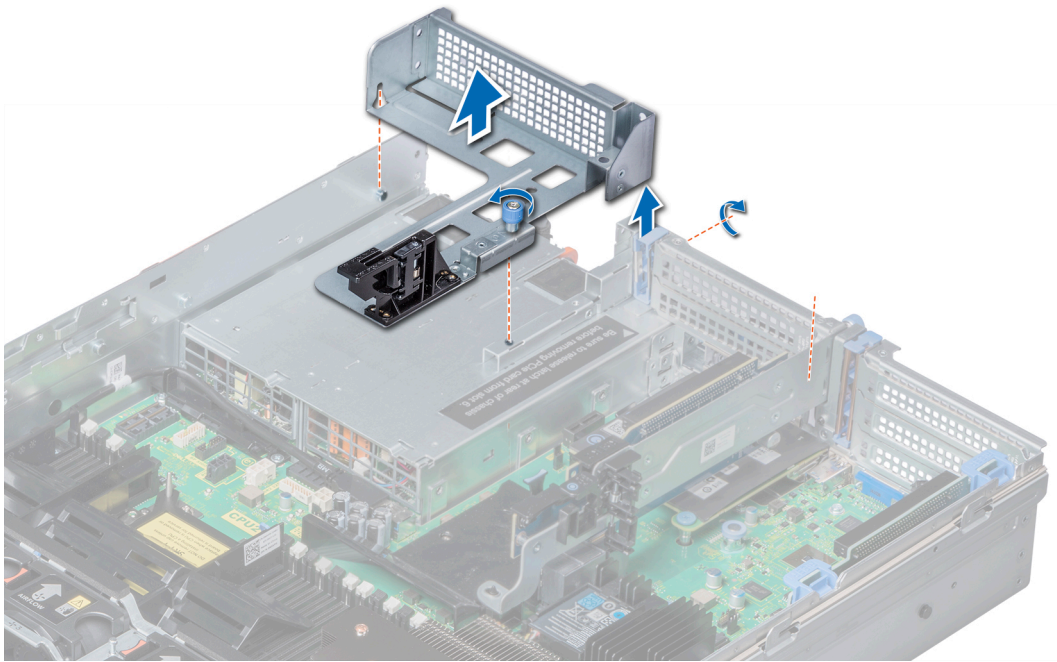
Abbildung 92. Entfernen des Platzhalters für Riser 3
