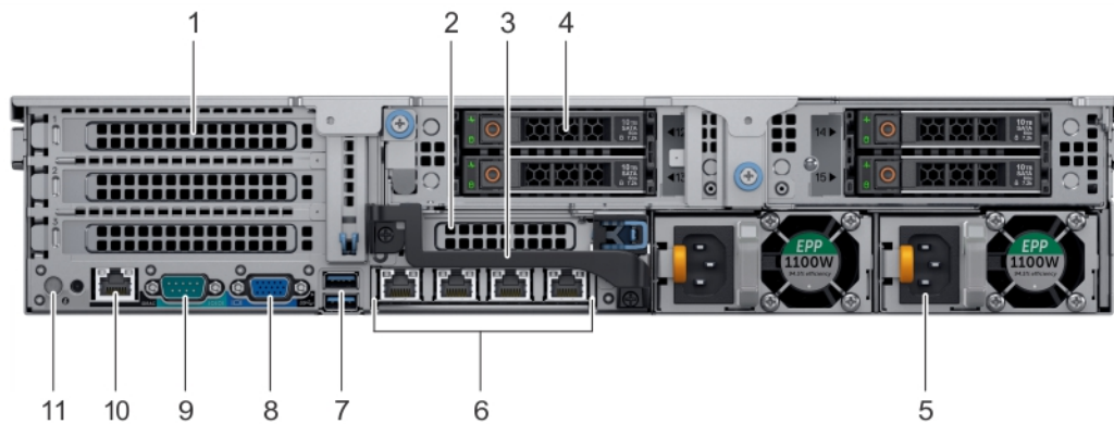
Abbildung 8. Rückansicht des Systems mit 4 x 2,5-Zoll-Laufwerken
