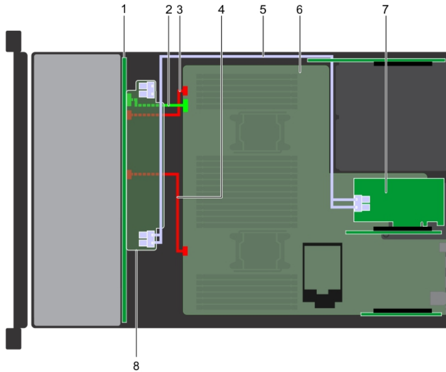
Abbildung 148. Kabelführung – 24 x 2,5-Zoll-Laufwerk-Rückwandplatine mit Adapter-PERC
