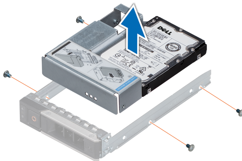
Abbildung 61. Entfernen des 3,5-Zoll-Adapters aus dem 3,5-Zoll-Laufwerkträger
