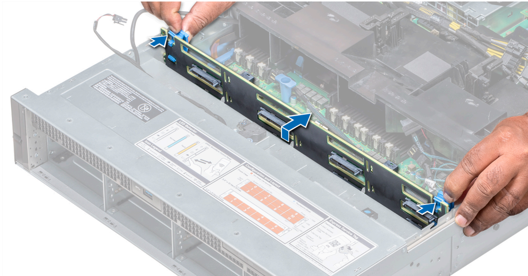
Abbildung 131. Entfernen der Rückwandplatine
