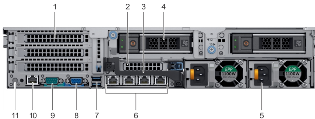
Abbildung 9. Rückansicht des Systems mit 2 x 3,5-Zoll-Laufwerken
