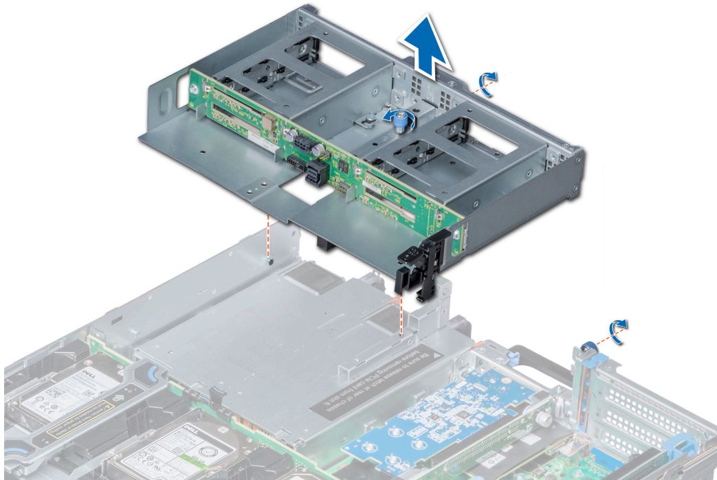
Abbildung 65. Entfernen des hinteren 4 x 2,5-Zoll-Laufwerksgehäuses
