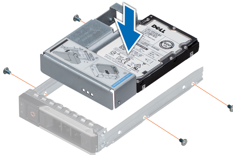
Abbildung 62. Installieren eines 3,5-Zoll-Adapters in einem 3,5-Zoll-Laufwerkträger
