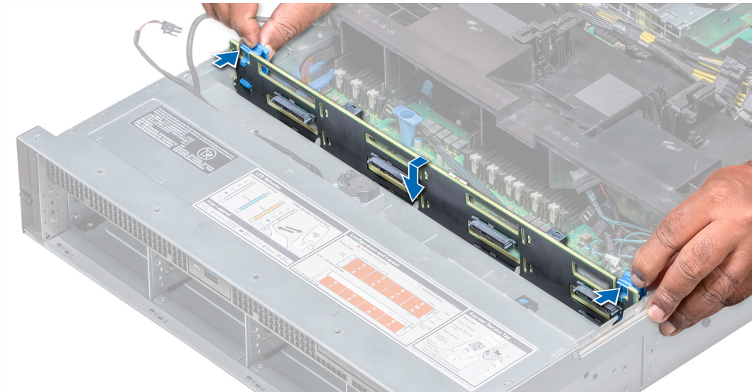
Abbildung 132. Installieren der Rückwandplatine
