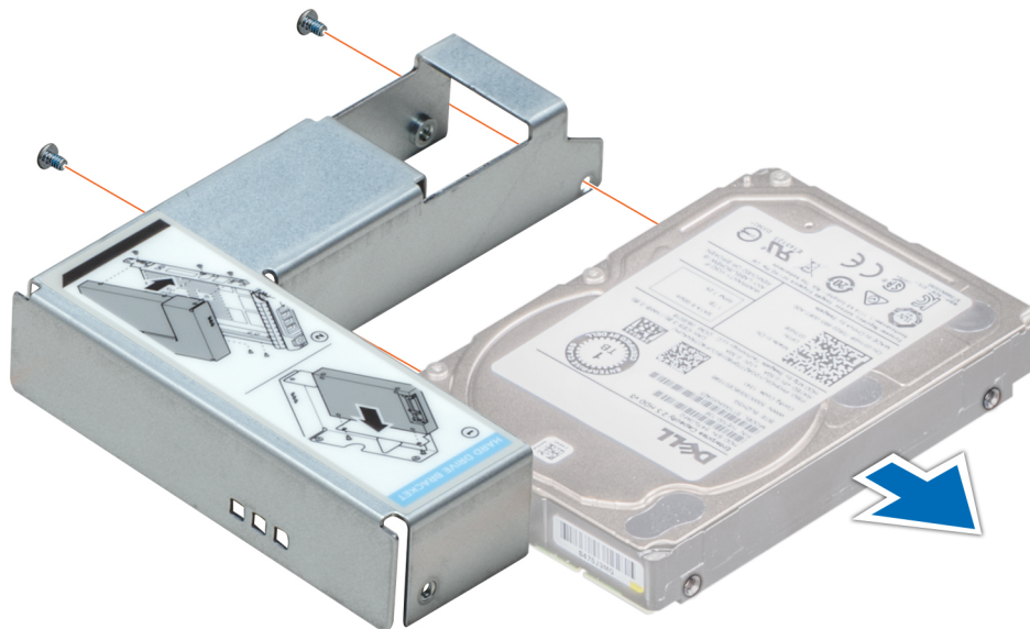
Abbildung 59. Entfernen eines 2,5-Zoll-Laufwerks aus einem 3,5-Zoll-Laufwerkadapter
