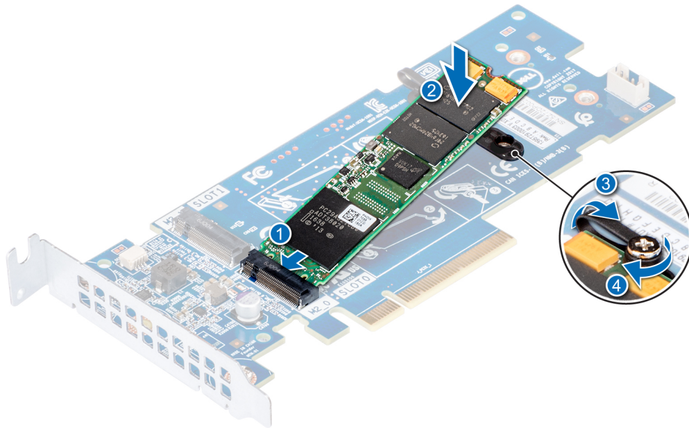
Abbildung 115. Installieren des M.2-SSD-Moduls
