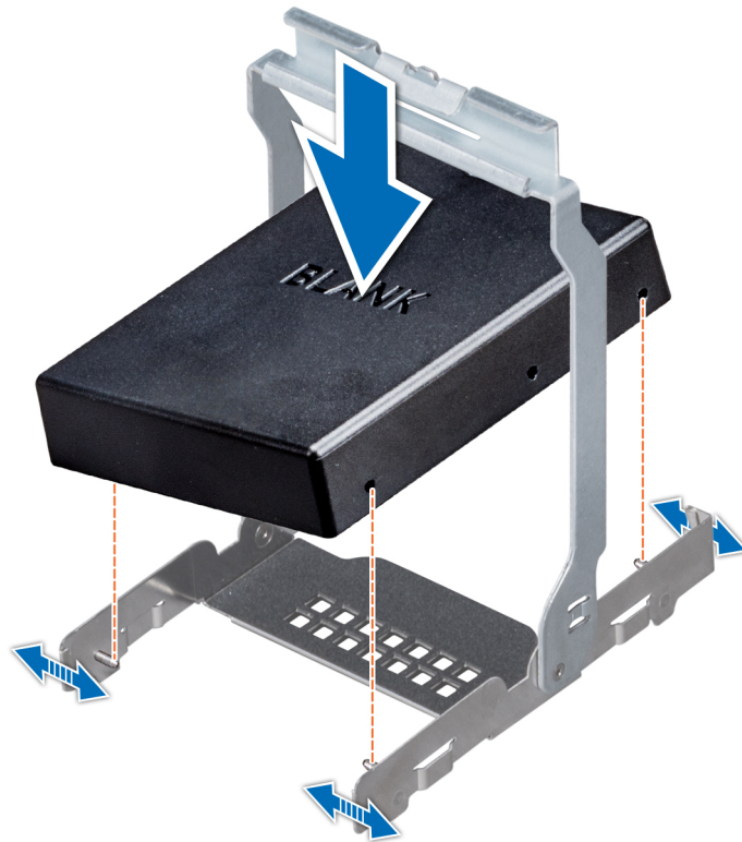
Abbildung 48. Installieren eines Laufwerkplatzhalters im mittleren Laufwerkträger
