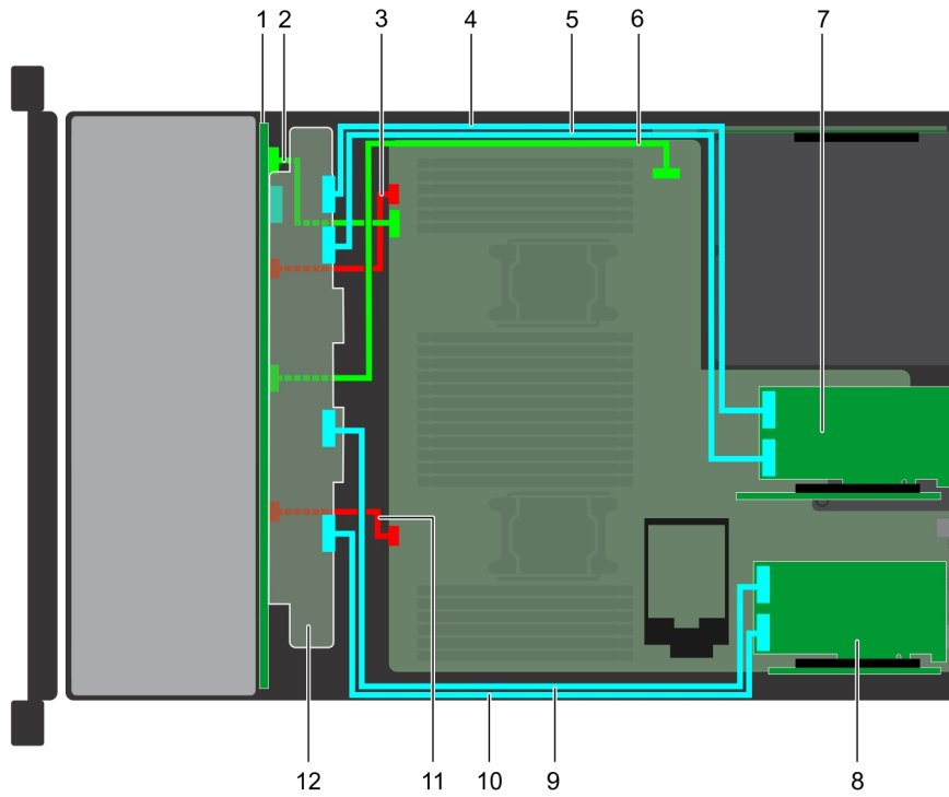
Abbildung 153. Kabelführung – 24 x 2,5-Zoll-NVMe-Laufwerk-Rückwandplatine
