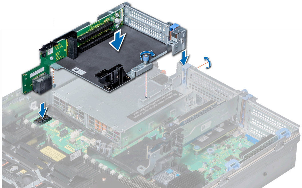
Abbildung 101. Einsetzen des Erweiterungskarten-Risers 3
