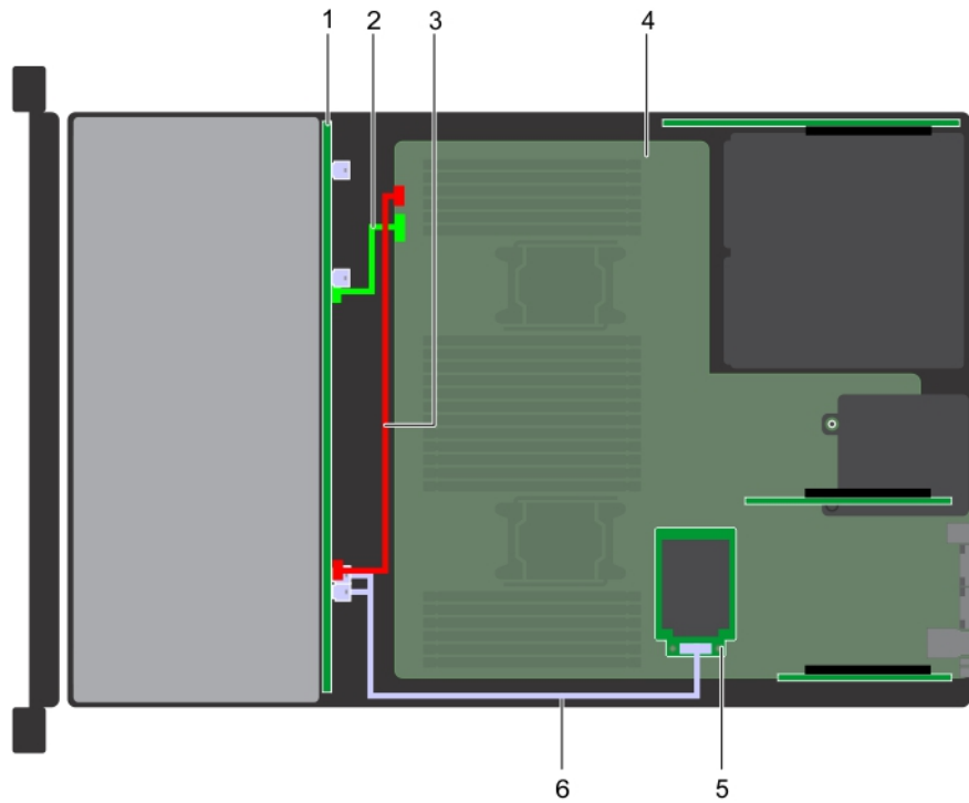
Abbildung 155. Kabelführung – 12 x 3,5-Zoll-Laufwerk-Rückwandplatine mit Mini-PERC
