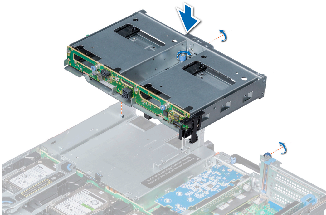
Abbildung 68. Einsetzen des hinteren 2 x 3,5-Zoll-Laufwerksgehäuses
