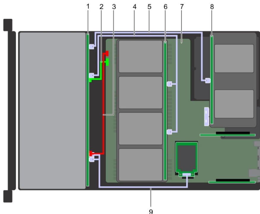
Abbildung 158. Kabelführung – 12 x 3,5-Zoll-Laufwerk-Rückwandplatine mit 4 x 3,5-Zoll-Rückwandplatine des mittleren Laufwerkfachs (mit 4 x 2,5-Zoll-Laufwerksadapter) und 4 x 2,5-Zoll-Laufwerk-Rückwandplatine (hinten)
