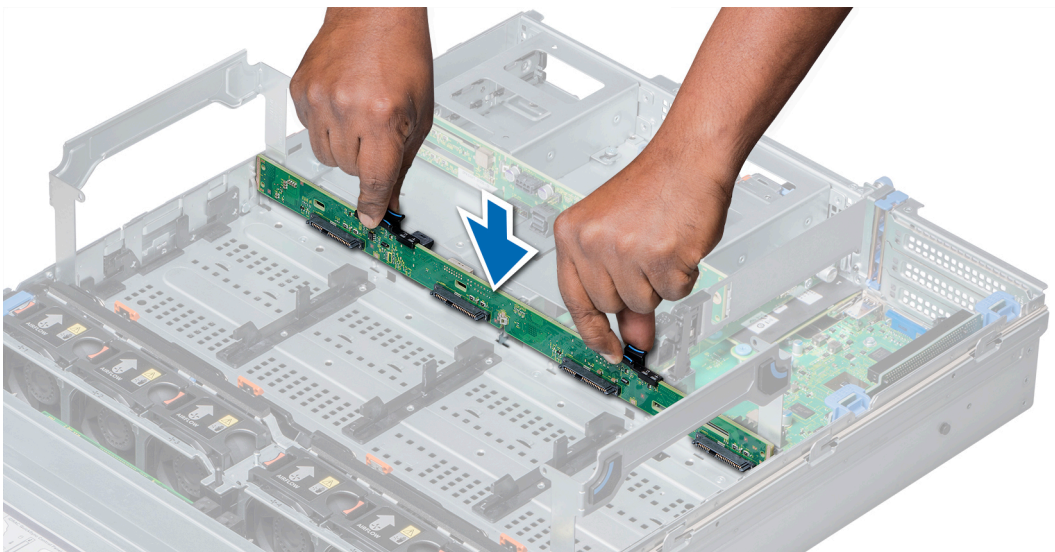
Abbildung 134. Installieren einer Rückwandplatine des mittleren Laufwerksfachs
