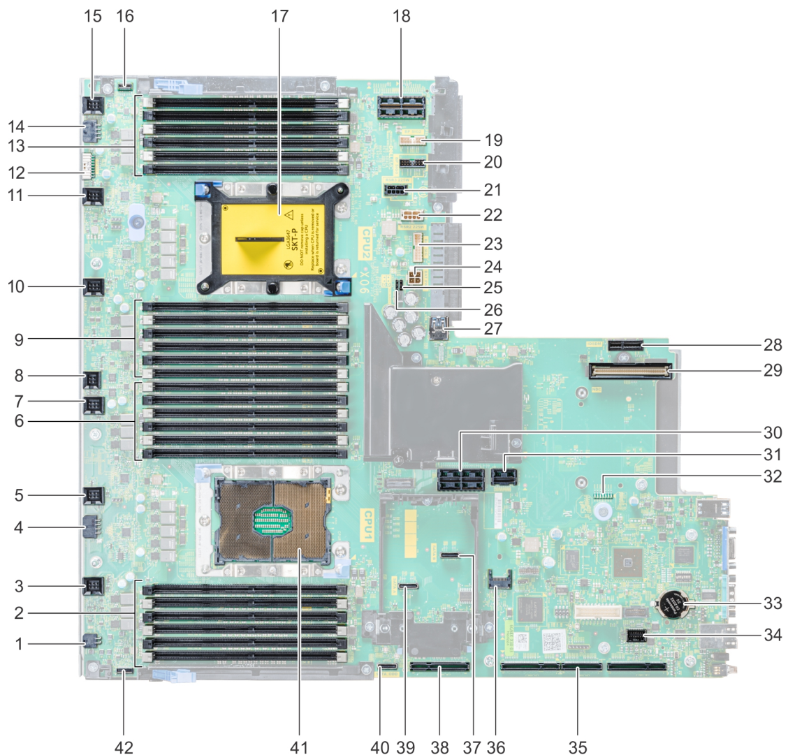
Abbildung 178. Jumper und Anschlüsse auf der Systemplatine
