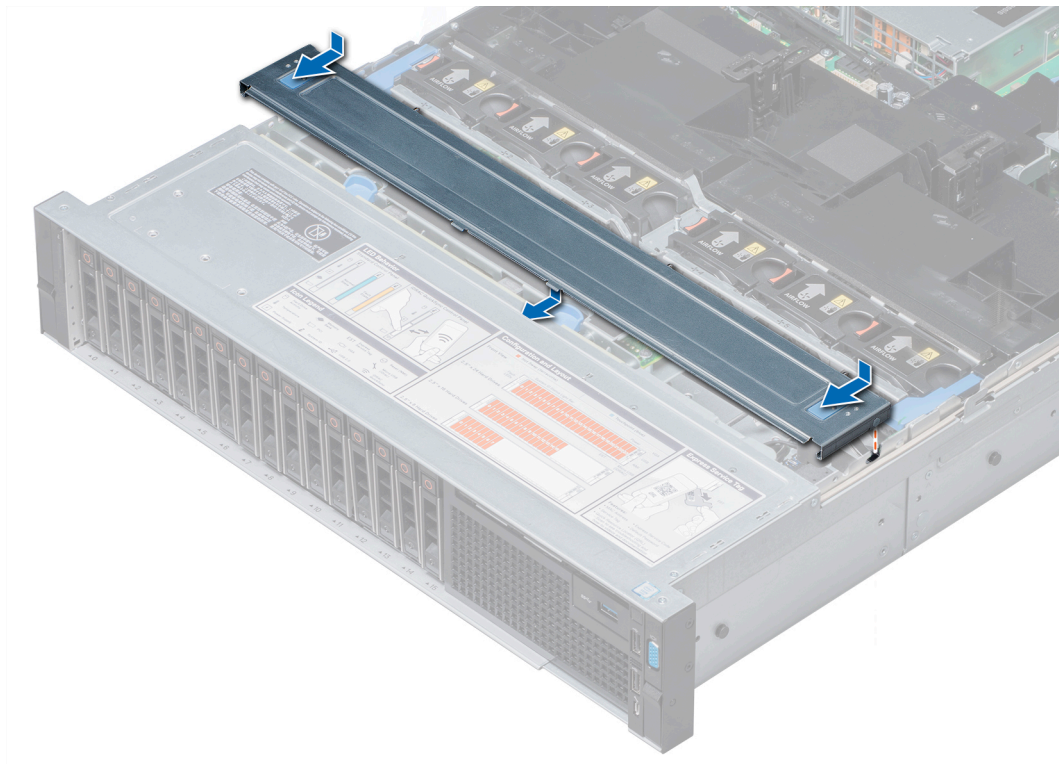
Abbildung 28. Anbringen der Rückwandplattenabdeckung
