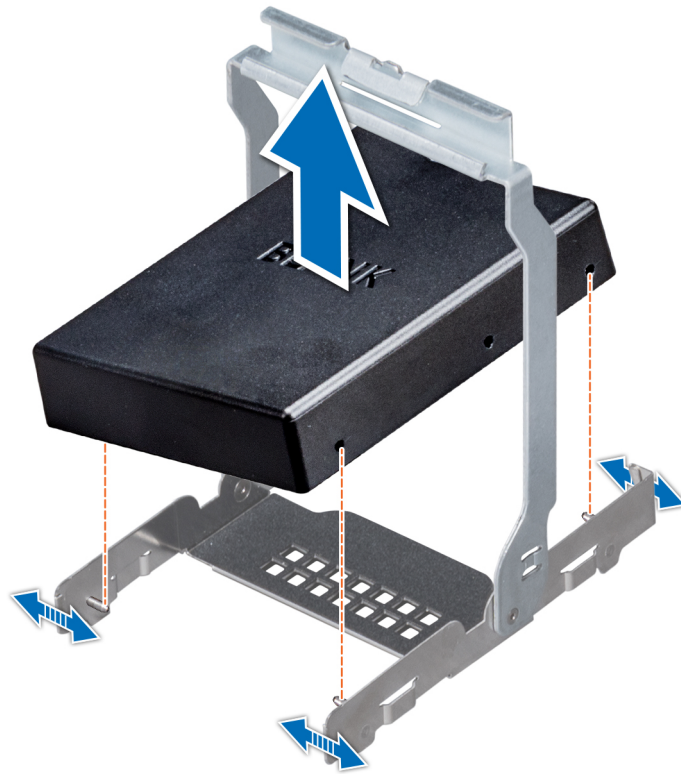
Abbildung 47. Entfernen eines Laufwerkplatzhalters aus dem mittleren Laufwerkträger
