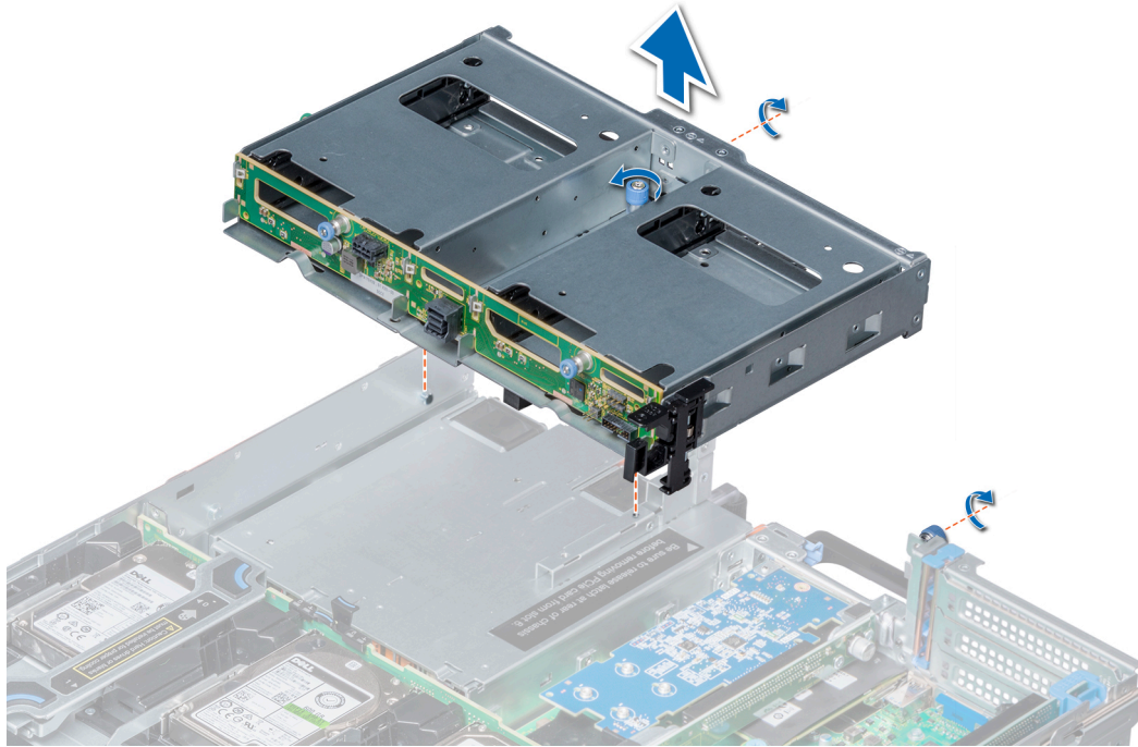
Abbildung 66. Entfernen des hinteren 2 x 3,5-Zoll-Laufwerksgehäuses
