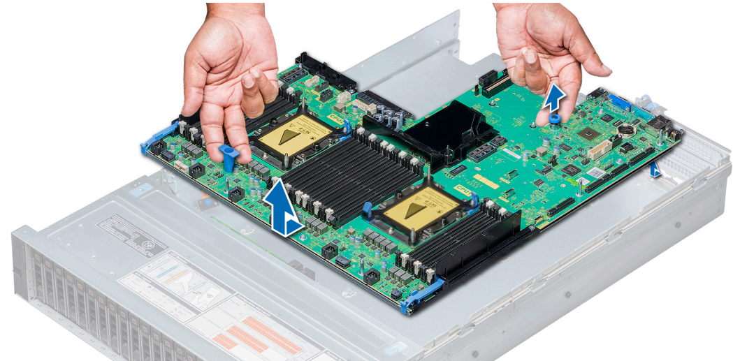
Abbildung 171. Entfernen der Systemplatine
