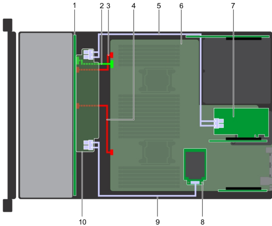
Abbildung 149. Kabelführung – 24 x 2,5-Zoll-Laufwerk-Rückwandplatine mit Mini-PERC/HBA und Adapter-PERC/HBA
