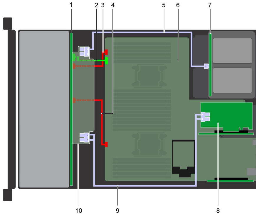
Abbildung 142. Kabelführung – 24 x 2,5-Zoll-Laufwerk-Rückwandplatine mit hinterer 4 x 2,5-Zoll-Laufwerk-Rückwandplatine mit Adapter-PERC11/HBA
