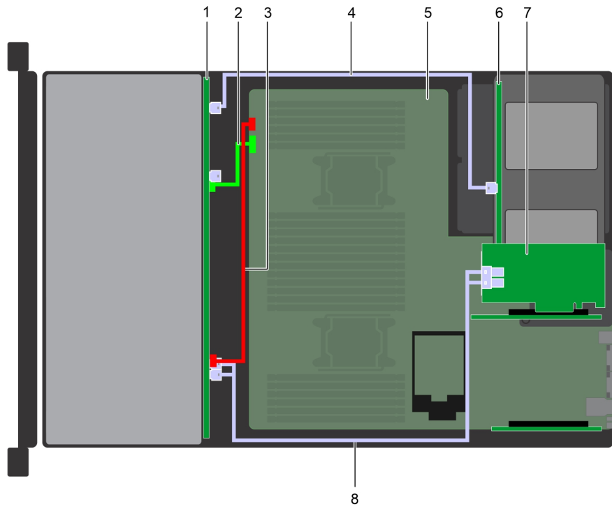
Abbildung 145. Kabelführung – 12 x 3,5-Zoll-Laufwerk-Rückwandplatine mit 4 x 2,5-Zoll-Laufwerk-Rückwandplatine hinten mit Adapter-PERC11/HBA
