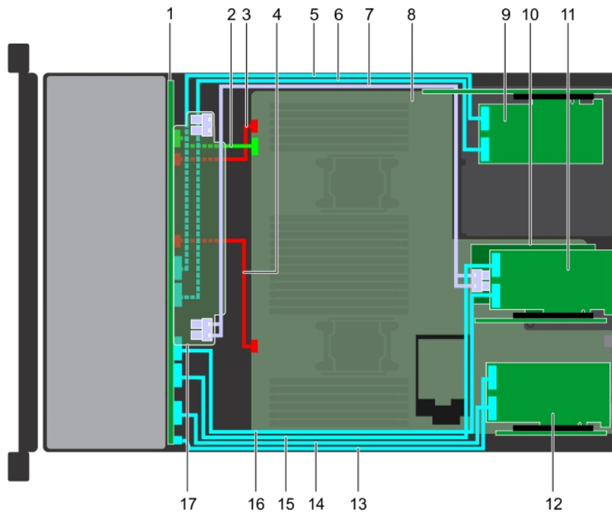
Abbildung 152. Kabelführung – 24 x 2,5-Zoll-Laufwerk-Rückwandplatine mit 12 SAS und 12 PCIe sowie Adapter-PERC
