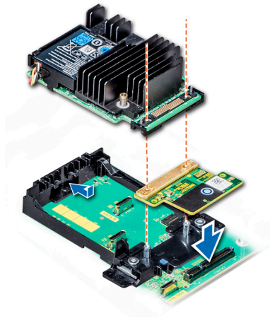
Abbildung 122. Installieren einer integrierten Speichercontrollerkarte
