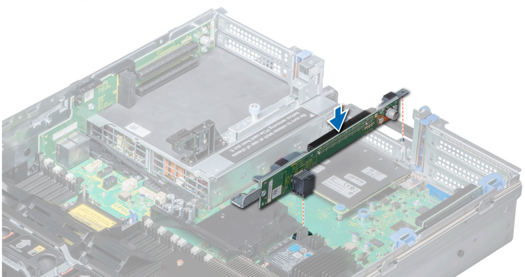
Abbildung 99. Einsetzen des Erweiterungskarten-Risers 2
