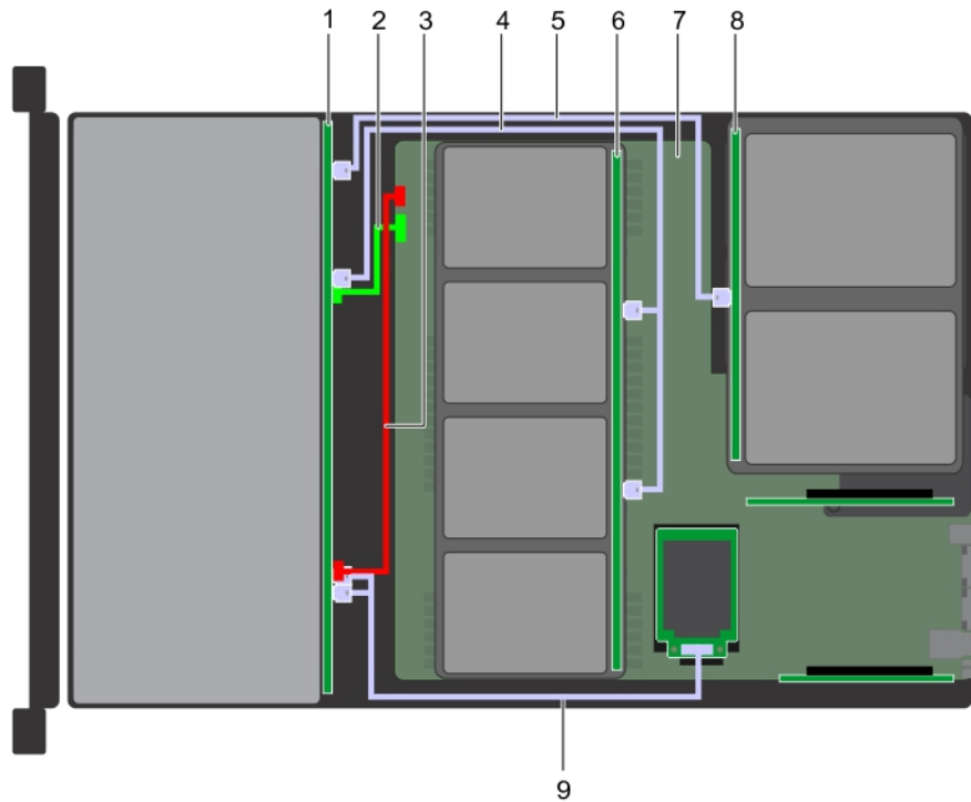
Abbildung 157. Kabelführung – 12 x 3,5-Zoll-Laufwerk-Rückwandplatine mit 4 x 3,5-Zoll-Rückwandplatine des mittleren Laufwerkfachs (mit 4 x 2,5-Zoll-Laufwerksadapter) und 2 x 3,5-Zoll-Laufwerk-Rückwandplatine (hinten)
