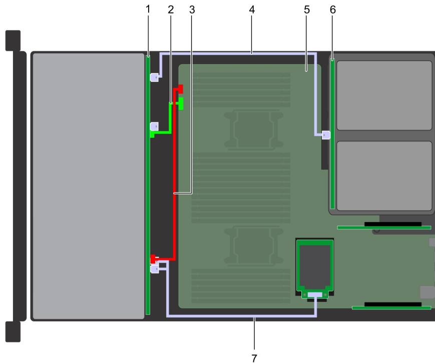
Abbildung 159. Kabelführung – 12 x 3,5-Zoll-Laufwerk-Rückwandplatine mit hinterer 2 x 3,5-Zoll-Laufwerk-Rückwandplatine
