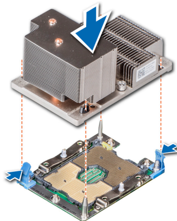
Abbildung 78. Einbauen des Prozessor- und Kühlkörpermoduls (2HE)
