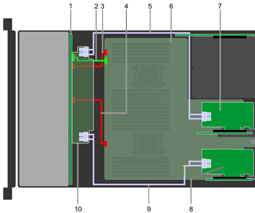
Abbildung 139. Kabelführung – 24 x 2,5-Zoll-Laufwerk-Rückwandplatine mit Dual-Adapter-PERC11/HBA
