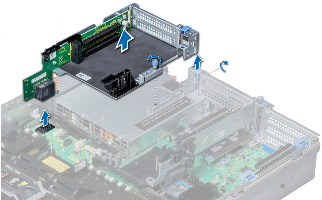
Abbildung 100. Entfernen des Erweiterungskarten-Risers 3
