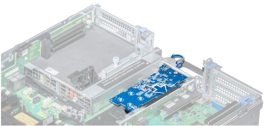
Abbildung 87. Installieren der Erweiterungskarte in Erweiterungskarten-Riser 2B
