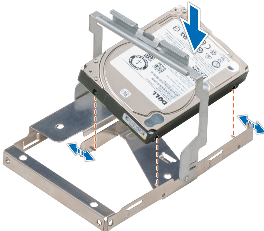
Abbildung 54. Einsetzen eines 2,5-Zoll-Laufwerks in den mittleren 3,5-Zoll-Laufwerksträger
