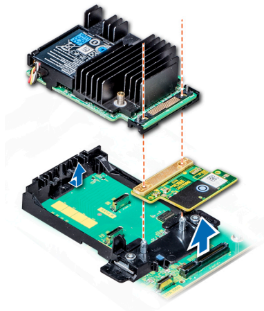
Abbildung 121. Entfernen der integrierten Speichercontrollerkarte
