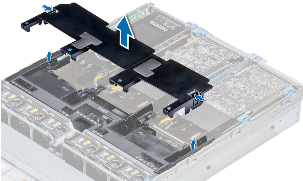
Abbildung 102. Entfernen der oberen Abdeckung des GPU-Kühlgehäuses
