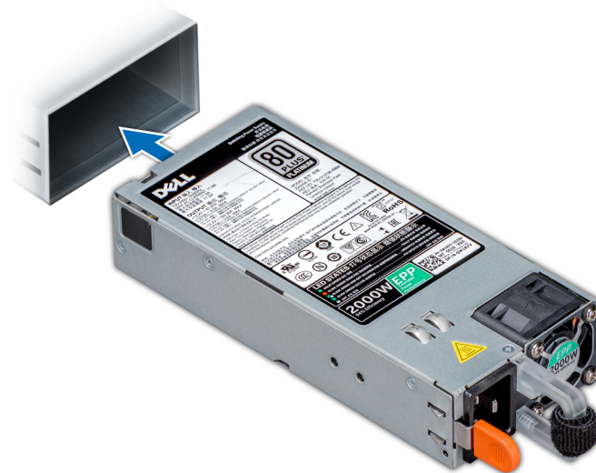
Abbildung 166. Installieren einer Netzteilereinheit
