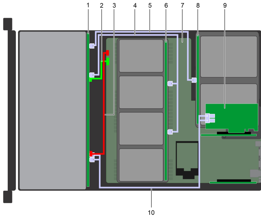
Abbildung 144. Kabelführung – 12 x 3,5-Zoll-Laufwerk-Rückwandplatine mit 4 x 3,5-Zoll-Rückwandplatine des mittleren Laufwerkfachs (mit 4 x 2,5-Zoll-Adapter) und 2 x 3,5-Zoll-Laufwerk-Rückwandplatine hinten mit Adapter-PERC11/HBA
