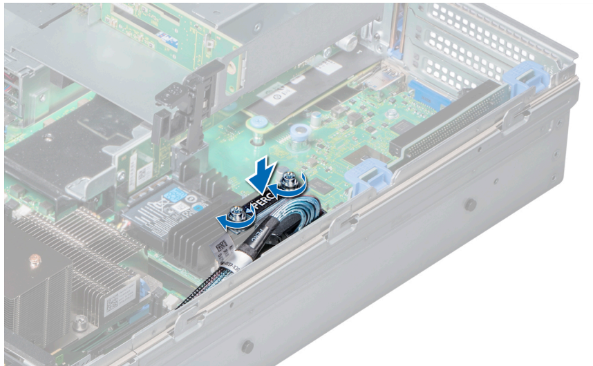
Abbildung 123. Anbringen eines integrierten Speicher-Controller-Kartenkabels
