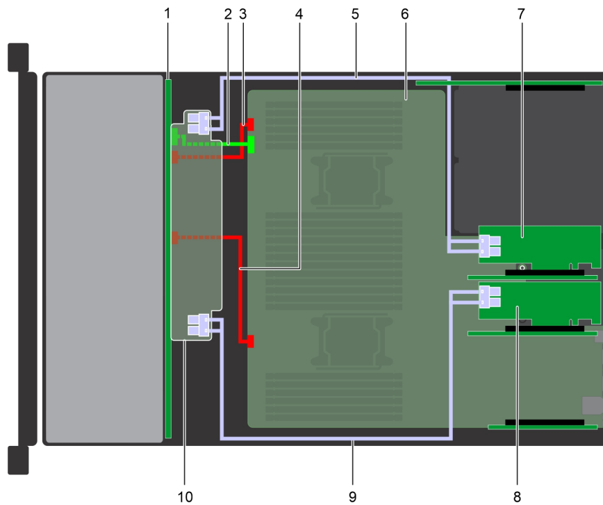
Abbildung 140. Kabelführung – 24 x 2,5-Zoll-Laufwerk-Rückwandplatine mit Dual-Adapter-PERC11/HBA
