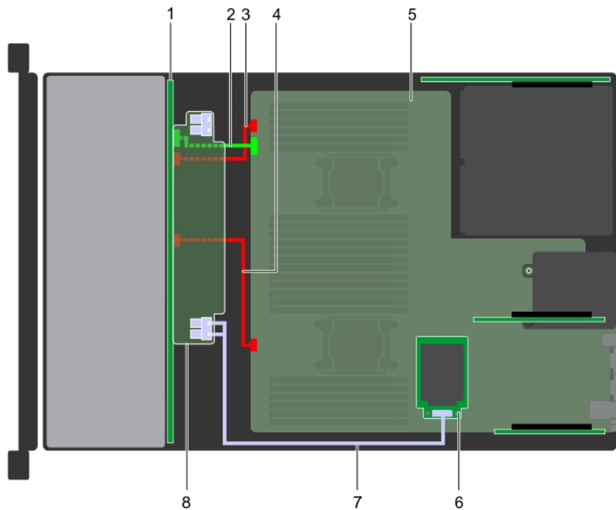
Abbildung 147. Kabelführung – 24-x-2,5-Zoll-Laufwerkrückwandplatine mit Mini-PERC
