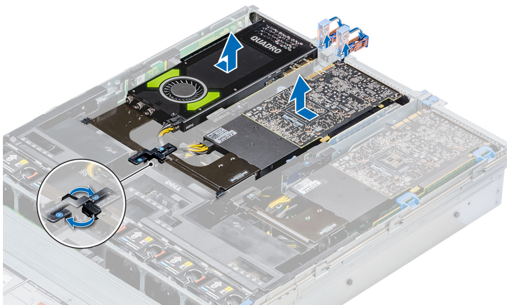
Abbildung 104. Entfernen der GPU 2 und 3
