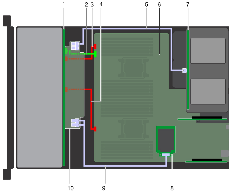
Abbildung 151. Kabelführung – 24 x 2,5-Zoll-Laufwerk-Rückwandplatine mit hinterer 4 x 2,5-Zoll-Laufwerk-Rückwandplatine
