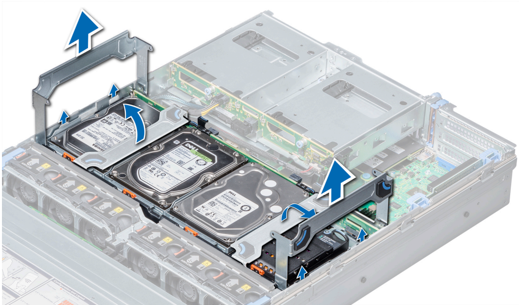
Abbildung 45. Entfernen des mittleren Laufwerkfachs
