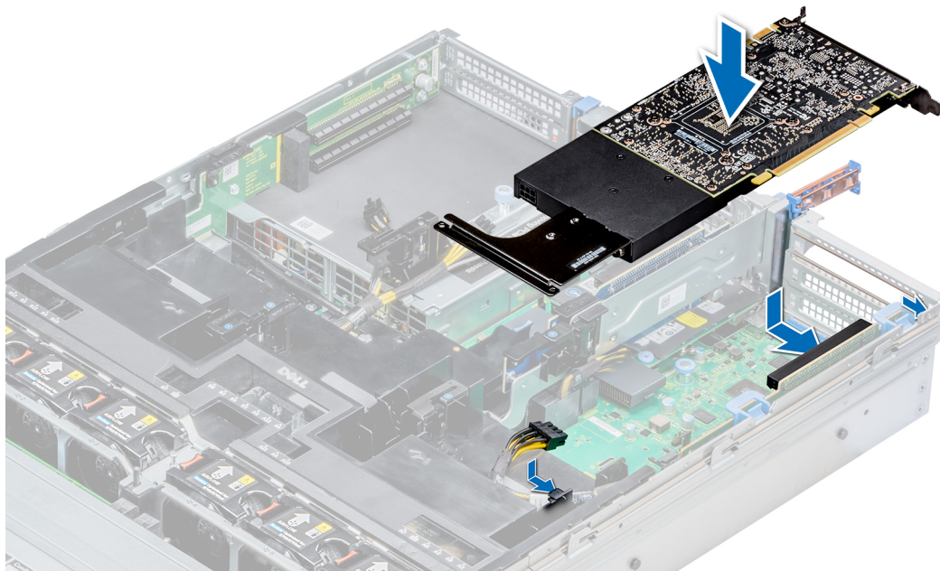
Abbildung 108. GPU 1 einsetzen
