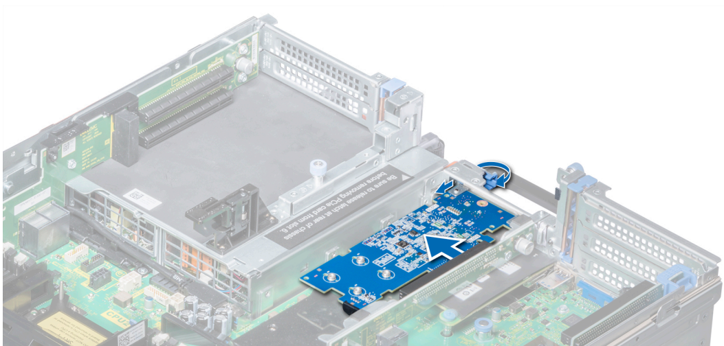
Abbildung 83. Entfernen der Erweiterungskarte aus Erweiterungskarten-Riser 2B
