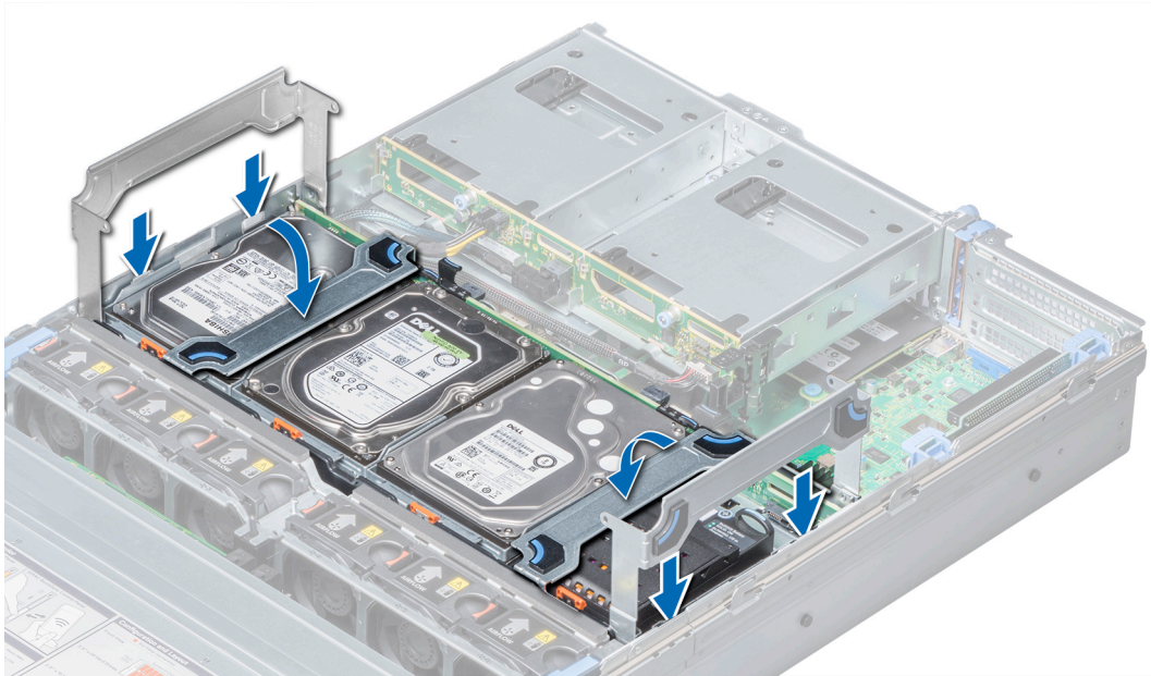
Abbildung 46. Einsetzen des mittleren Laufwerksfachs
