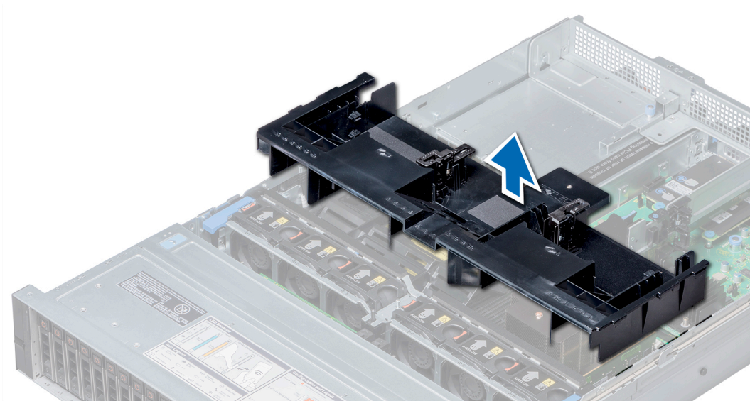
Abbildung 31. Entfernen des Kühlgehäuses
