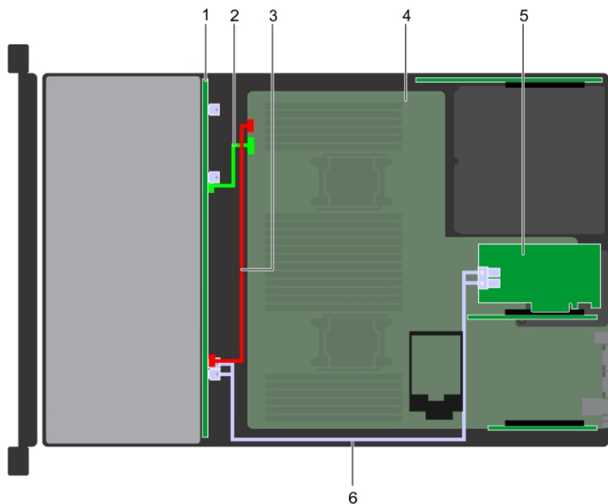
Abbildung 156. 12 x 3,5-Zoll-Laufwerk-Rückwandplatine mit Adapter-PERC
