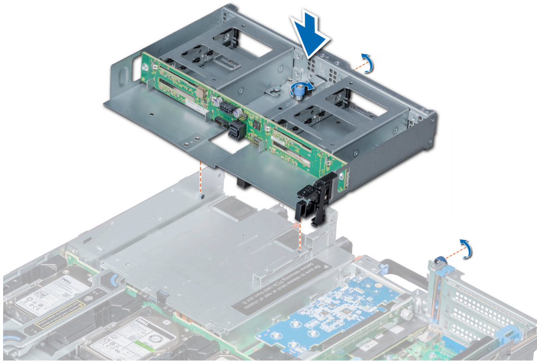
Abbildung 67. Einsetzen des hinteren 4 x 2,5-Zoll-Laufwerksgehäuses
