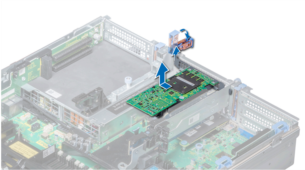
Abbildung 84. Entfernen der Erweiterungskarte aus Erweiterungskarten-Riser 2
