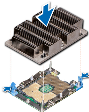
Abbildung 79. Prozessor-Kühlkörper-Modul (1 HE) einbauen
