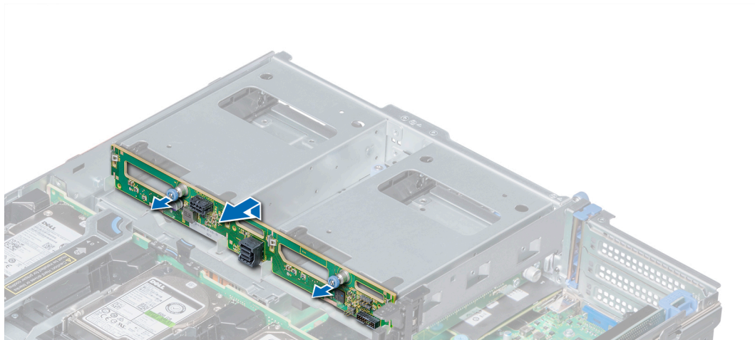
Abbildung 135. Entfernen der rückseitigen 3,5-Zoll-Laufwerkrückwandplatine
