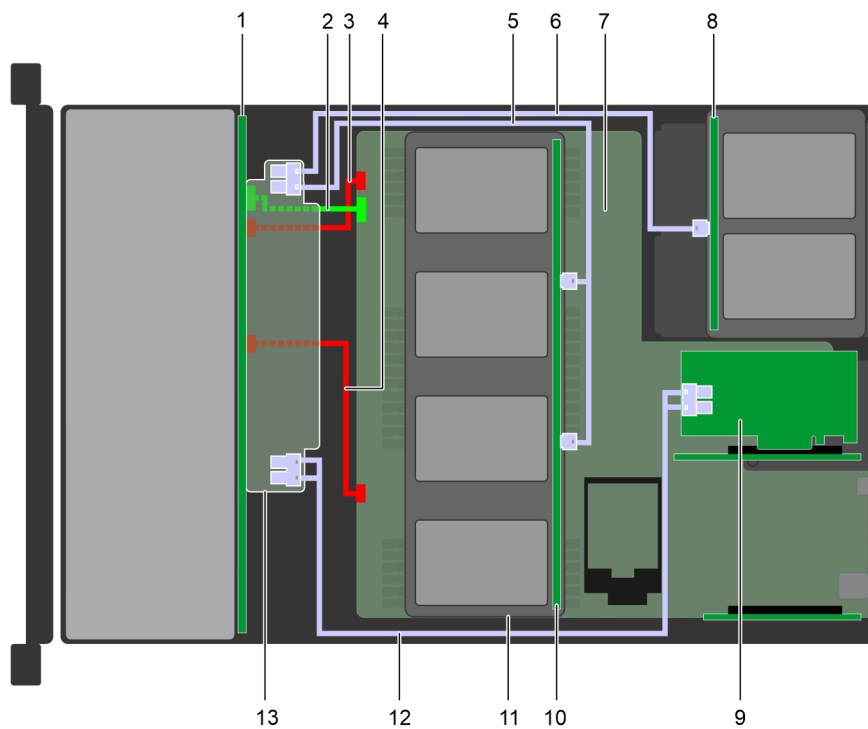
Abbildung 141. Kabelführung – 24 x 2,5-Zoll-Laufwerk-Rückwandplatine mit 4 x 2,5-Zoll-Adapter-Rückwandplatine des mittleren Laufwerkfachs und hintere 4 x 2,5-Zoll-Laufwerk-Rückwandplatine mit Adapter-PERC11/HBA
