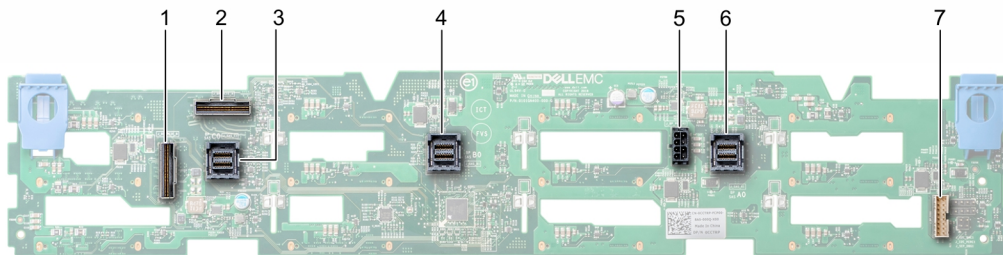
Abbildung 130. Rückansicht der Hybrid-Rückwandplatine mit 3,5-Zoll-Hot-Plug-Laufwerk (SATA und SAS) mit U.2-NVMe-SSD
