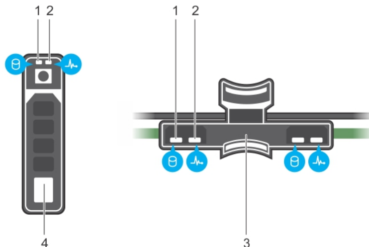
Abbildung 13. Laufwerkanzeigen auf dem Laufwerk und der Rückwandplatine des mittleren Laufwerkfachs
