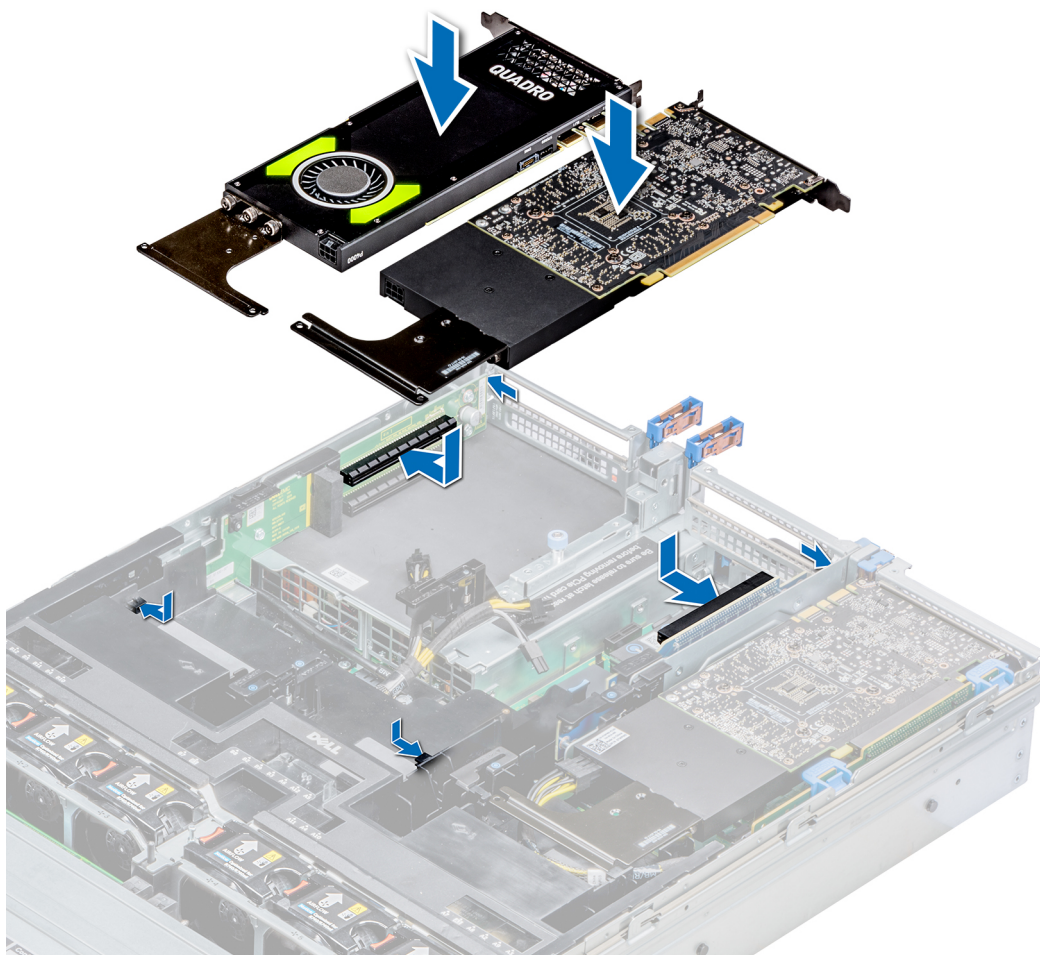
Abbildung 110. GPU 2 und 3 einsetzen
