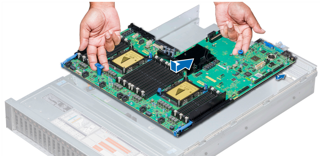
Abbildung 172. Installieren der Systemplatine
