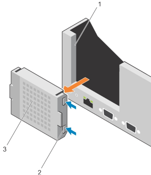
Figure 58. Retrait du cache de la carte de montage 1
