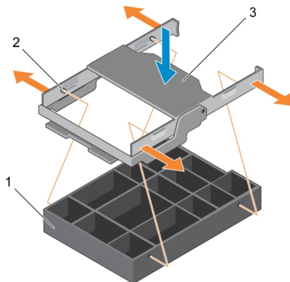
Figure 26. Installation d'un cache de disque dur dans un support de disque dur
