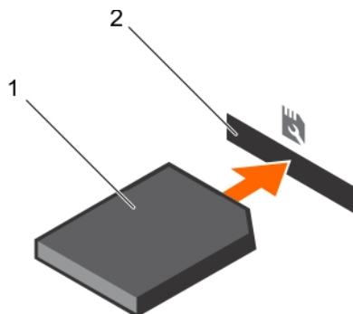
Figure 121. Installation de la carte mémoire SD vFlash
