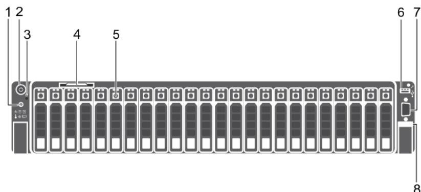
Figure 2. 24 x châssis SSD/disque dur de 2,5 pouces
