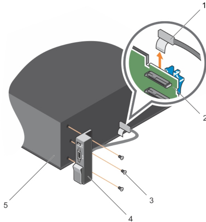
Figure 126. Retrait du panneau des entrées/sorties
