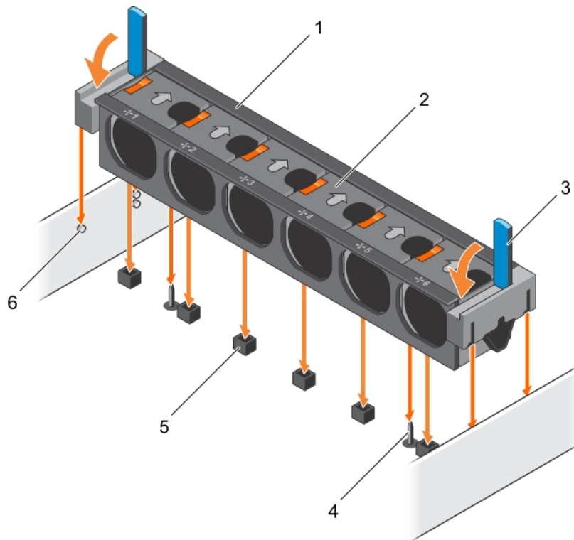
Figure 34. Installation de l'assemblage du ventilateur
