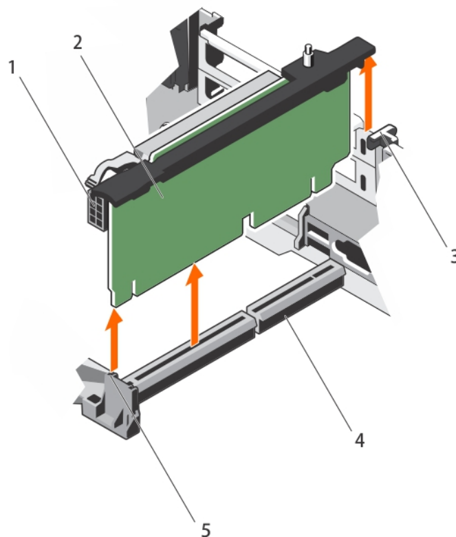
Figure 62. Retrait de la carte de montage pour carte d'extension 2
