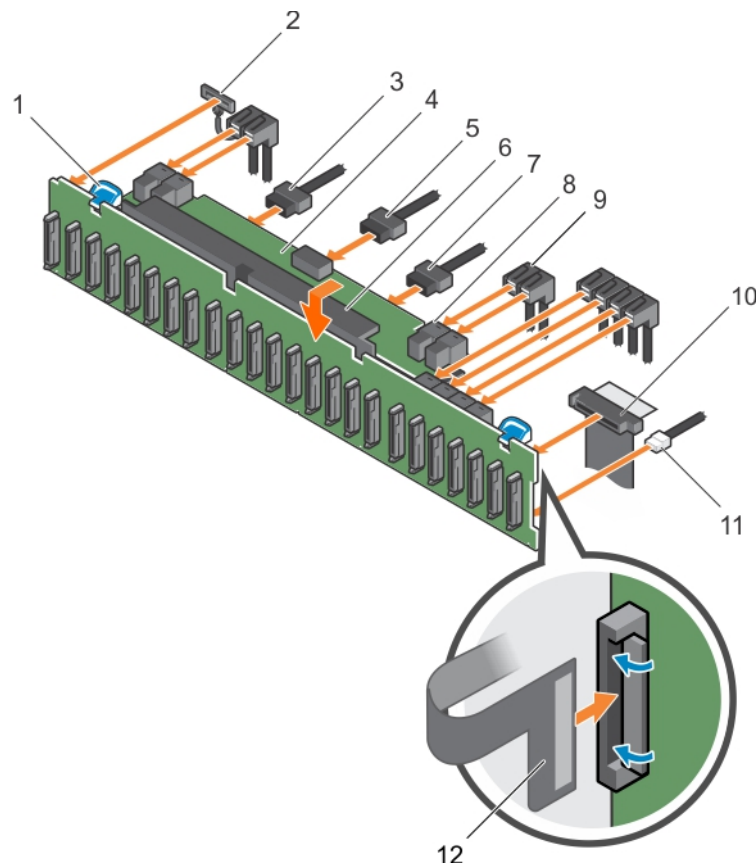
Figure 116. Installation du fond de panier SAS/SATA (x24) de 2,5 pouces
