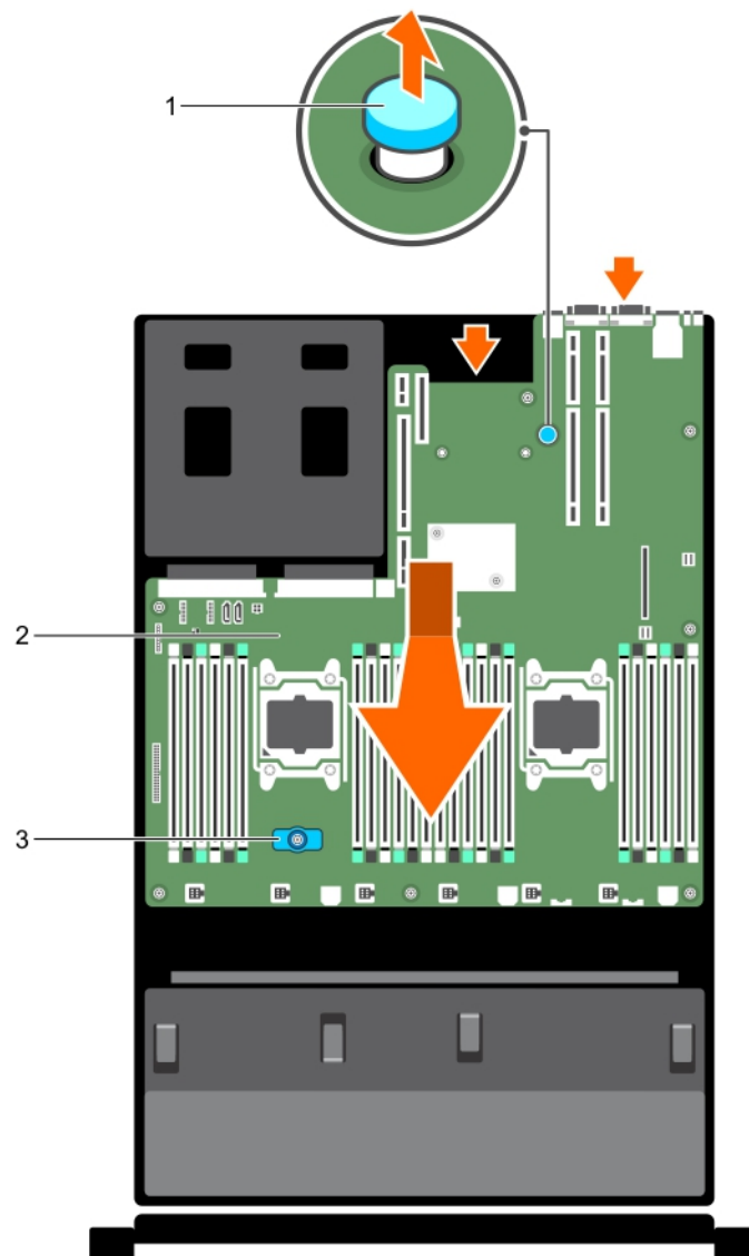
Figure 88. Retrait de la carte système
