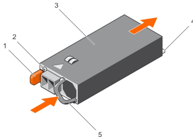
Figure 87. Installation d'un bloc d'alimentation en CC
