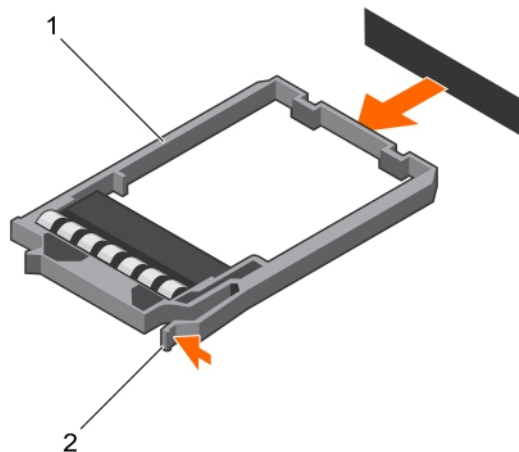
Figure 103. Retrait d'un cache de disque dur de 1,8 pouce
