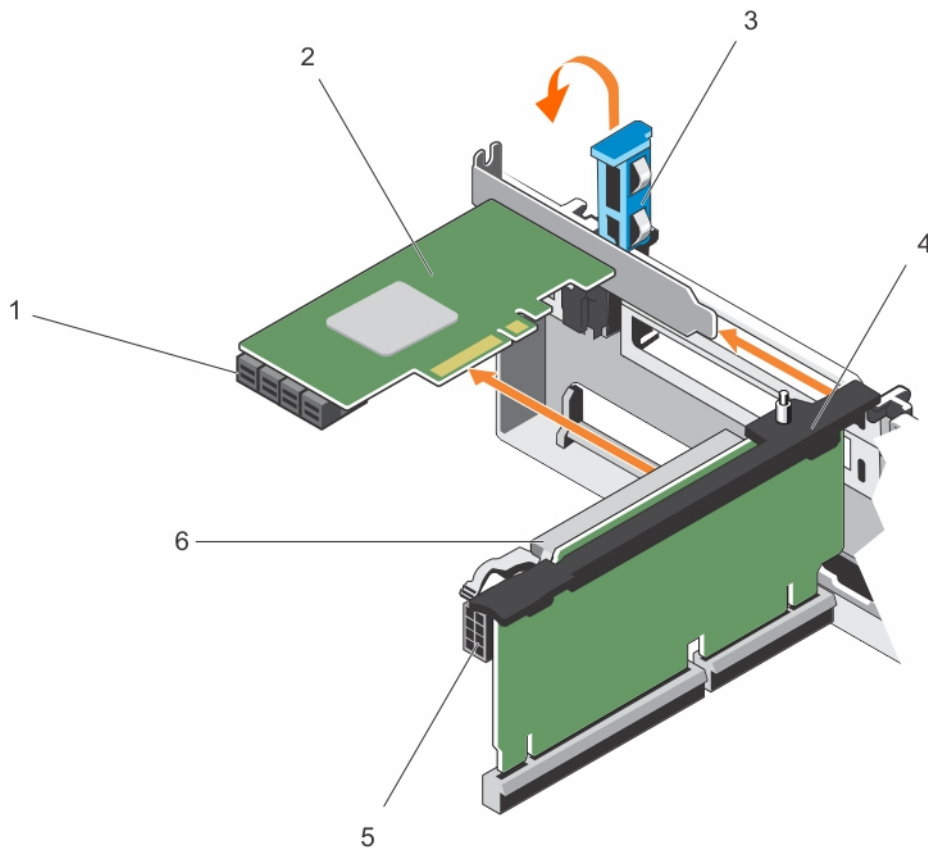
Figure 56. Retrait d'une carte d'extension NVMe de la carte de montage pour carte d'extension
