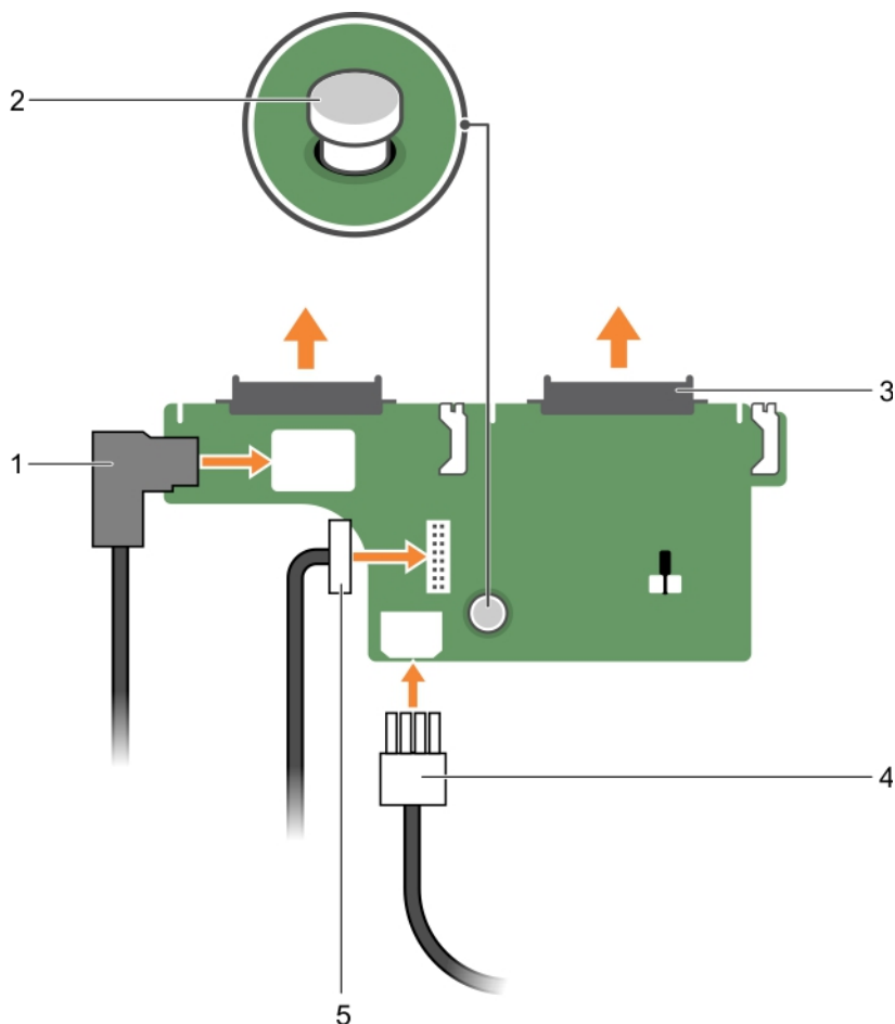
Figure 119. Installation du fond de panier de disque dur (x2) de 2,5 pouces facultatif
