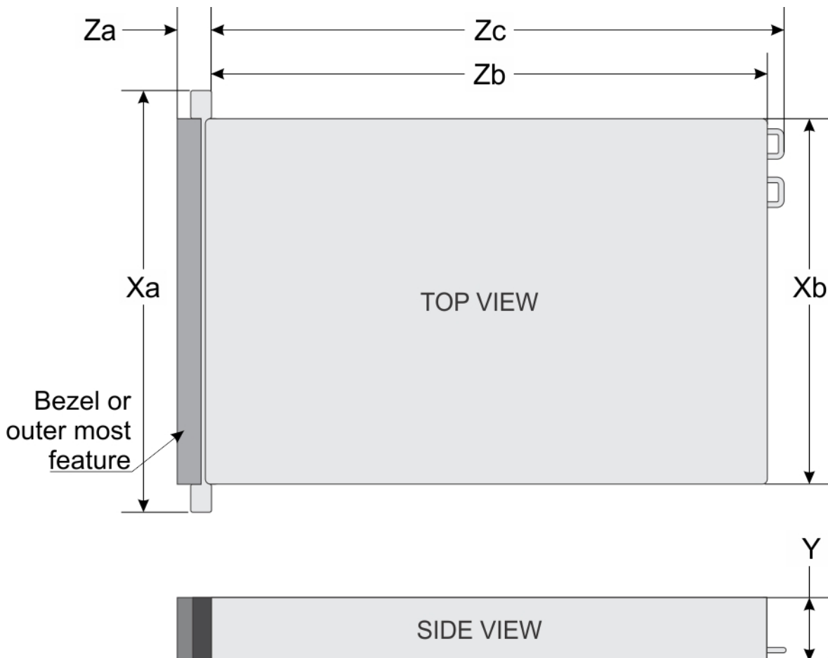
Figure 13. Dimensions du châssis du système PowerEdge R730xd
