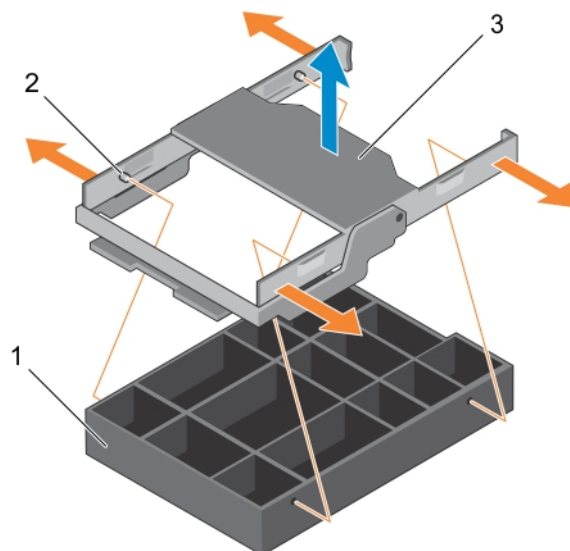
Figure 25. Retrait du cache de disque dur d'un support de disque dur
