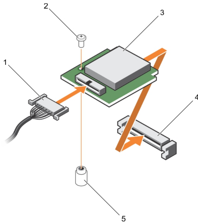
Figure 123. Installation de l'unité de support vFlash
