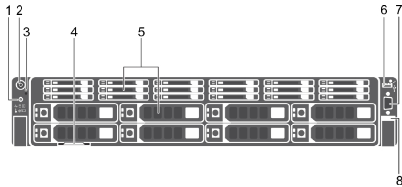
Figure 4. Châssis 8 x disques durs de 3,5 pouces et 18 x SSD de 1,8 pouce
