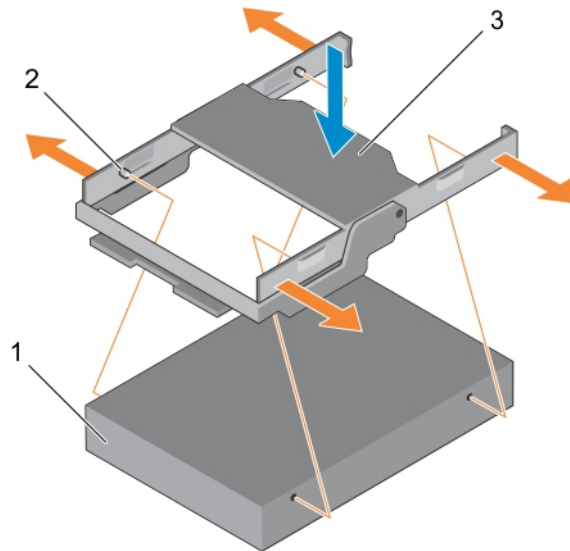
Figure 30. Installation d'un disque dur dans un support de disque dur
