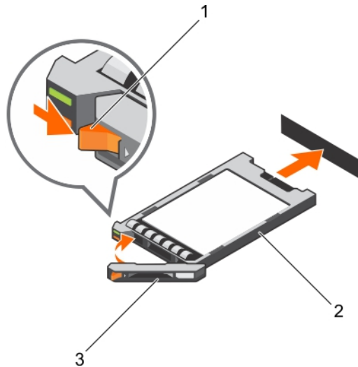
Figure 100. Installation d'un support de SSD uSATA de 1,8 pouce remplaçable à chaud
