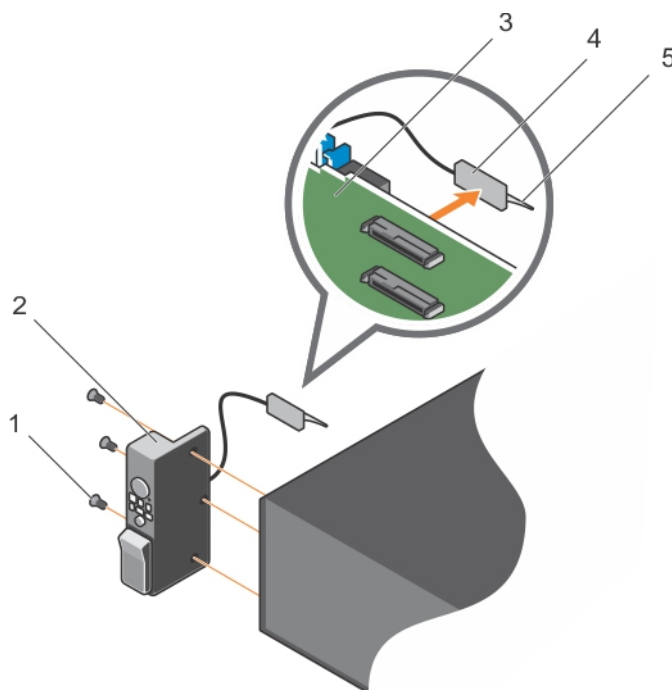
Figure 124. Retrait du panneau de commande
