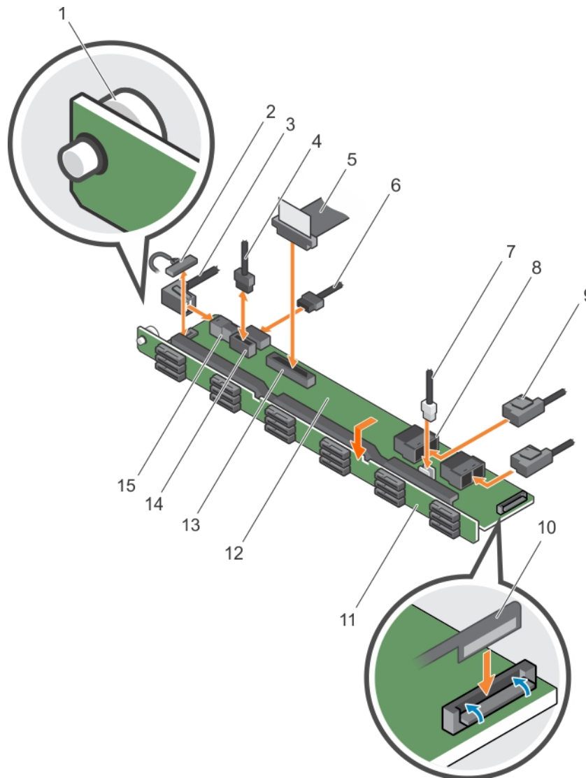
Figure 117. Installation du fond de panier SAS/SATA (x18) de 1,8 pouce
