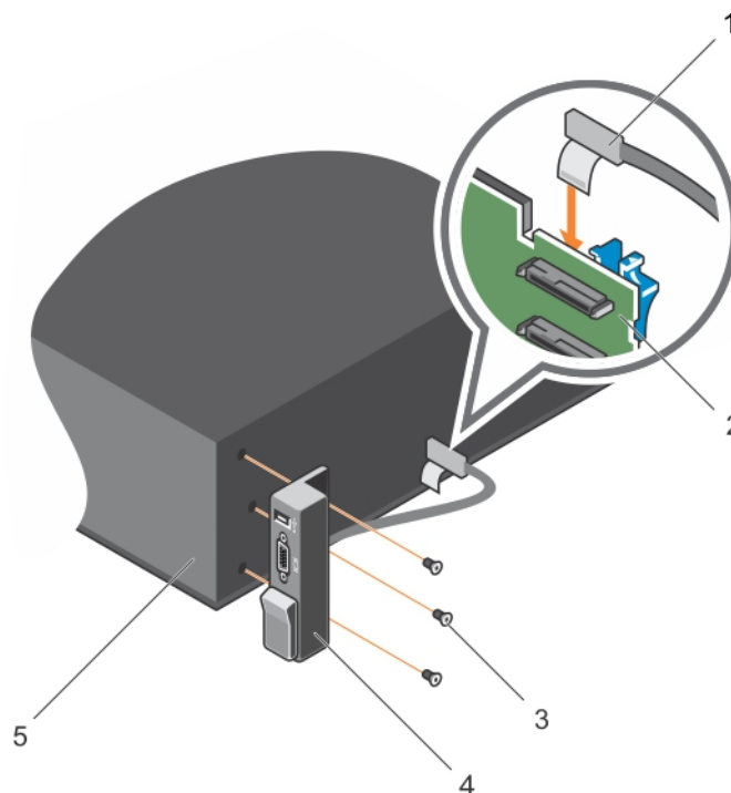
Figure 127. Installation du panneau des entrées/sorties
