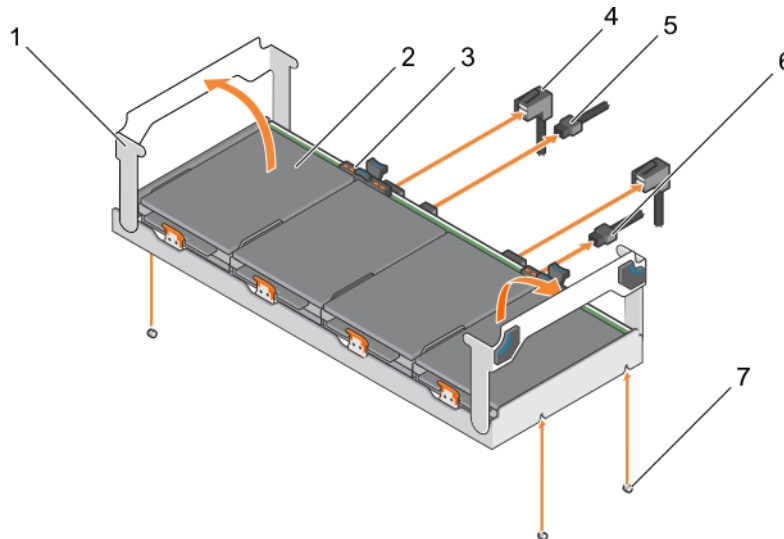
Figure 23. Retrait du plateau de disque dur
