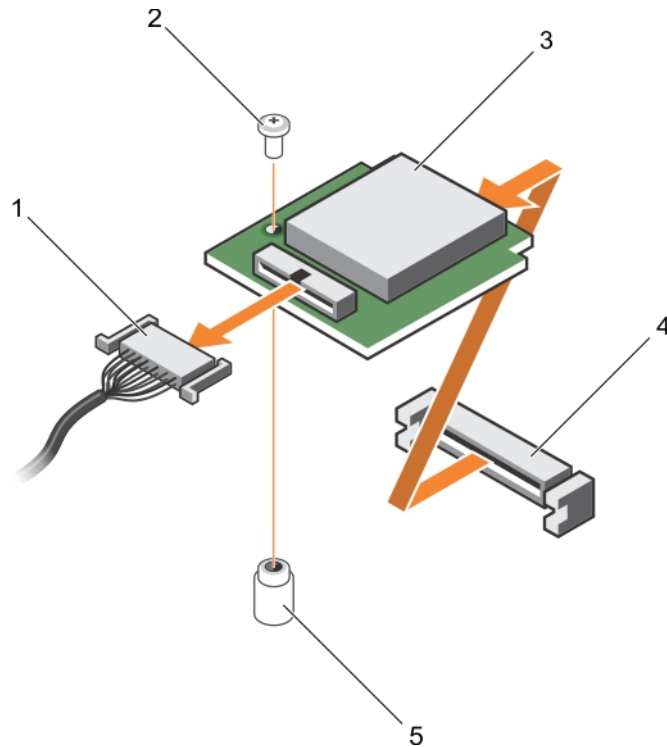
Figure 122. Retrait de l'unité de support vFlash
