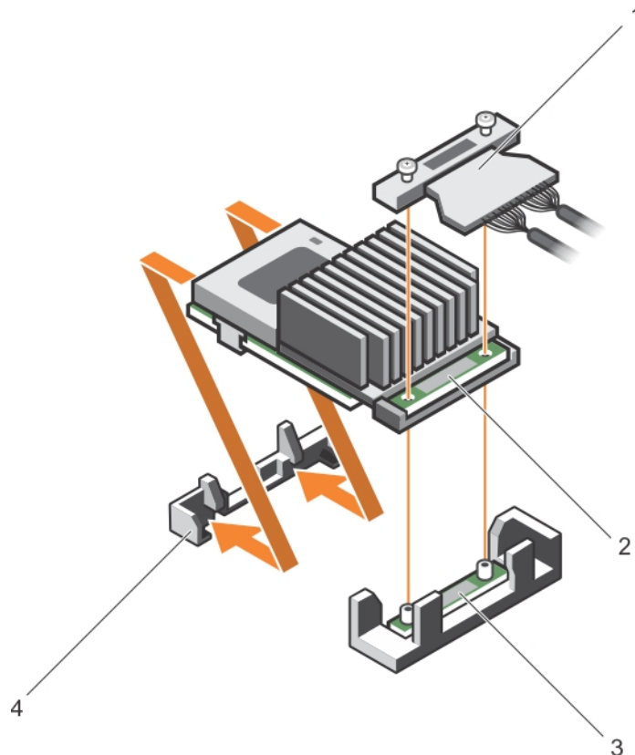
Figure 51. Installation de la carte contrôleur de stockage intégrée
