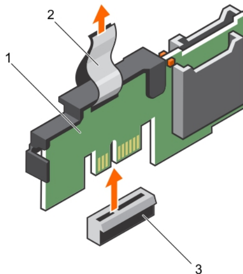
Figure 71. Retrait du module SD interne double (IDSDM)
