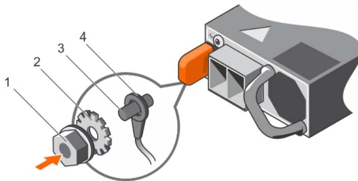
Figure 82. Assemblage et connexion du câble de mise à la terre
