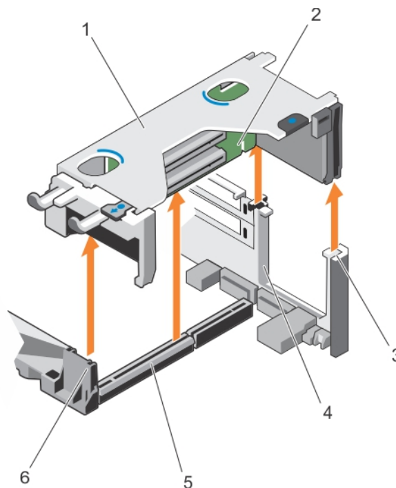
Figure 60. Retrait de la carte de montage pour carte d'extension 1
