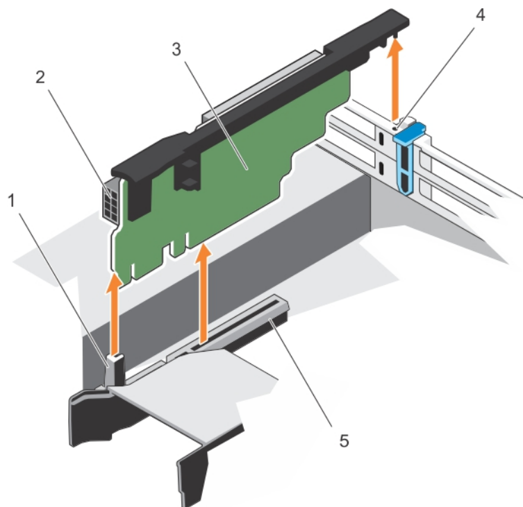
Figure 64. Retrait de la carte de montage pour carte d'extension 3
