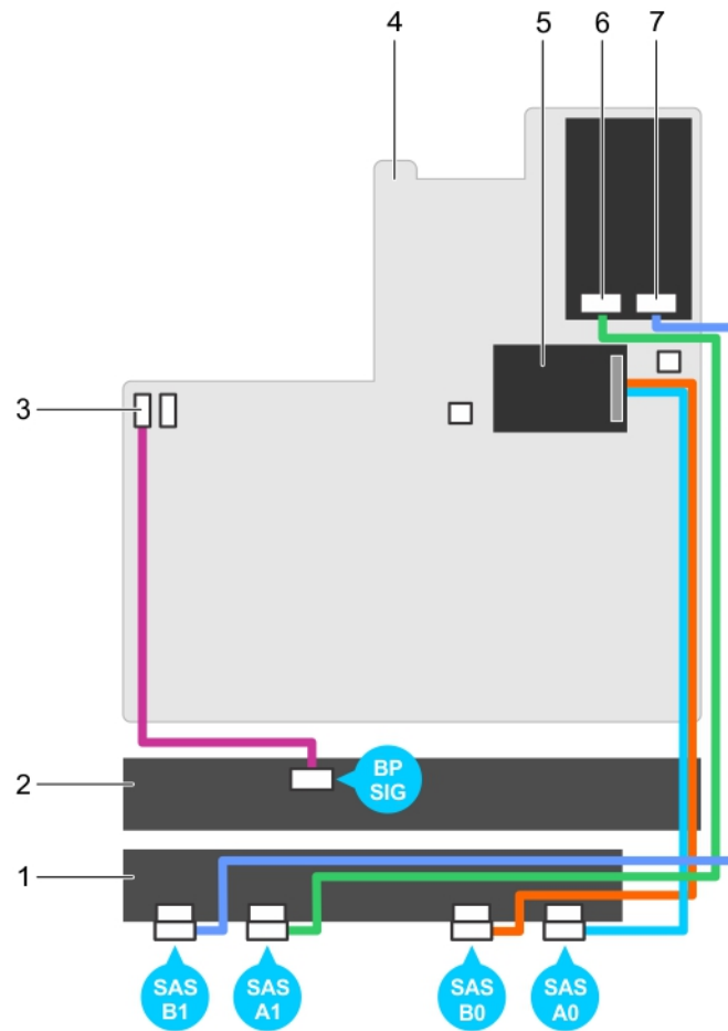
Figure 109. Schéma de câblage : fond de panier SAS/SATA (x24) de 2,5 pouces (option 2)
