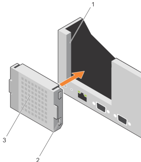
Figure 59. Installation du cache de la carte de montage 1
