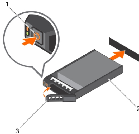
Figure 99. Installation d'un disque dur ou SSD remplaçable à chaud
