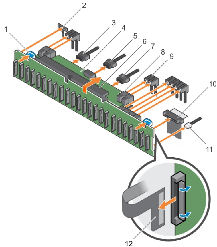
Figure 107. Retrait du fond de panier SAS/SATA (x24) de 2,5 pouces
