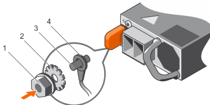
図 75. 安全用接地線の組み立てと接続
