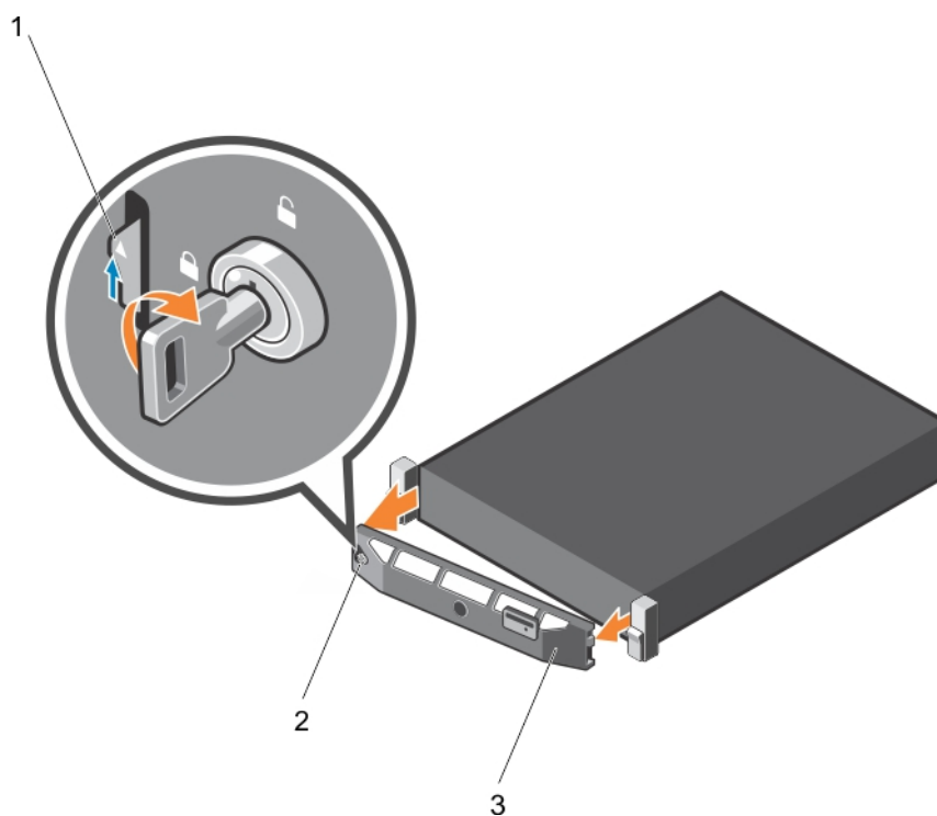
图 15: 卸下可选的快速同步前挡板
