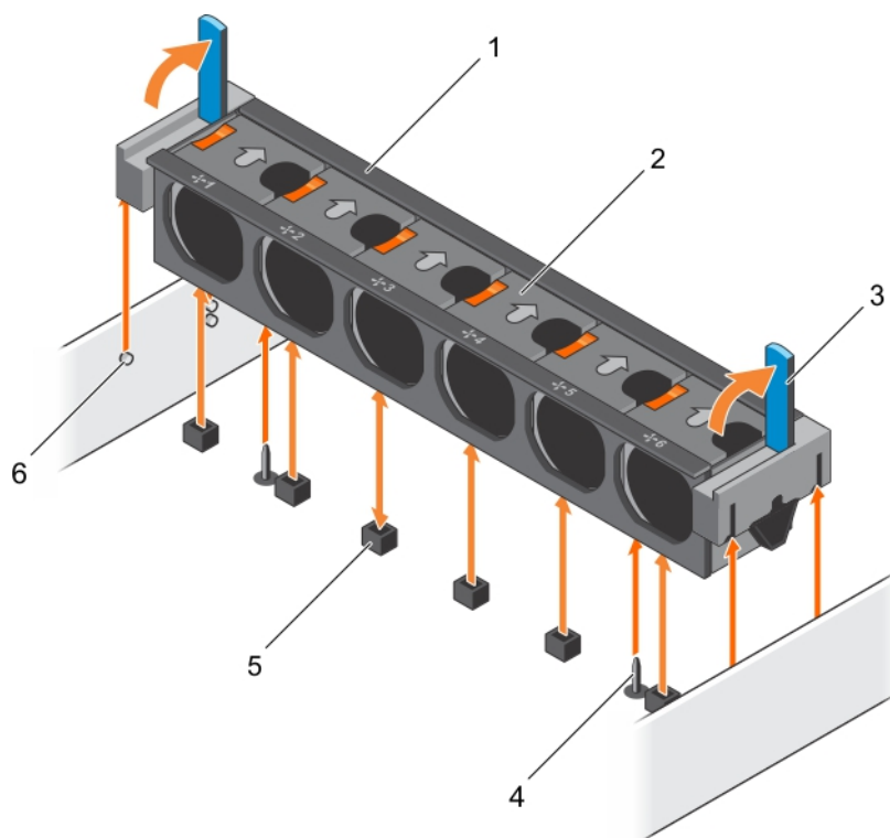
図 24. 冷却ファンアセンブリーの取り外し
