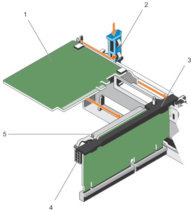
図 46. 拡張カードライザー 2 または 3 への拡張カードの取り付け
