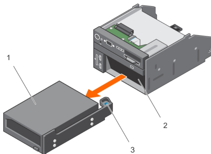
図 109. テープバックアップユニットの取り外しと取り付け
