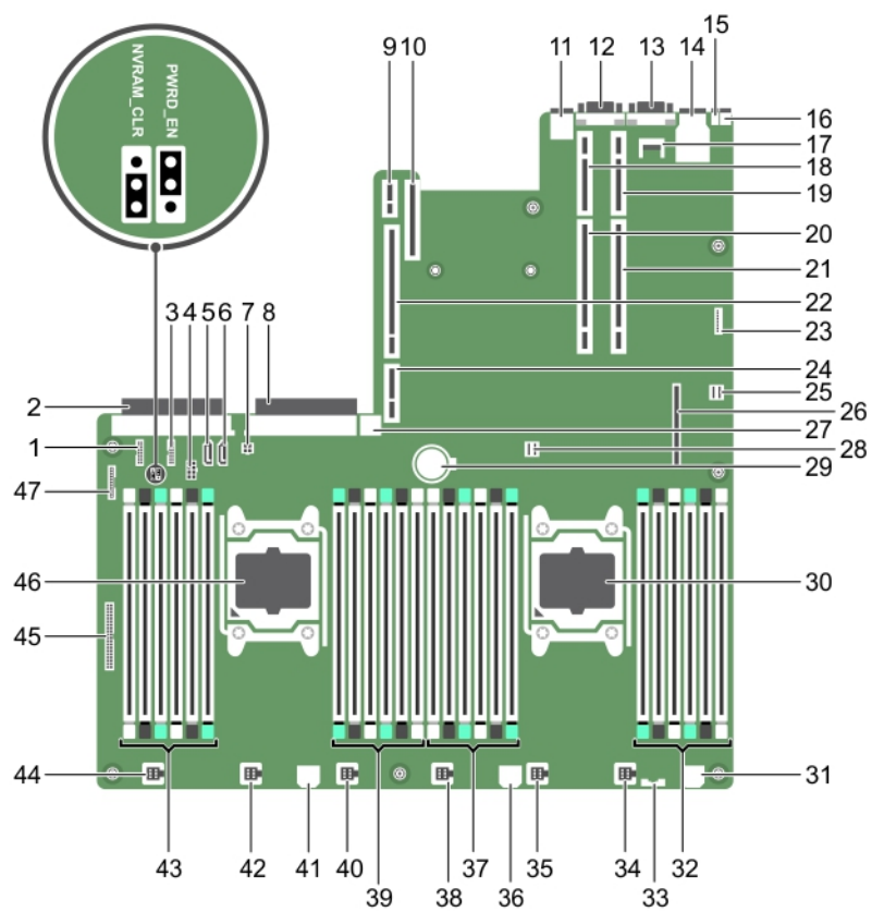
図 121. システム基板のジャンパとコネクタ
