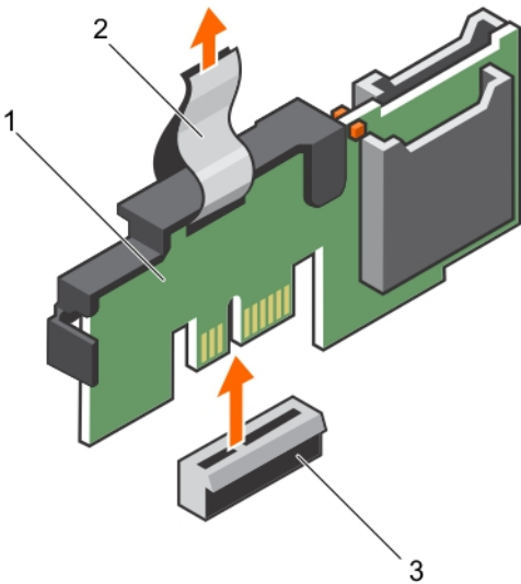
図 64. 内蔵デュアル SD モジュール ( IDSDM ) の取り外し
