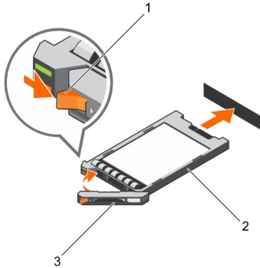
図 91. 1.8 インチホットスワップ対応 uSATA SSD キャリアの取り付け
