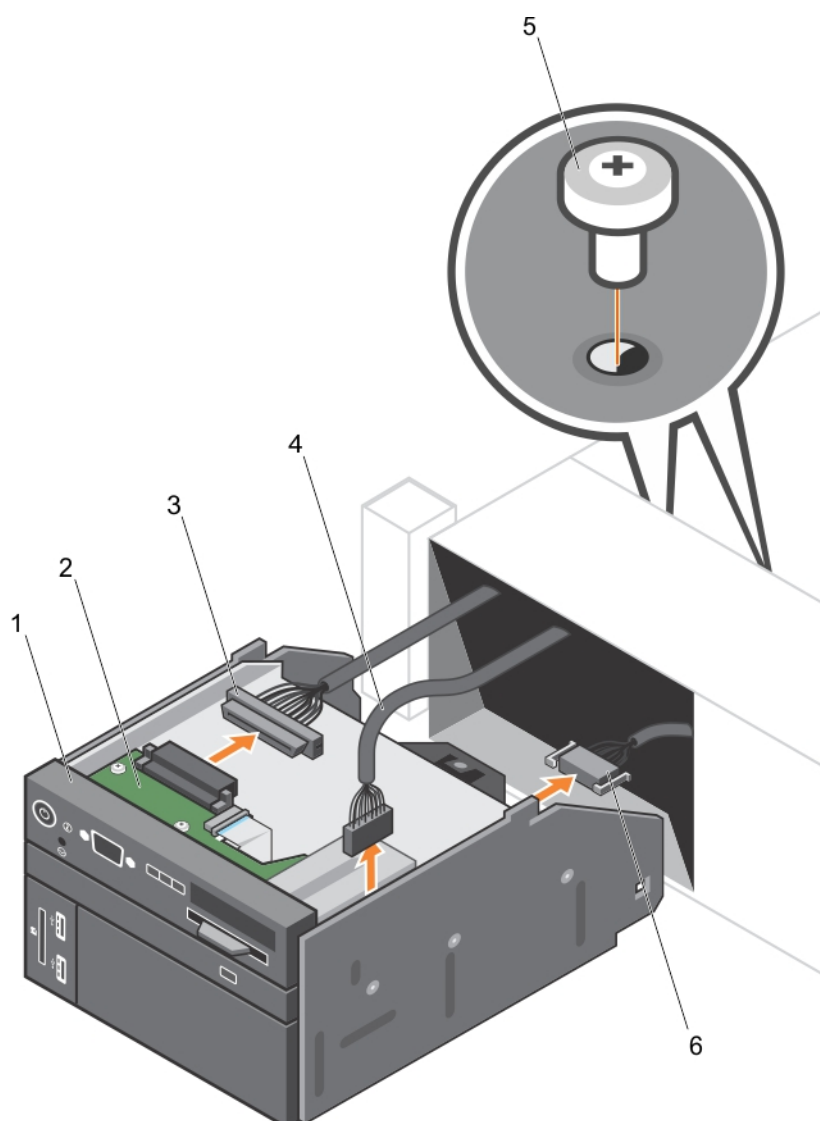
図 116. コントロールパネルの取り外し - 2.5 インチ ハード ドライブ システム
