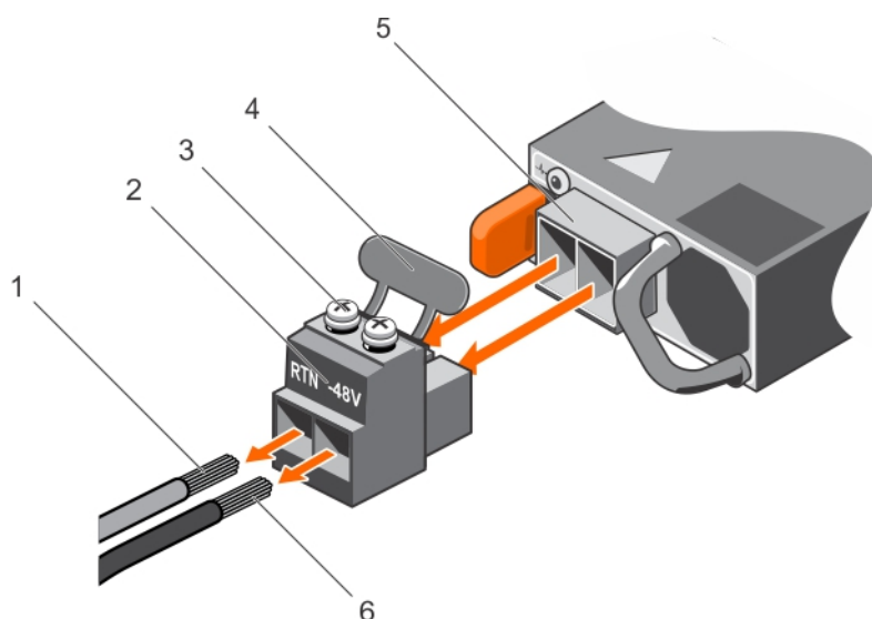
図 78. DC 入力電源ワイヤの取り外し
