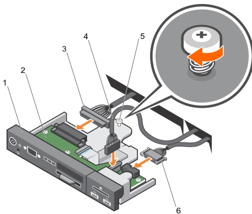
図 118. コントロールパネルの取り付け - 3.5 インチ ハード ドライブ システム
