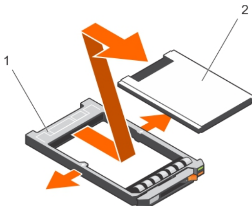
図 96. ハードドライブキャリアからの 1.8 インチハードドライブの取り外し
