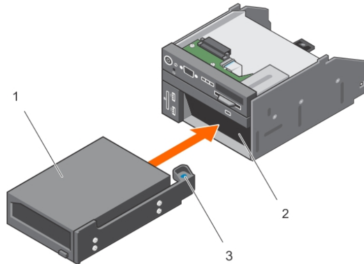
図 110. テープバックアップユニットの取り付け
