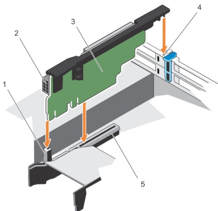
図 59. 拡張カードライザー 3 の取り付け
