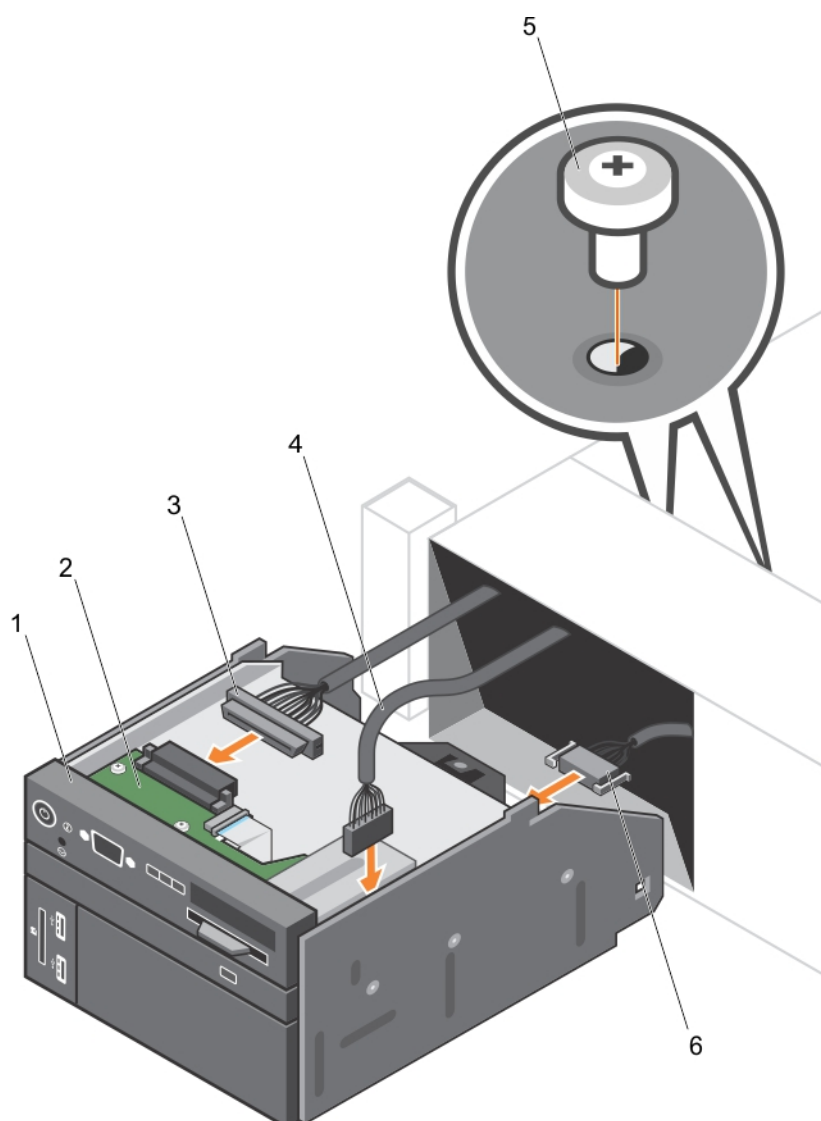
図 119. コントロールパネルの取り付け - 2.5 インチ ハード ドライブ システム
