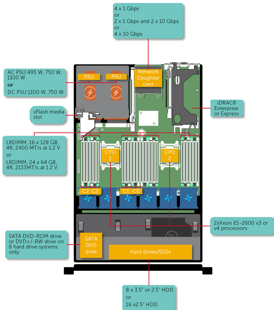
図 1. PowerEdge R730 システムでサポートされている構成
