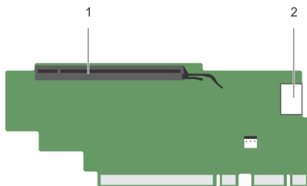
図 56. 拡張カード ライザー 3 のコネクタの識別
