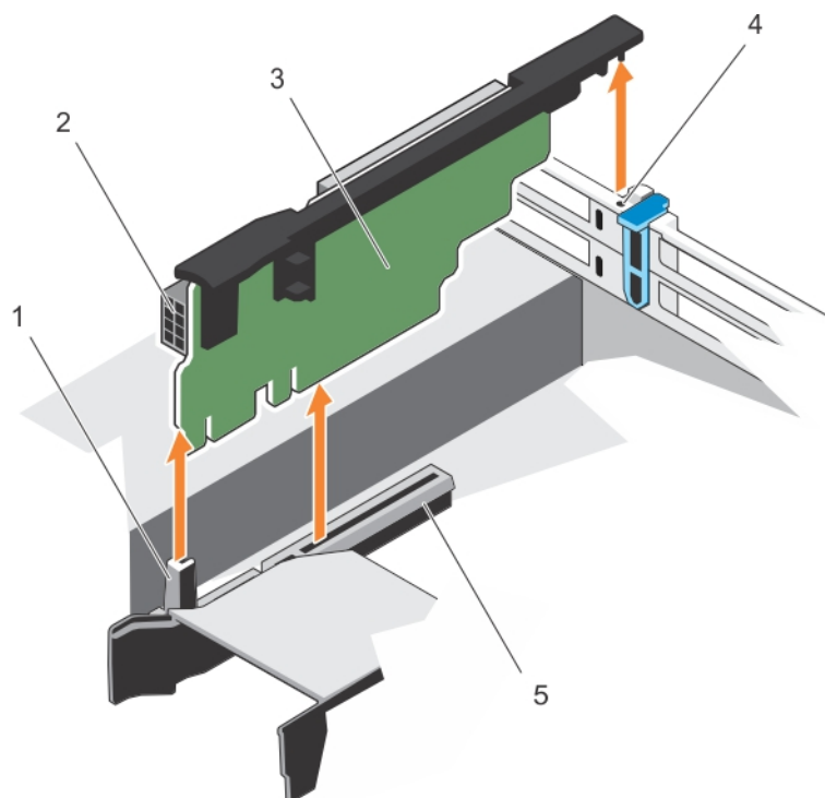
図 55. 拡張カードライザー 3 の取り外し
