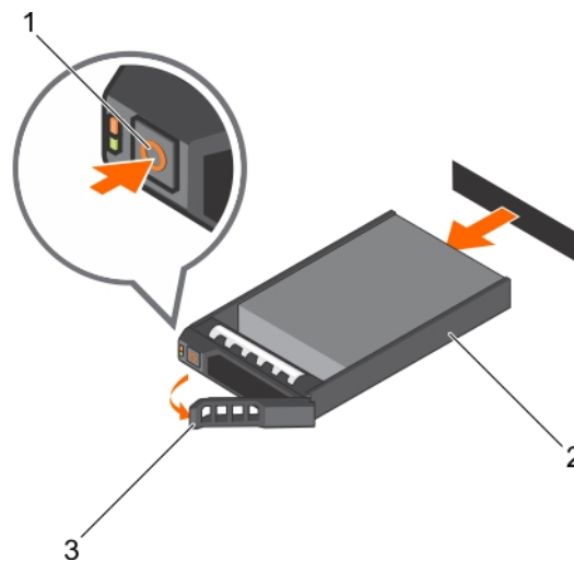
図 88. ホットスワップ対応ハードドライブまたは SSD の取り外し
