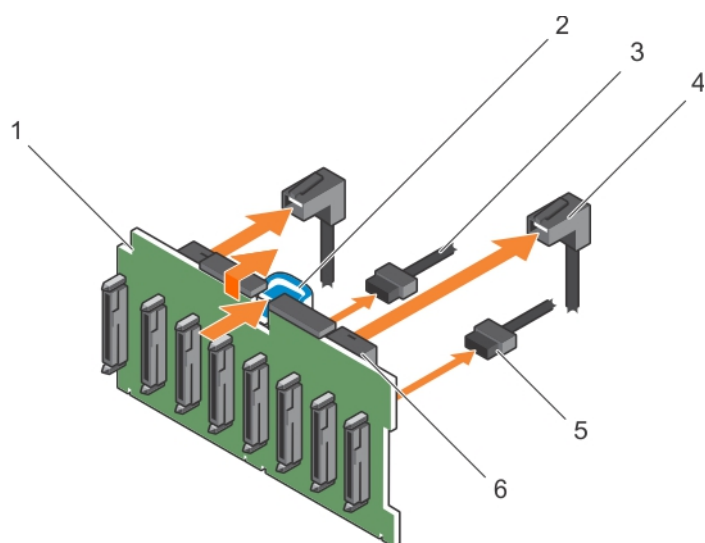
図 100. 2.5 インチ (x8) SAS/SATA バックプレーンの取り外し
