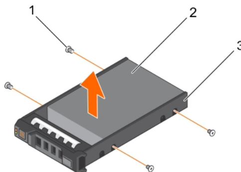
図 92. ハードドライブキャリアからのハードドライブの取り外し
