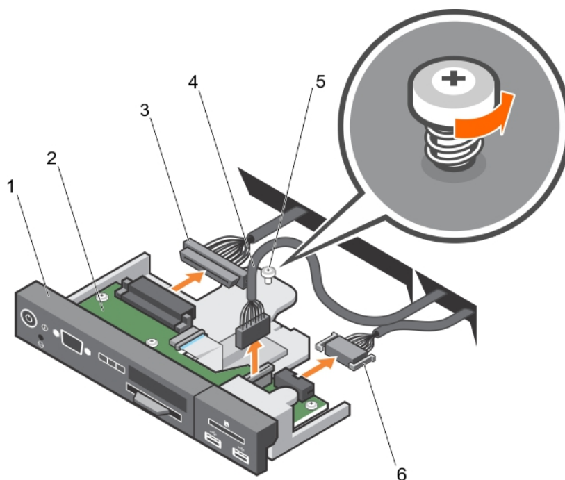
図 115. コントロール パネルの取り外し - 3.5 インチ ハード ドライブ システム
