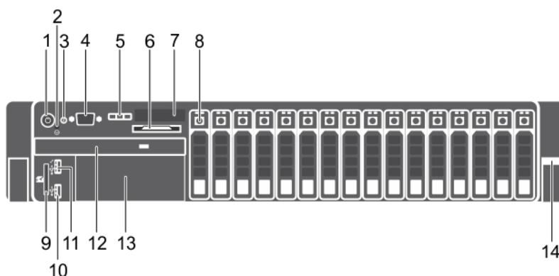
図 3. 前面パネルの機能 ( 2.5 インチハードドライブ /SSD シャーシ )
