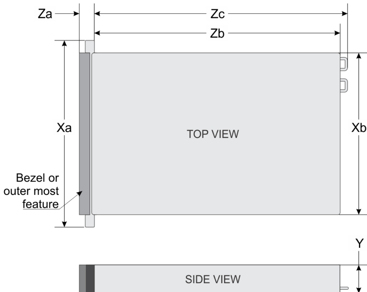
図 13. PowerEdge R730 システムのシャーシ寸法
