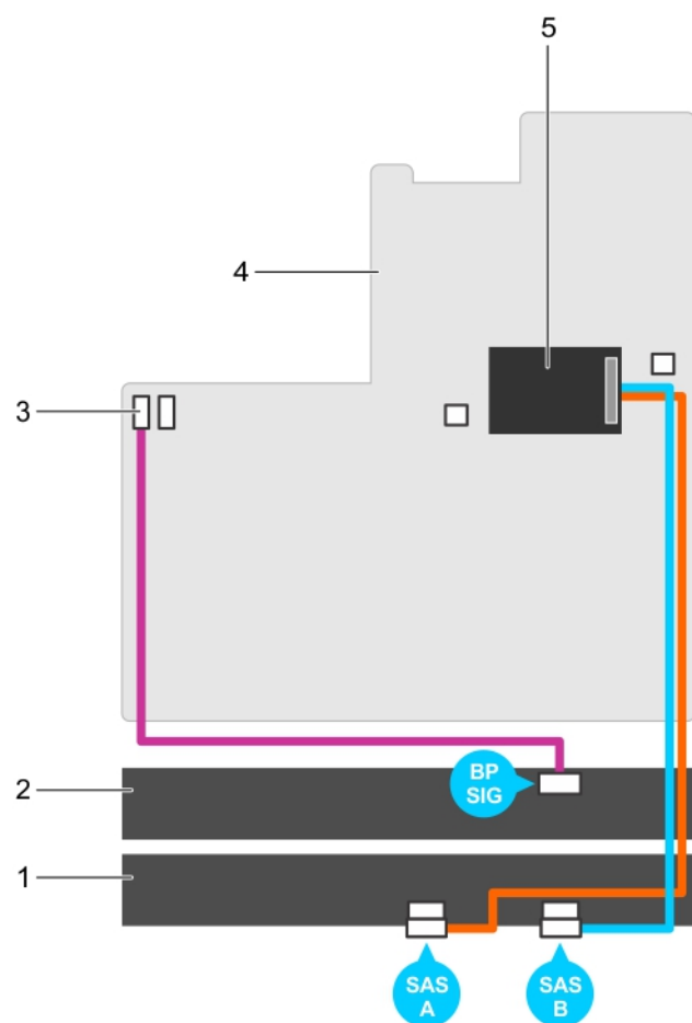
図 99. ケーブル配線図 — 2.5 インチ (x16) SAS/SATA バックプレーン
