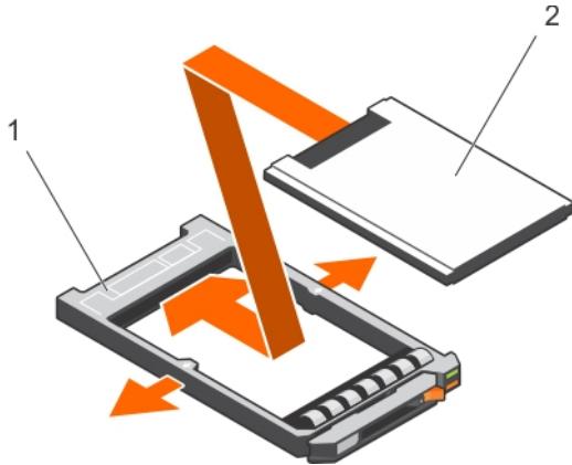
図 97. ハードドライブキャリアへの 1.8 インチハードドライブの取り付け
