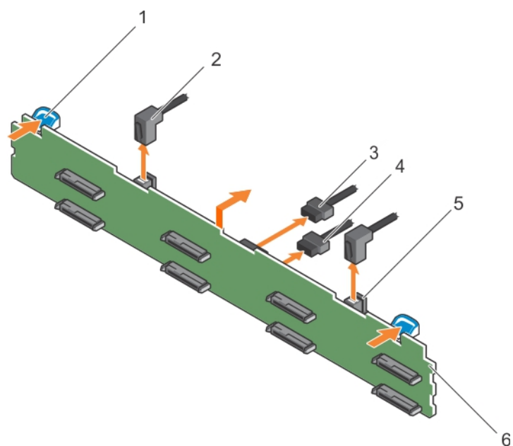
図 103. 3.5 インチ ( x8 ) SAS/SATA バックプレーンの取り外し
