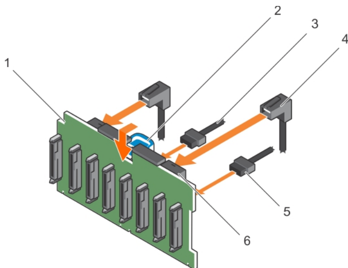
図 107. 2.5 インチ (x8) SAS/SATA バックプレーンの取り付け
