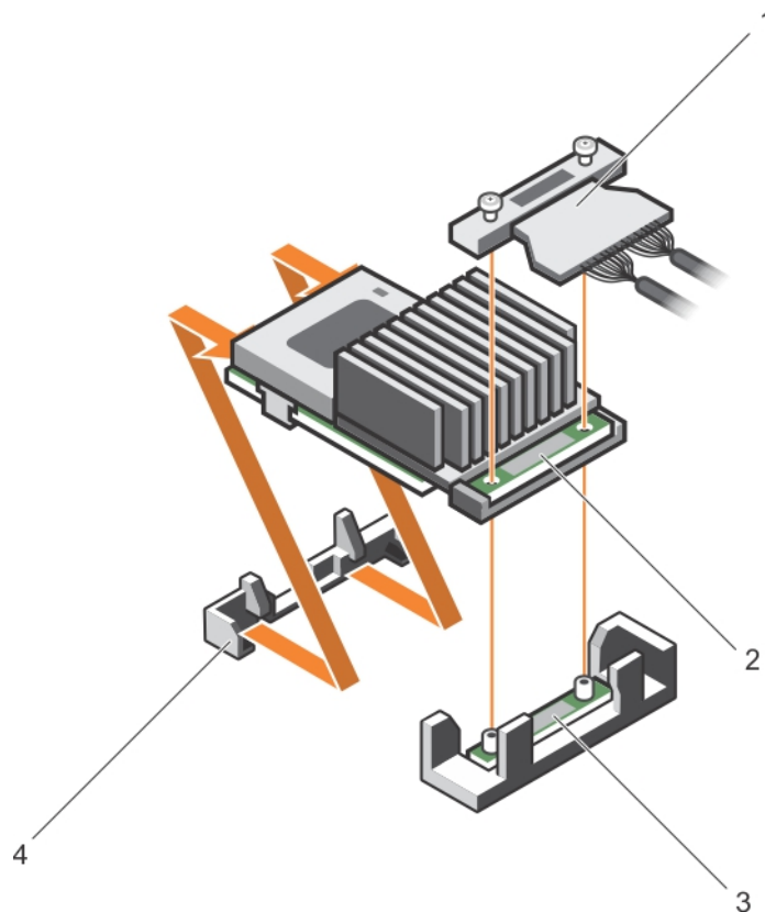
図 43. 内蔵ストレージコントローラカードの取り外し
