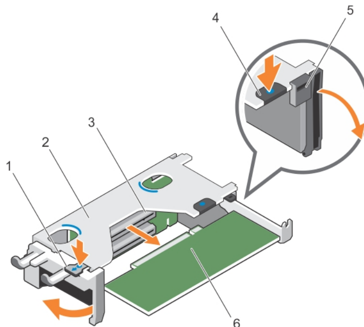
図 47. 拡張カードライザー 1 からの拡張カードの取り外し
