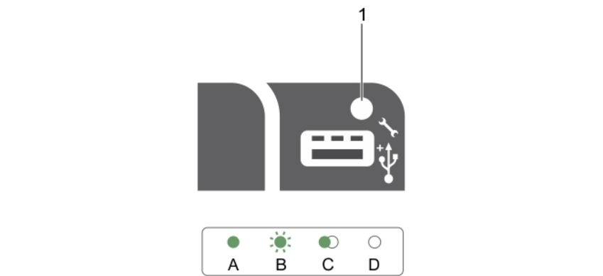
図 11. iDRAC ダイレクト LED インジケータコード
