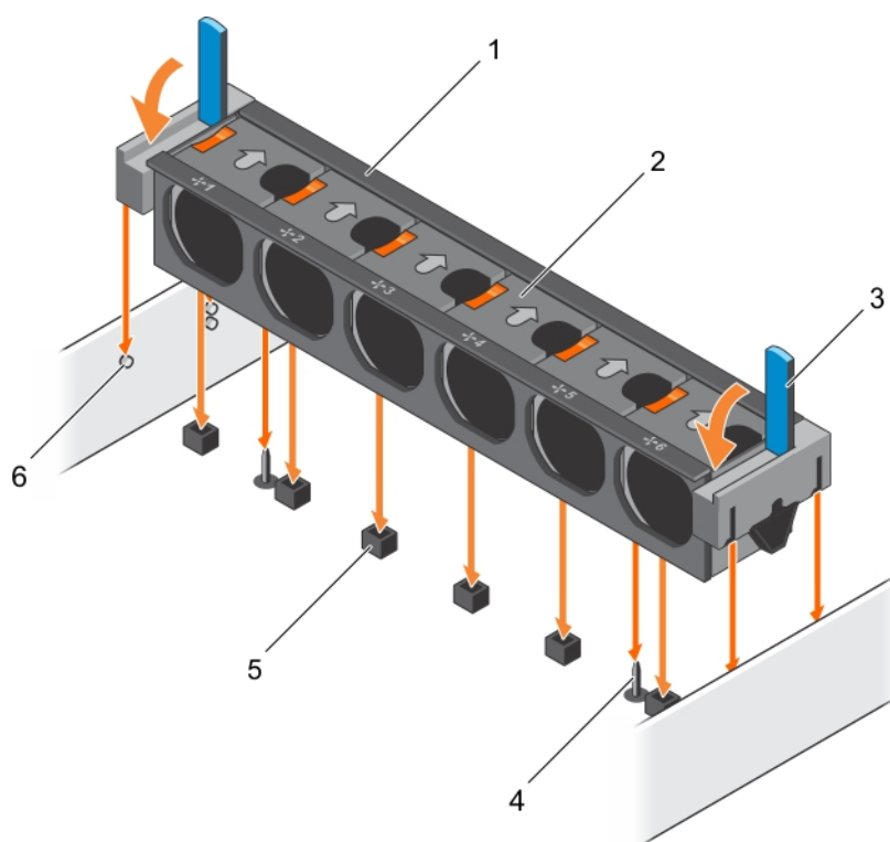
Figure 25. Installation de l'assemblage du ventilateur
