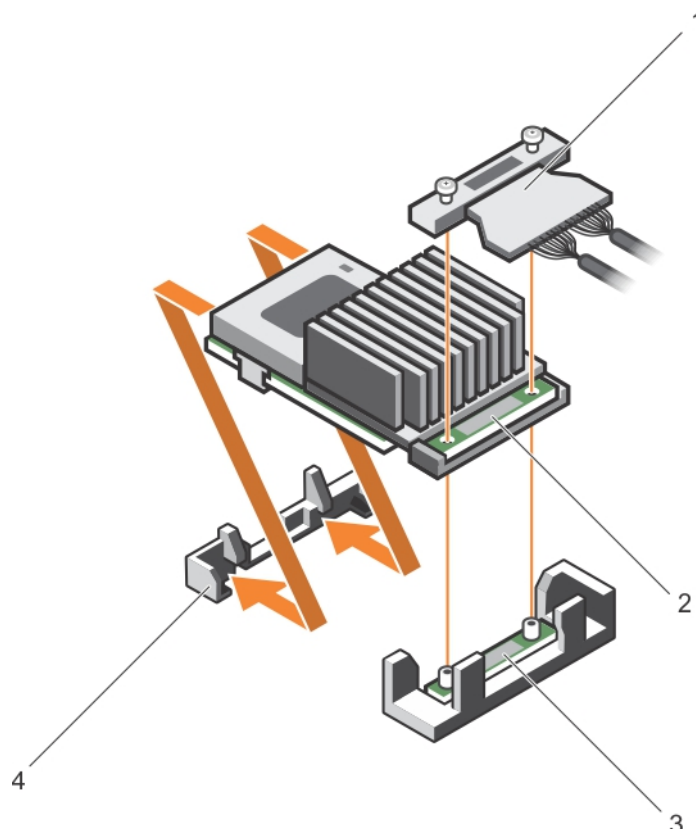
Figure 44. Installation de la carte contrôleur de stockage intégrée
