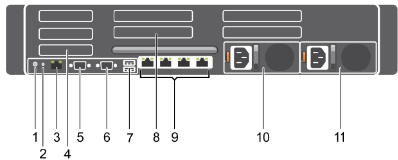
Figure 5. Caractéristiques du panneau arrière
