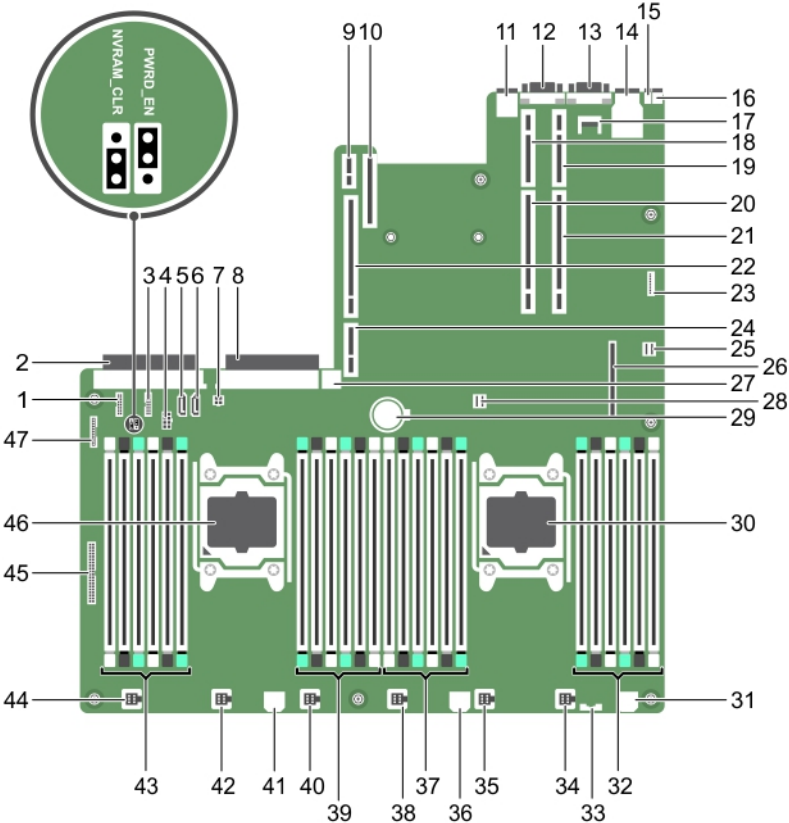
Figure 121. Connecteurs et cavaliers de la carte système
