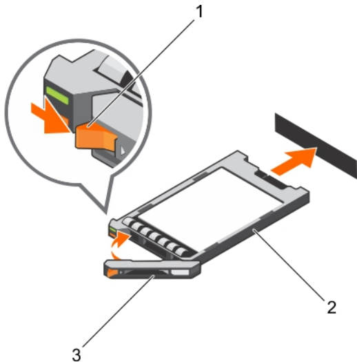
Ilustración 91. Instalación de un portaunidades de SSD uSATA de 1,8 pulgadas de intercambio directo
