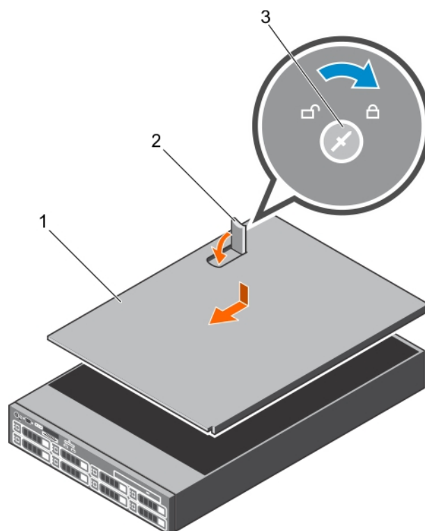
Ilustración 19. Instalación de la cubierta del sistema
