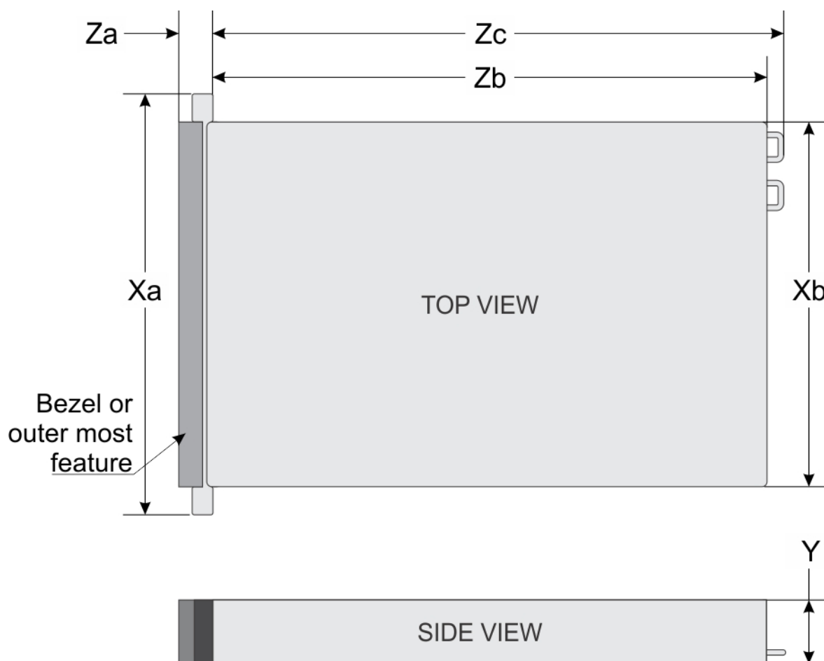
Ilustración 13. Dimensiones del chasis del sistema Dell PowerEdge R730
