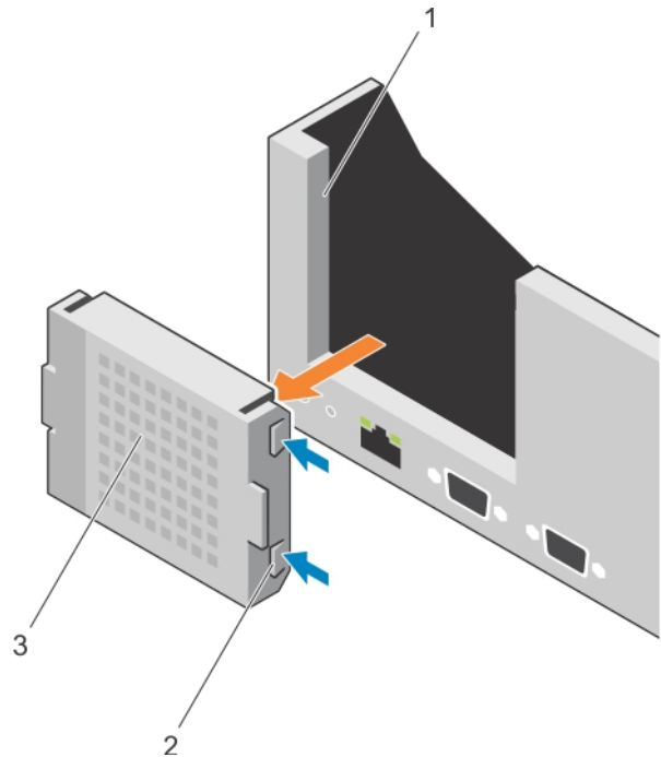
Ilustración 49. Extracción del soporte vertical de relleno 1
