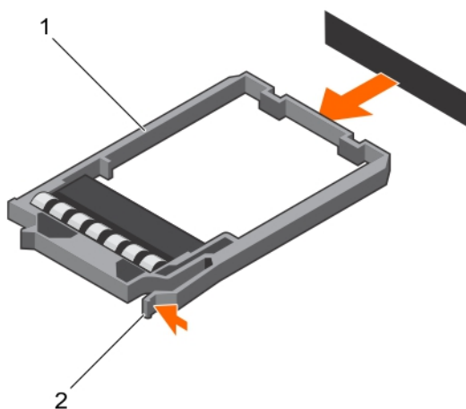
Ilustración 94. Extracción de una unidad de disco duro de relleno de 1,8 pulgadas
