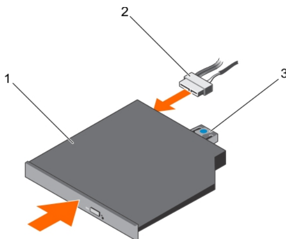
Ilustración 112. Instalación de la unidad óptica opcional
