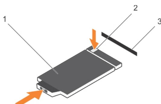
Ilustración 120. Instalación de la etiqueta de información
