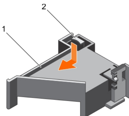
Ilustración 38. Instalación del soporte para tarjetas PCIe
