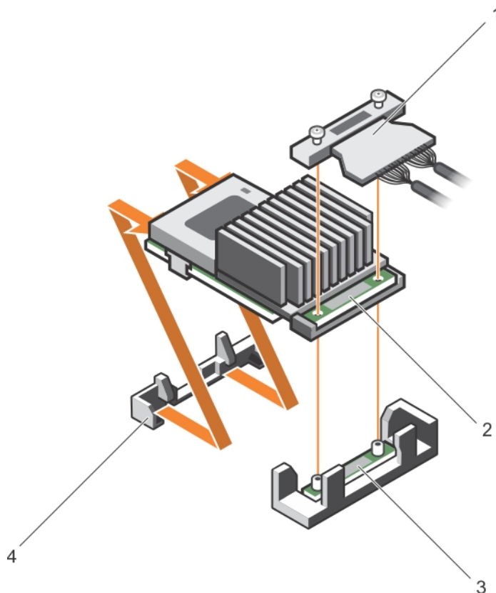
Ilustración 43. Extracción de la tarjeta controladora de almacenamiento integrada
