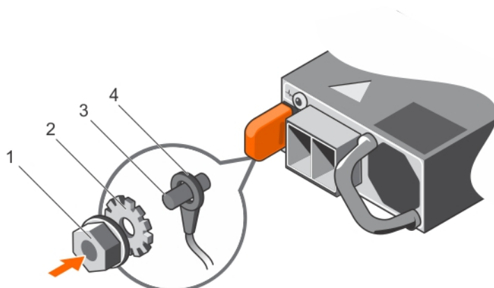
Ilustración 75. Ensamblaje y conexión del cable de toma de tierra de seguridad
