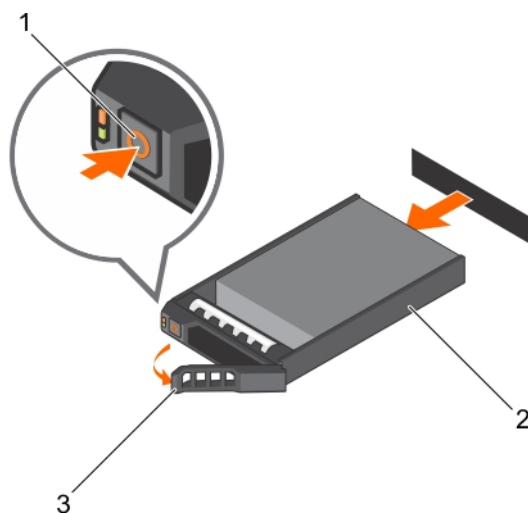
Ilustración 88. Extracción de una unidad de disco duro o SSD de intercambio directo
