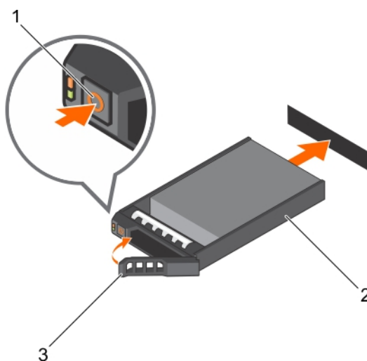
Ilustración 90. Instalación de una SSD o unidad de disco duro de intercambio directo
