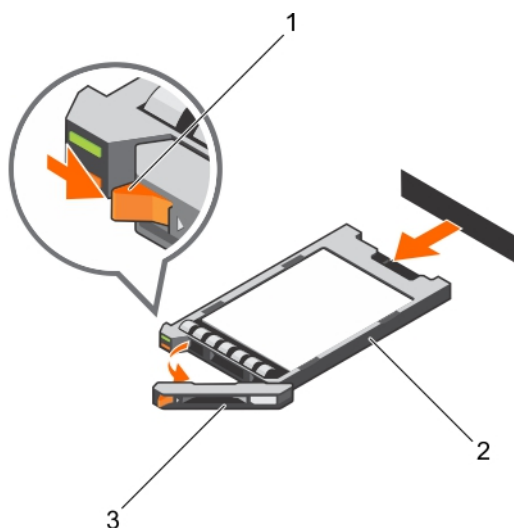
Ilustración 89. Extracción de un portaunder de SSD uSATA de 1,8 pulgadas de intercambio activo
