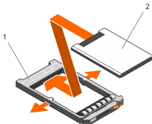
Ilustración 97. Instalación de una unidad de disco duro de 1,8 pulgadas en un portaunidades de disco duro
