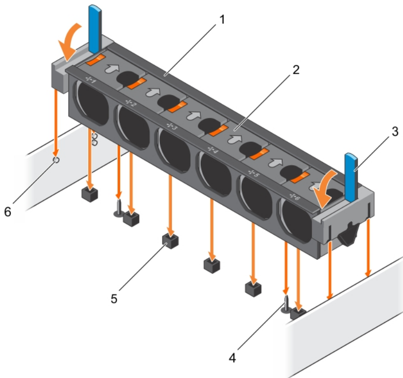
Abbildung 25. Installieren der Lüfterbaugruppe
