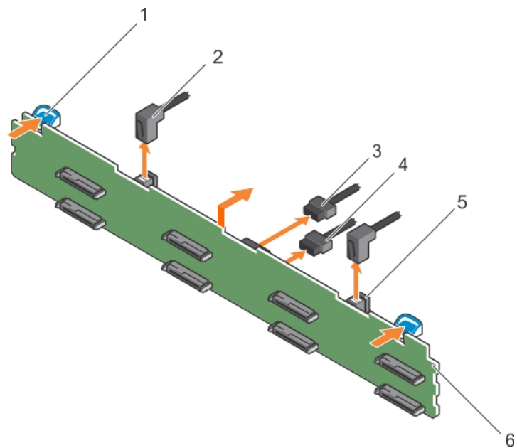
Abbildung 103. Entfernen der 3,5-Zoll-SAS/SATA-Rückwandplatine für acht Festplatten
