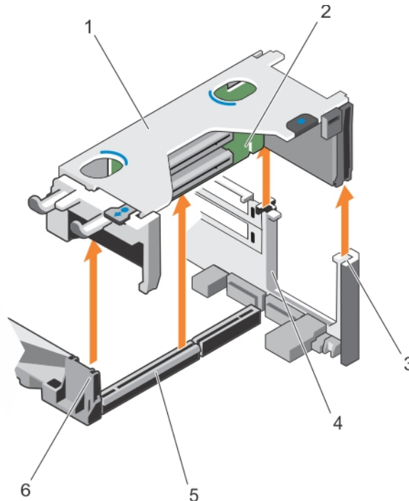
Abbildung 51. Entfernen des Erweiterungskarten-Risers 1
