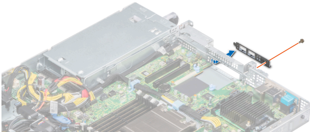
图 63: 卸下 LOM 支架
