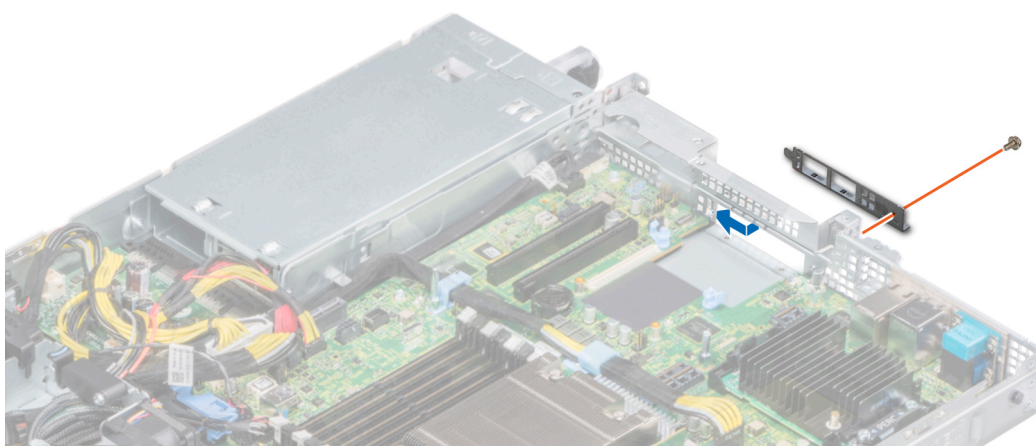
图 66: 安装 LOM 支架
