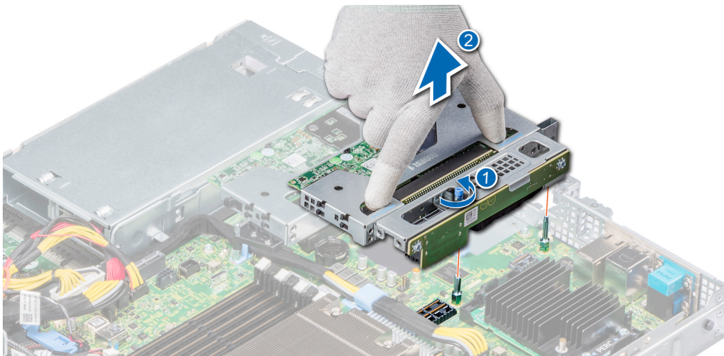
图 53: 卸下薄型右提升板
