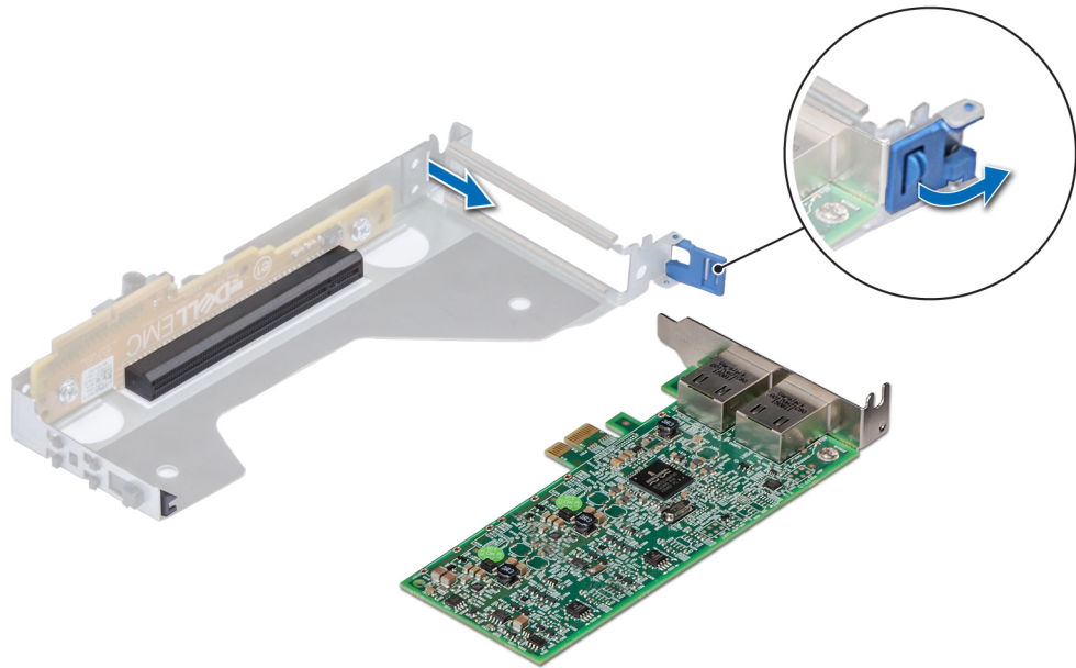
图 56: 从提升板中卸下扩充卡
