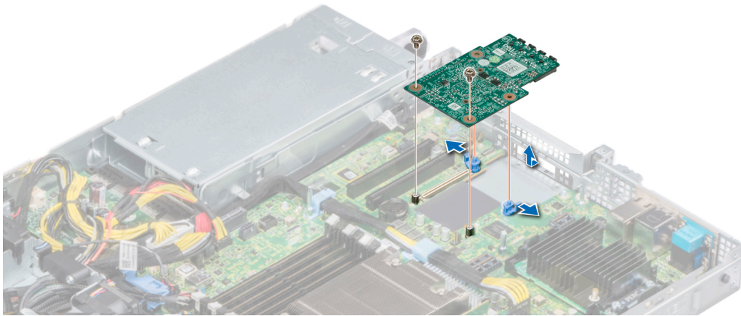
图 62: 卸下 LOM 提升卡
