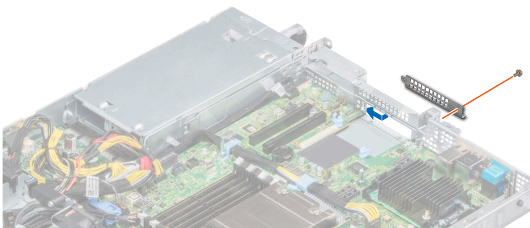
图 64: 安装 LOM 填充挡片
