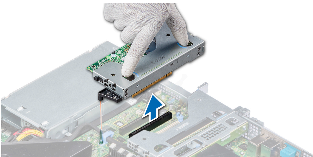
图 52: 卸下薄型左提升板
