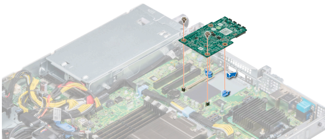
图 67: 安装 LOM 提升卡
