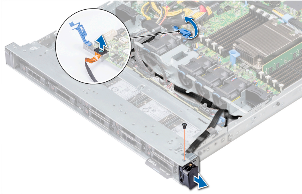
图 94: 卸下右控制面板
