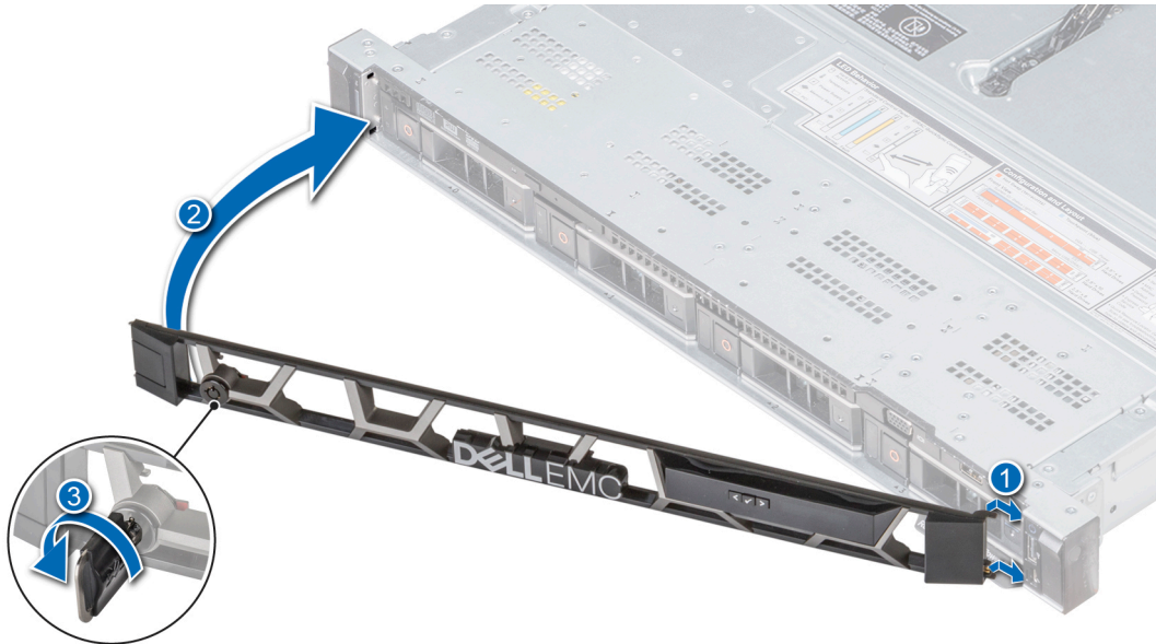
图 23: 安装带 LCD 面板的前挡板
