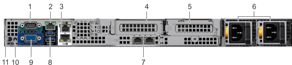
图 12: 带冗余 PSU 的系统的背面视图
