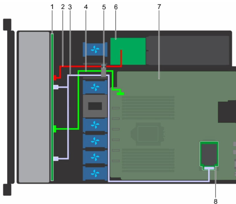
图 77: 电缆布线 - 8 x 2.5 英寸驱动器背板到 mini-PERC 卡
