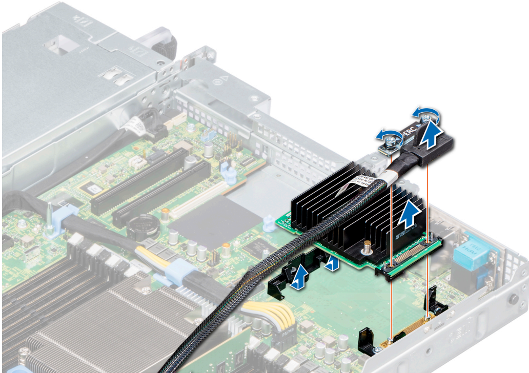
图 68: 卸下 mini PERC 卡
