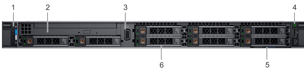
图 2: 8 x 2.5 英寸驱动器系统的前视图
