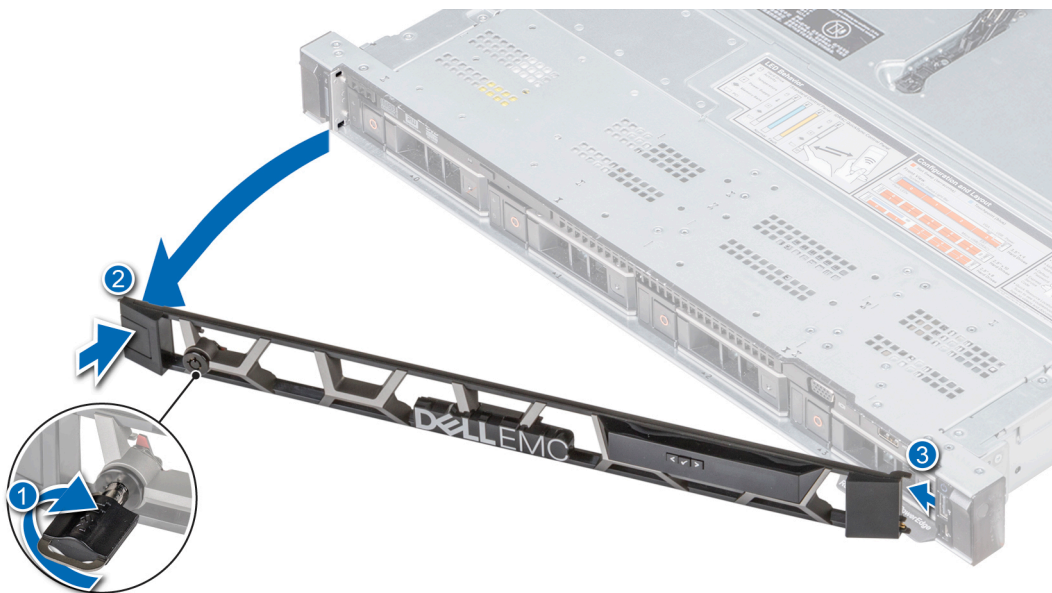
图 22: 卸下带 LCD 面板的前挡板
