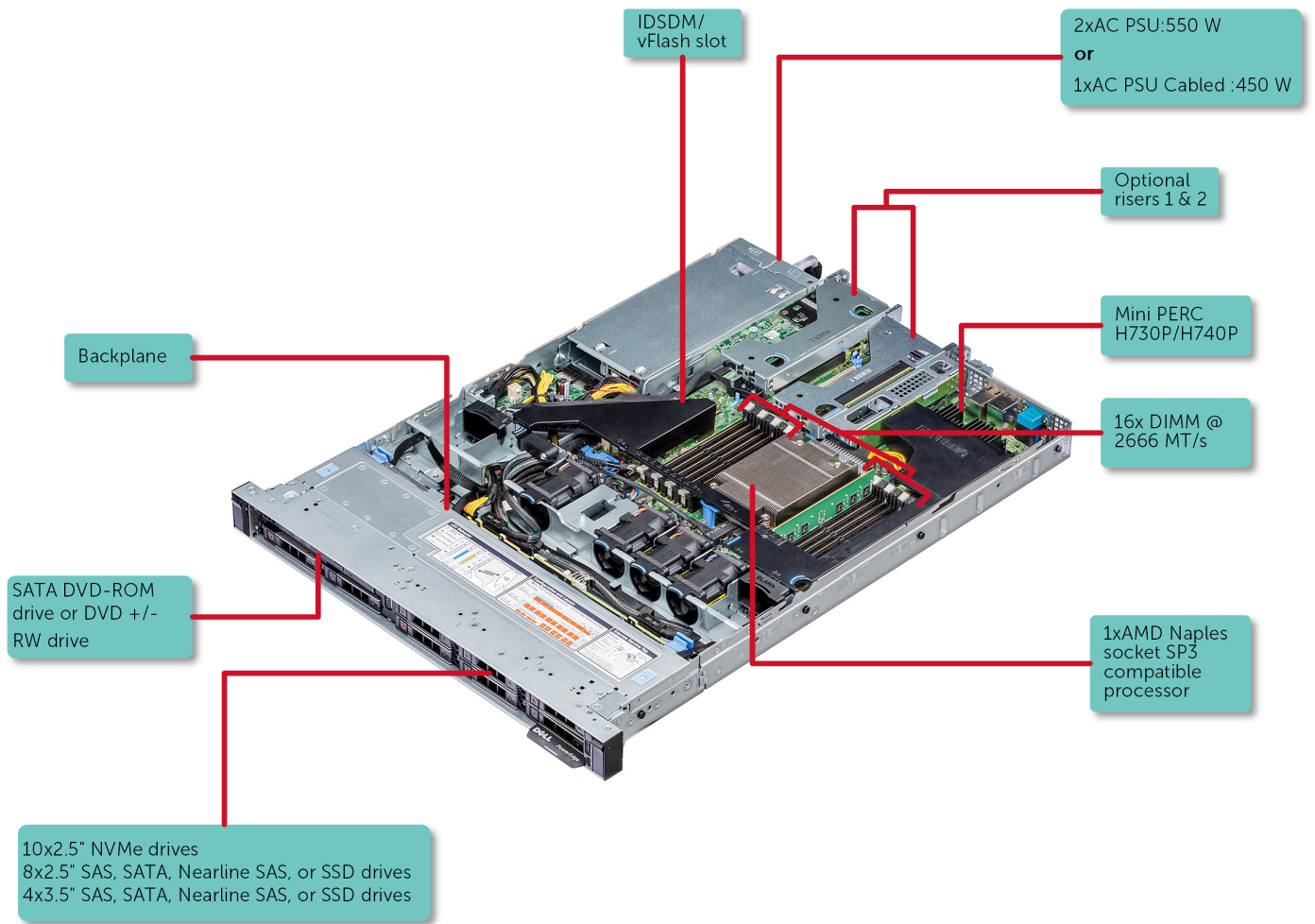
图 1: PowerEdge R6415 支持的配置
