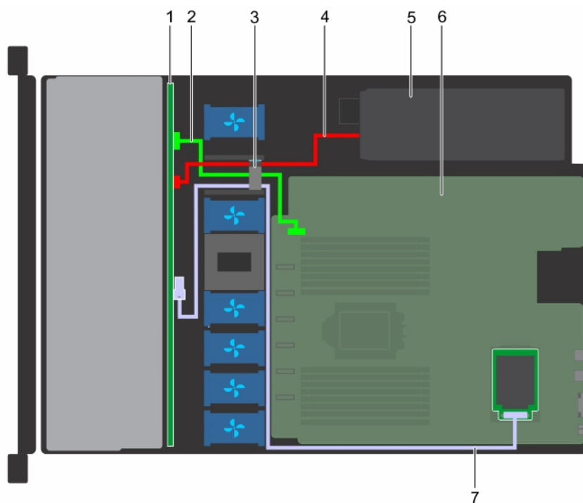
图 75: 电缆布线 - 4 x 3.5 英寸驱动器背板到 mini-PERC 卡
