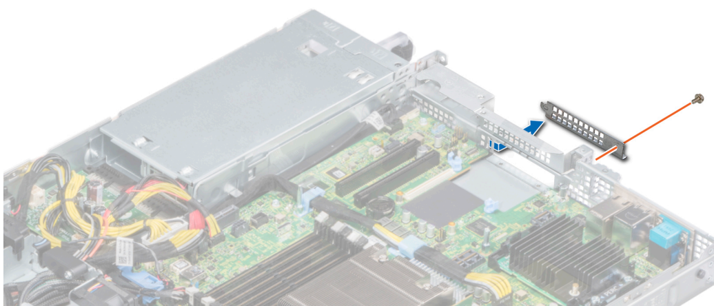
图 65: 卸下 LOM 填充挡片
