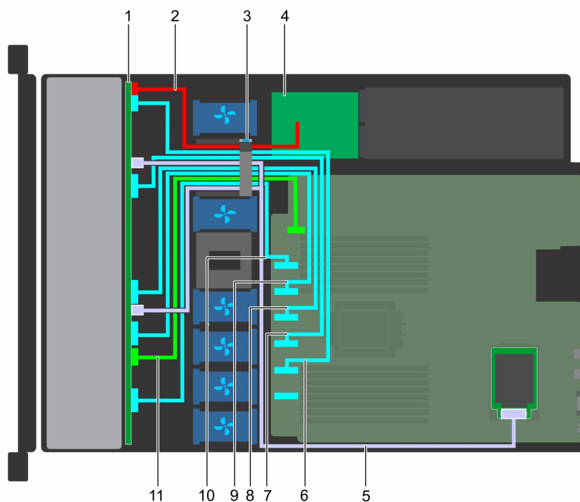
图 78: 电缆布线 — 10 x 2.5 英寸驱动器背板到机载控制器 (NVMe)
