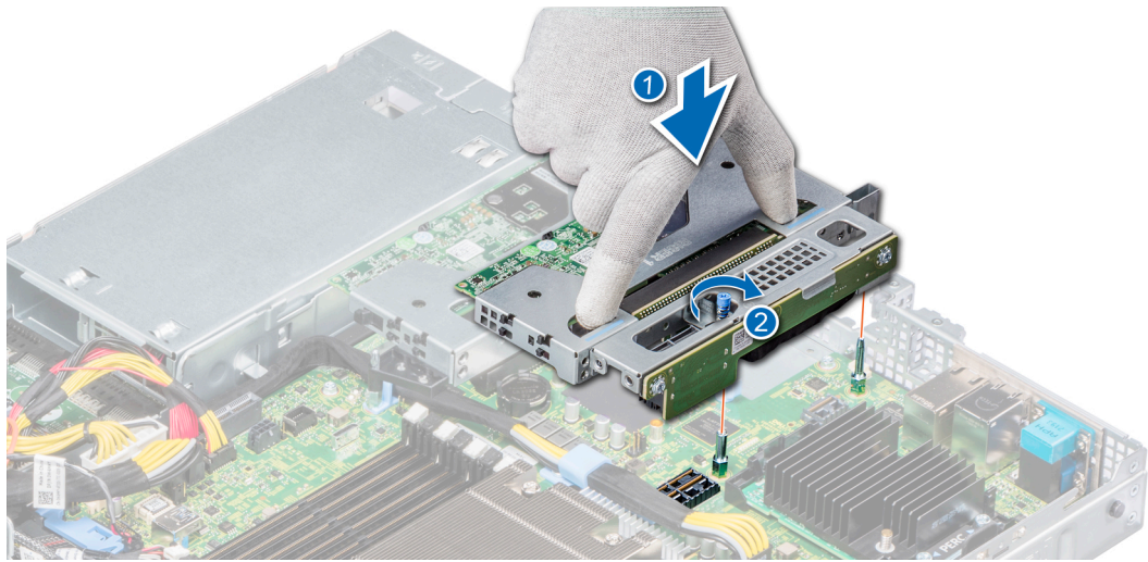
图 55: 安装薄型右提升板
