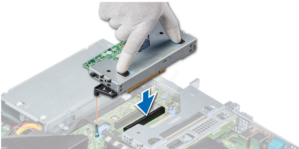
图 54: 安装薄型左提升板
