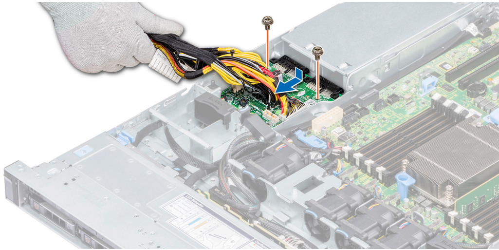
图 90: 安装电源插入器板
