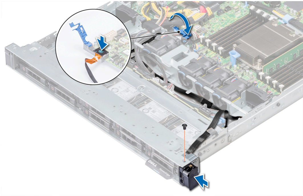
图 95: 安装右控制面板
