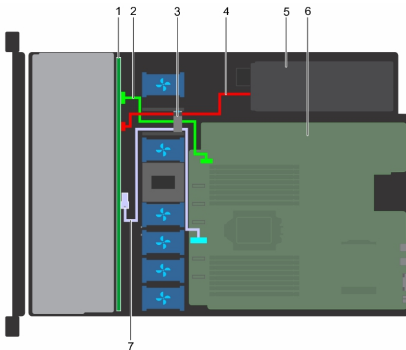
图 76: 电缆布线 — 4 x 3.5 英寸驱动器背板到机载控制器
