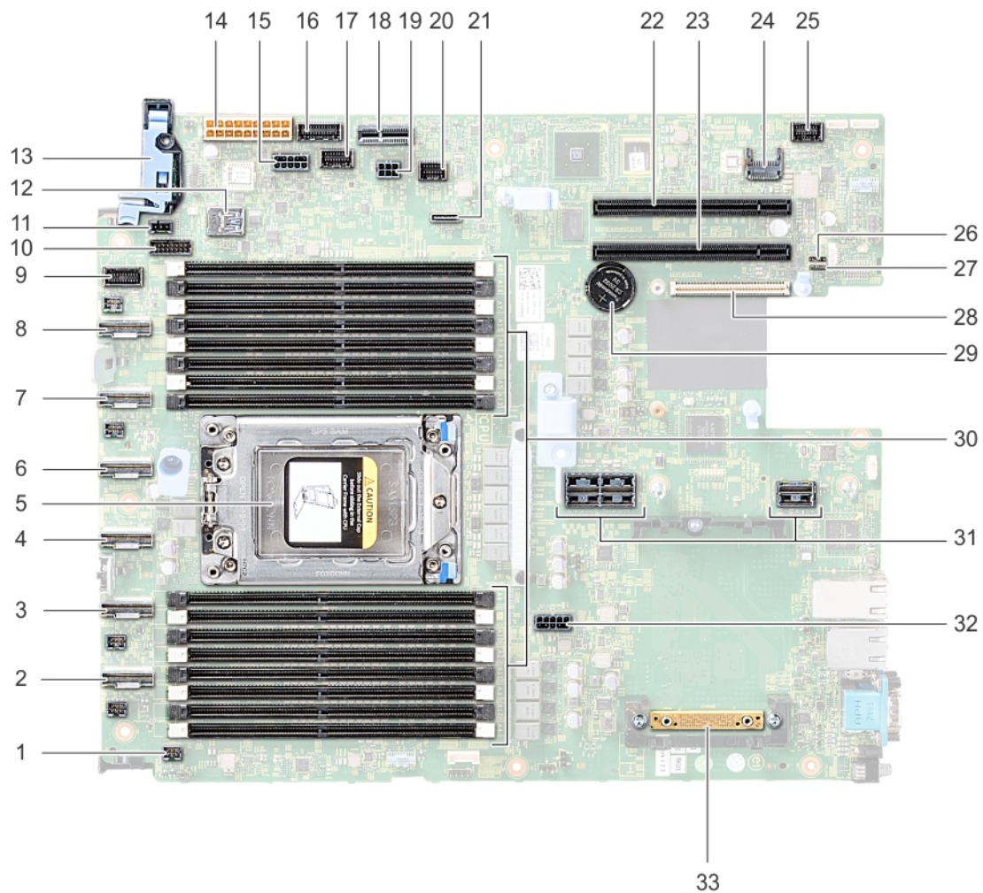
图 100: 系统板跳线和连接器
