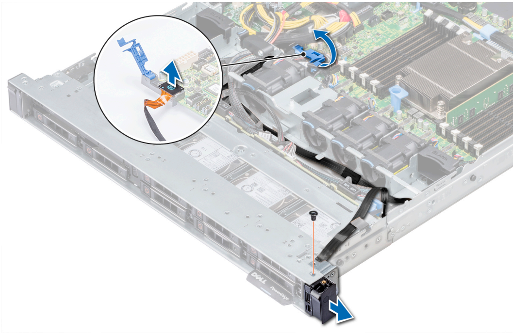
그림 94 . 오른쪽 제어판 분리
