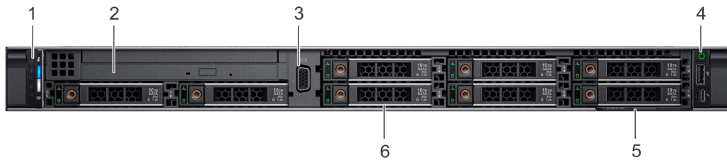
그림 2. 8개 6.35cm(2.5인치) 드라이브 시스템의 전면 모습
