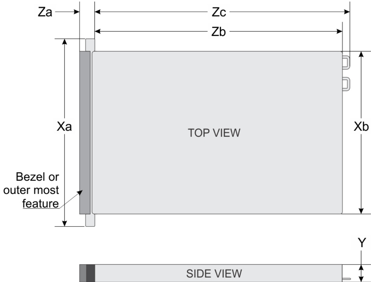
그림 21. PowerEdge R6415 시스템의 크기
