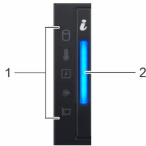
그림 5 . iDRAC Quick Sync 2.0 표시등(선택 사항)이 없는 왼쪽 컨트롤 패널
