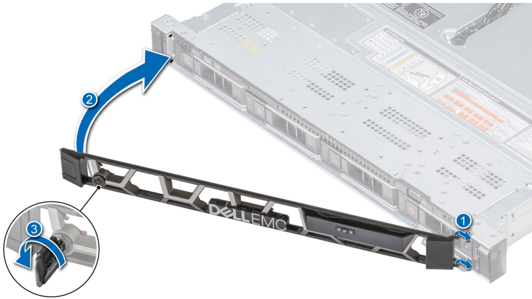
그림 23 . LCD 패널을 포함하는 전면 베젤 설치
