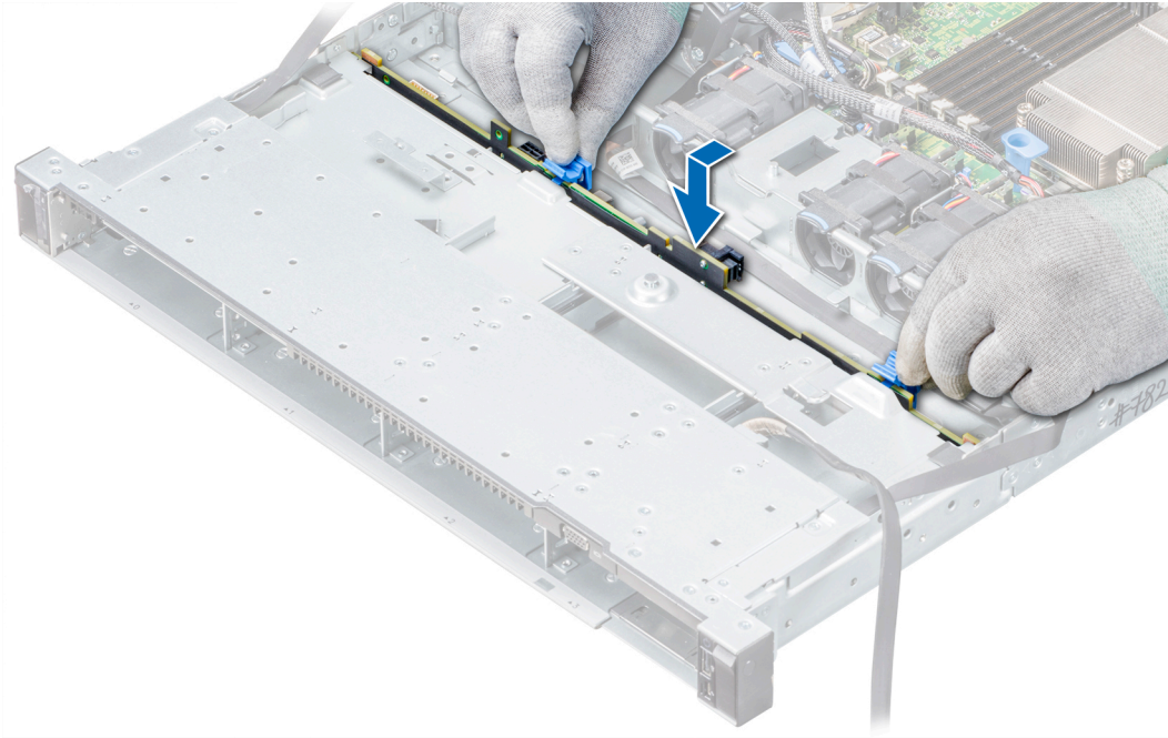
그림 74. 후면판 설치
