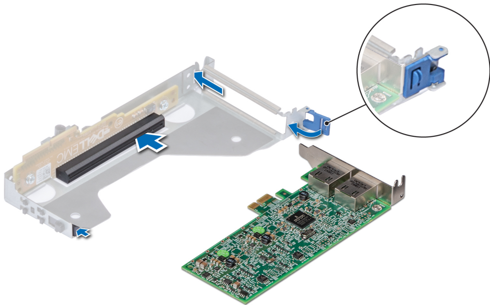
그림 59. 라이저에 확장 카드 설치
