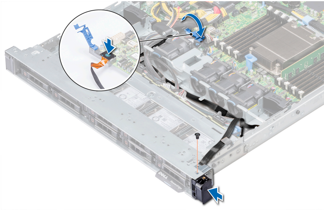
그림 95 . 오른쪽 제어판 설치
