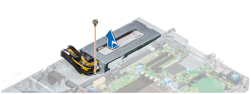
그림 87. 케이블 연결된 PSU 분리
