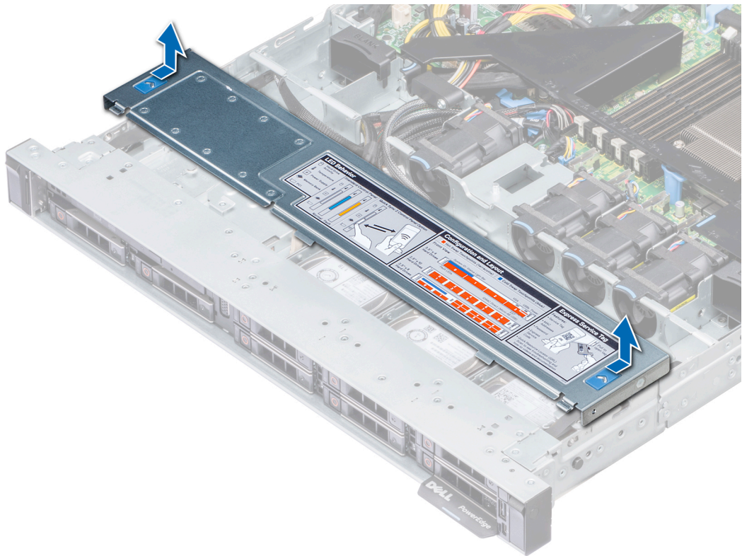
그림 26. 후면판 덮개 분리
