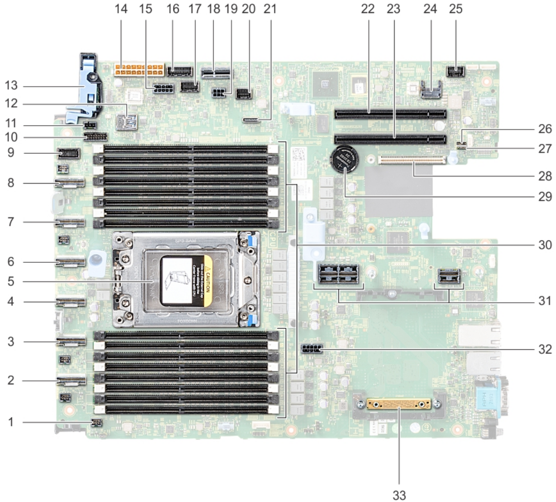
그림 100. 시스템 보드 점퍼 및 커넥터
