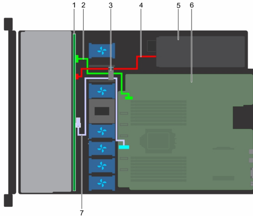
그림 76. 케이블 배선 - 4개의 3.5인치 드라이브 후면판과 온보드 컨트롤러
