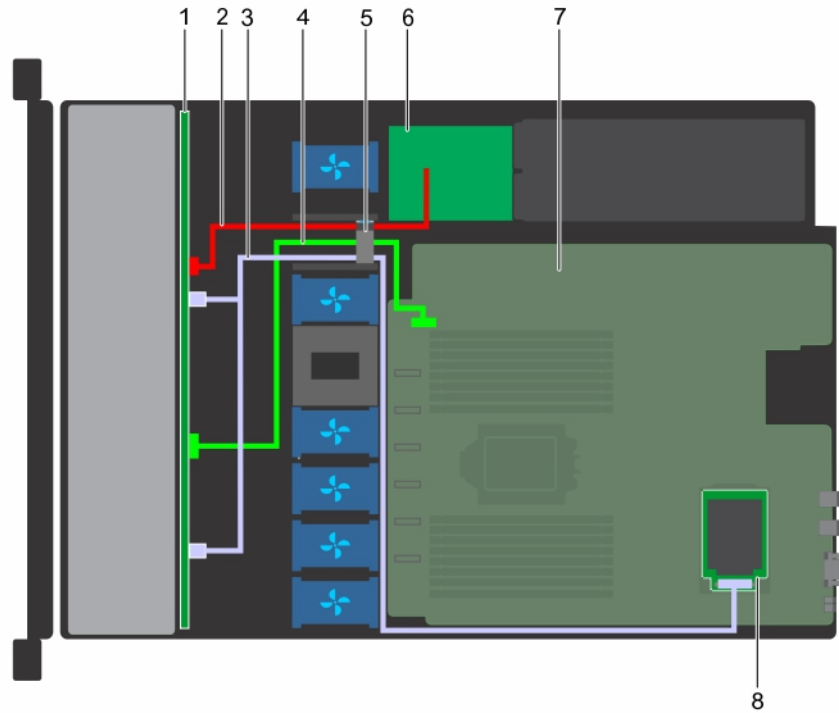
그림 77. 케이블 배선 - 8개의 2.5인치 드라이브 후면판과 미니 PERC 카드
