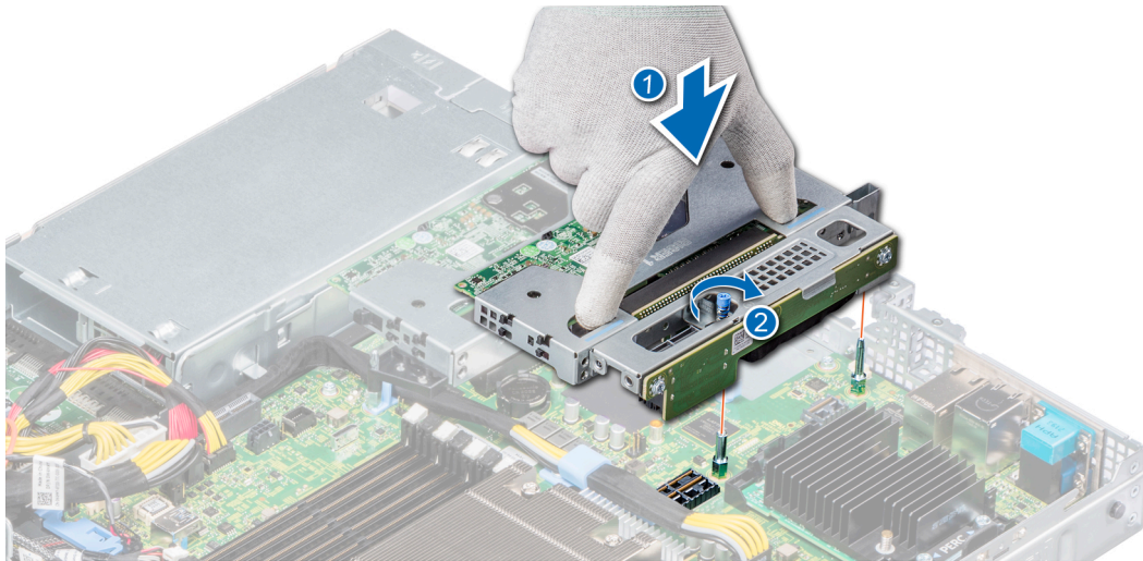
그림 55. 로우 프로파일 오른쪽 라이저 설치
