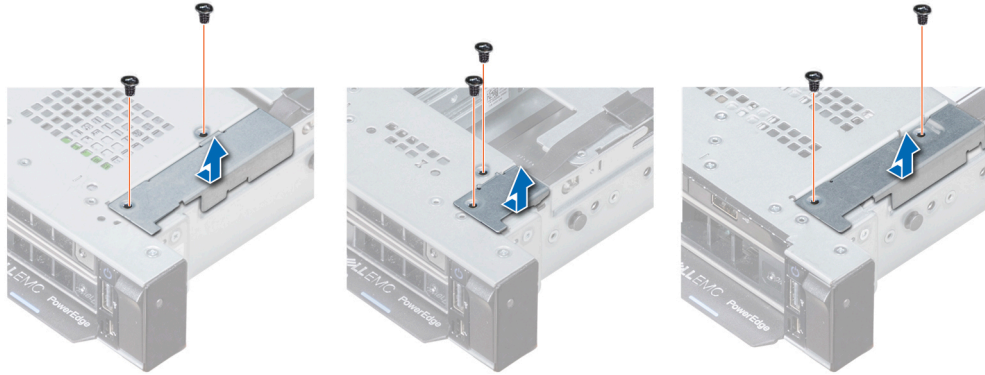
그림 93. 케이블 덮개 분리
