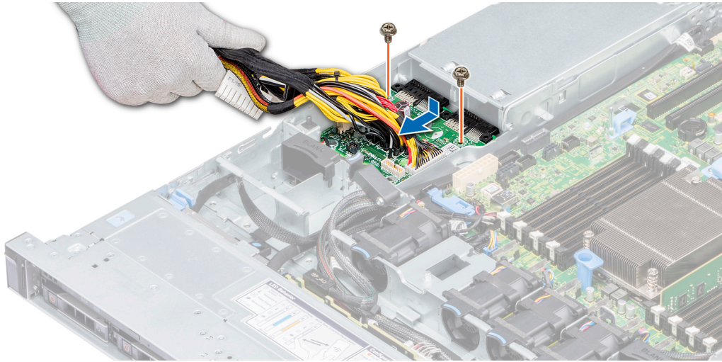
그림 90. 전원 점속기 보드 설치
