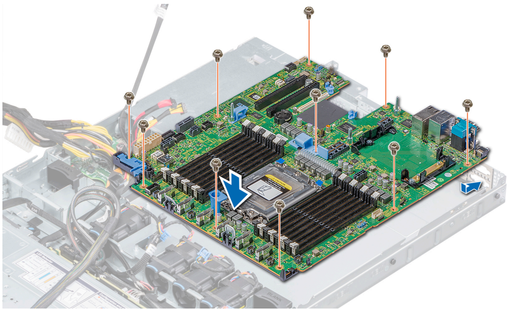
그림 98. 시스템 보드 설치
