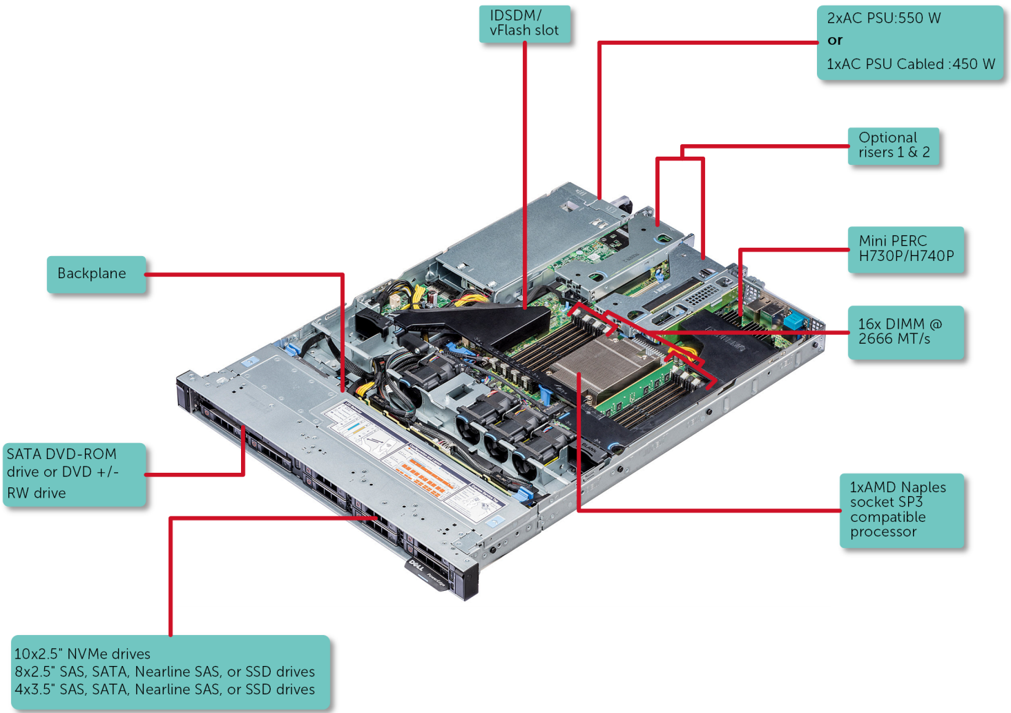
그림 1. PowerEdge R6415 시스템이 지원하는 구성
