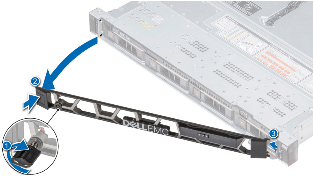
그림 22. LCD 패널을 포함하는 전면 베젤 분리
