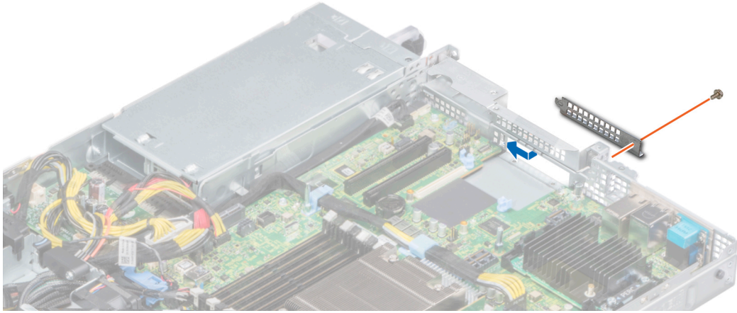
그림 64. LOM 필러 브래킷 설치
