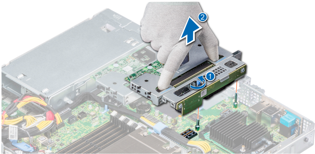
그림 53. 로우 프로파일 오른쪽 라이저 분리
