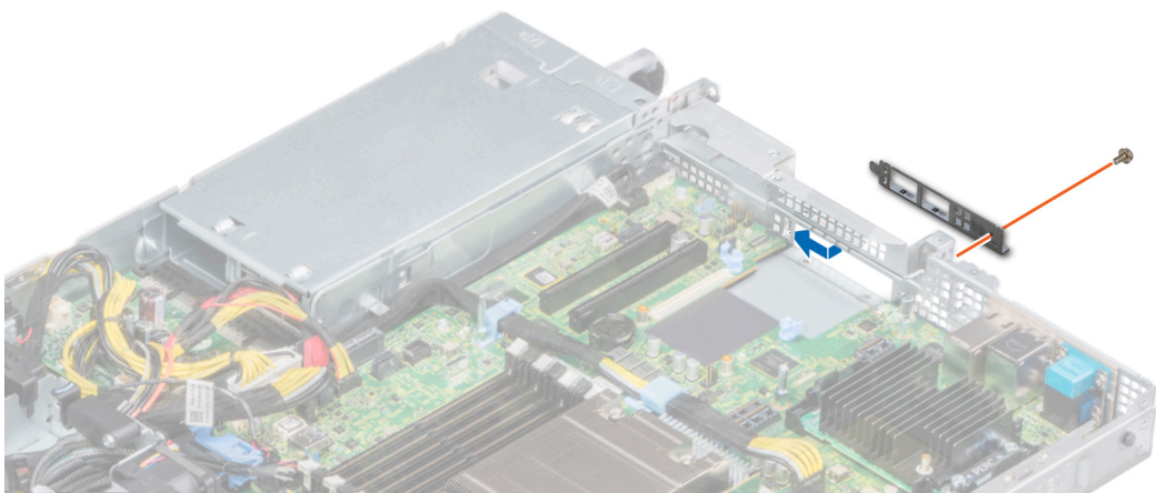
그림 66 . LOM 브래킷 설치
