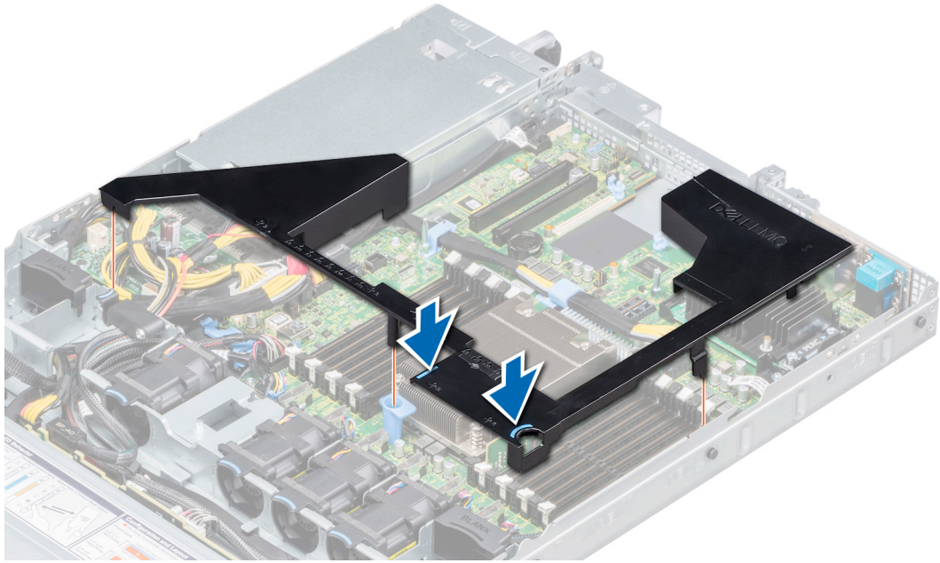
그림 30. 공기 덮개 장착
