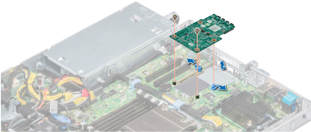
그림 62. LOM 라이저 카드 분리
