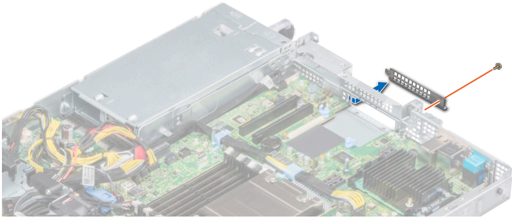
그림 65 . LOM 필러 브래킷 분리
