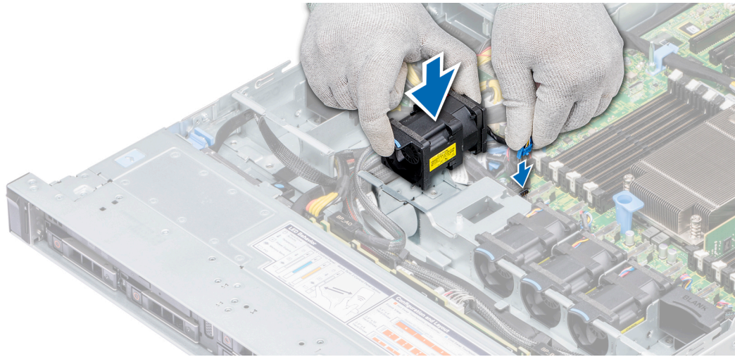
그림 32. 냉각 팬 설치
