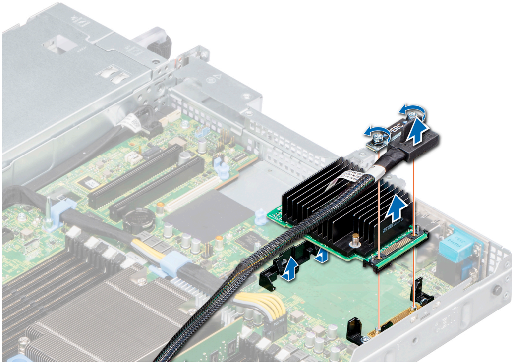
그림 68 . 미니 PERC 카드 분리
