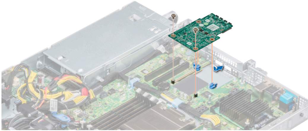
그림 67. LOM 라이저 카드 설치
