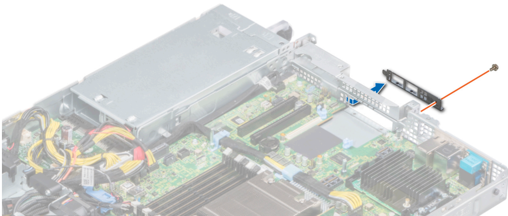
그림 63. LOM 브래킷 분리
