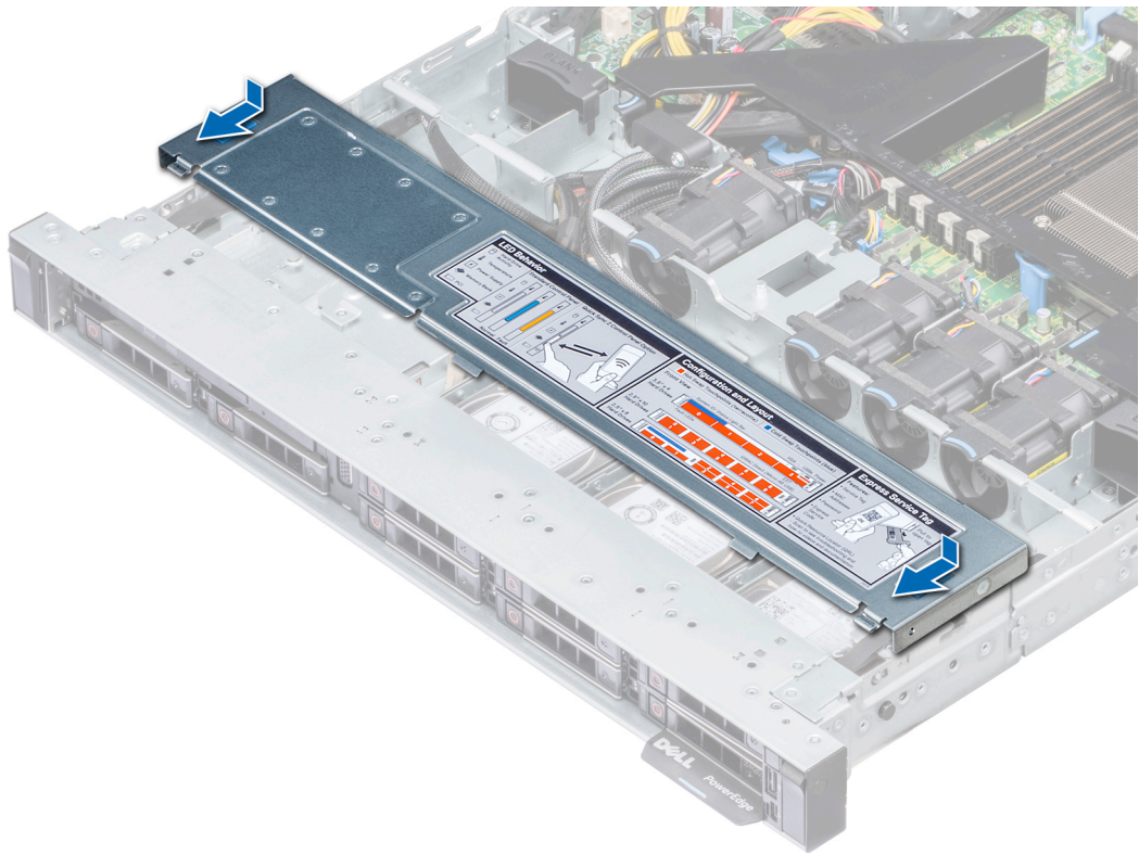
그림 27. 후면판 덮개 설치
