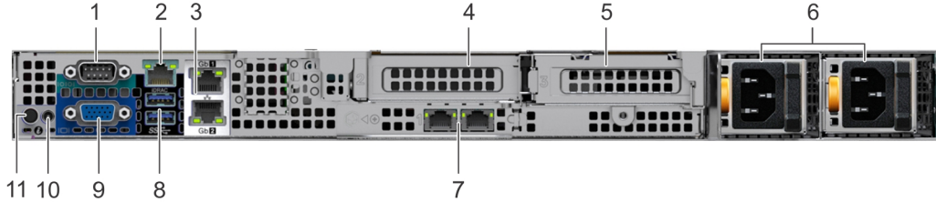
그림 12. 이중화된 PSU가 있는 시스템의 후면 모습
