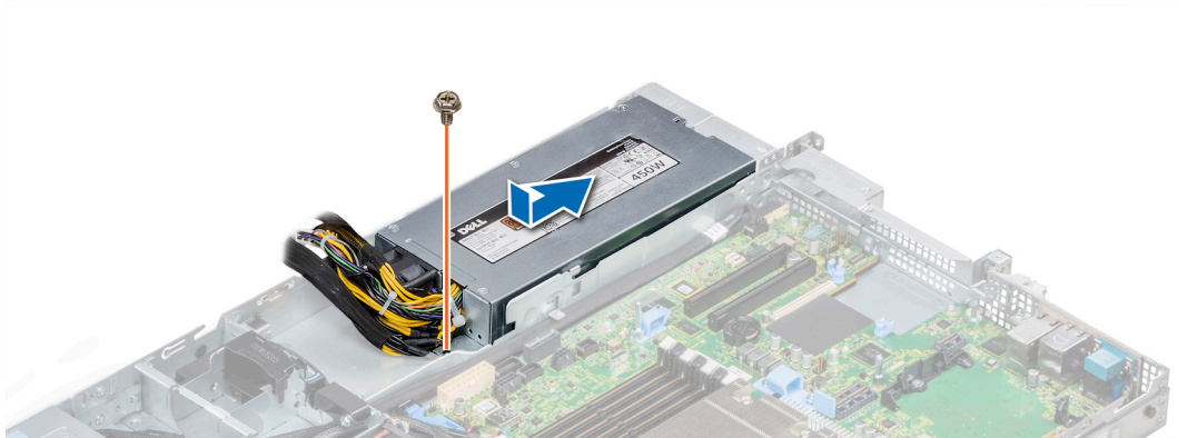
그림 88. 케이블 연결된 PSU 설치
