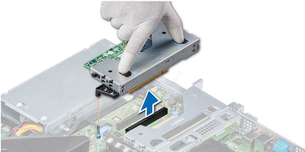
그림 52. 로우 프로파일 왼쪽 라이저 분리
