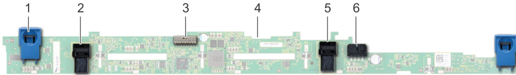
그림 71. 8개의 2.5 드라이브 후면판
