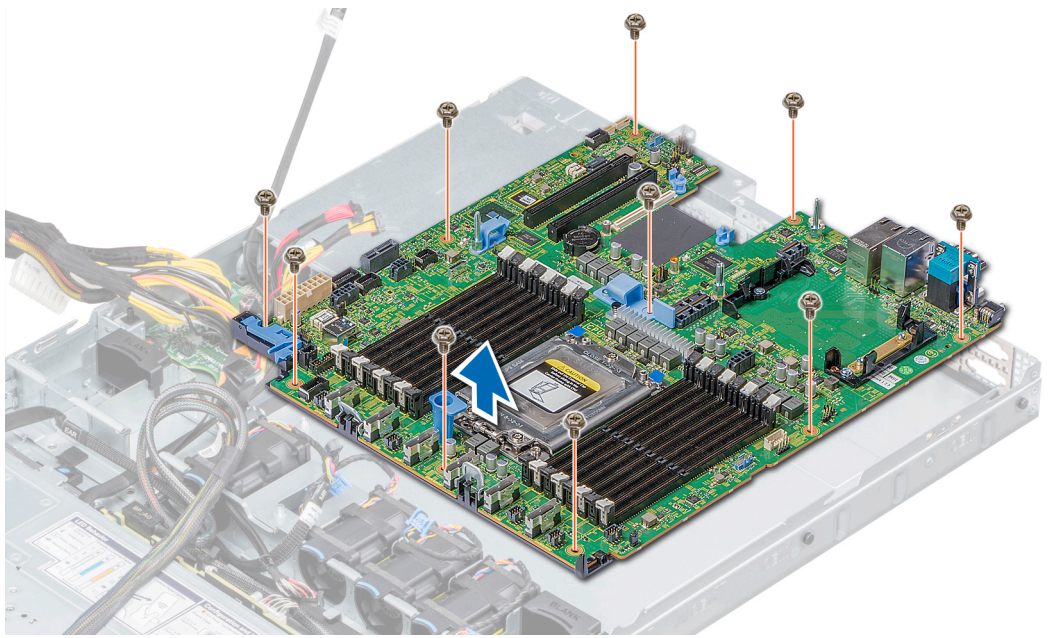
그림 97. 시스템 보드 제거
