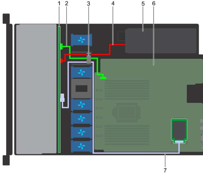
그림 75. 케이블 배선 - 4개의 3.5인치 드라이브 후면판과 미니 PERC 카드
