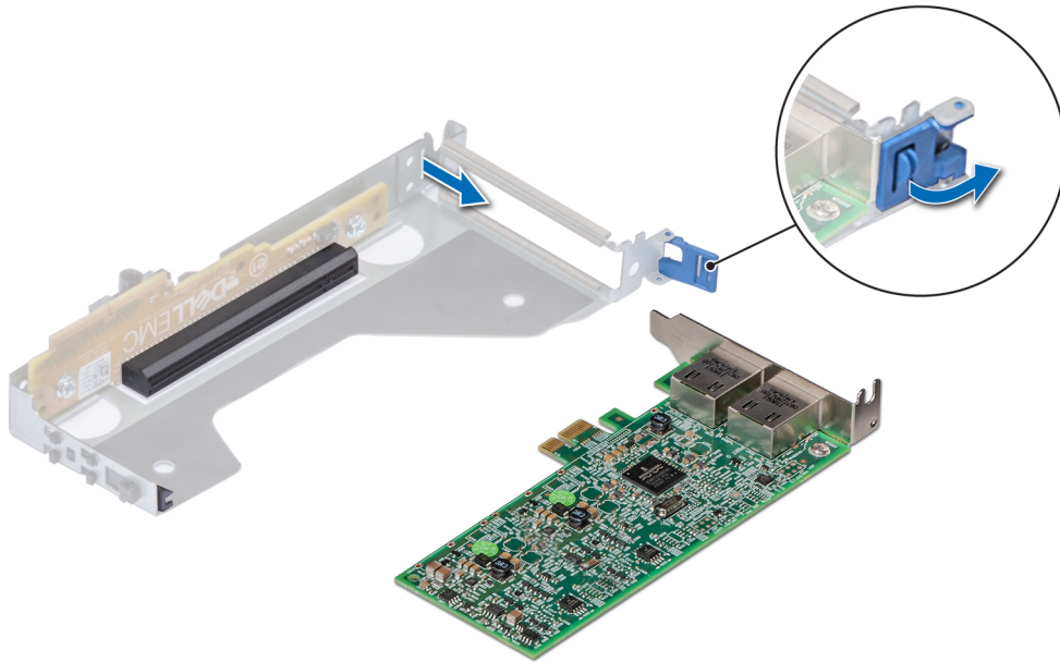
그림 56. 라이저에서 확장 카드 분리
