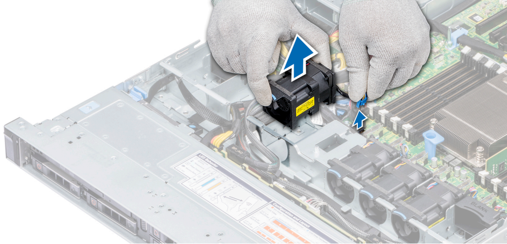
그림 31. 냉각 팬 분리
