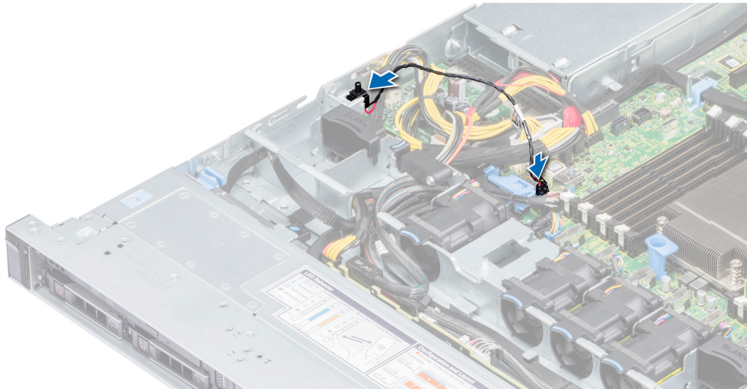
그림 34. 침입 스위치 설치
