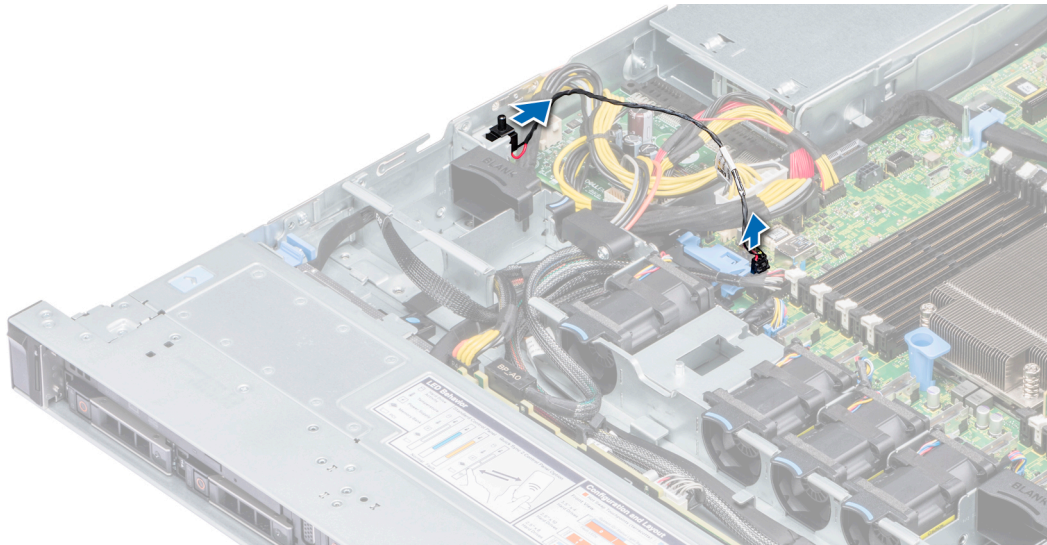
그림 33. 침입 스위치 제거
