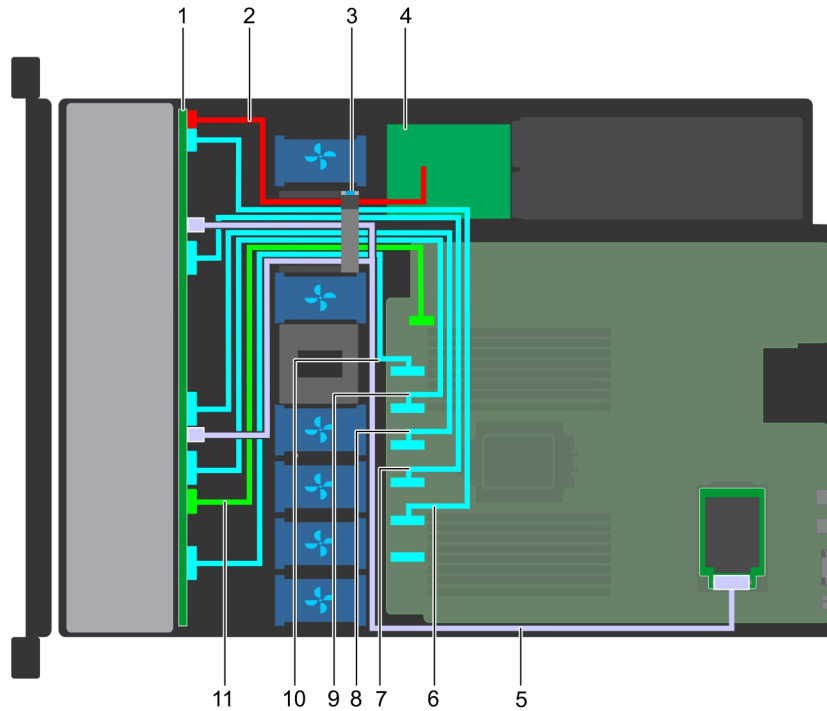
그림 78. 케이블 배선 - 10개의 2.5인치 드라이브 후면판과 온보드 컨트롤러(NVMe)
