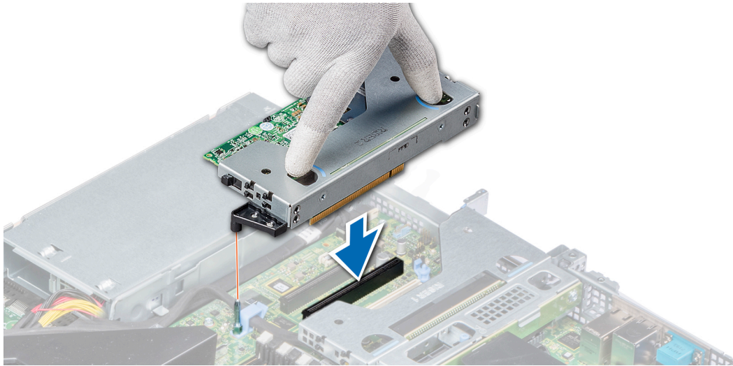
그림 54. 로우 프로파일 왼쪽 라이저 설치
