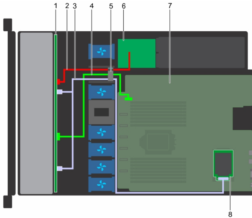
Figure 77. Acheminement des câbles : fond de panier de 8 disques de 2,5 pouces avec carte mini-PCIe
