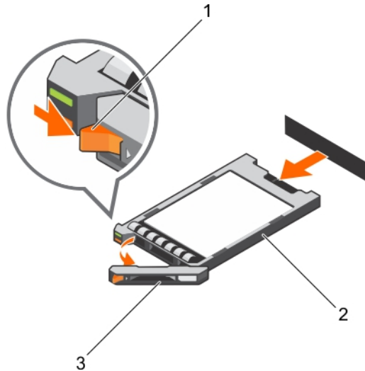
그림 34. 1.8인치 핫 스왑 가능 uSATA SSD 캐리어 분리
