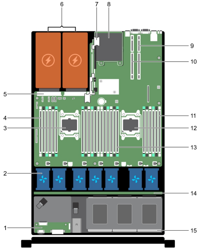
그림 22. 시스템 내부 — 8개 하드 드라이브 시스템
