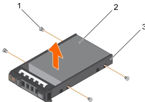
그림 37 . 하드 드라이브 캐리어에서 하드 드라이브 분리
