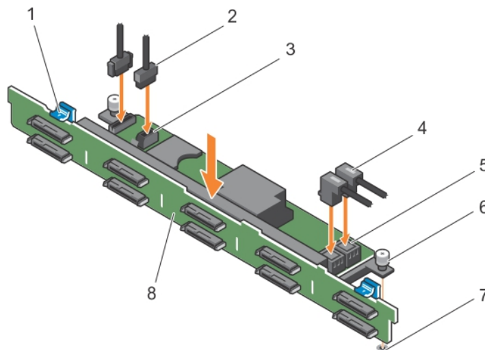
그림 86 . 2.5인치(x10) 하드 드라이브 후면판 설치
