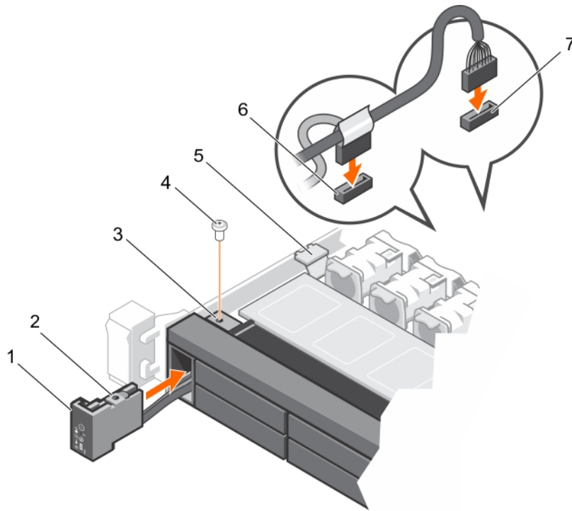
그림 93. 10 하드 드라이브 및 24 하드 드라이브 시스템의 제어판 설치
