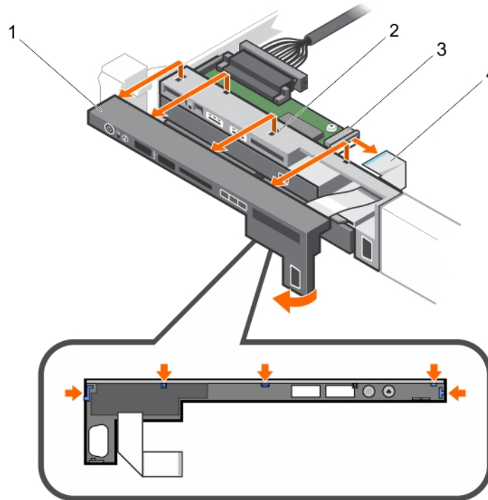
그림 90 . 8개 하드 드라이브 시스템의 제어판 분리
