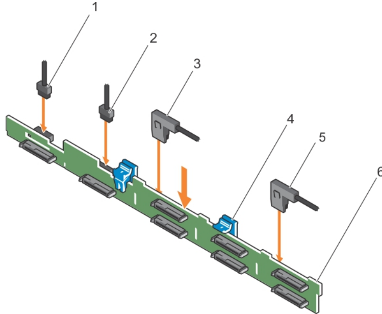
그림 85 . 2.5인치(x8) 하드 드라이브 후면판 설치
