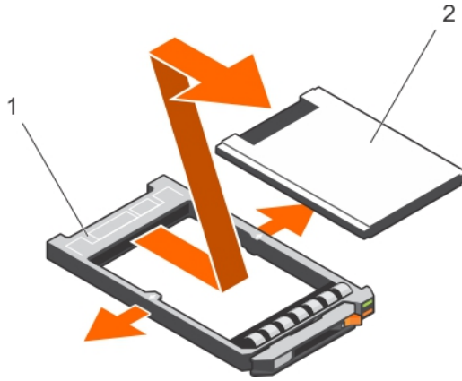
그림 39 . 하드 드라이브 캐리어에서 1.8인치 하드 드라이브 분리
