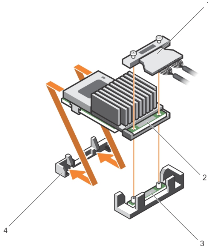
그림 58. 내장형 스토리지 컨트롤러 카드 설치
