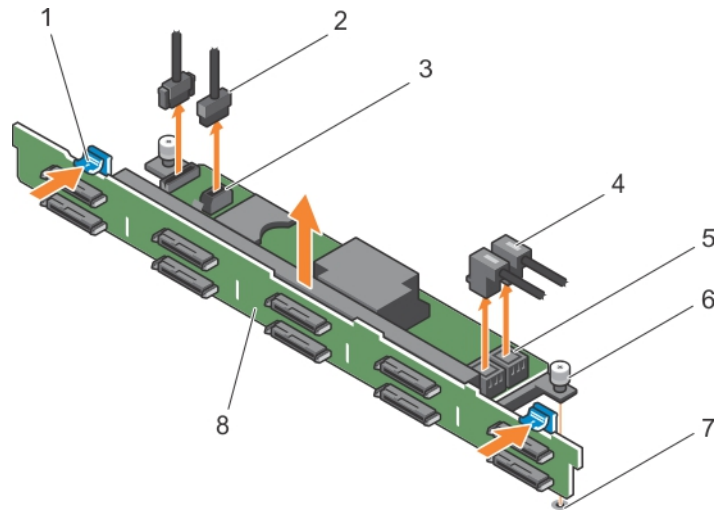
그림 81 . 2.5인치(x10) 하드 드라이브 후면판 분리
