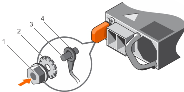
그림 71. 안전 접지 와이어 조립 및 연결
