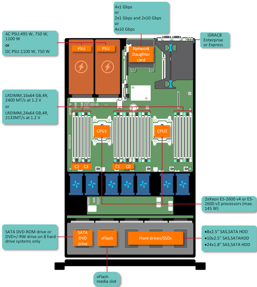
그림 1. PowerEdge R630 시스템이 지원하는 구성
