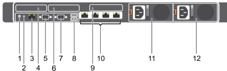
그림 7. 후면 패널 구조(PCle 확장 카드 3개)
