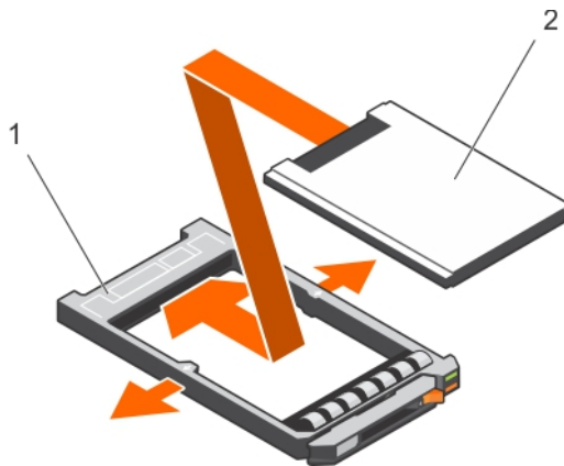
그림 40 . 하드 드라이브 캐리어에 1.8인치 하드 드라이브 설치
