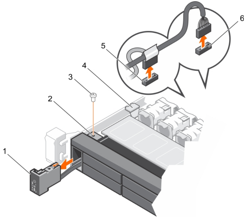
그림 92. 10 하드 드라이브 및 24 하드 드라이브 시스템의 제어판 분리
