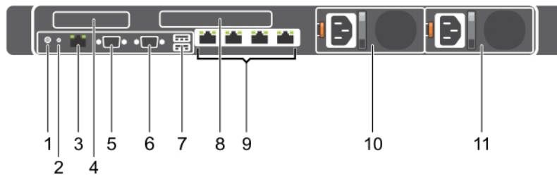
그림 6. 후면 패널 구조(PCle 확장 카드 2개)
