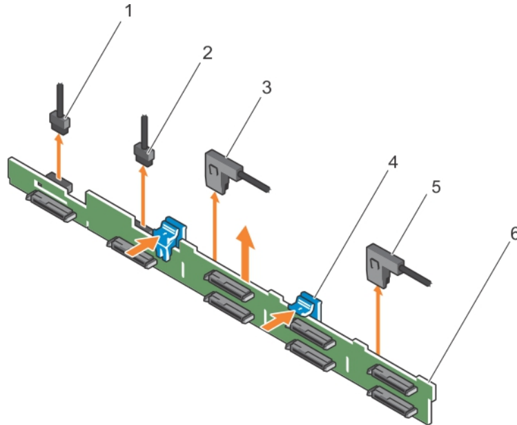
그림 79. 2.5인치(x8) 하드 드라이브 후면판 분리
