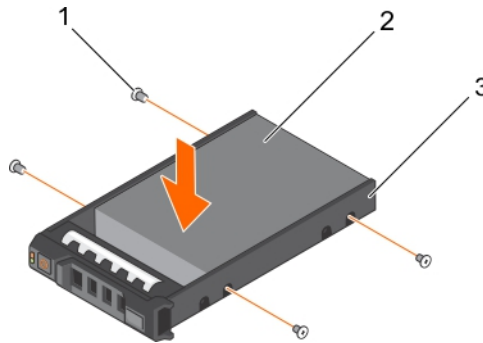
그림 38. 핫 스왑 가능한 하드 드라이브 캐리어에 핫 스왑 가능 하드 드라이브 설치
