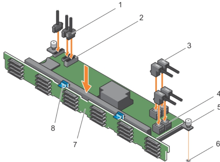
그림 87. 1.8인치(x24) 하드 드라이브 후면판 설치
