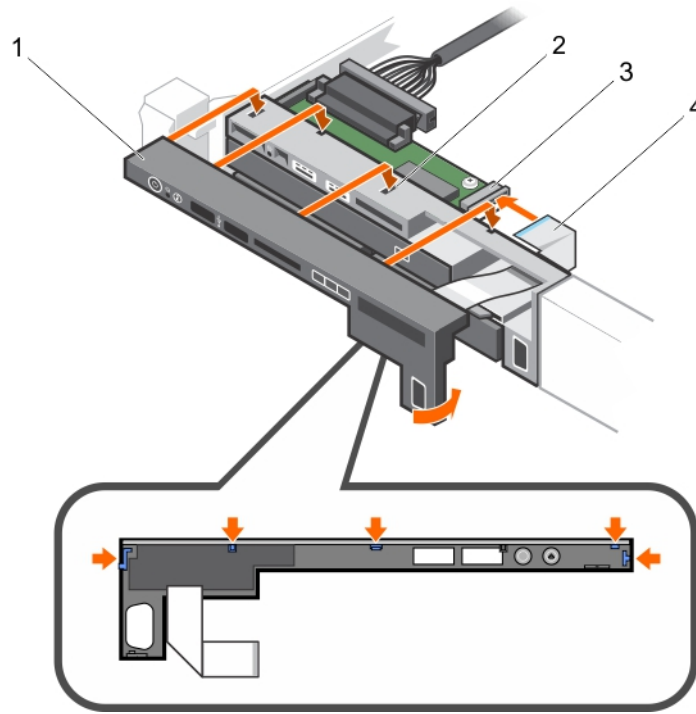
그림 91. 8개 하드 드라이브 시스템의 제어판 설치
