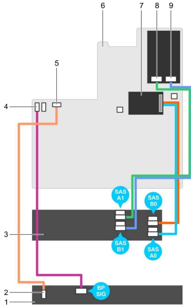
그림 84 . 케이블 연결 다이어그램 - 1.8인치(x24) 하드 드라이브 시스템
