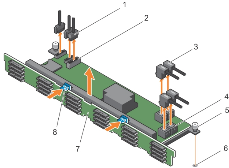
그림 83 . 1.8인치(x24) 하드 드라이브 후면판 분리
