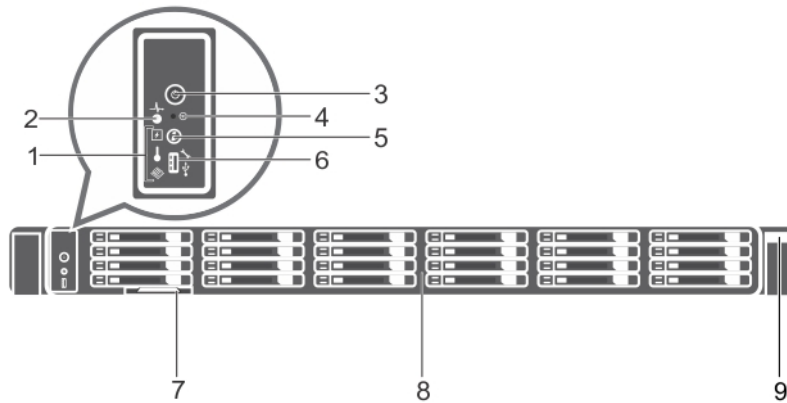
그림 4. 24 x 1.8인치 하드 드라이브 PowerEdge R630 새시의 전면 패널 구조
