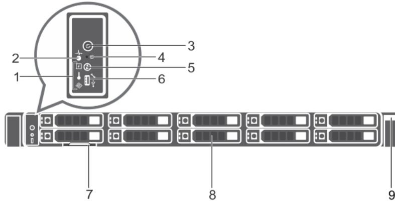
그림 2. 10 x 2.5인치 하드 드라이브 PowerEdge R630 새시의 전면 패널 구조
