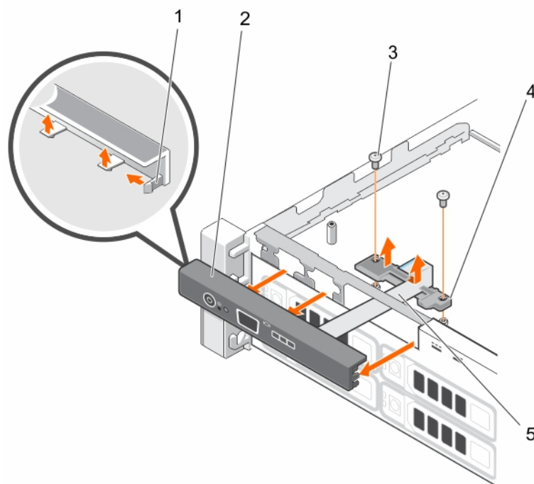
Abbildung 82. Entfernen des Bedienfelds
