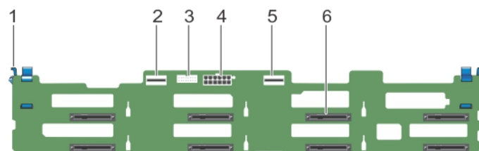
Abbildung 76. Entfernen der Festplatten-Rückwandplatine
