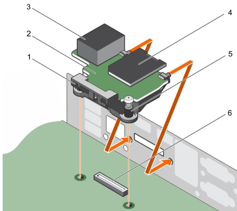
Abbildung 47. Installieren der iDRAC-Port-Karte
