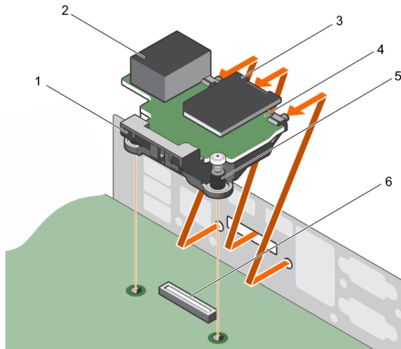
Abbildung 46. Entfernen der iDRAC-Port-Karte
