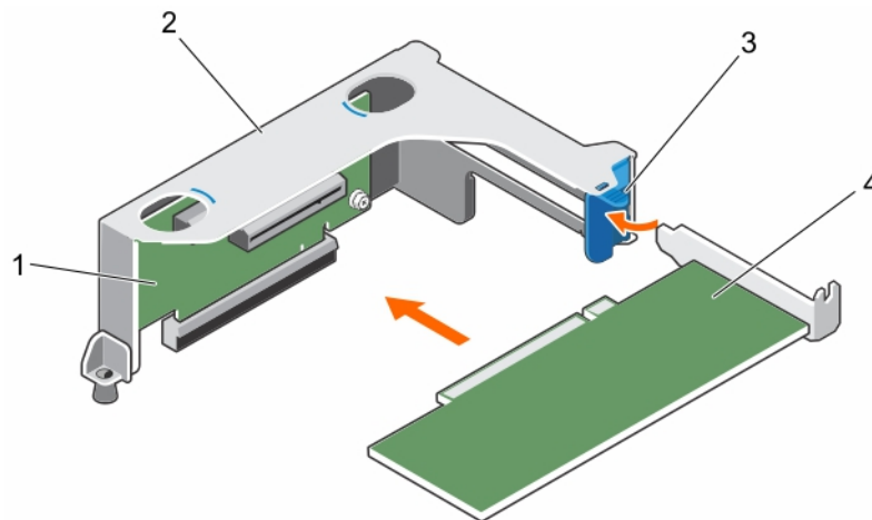
Abbildung 44. Installieren einer Erweiterungskarte in den Erweiterungskarten-Riser
