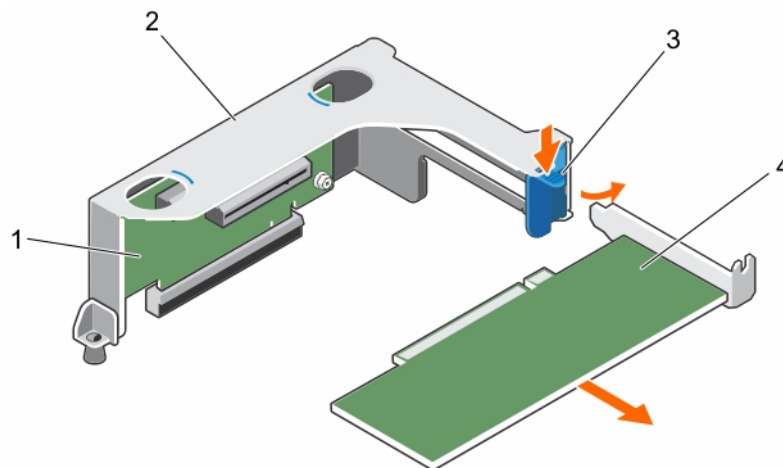
Abbildung 42. Entfernen einer Erweiterungskarte aus dem Erweiterungskarten-Riser
