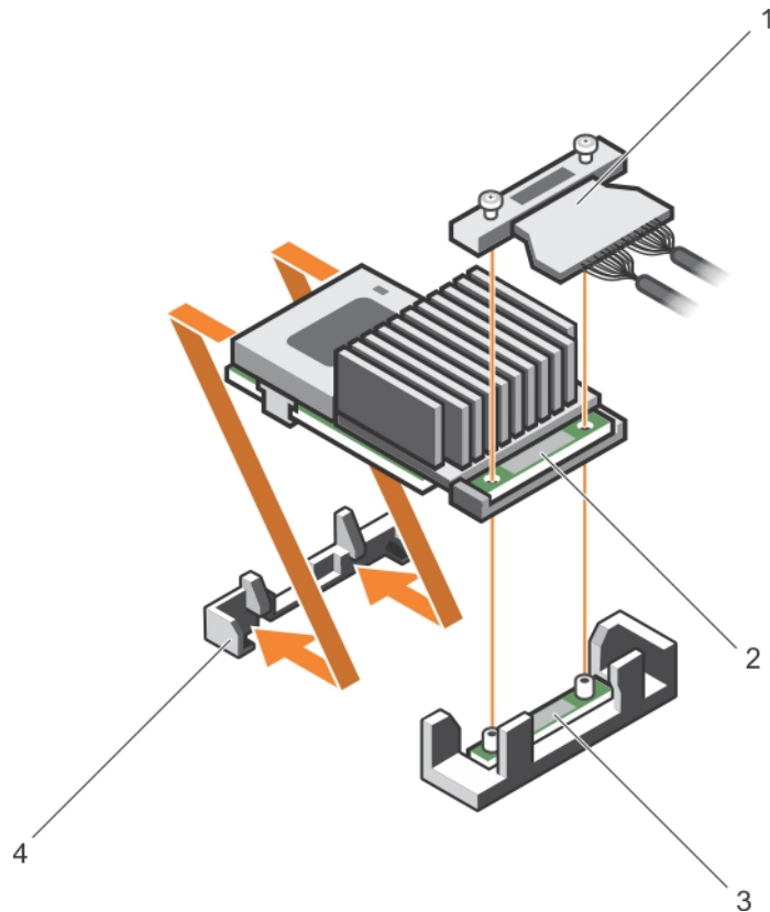
Abbildung 54. Installieren der integrierten Speichercontrollerkarte
