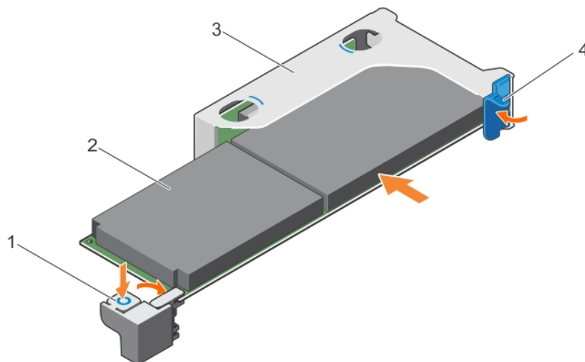
Abbildung 45. Installieren einer Erweiterungskarte voller Bauhöhe und voller Baulänge in den Erweiterungskarten-Riser
