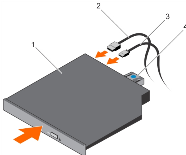
Abbildung 33. Einbauen des optischen Laufwerks
