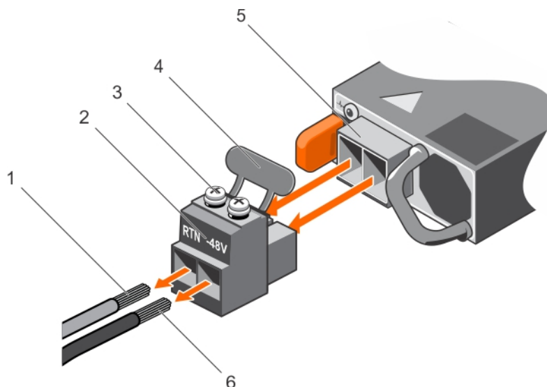
Abbildung 70. Eingangsgleichstromkabel entfernen
