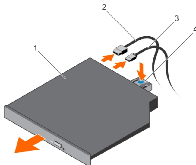
Abbildung 32. Entfernen des optischen Laufwerks
