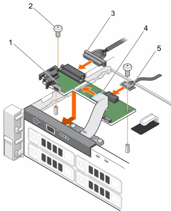
Abbildung 81. Installieren der Bedienfeldplatine
