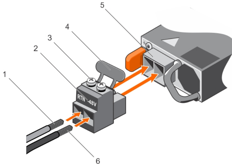
Abbildung 69. Eingangsgleichstromkabel montieren
