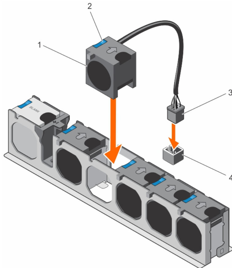
Abbildung 35. Installieren des Kühlungslüfters
