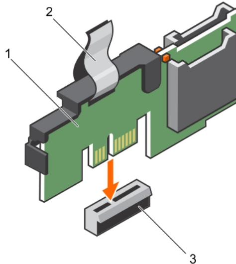
Abbildung 52. Installieren des optionalen internen Dual SD-Moduls
