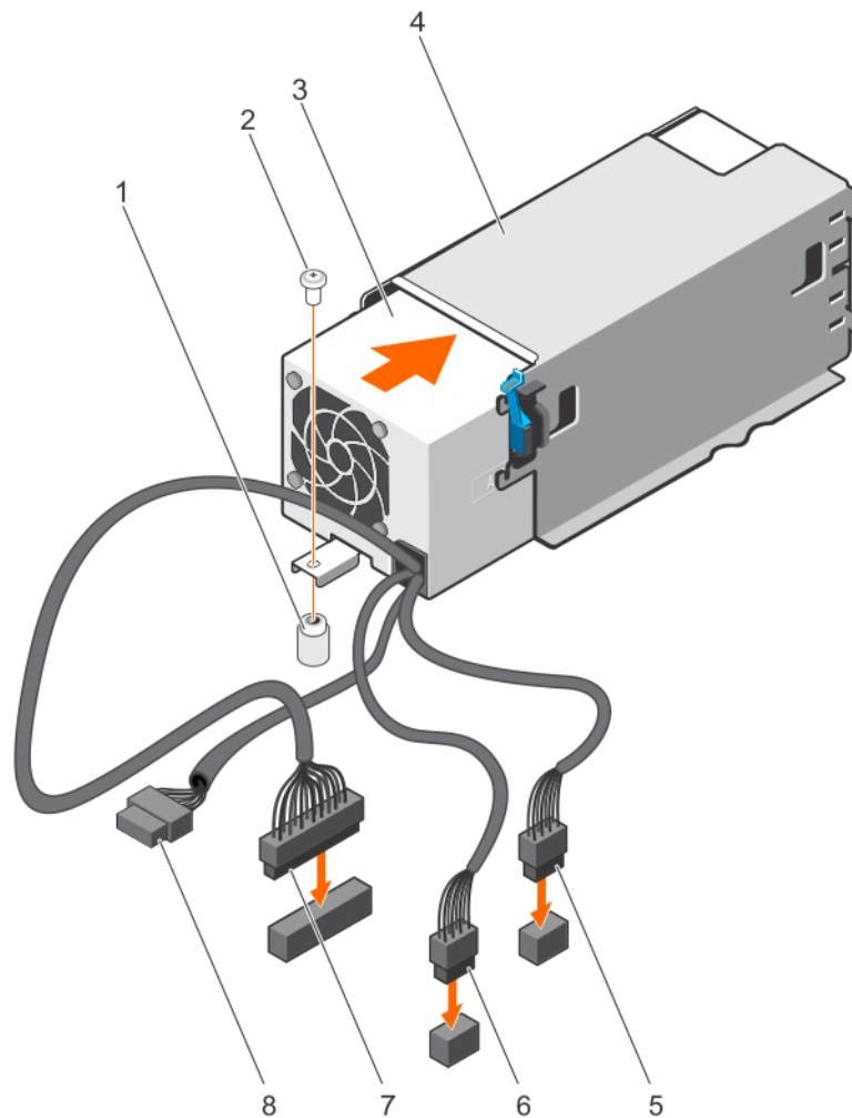
Abbildung 66. Installieren eines nicht redundanten Wechselstrom-Netzteils
