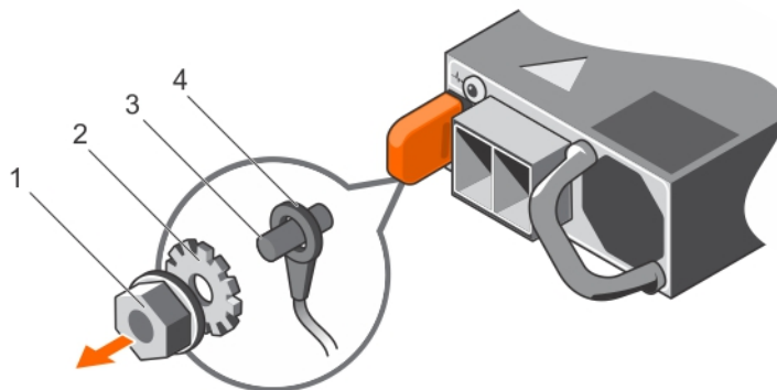
Abbildung 68. Entfernen des Schutzerdungskabels
