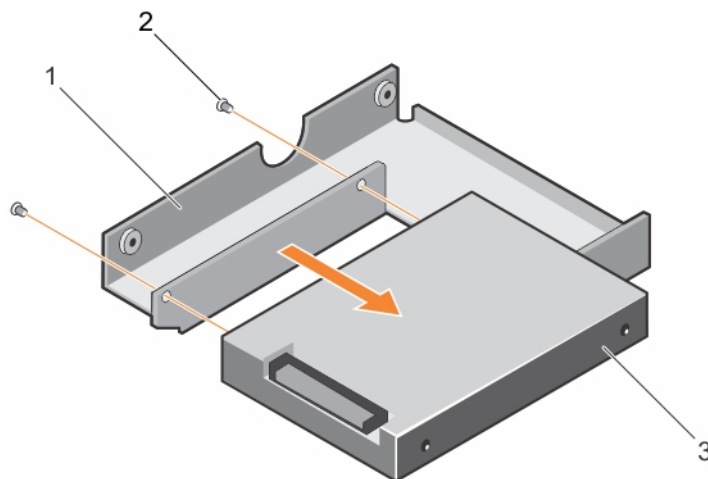
Abbildung 26. Entfernen einer hot-swap-fähigen 2,5-Zoll-Festplatte aus einem 3,5-Zoll-Festplattenadapter
