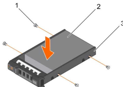
Abbildung 31. Installieren einer Festplatte in einem Laufwerksträger
