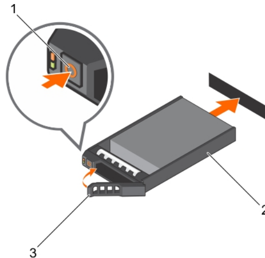
Abbildung 23. Installieren einer hot-swap-fähigen Festplatte oder SSD
