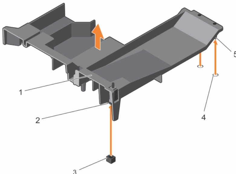
Abbildung 17. Entfernen des Kühlgehäuses
