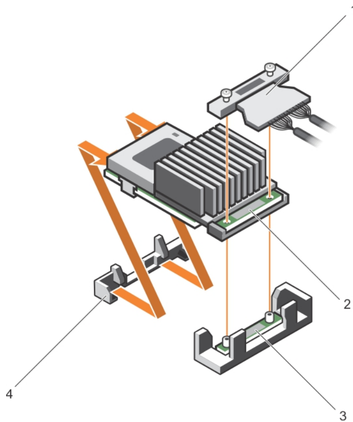
Abbildung 53. Entfernen der integrierten Speichercontrollerkarte
