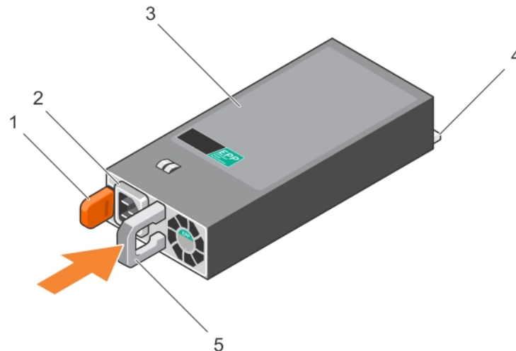
Abbildung 64. Installieren eines Wechselstrom-Netzteils
