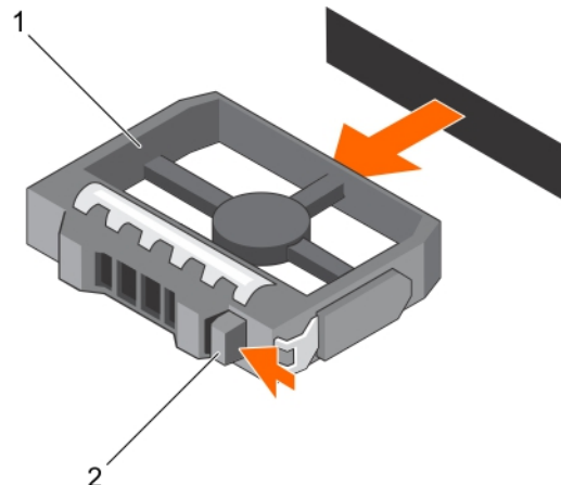
Abbildung 24. Entfernen eines 3,5-Zoll-Festplattenplatzhalters
