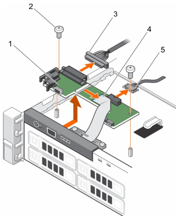
Abbildung 80. Entfernen der Bedienfeldplatine
