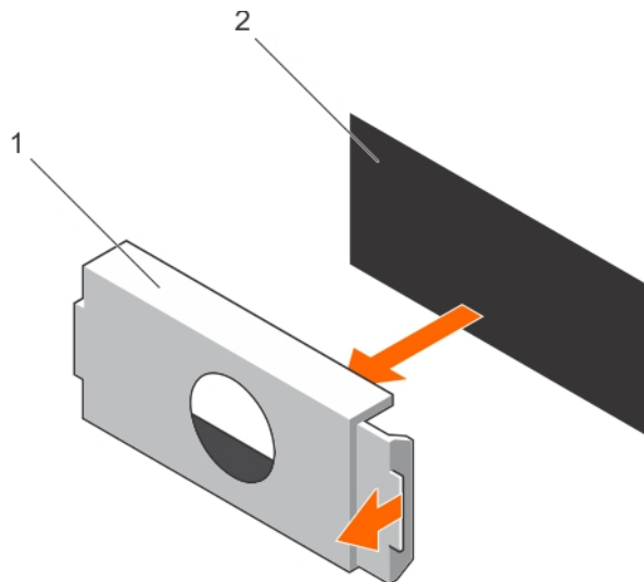
Abbildung 61. Entfernen der Netzteilplatzhalterkarte
