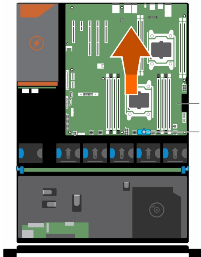
Abbildung 86. Einsetzen der Systemplatine
