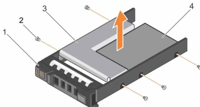
Abbildung 28. Entfernen eines hot-swap-fähigen 3,5-Zoll-Laufwerksadapters aus einem hot-swap-fähigen 3,5-Zoll-Laufwerksträger
