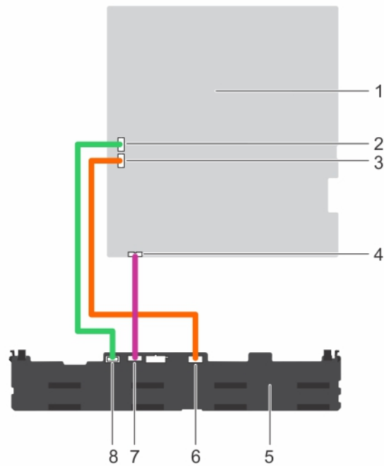
Abbildung 77. Verkabelungsdiagramm der Festplattenrückwandplatine unter Verwendung des integrierten Controllers
