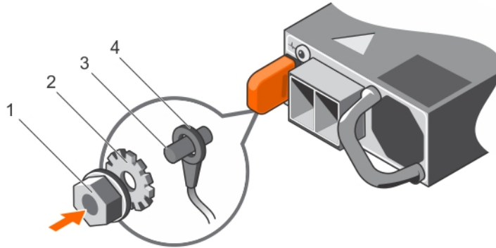
Abbildung 67. Montieren und Anschließen des Schutzerdungskabels
