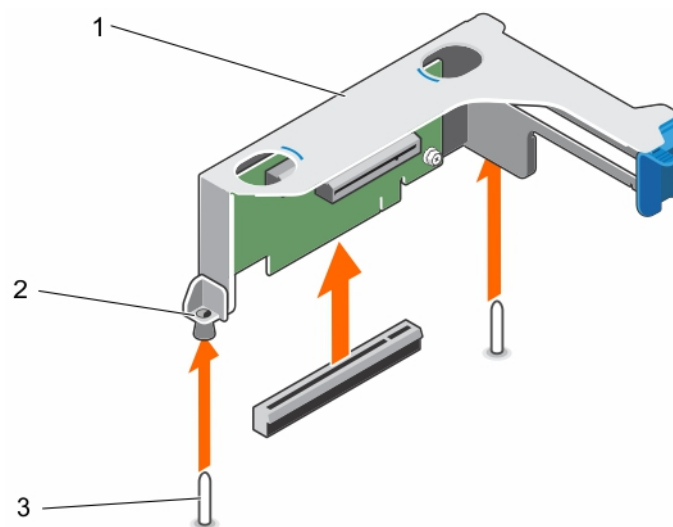
Abbildung 40. Entfernen des Erweiterungskarten-Risers
