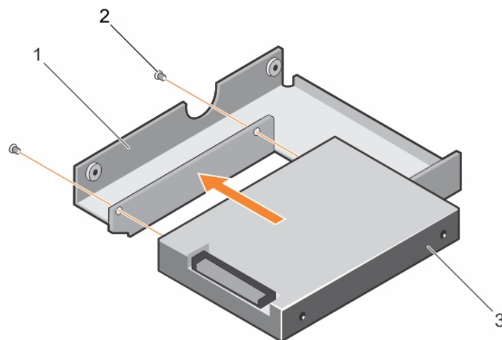
Abbildung 27. Installieren eines Hot-Swap-fähigen 2,5-Zoll-Festplattenlaufwerks in einem 3,5-Zoll-Festplattenadapter
