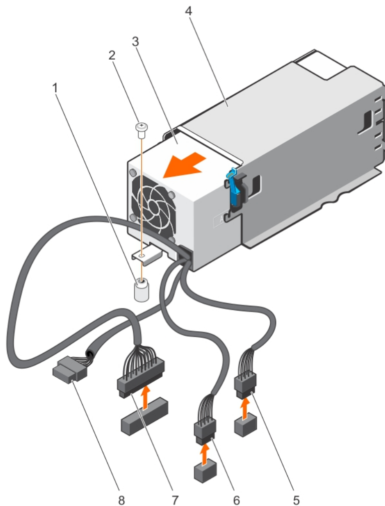
Abbildung 65. Entfernen eines nicht redundanten Wechselstrom-Netzteils (verkabelt)
