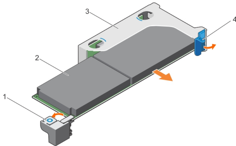
Abbildung 43. Entfernen einer Erweiterungskarte voller Bauhöhe und voller Baulänge aus dem Erweiterungskarten-Riser
