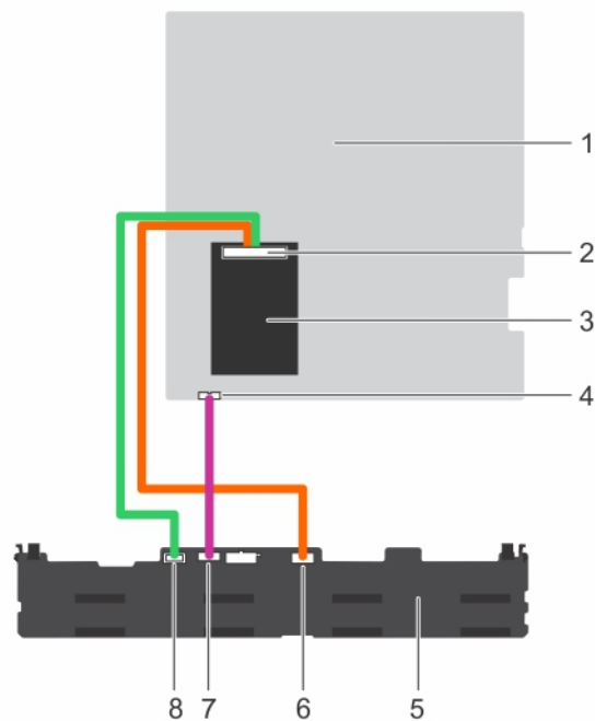
Abbildung 78. Verkabelungsdiagramm der Festplattenrückwandplatine unter Verwendung des integrierten Speichercontrollers
