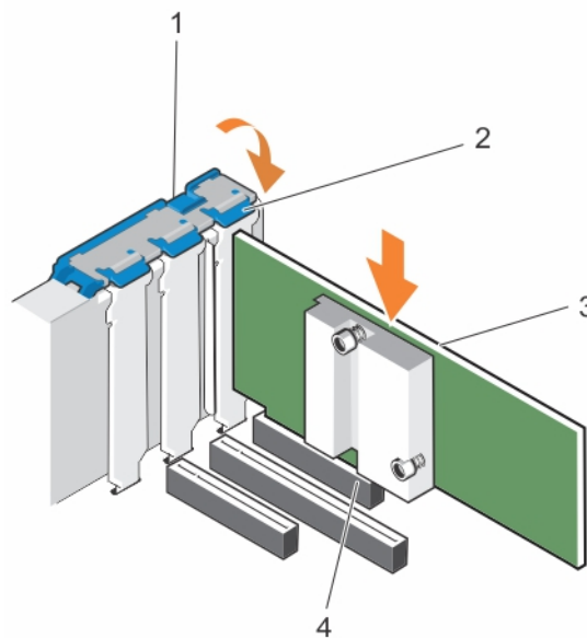
Abbildung 39. Installieren einer Erweiterungskarte
