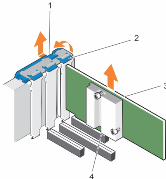
Abbildung 38. Entfernen einer Erweiterungskarte von der Systemplatine
