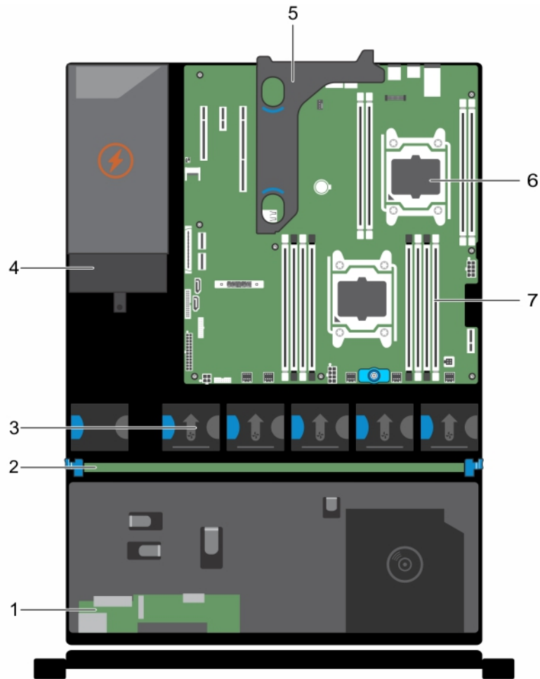
Abbildung 16. Das Innere des Systems – Gehäuse eines nicht redundanten Netzteils
