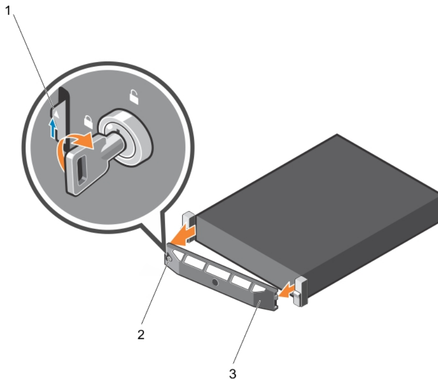
Abbildung 11. Entfernen der optionalen Frontverkleidung (Blende)
