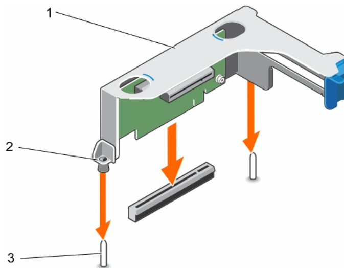
Abbildung 41. Installieren des (optionalen) Erweiterungskarten-Risers
