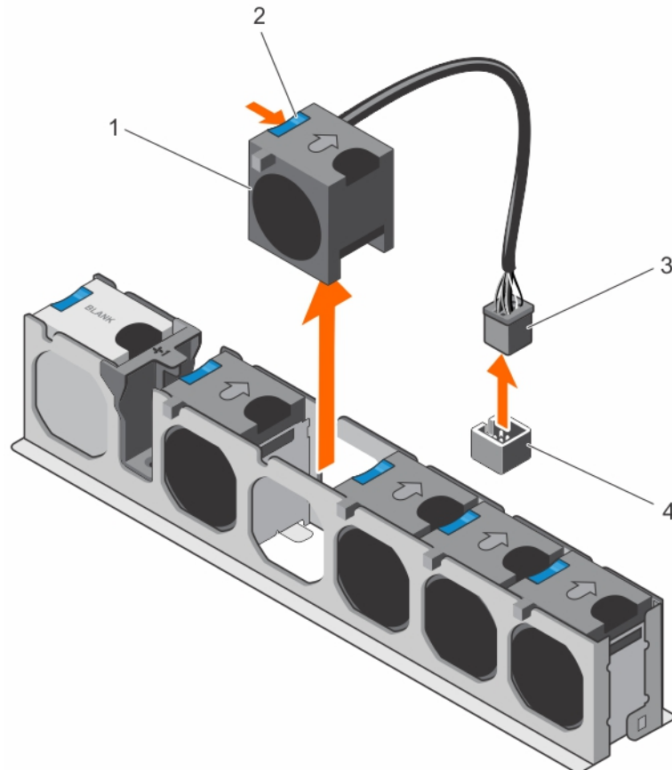
Abbildung 34. Entfernen eines Kühlungsüfters
