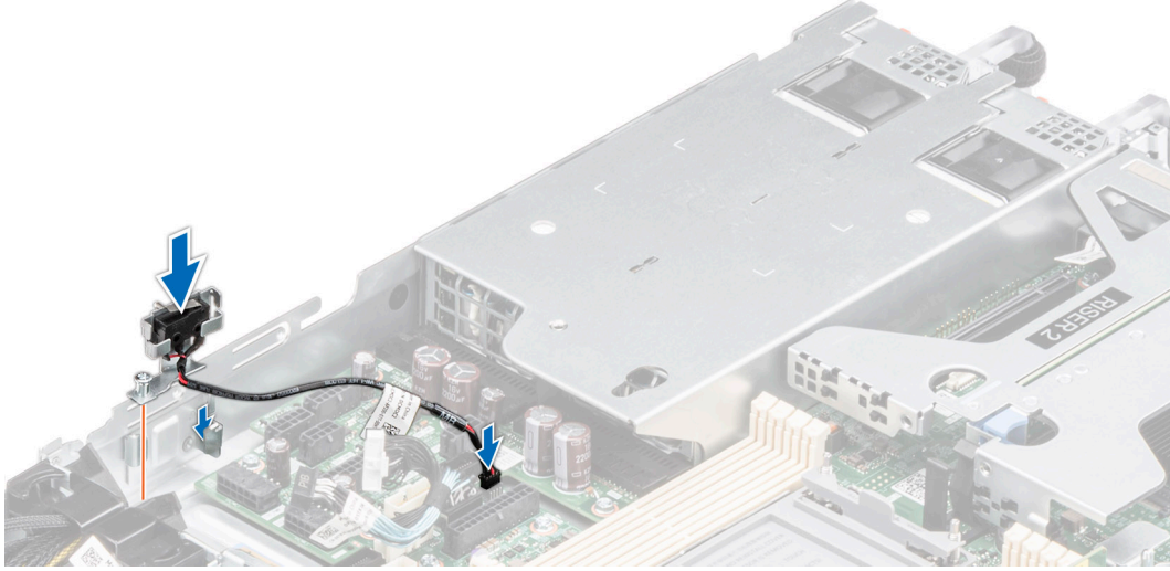
Rakam 26. İzinsiz girişi önleme anahtarını takma
