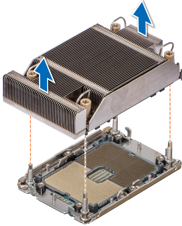
Rakam 46. İşlemciyi ve ısı emici modülünü çıkarma
