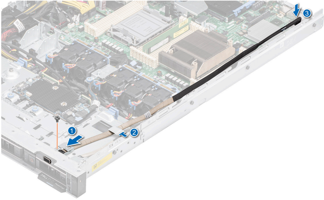
Rakam 93. VGA modülünü takma
