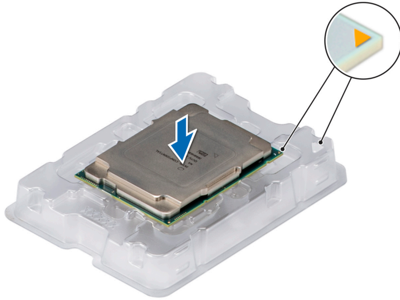
Rakam 48. İşlemcinin pim 1 işaretlerini tepsi ile hizalama
