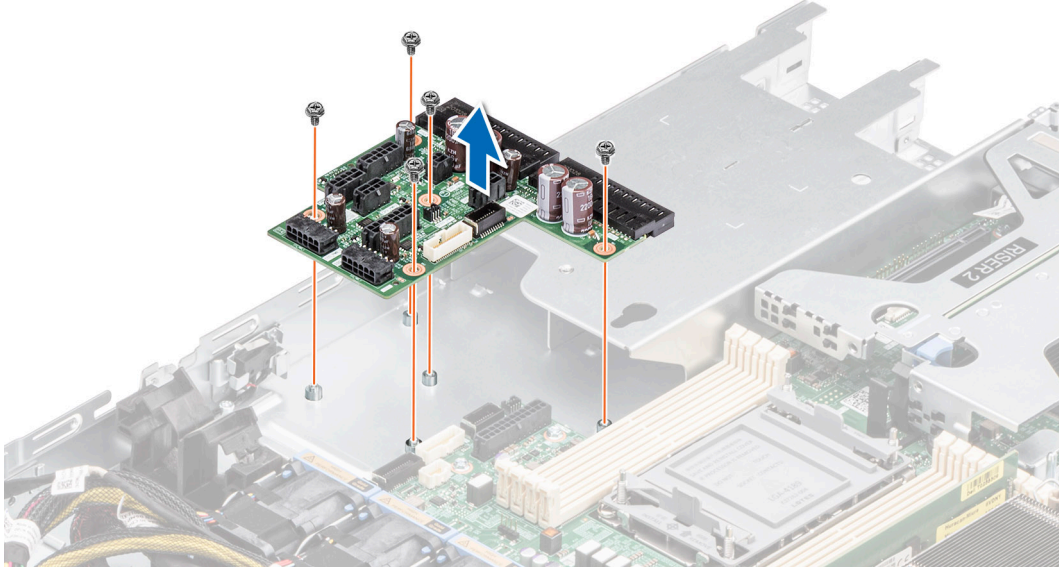
Rakam 98. Güç aracı kartını çıkarma
