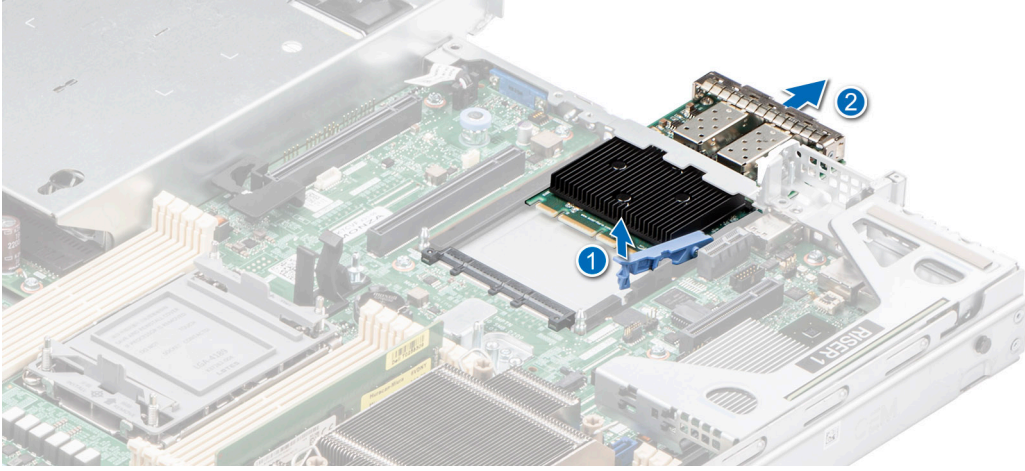
Rakam 82. OCP kartını çıkarma
