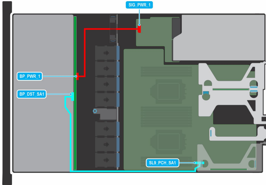
Rakam 41. Kablo yerleşimi - ODD, Kelebek yükselticisi, BOSS ve SNAPI yükselticisi ile 4 x 3,5 inç sürücü SATA arka paneli
