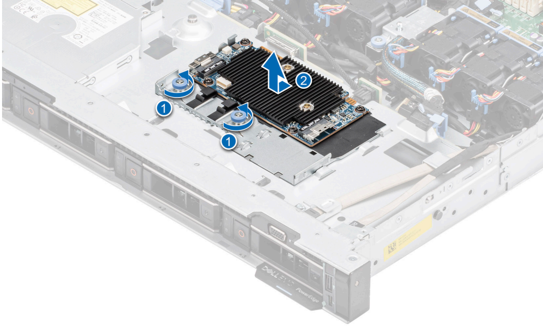
Rakam 84. 4x3,5 inç sistemi için ön montaj ön PERC modülünü çıkarma
