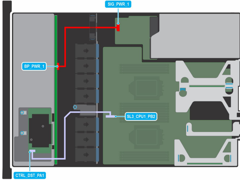
Rakam 39. Kablo yerleşimi - Kelebek yükselticisi, BOSS ve SNAPİ yükselticisi ile 8 x 2,5 inç sürücü SAS veya SATA arka paneli
