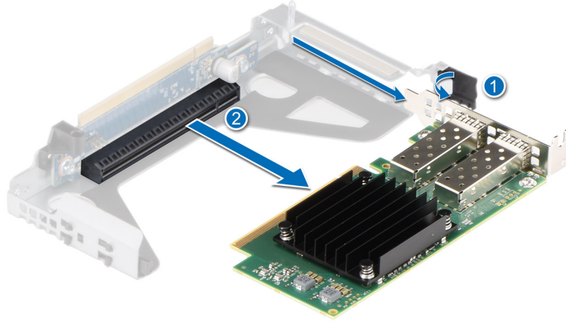
Rakam 64. Genişletme kartını Yükseltici 1'den çıkarma
