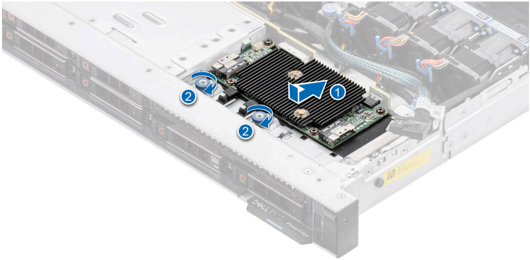
Rakam 87. 8x2,5 inç sistemi için ön montaj ön PERC modülünü takma
