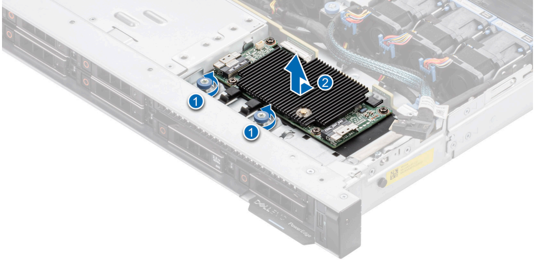
Rakam 85. 8x2,5 inç sistemi için ön montaj ön PERC modülünü çıkarma
