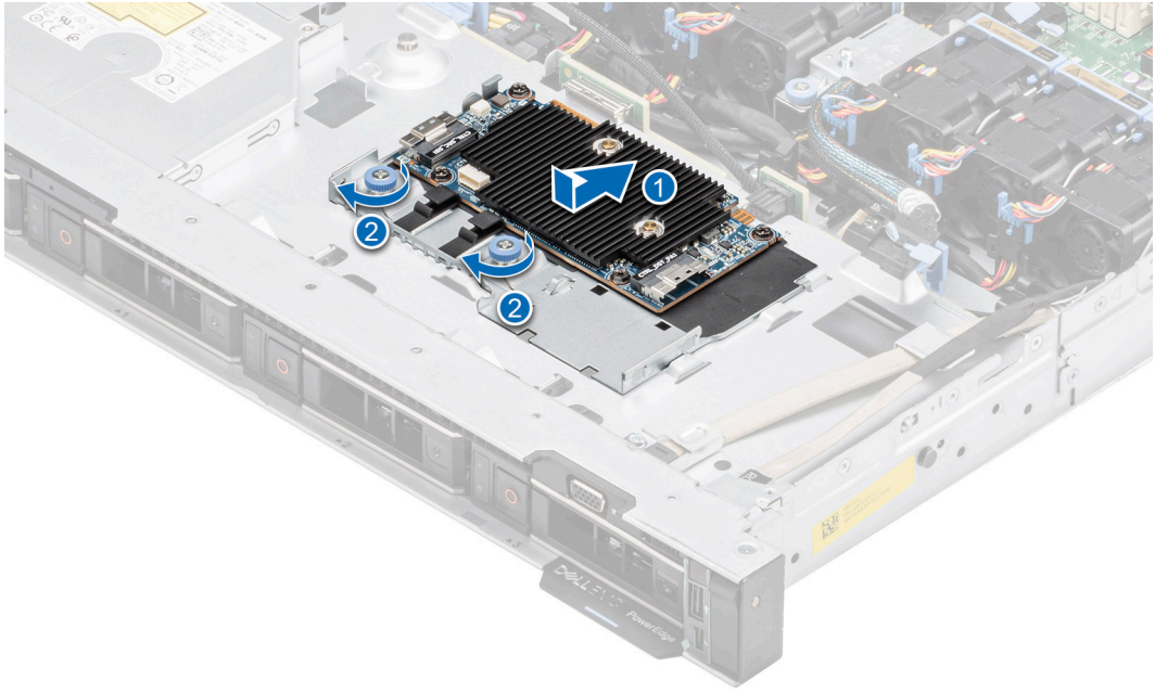
Rakam 86. 4x3,5 inç sistemi için ön montaj ön PERC modülünü takma
