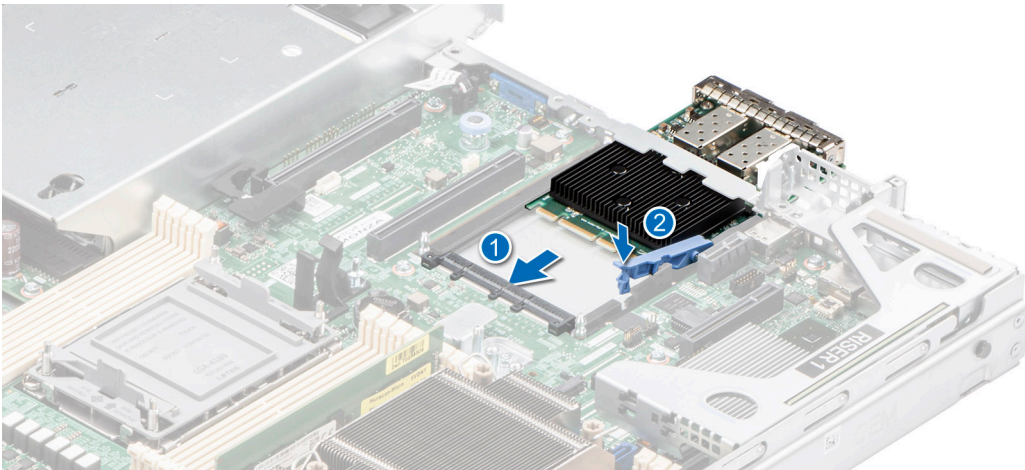
Rakam 83. OCP kartını takma
