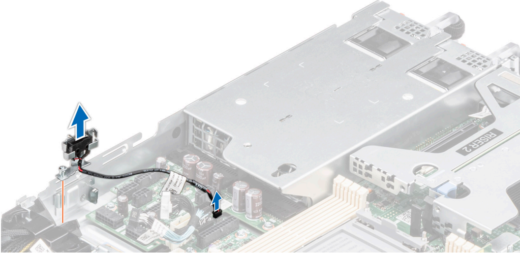
Rakam 25. İzinsiz giriş önleme anahtarı modülünü çıkarma
