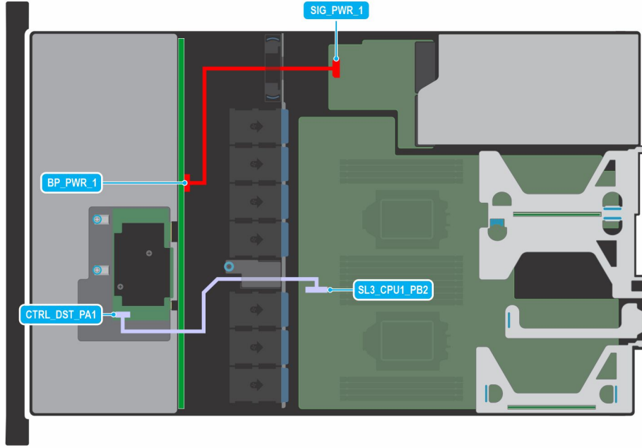
Rakam 40. Kablo yerleşimi - ODD, Kelebek yükselticisi, BOSS ve SNAPI yükselticisi ile 4 x 3,5 inç sürücü SAS veya SATA arka paneli
