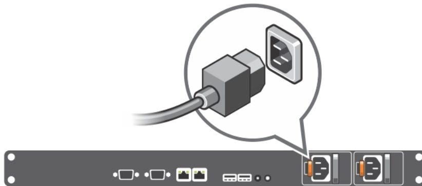
그림 3. 전원 케이블 연결
