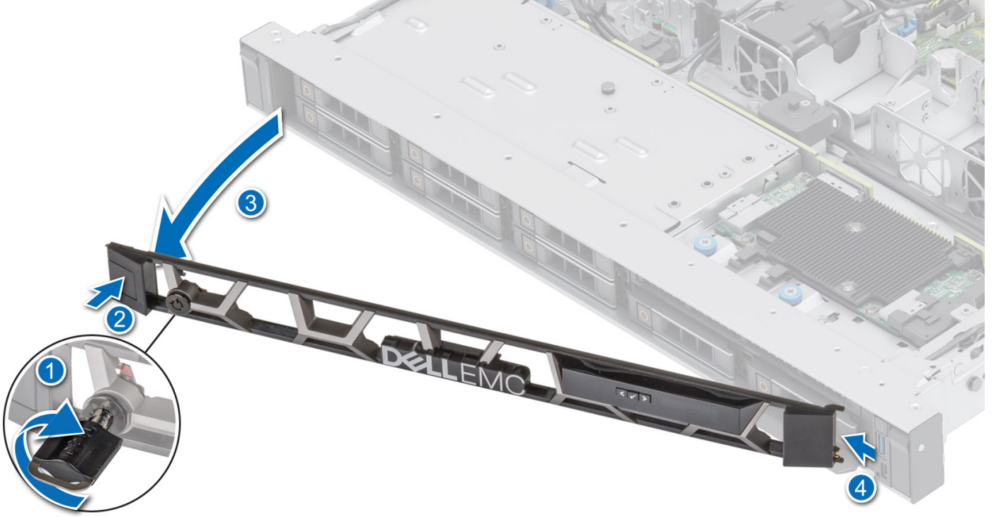
Rakam 9. LCD panelli ön çerçeveyi çıkarma
