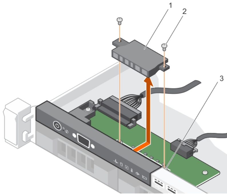
그림 100 . LED 모듈 설치 - 4개의 케이블 연결된 하드 드라이브 새시
