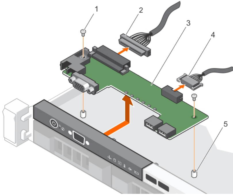
그림 99. LED 컨트롤 패널 보드 제거 - 4개의 케이블 연결된 하드 드라이브 새시
