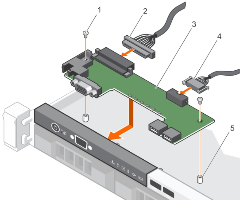
그림 101 . LED 컨트롤 패널 보드 설치 - 4개의 케이블 연결된 하드 드라이브 새시
