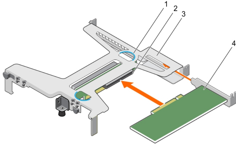
그림 58 . 확장 카드 라이저에 확장 카드 설치
