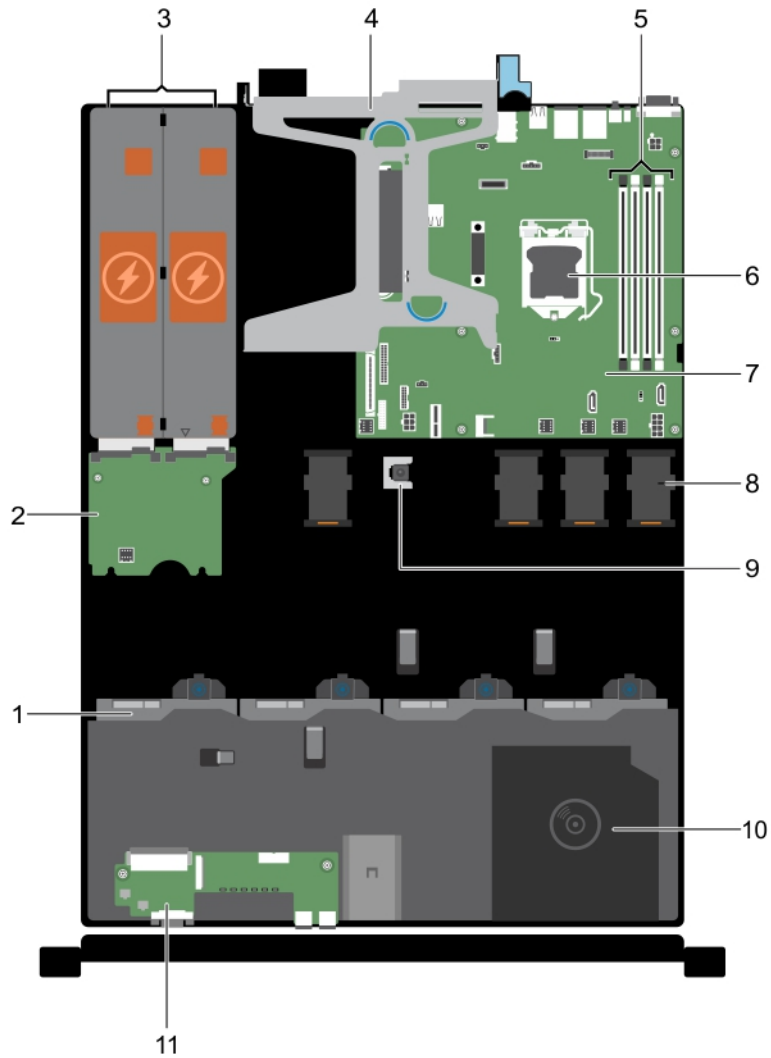
그림 18. 시스템 내부 - 4개의 3.5인치 케이블 연결 하드 드라이브 장착
