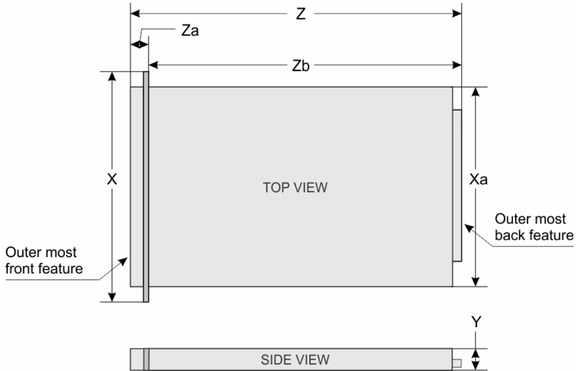
그림 11. PowerEdge R330 시스템의 새시 크기
