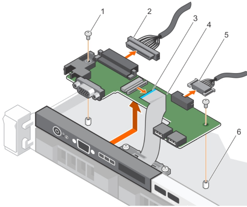
그림 95 . LCD 컨트롤 패널 보드 제거 - 4개의 하드 드라이브 새시
