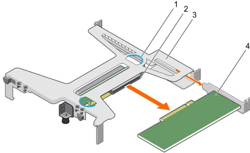
그림 57. 확장 카드 라이저에서 확장 카드 제거
