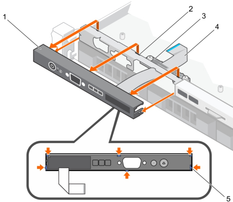
그림 94 . LCD 컨트롤 패널 제거 - 4개의 8.89cm(3.5인치) 핫 스왑 가능 하드 드라이브 새시
