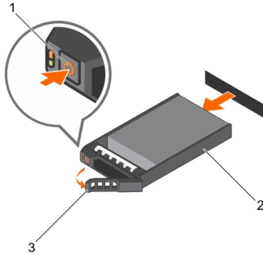
그림 34. 핫 스왑 가능한 하드 드라이브 또는 SSD 분리
