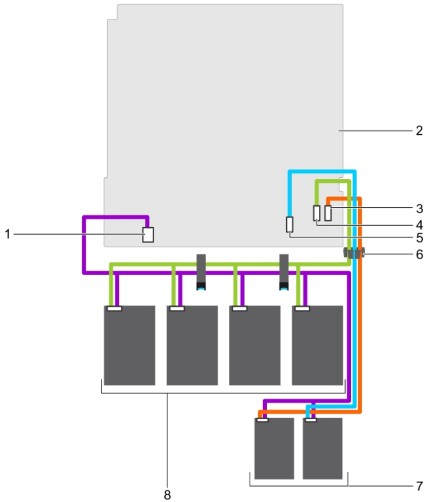
그림 90 . 케이블 연결 다이어그램- 케이블로 연결된 4개의 3.5인치 하드 드라이브 및 2개의 1.8인치 SSD
