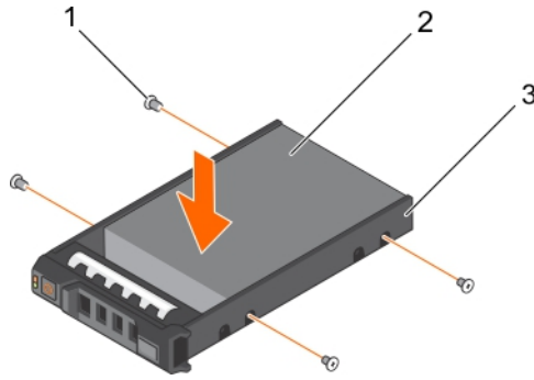
그림 45. 핫 스왑 가능한 하드 드라이브 캐리어에 핫 스왑 가능 하드 드라이브 설치
