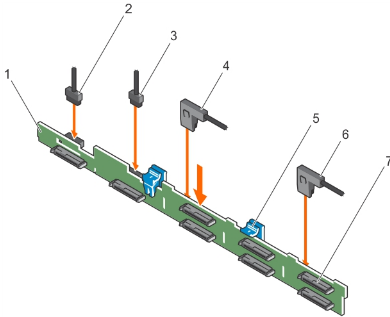
그림 93 . 8개의 2.5인치 SAS/SATA 후면판 설치
