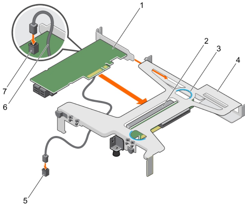
그림 59 . 확장 카드 라이저에 확장 카드 설치
