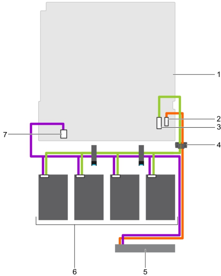
그림 88 . 케이블 연결 다이어그램- 케이블로 연결된 4개의 3.5인치 하드 드라이브
