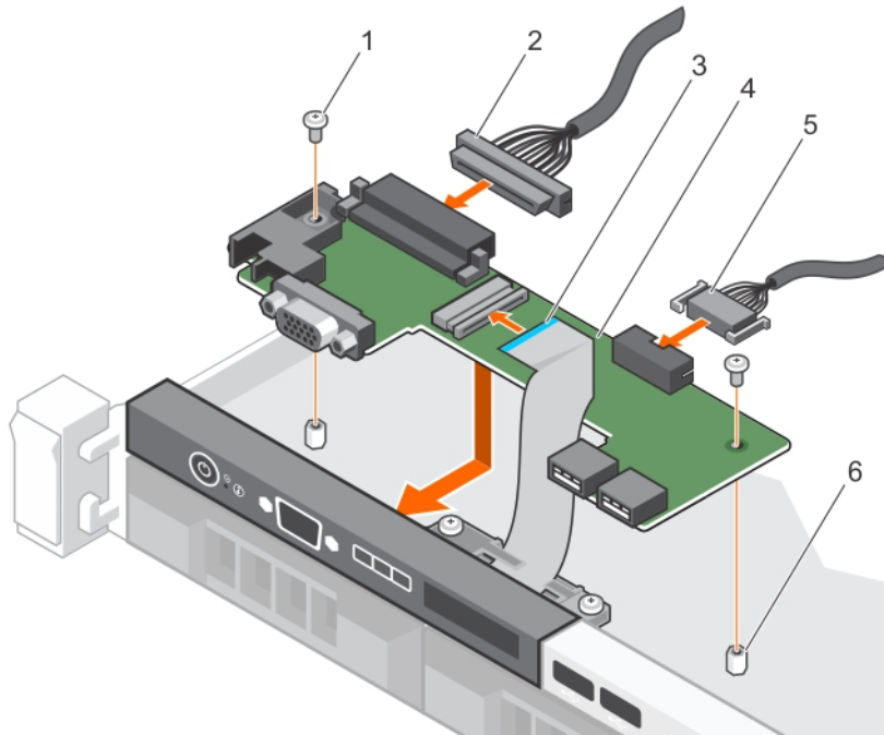
그림 97 . LCD 컨트롤 패널 보드 설치 - 4개의 하드 드라이브 새시
