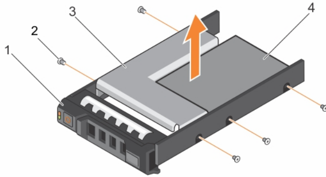
그림 42. 하드 드라이브 캐리어에서 3.5인치 하드 드라이브 어댑터 분리
