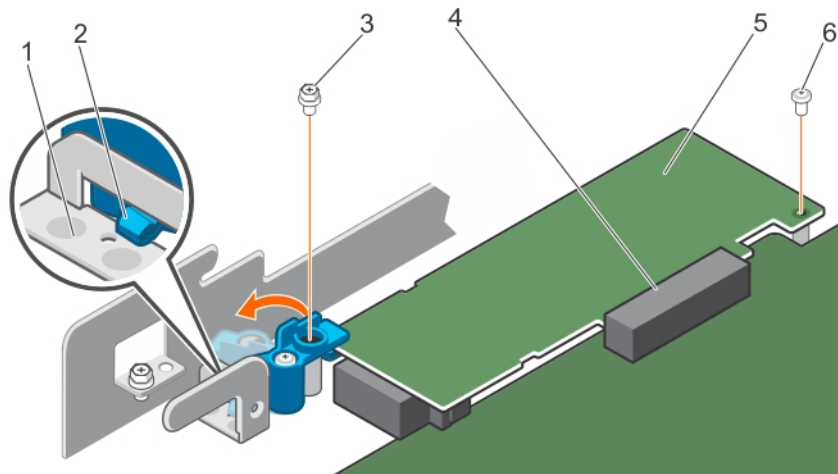
그림 60 . PERC 카드 잠금 장치 열기
