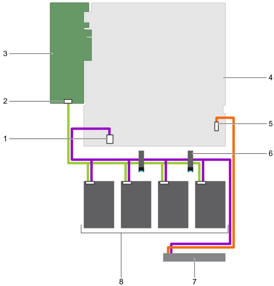
그림 89 . 케이블 연결 다이어그램- 케이블로 연결된 4개의 3.5인치 하드 드라이브 및 PERC 카드
