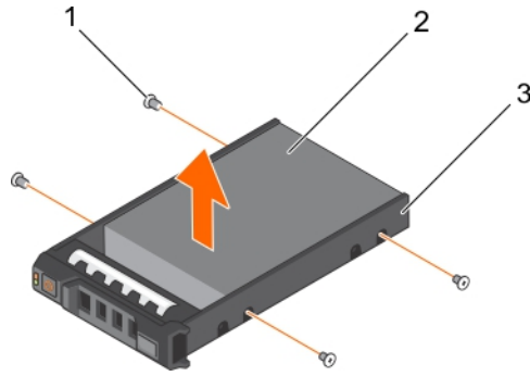
그림 44. 하드 드라이브 캐리어에서 핫 스왑 가능한 하드 드라이브 분리
