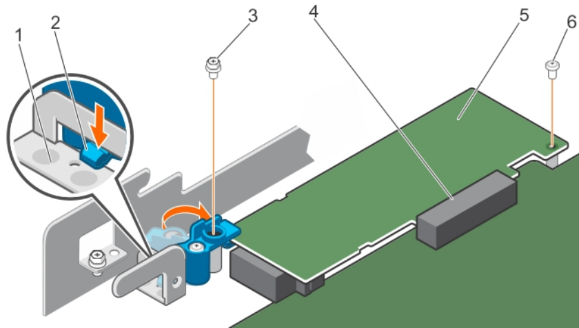
그림 63. PERC 카드 잠금 장치 닫기
