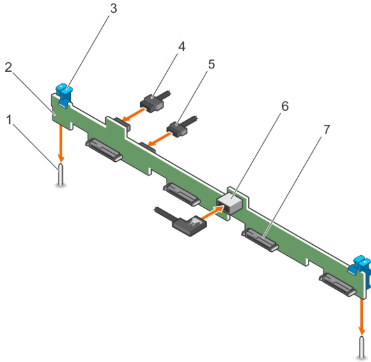
그림 92. 4개의 3.5인치 하드 드라이브 SAS/SATA 후면판 설치
