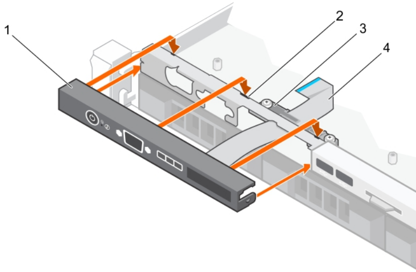
그림 96 . LCD 컨트롤 패널 설치 - 4개의 8.89cm(3.5인치) 핫 스왑 가능 하드 드라이브 새시
