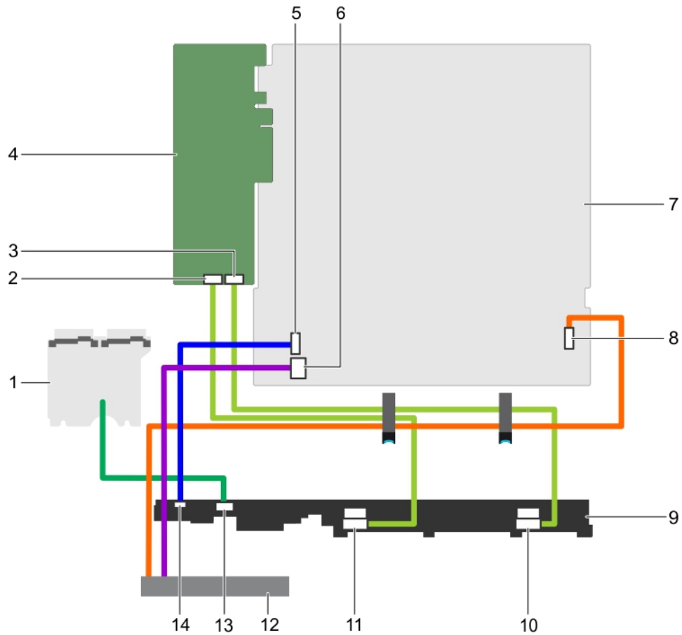
그림 87. 케이블 연결 다이어그램- PERC 카드와 8개의 2.5인치 SAS/SATA 후면판
