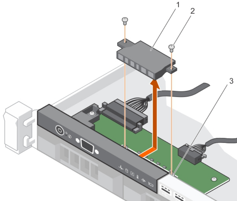
그림 98 . LED 모듈 제거 - 4개의 케이블 연결된 하드 드라이브 샤페
