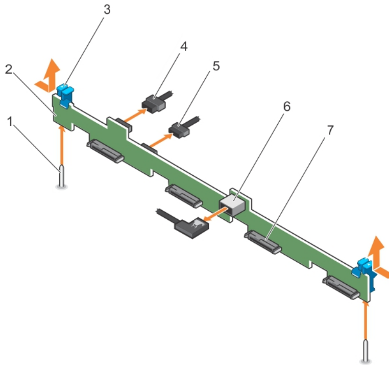
그림 84 . 4개의 8.89cm(3.5인치) 또는 4개의 6.35cm(2.5인치) 하드 드라이브 SAS/SATA 백플레인 제거
