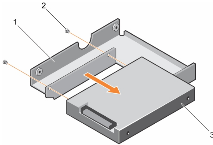
그림 40. 3.5인치 하드 드라이브 어댑터에서 2.5인치 하드 드라이브 분리
