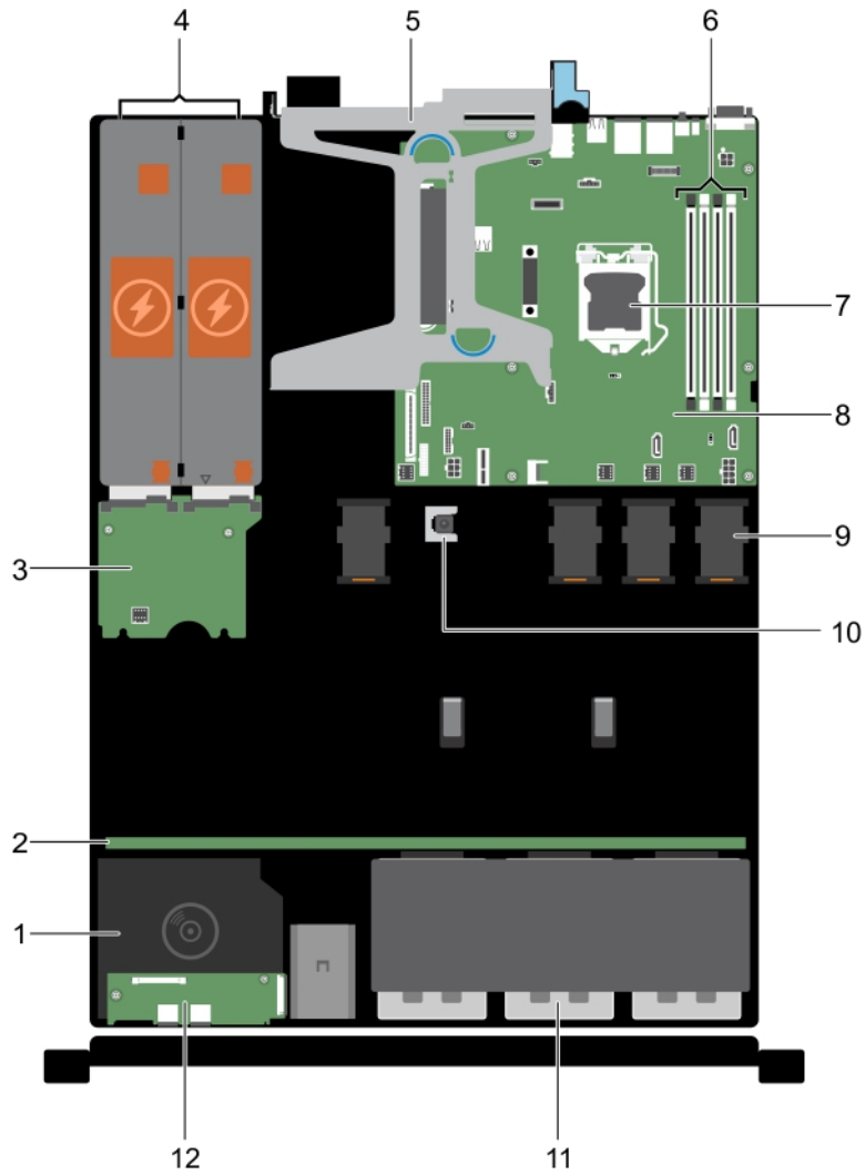
그림 17. 시스템 내부 - 8개의 2.5인치 하드 드라이브 장착
