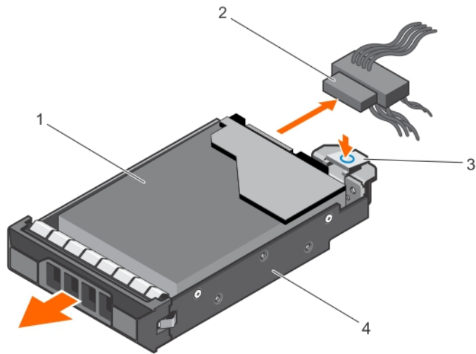
그림 30. 케이블 연결된 하드 드라이브 캐리어 분리
