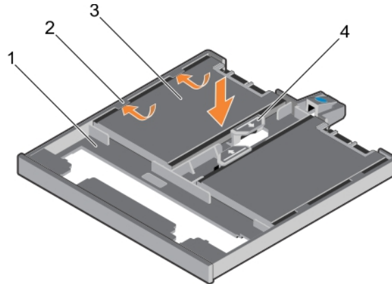
그림 38 . SSD 트레이에 4.57cm(1.8인치) 솔리드 스테이트 드라이브 설치
