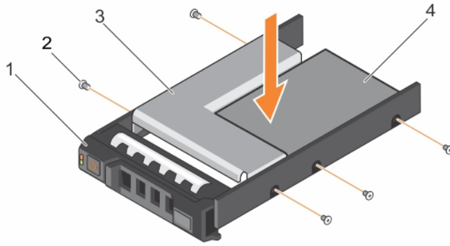
그림 43. 핫 스왑 가능한 하드 드라이브 캐리어에 3.5인치 하드 드라이브 어댑터 설치
