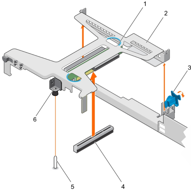
그림 55. 확장 카드 라이저 분리 및 설치
