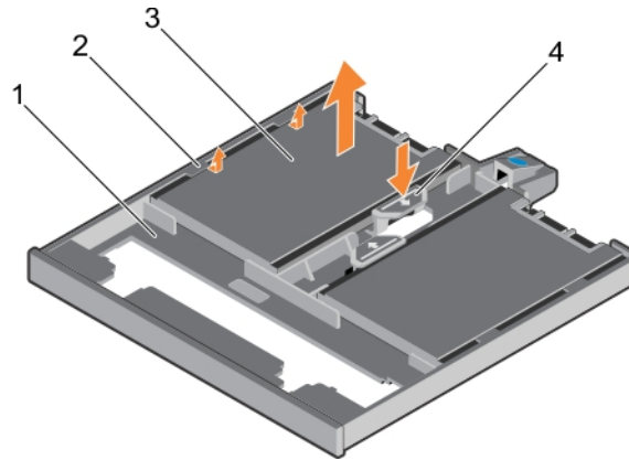
그림 37 . SSD 트레이에서 4.57cm(1.8인치) 솔리드 스테이트 드라이브 제거
