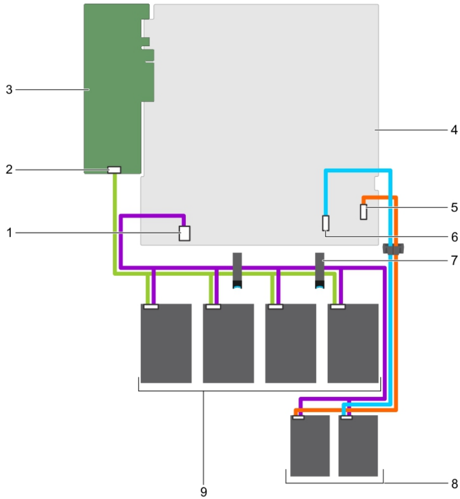
그림 91. 케이블 연결 다이어그램- 케이블로 연결된 4개의 3.5인치 하드 드라이브, 2개의 1.8인치 SSD 및 PERC 카드
