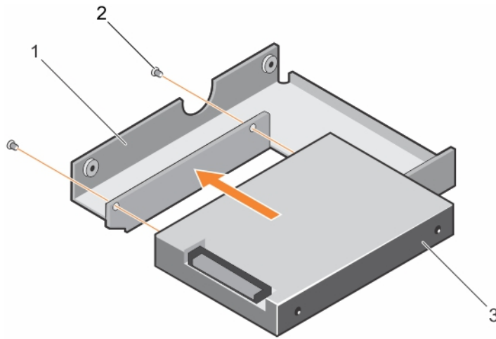
그림 41. 3.5인치 하드 드라이브 어댑터에 2.5인치 핫 스왑 가능한 하드 드라이브 설치
