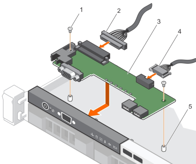
図 101. LED コントロール パネル ボードの取り付け—4 台のケーブル接続式ハードドライブ シャーシ
