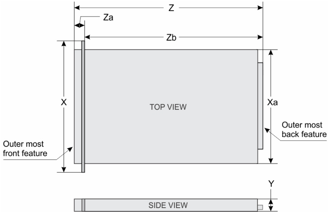
図 11. PowerEdge R330 システムのシャーシ寸法
