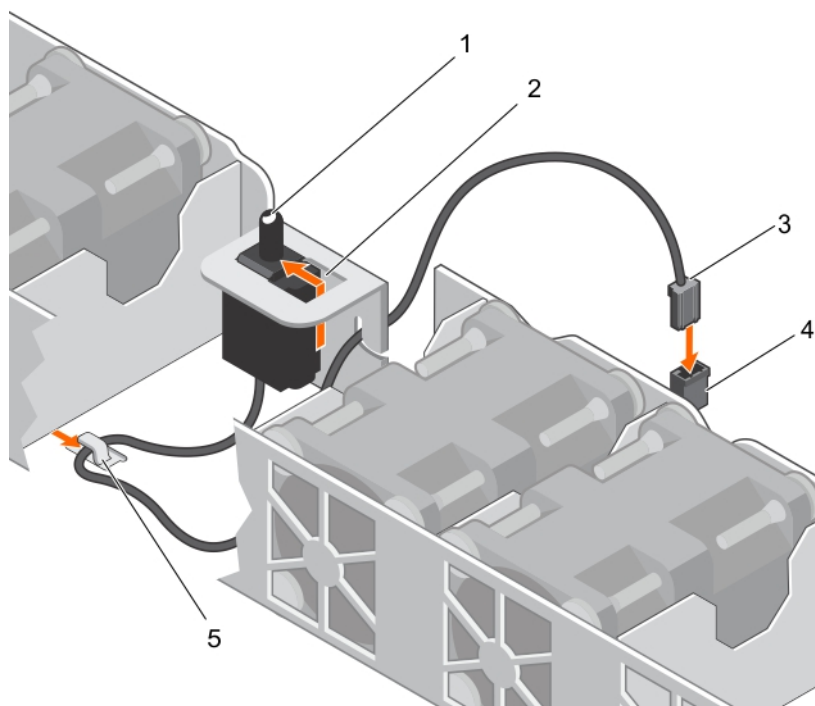
図 20. インタージョンスイッチの取り付け
