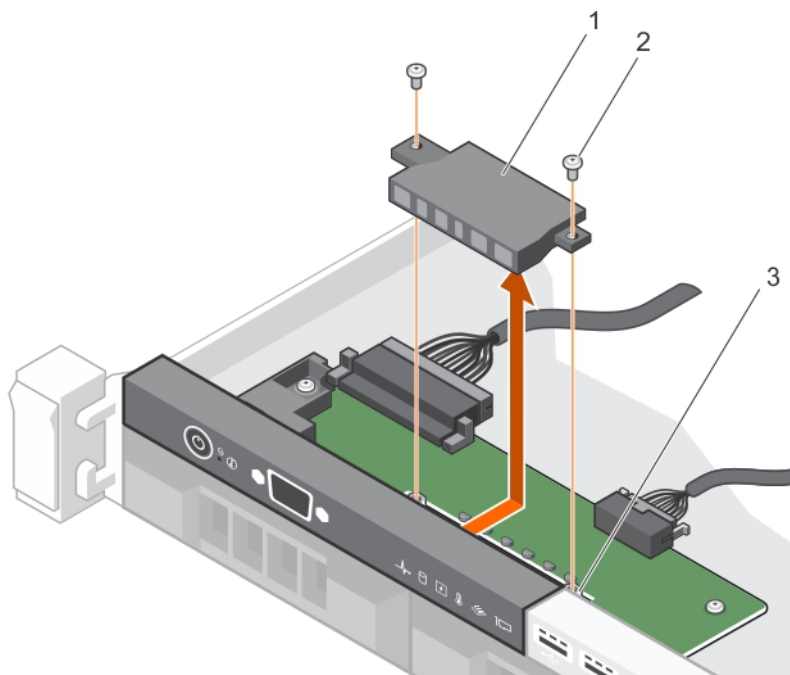
図 98. LED モジュールの取り外し—4 台のケーブル接続式ハードドライブ シャーシ
