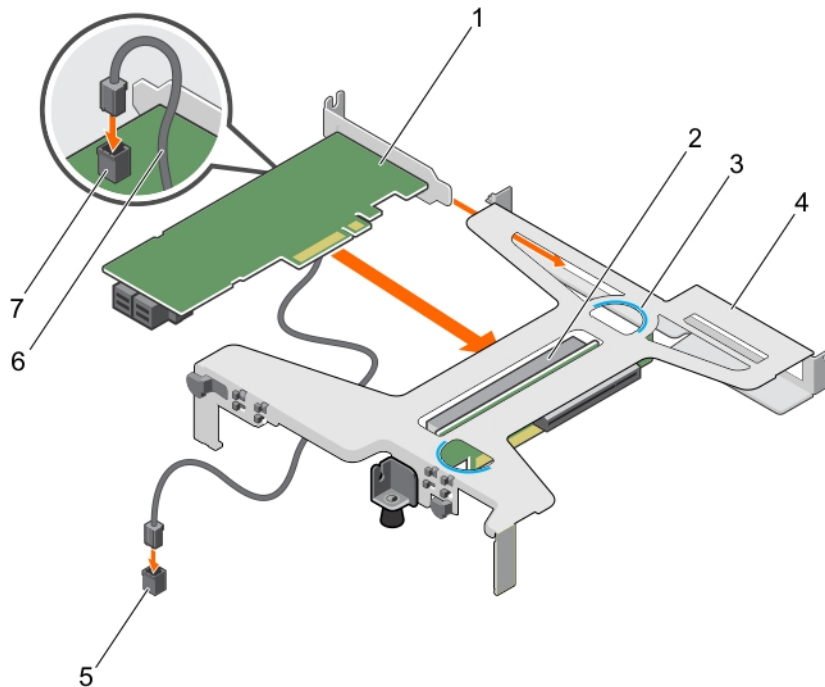
図 59. 拡張カードライザーへの拡張カードの取り付け
