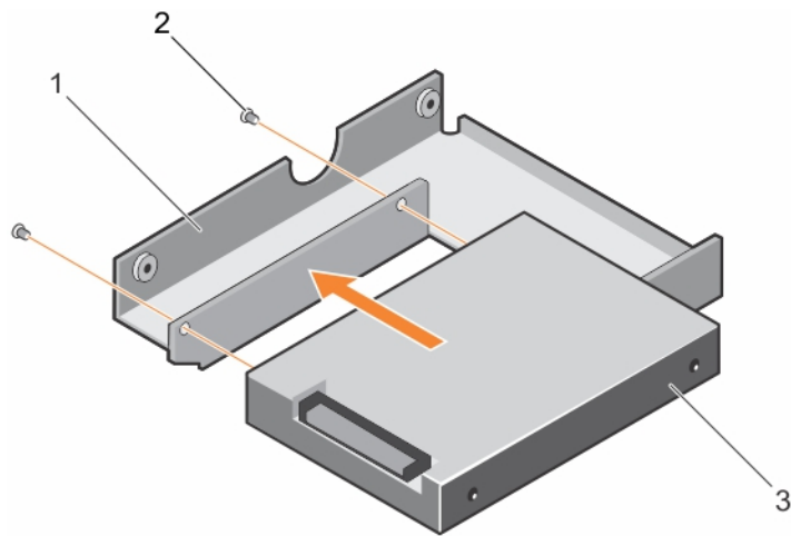
図 41. 3.5 インチハードドライブアダプタへのホットスワップ対応 2.5 インチハードドライブの取り付け
