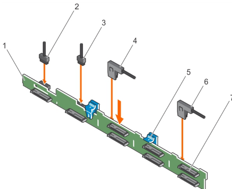
図 93. 2.5 インチ 8 台搭載の SAS/SATA バックプレーンの取り付け
