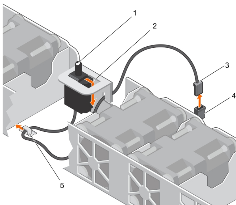
図 19. イントルージョンスイッチの取り外し
