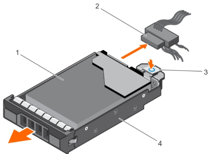
図 30. ケーブル接続式ハードドライブキャリアの取り外し
