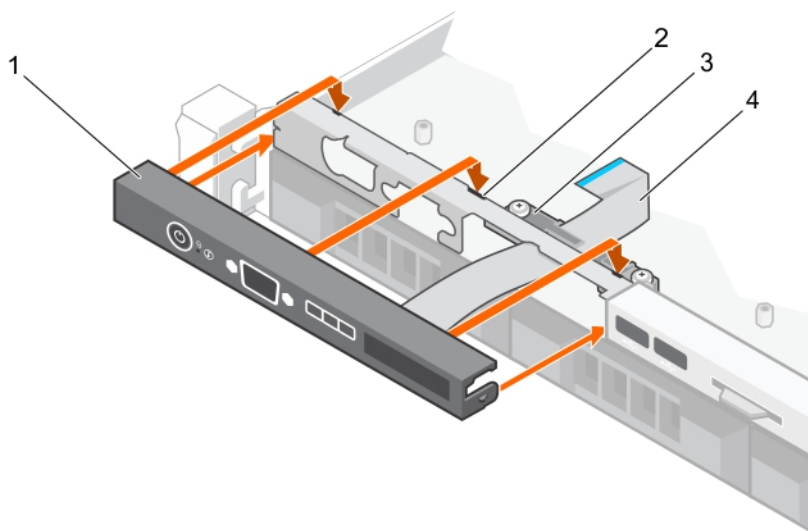
図 96. LCDコントロールパネルの取り付け—4 台の 3.5 インチ ホットスワップ対応ハードドライブ シャーシ
