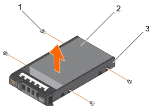
図 44. ハードドライブキャリアからのホットスワップ対応ハードドライブの取り外し
