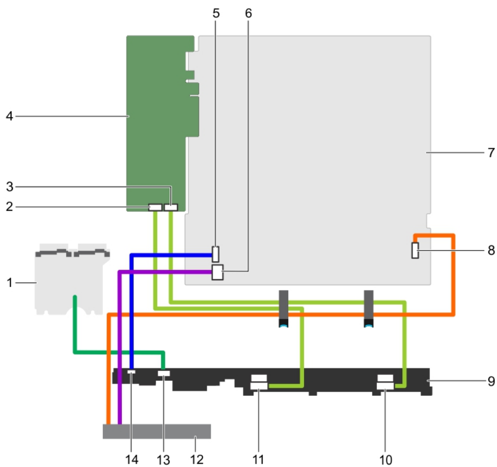
図 87. ケーブル配線図 — PERC カード搭載 2.5 インチ SAS/SATA バックプレーン 8 台
