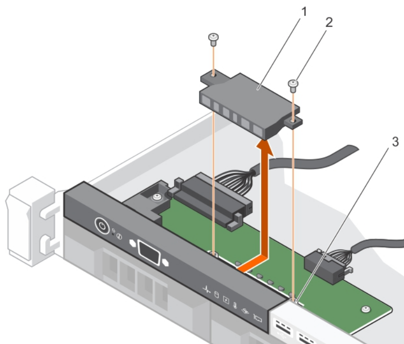
図 100. LED モジュールの取り付け—4 台のケーブル接続式ハードドライブ シャーシ
