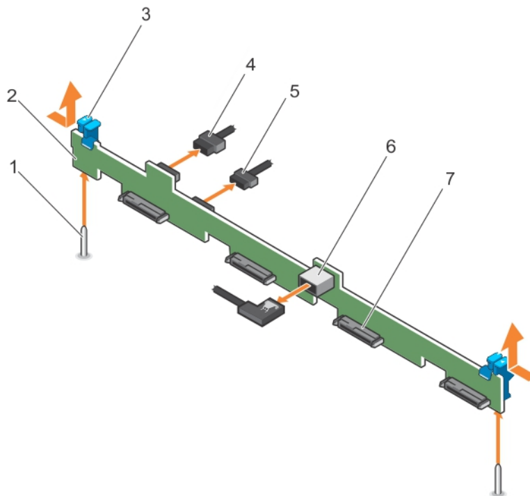
図 84. 4 台の 3.5 インチまたは 2.5 インチ ハードドライブの SAS/SATA バックプレーンの取り外し
