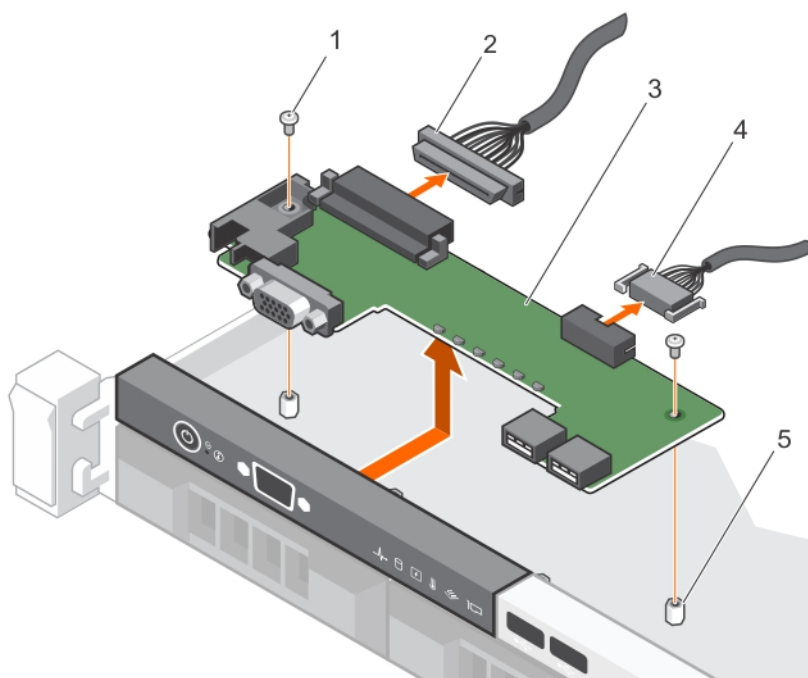
図 99. LED コントロール パネル ボードの取り外し—4 台のケーブル接続式ハードドライブ シャーシ
