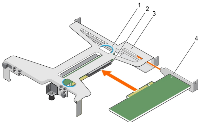
図 58. 拡張カードライザーへの拡張カードの取り付け
