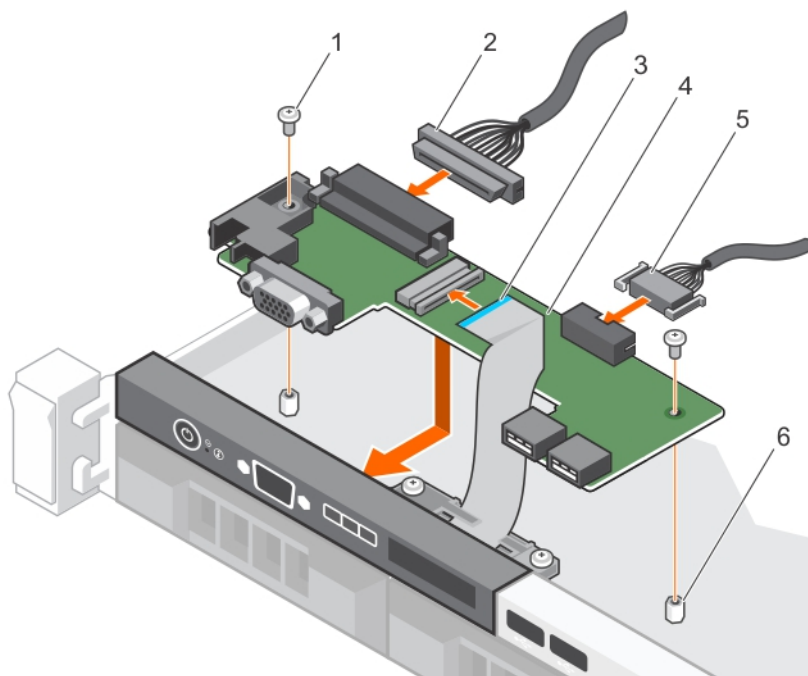
図 97. LCDコントロールパネルボードの取り付け—4 台のハードドライブ シャーシ
