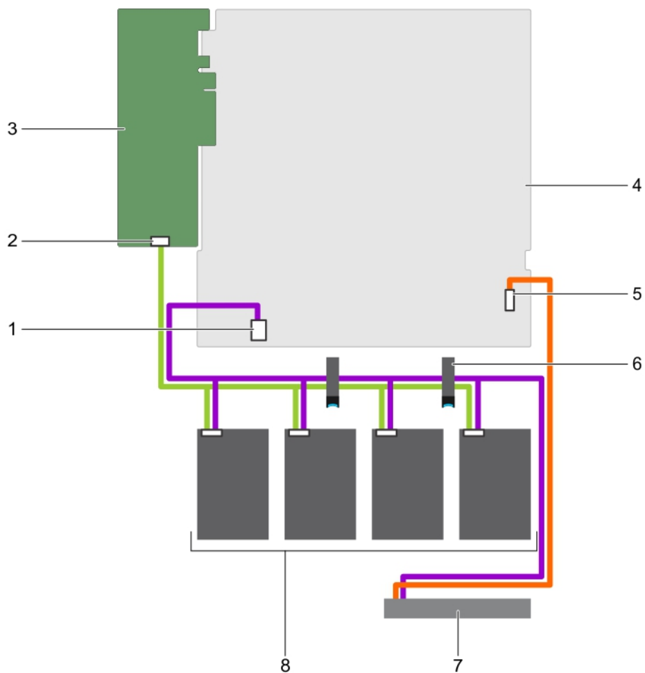
図 89. ケーブル配線図 — 4 台の 3.5 インチケーブル接続式ハードドライブおよび PERC カード
