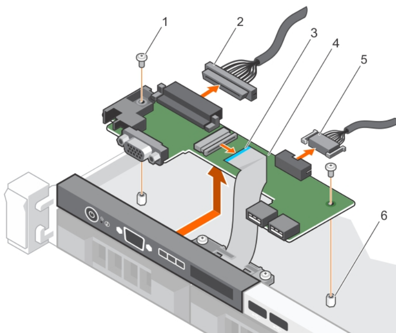
図 95. LCD コントロール パネル ボードの取り外し—4 台のハード ドライブ シャーシ
