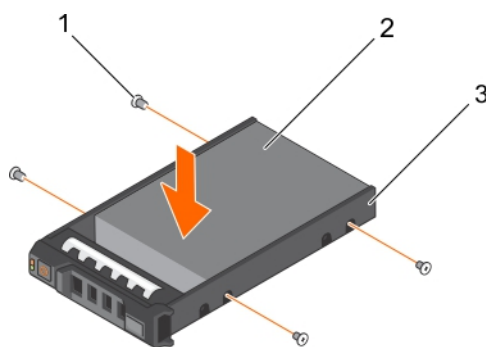
図 45. ホットスワップ対応ハードドライブキャリアへのホットスワップ対応ハードドライブの取り付け
