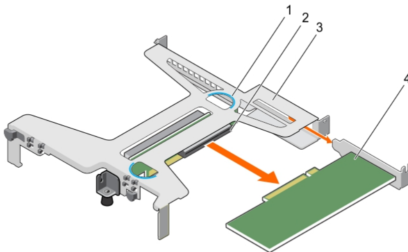
図 57. 拡張カードライザーからの拡張カードの取り外し
