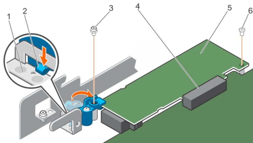
図 63. PERC カードのロックを閉める
