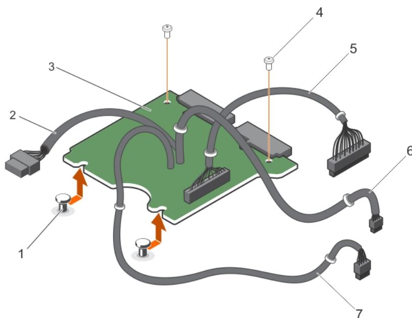
図 102. 電源インタポーザボードの取り外し
