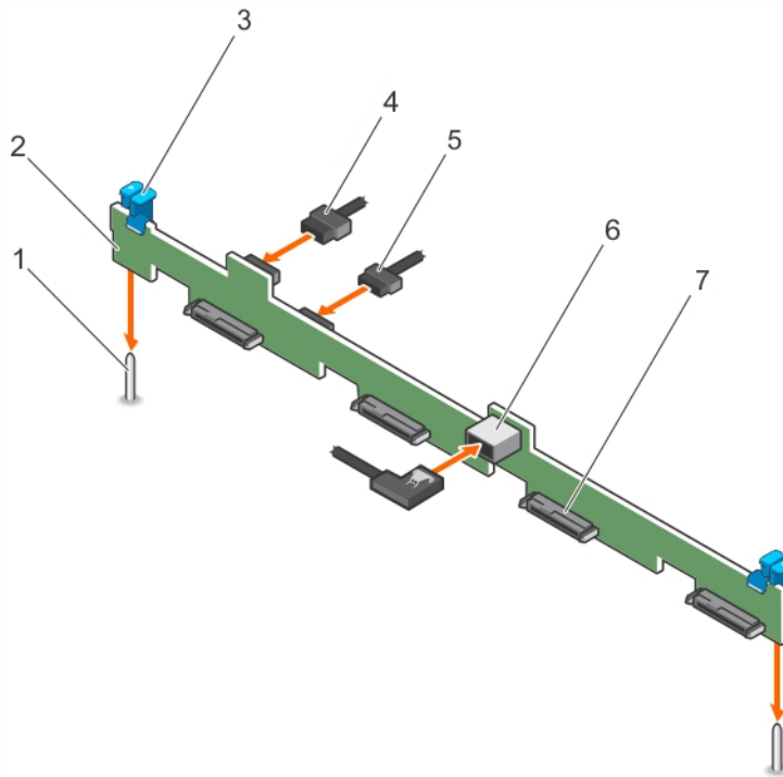
図 92. 3.5 インチハードドライブ 4 台搭載の SAS/SATA バックプレーンの取り付け
