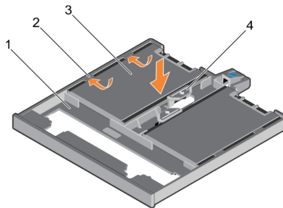
図 38. SSD トレイへの 1.8 インチソリッドステートドライブの取り付け
