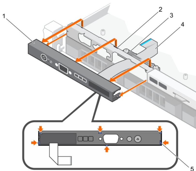
図 94. LCD コントロール パネルの取り外し—4 台の 3.5 インチ ホットスワップ対応ハード ドライブ シャーシ
