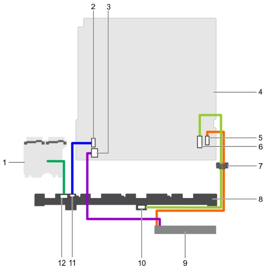
図 85. ケーブル配線図 — 3.5 インチまたは 2.5 インチ ハードドライブ SAS/SATA バックプレーン 4 台
