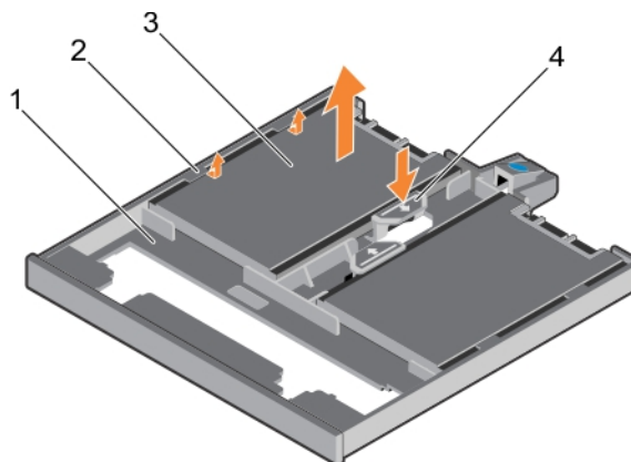
図 37. SSD トレイからの 1.8 インチ ソリッド ステート ドライブの取り外し
