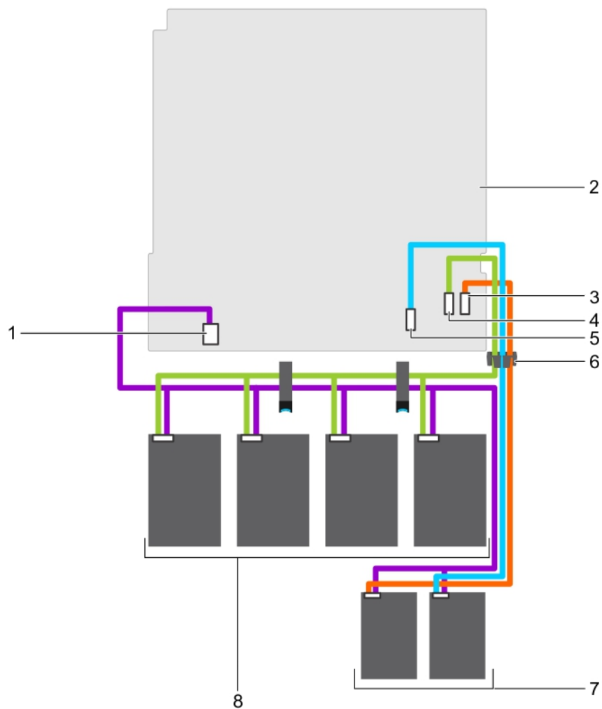
図 90. ケーブル配線図 — 4 台の 3.5 インチケーブル接続式ハードドライブと 2 台の 1.8 インチ SSD
