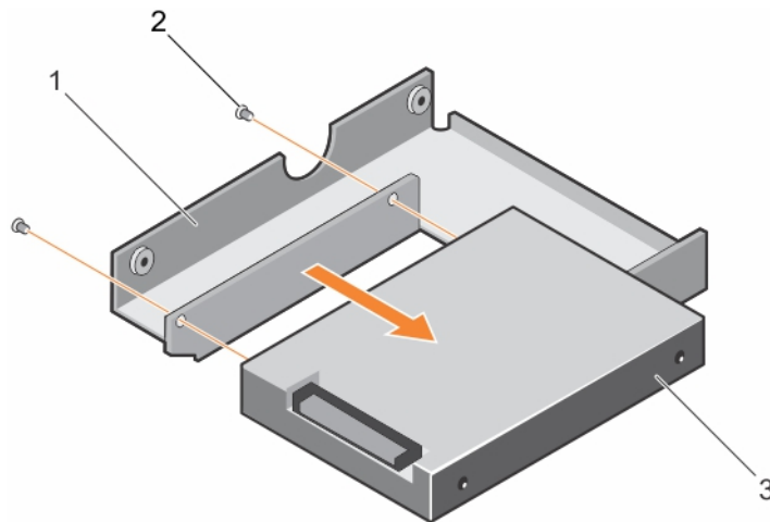
그림 38. 3.5인치 하드 드라이브 어댑터에서 2.5인치 핫 스왑 가능한 하드 드라이브 분리
