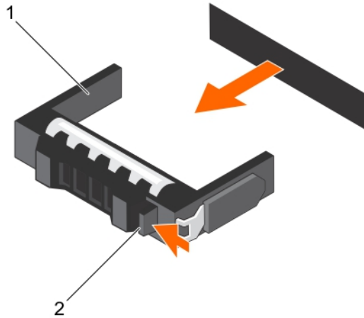
그림 25 . 3.5인치 핫 스왑 가능한 하드 드라이브 캐리어 보호물 분리
