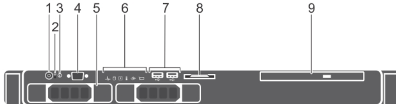
그림 4. 전면 패널 구조 및 표시등 - 2개의 3.5인치 케이블 연결된 하드 드라이브 새시
