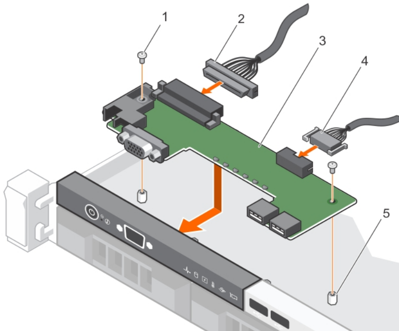
그림 81 . LED 컨트롤 패널 보드 설치 - 4개의 케이블 연결된 하드 드라이브 새시
