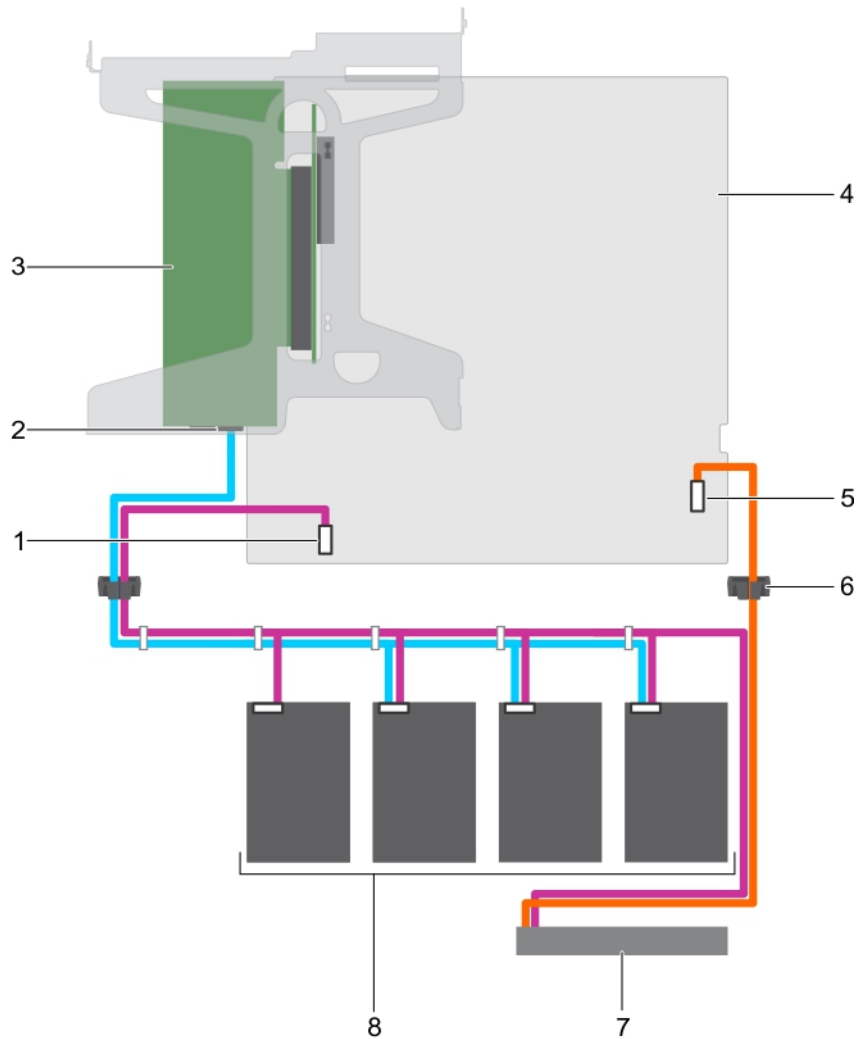
그림 39 . PERC 카드에 4개의 3.5인치 하드 드라이브를 케이블 연결
