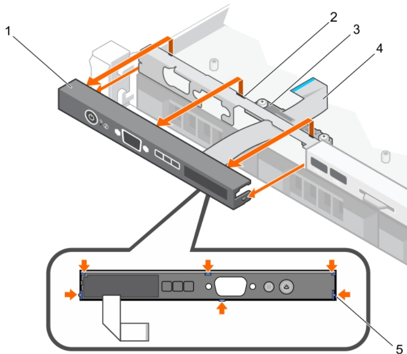
그림 74 . LCD 컨트롤 패널 제거 - 4개의 8.89cm(3.5인치) 핫 스왑 가능 하드 드라이브 새시
