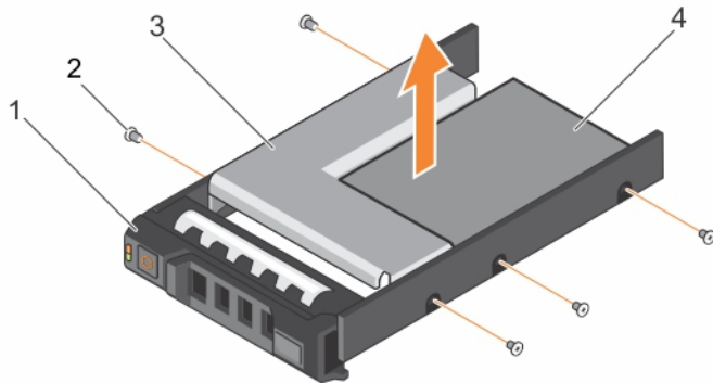
그림 37. 하드 드라이브 캐리어에서 3.5인치 하드 드라이브 어댑터 분리
