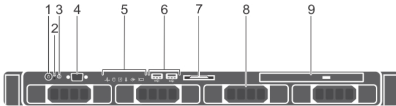
그림 3. 전면 패널 구조 및 표시등 - 4개의 3.5인치 케이블 연결된 하드 드라이브 새시
