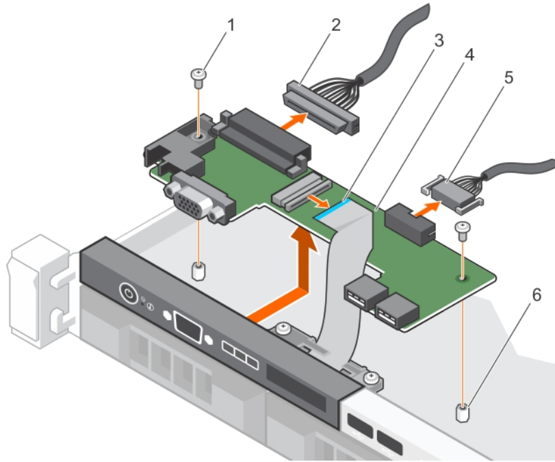
그림 75 . LCD 컨트롤 패널 보드 제거 - 4개의 하드 드라이브 새시
