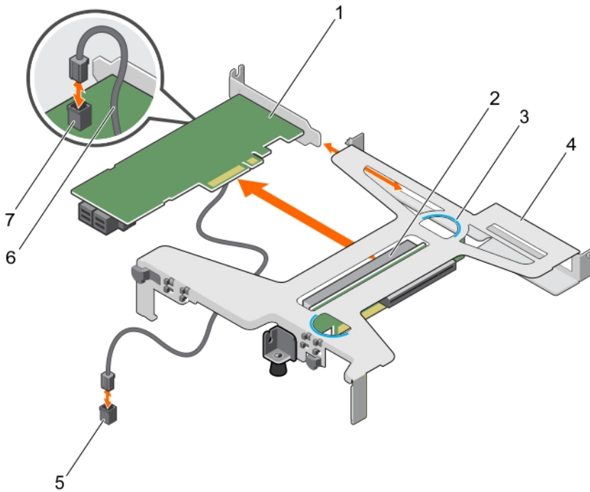
그림 54. 확장 카드 라이저에서 확장 카드 제거
