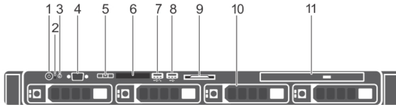
그림 2. 전면 패널 구조 및 표시등 - 4개의 3.5인치 또는 2.5인치 핫 스왑 가능한 하드 드라이브 새시
