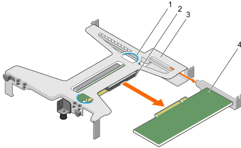
그림 53. 확장 카드 라이저에서 확장 카드 제거
