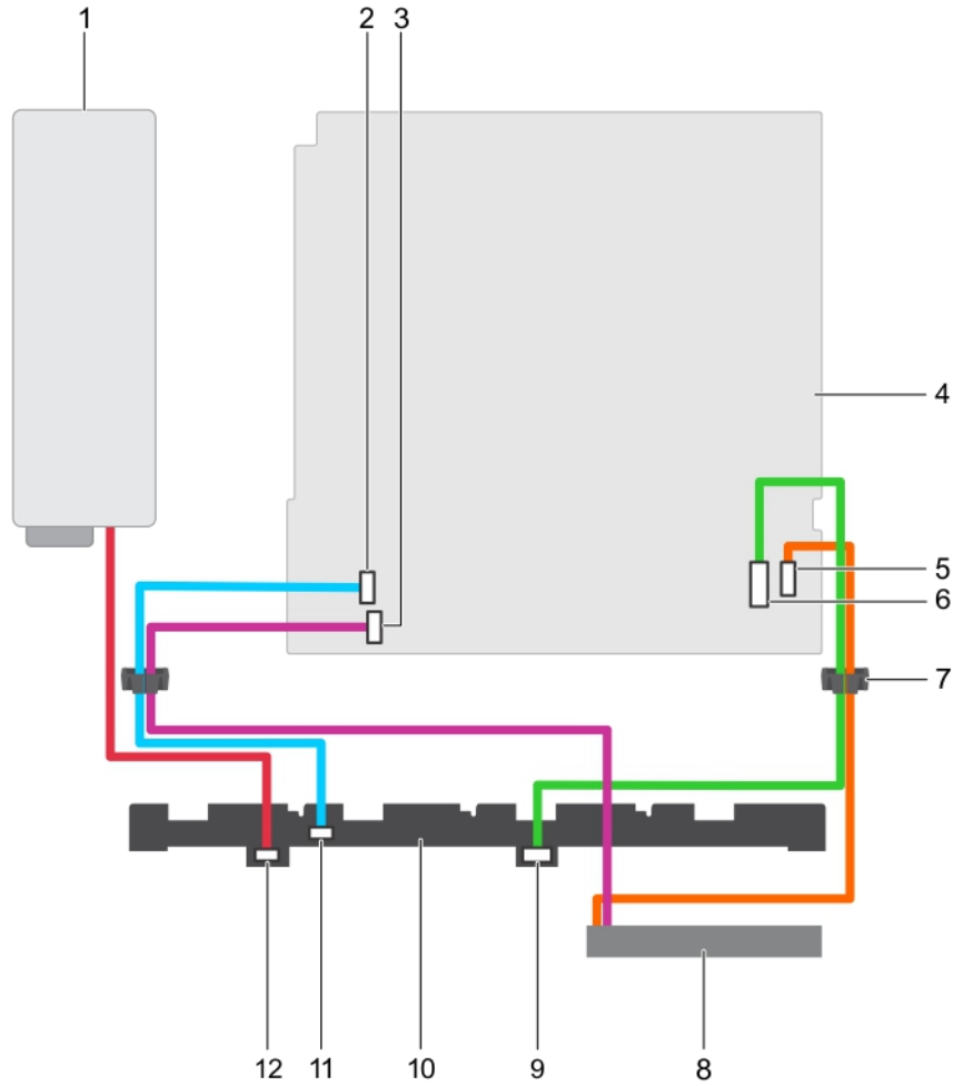
그림 72 . 케이블 연결 다이어그램-4개의 3.5인치 핫 스왑 가능 SAS/SATA 하드 드라이브 후면판
