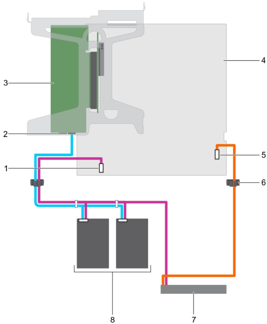
그림 41 . PERC 카드에 2개의 3.5인치 하드 드라이브를 케이블 연결
