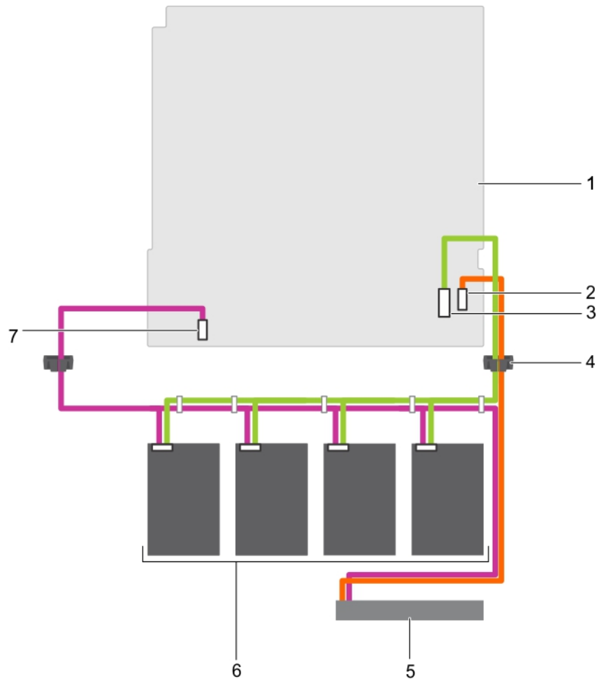
그림 40. 4개의 3.5인치 하드 드라이브를 시스템 보드의 SATA 커넥터에 케이블 연결
