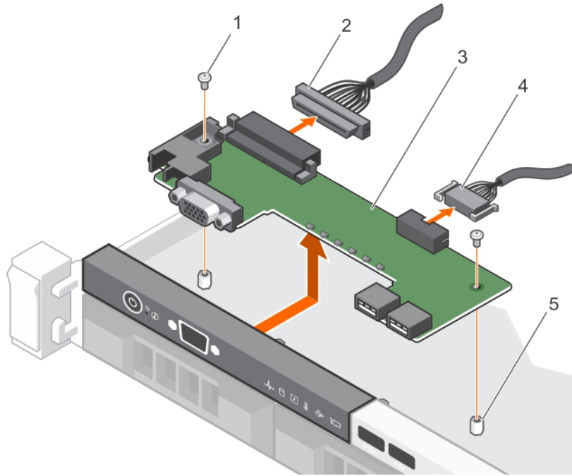
그림 79 . LED 컨트롤 패널 보드 제거 - 4개의 케이블 연결된 하드 드라이브 새시
