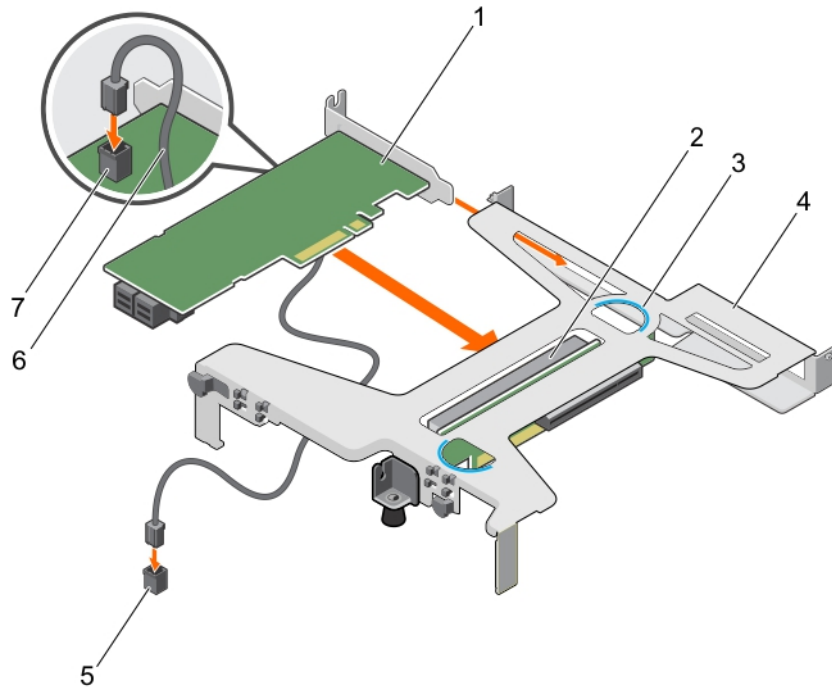
그림 56. 확장 카드 라이저에 확장 카드 설치
