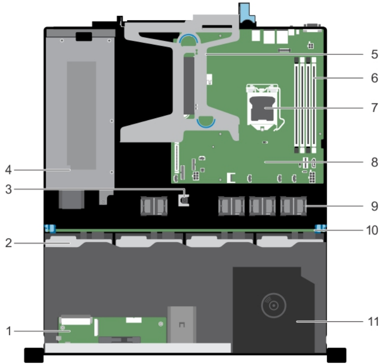
그림 15 . 시스템 내부 - 4개의 3.5인치 또는 2.5인치 핫 스왑 가능한 하드 드라이브 시스템
