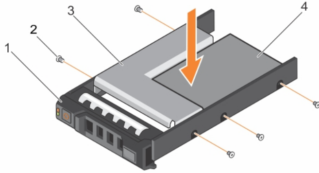
그림 36. 핫 스왑 가능한 하드 드라이브 캐리어에 3.5인치 하드 드라이브 어댑터 설치
