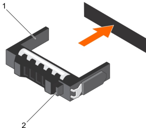
그림 26 . 3.5인치 핫 스왑 가능한 하드 드라이브 캐리어 보호물 설치
