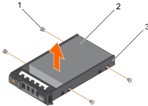
그림 32. 하드 드라이브 캐리어에서 핫 스왑 가능한 하드 드라이브 분리
