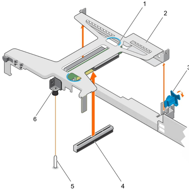
그림 51. 확장 카드 라이저 분리 및 설치
