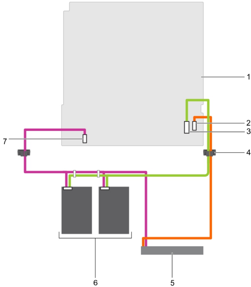
그림 42 . 2개의 3.5인치 하드 드라이브를 시스템 보드의 SATA 커넥터에 케이블 연결
