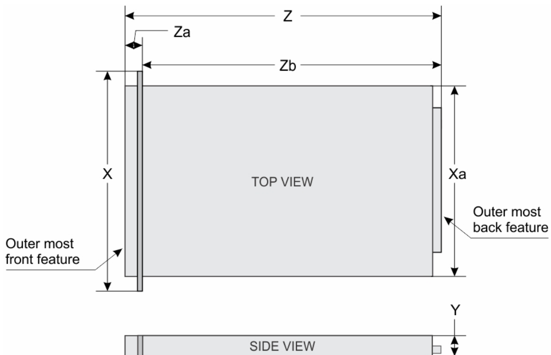
그림 10 . PowerEdge R230 시스템의 새시 크기
