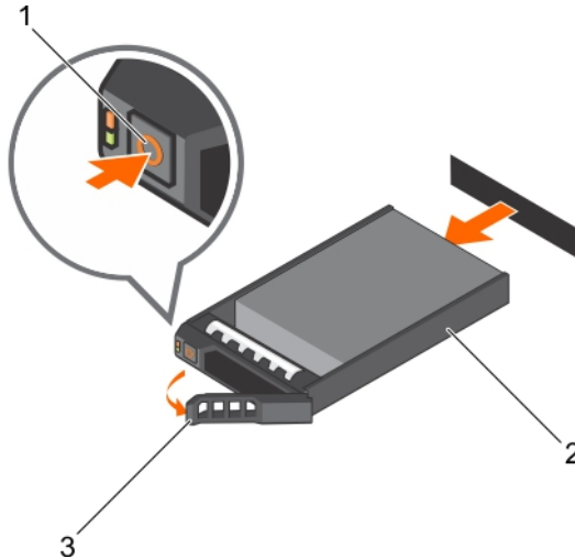
그림 31. 핫 스왑 가능한 하드 드라이브 또는 SSD 분리
