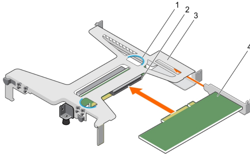
그림 55. 확장 카드 라이저에 확장 카드 설치
