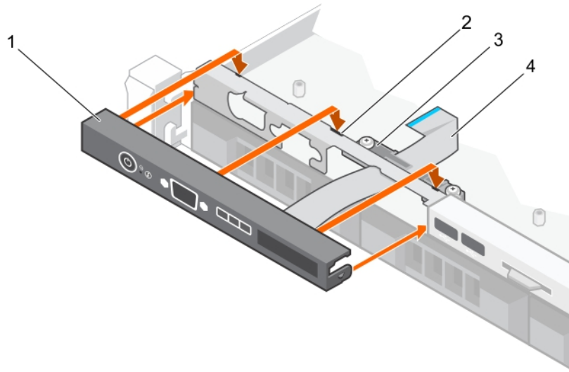
그림 76 . LCD 컨트롤 패널 설치 - 4개의 8.89cm(3.5인치) 핫 스왑 가능 하드 드라이브 새시
