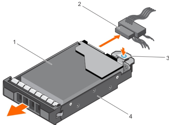
그림 27. 케이블 연결된 하드 드라이브 캐리어 분리
