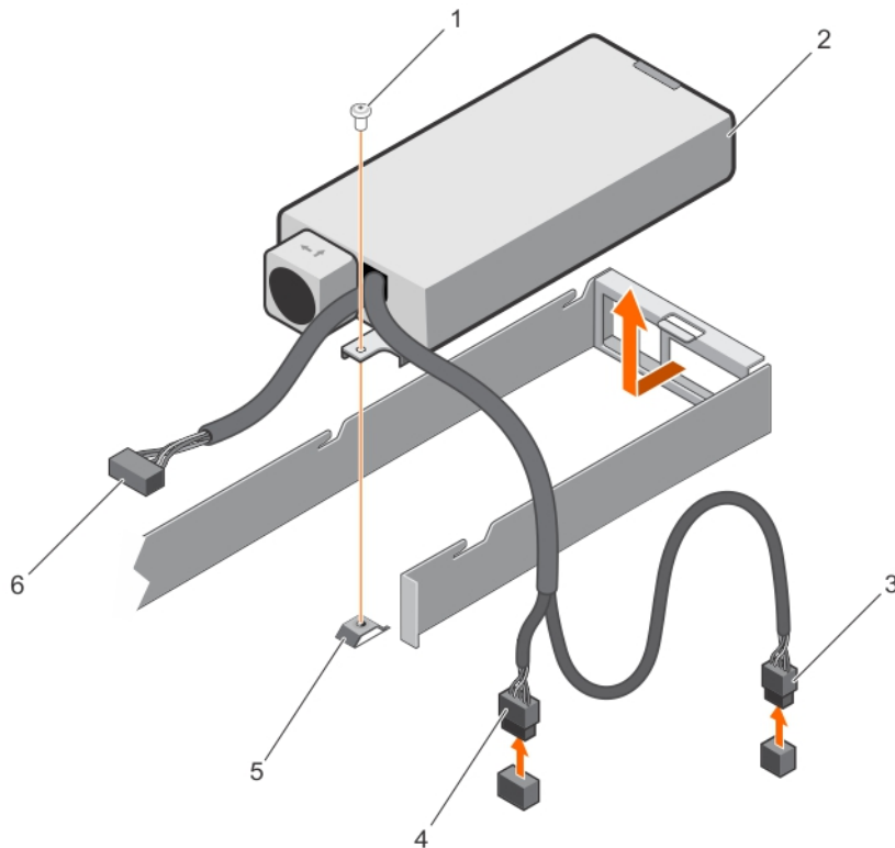
그림 67. 케이블 연결된 전원 공급 장치 분리
