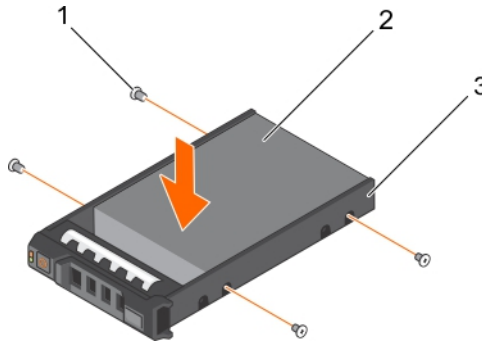
그림 33. 핫 스왑 가능한 하드 드라이브 캐리어에 핫 스왑 가능 하드 드라이브 설치
