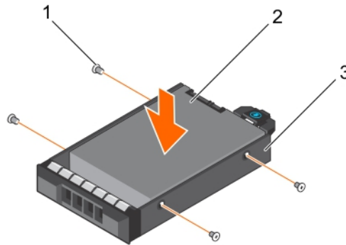
그림 29. 케이블 연결된 하드 드라이브 캐리어에 케이블 연결된 하드 드라이브 설치
