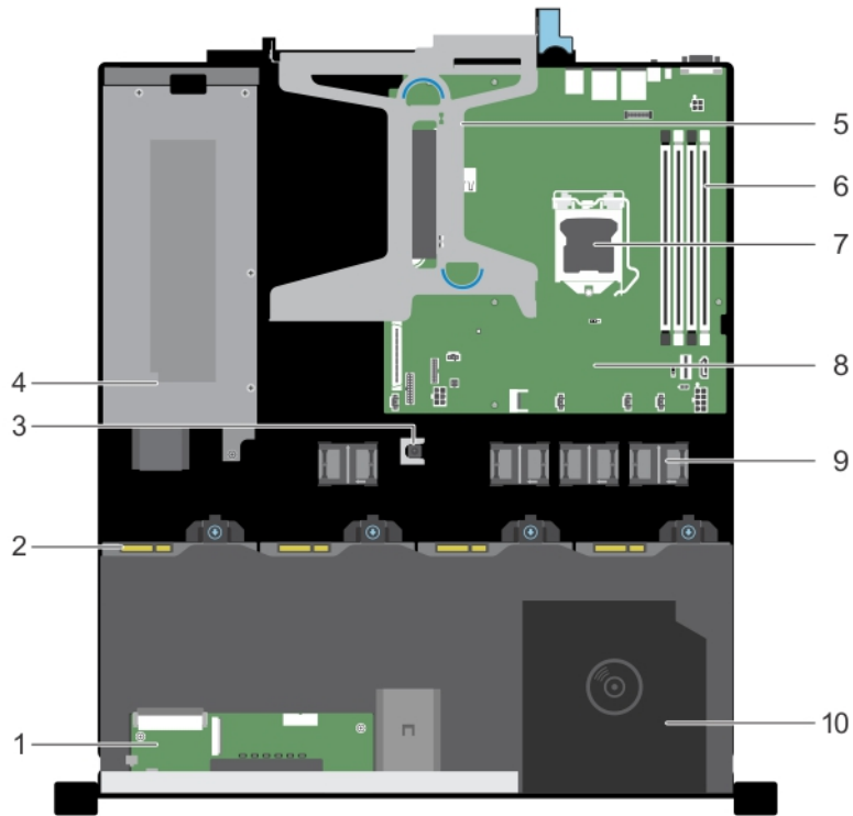
그림 16 . 시스템 내부 - 4개의 3.5인치 케이블 연결된 하드 드라이브 시스템
