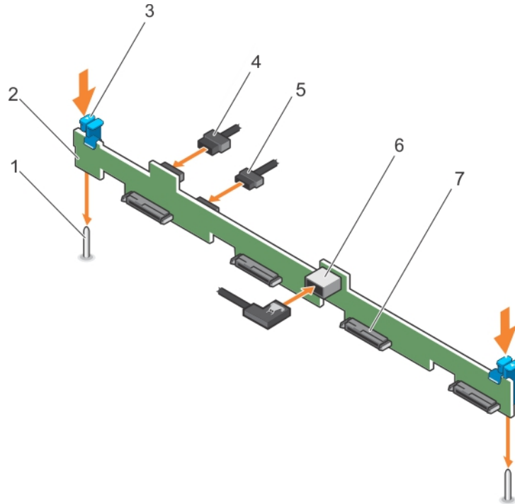
그림 73 . 4개의 8.89cm(3.5인치) 핫 스왑 가능 SAS/SATA 하드 드라이브 백플레인 설치
