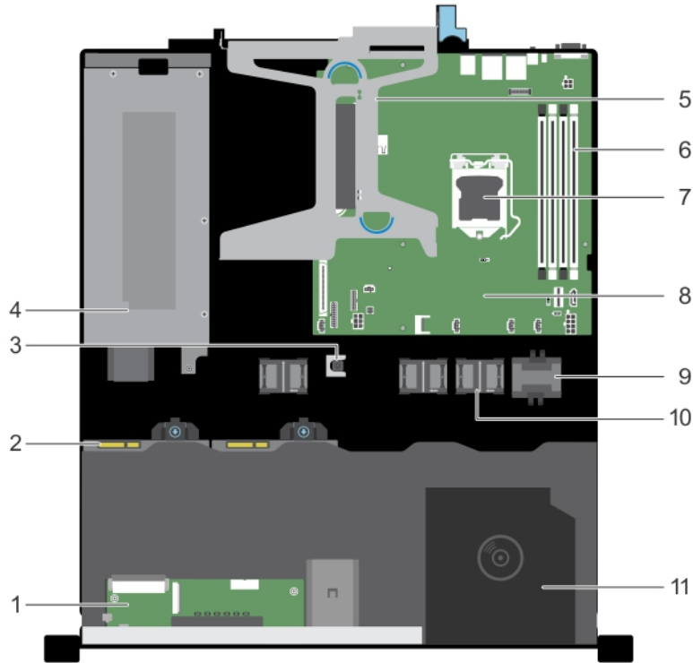
그림 17. 시스템 내부 - 2개의 3.5인치 케이블 연결된 하드 드라이브 시스템
