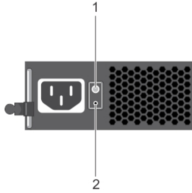
그림 9. 비중복 케이블 연결 AC PSU 상태 표시등 및 자체 진단 단추
