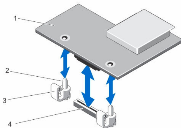
图 23: 卸下和安装 iDRAC7 Enterprise 卡
