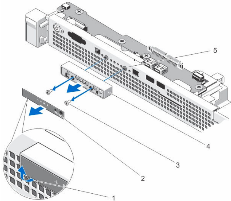
图 13: 卸下和安装 LED 模块
