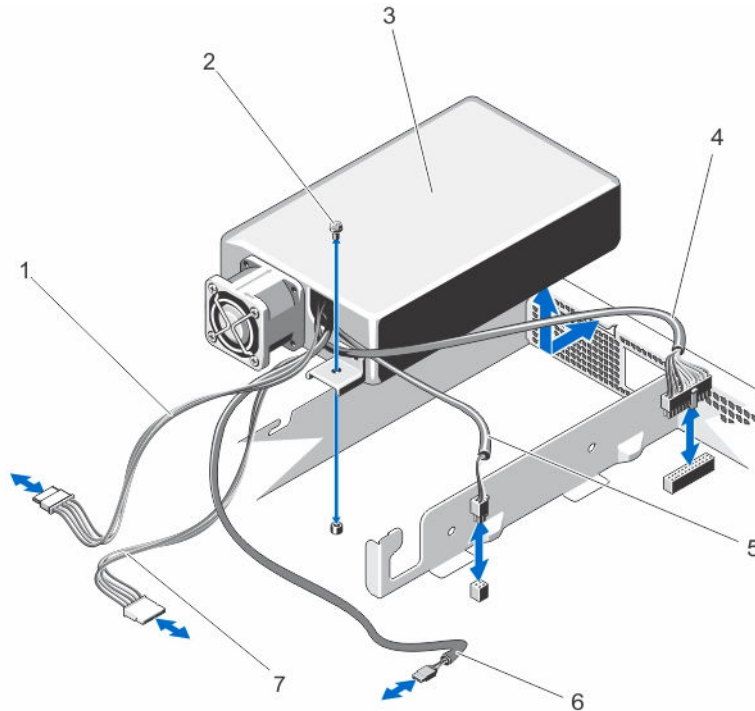
图 27: 卸下和安装电源设备
