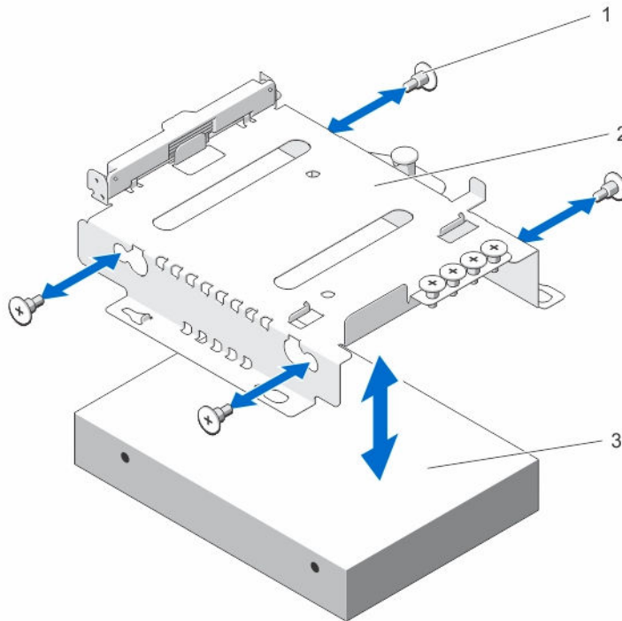
图 10: 在硬盘驱动器固定框架中卸下和安装 3.5 英寸硬盘驱动器
