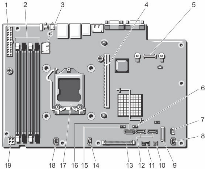
图 29: 系统板跳线和连接器
