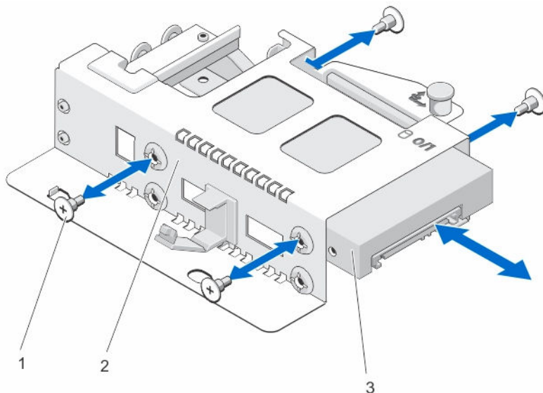
图 12: 在硬盘驱动器固定框架中卸下和安装 2.5 英寸硬盘驱动器
