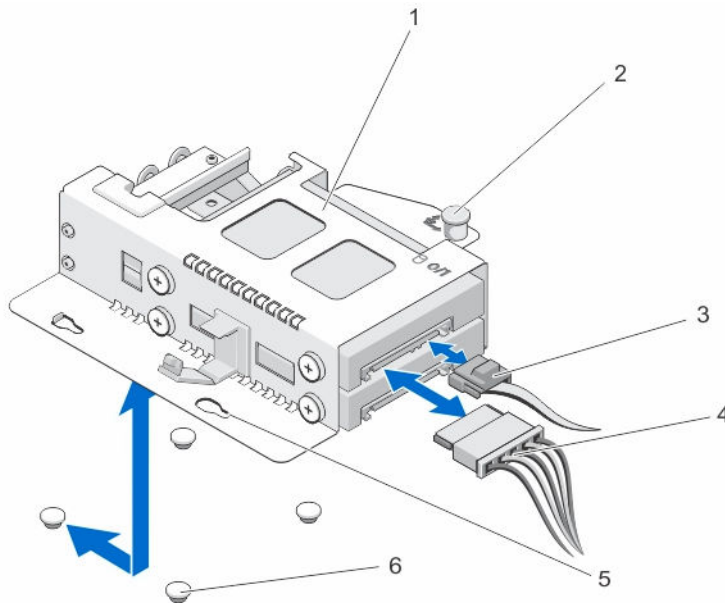
图 11: 卸下和安装 2.5 英寸硬盘驱动器固定框架
