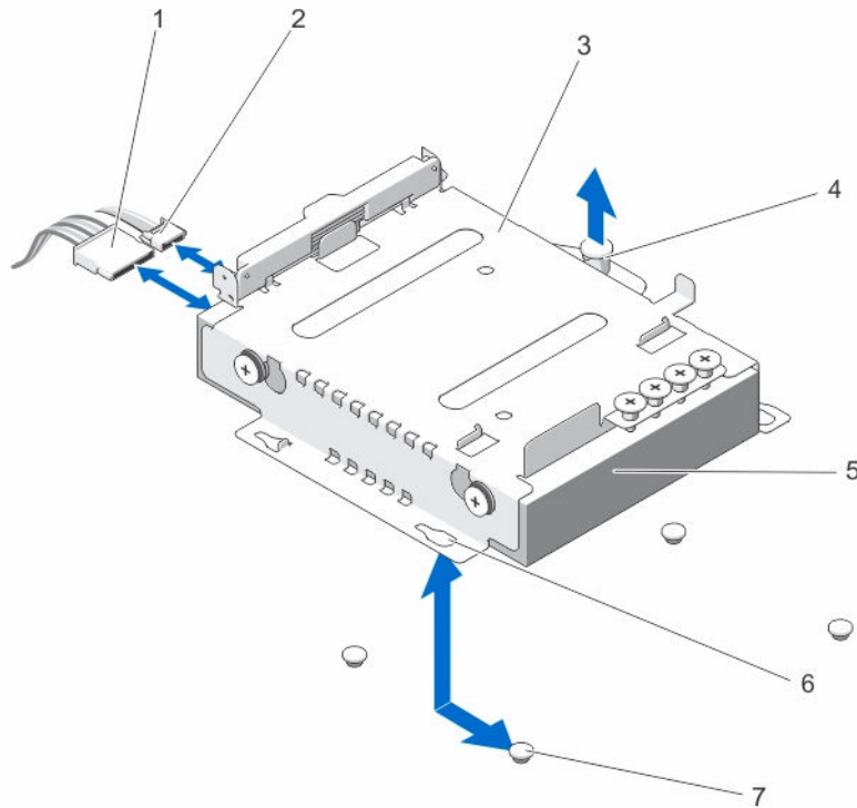
图 9: 卸下和安装 3.5 英寸硬盘驱动器 (HDD1) 固定框架
