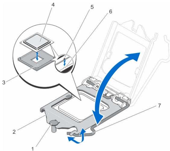
图 26: 卸下和安装处理器
