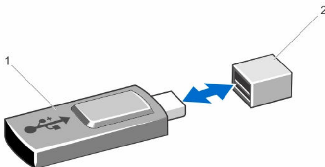
图 20: 卸下和安装内部 USB 盘
