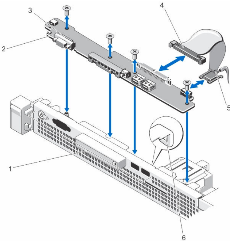
图 14: 卸下和安装控制面板线路板
