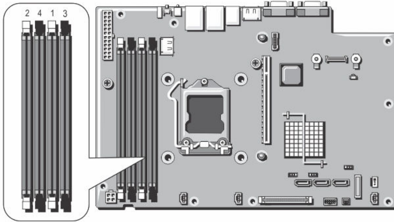
图 17: 内存插槽位置
