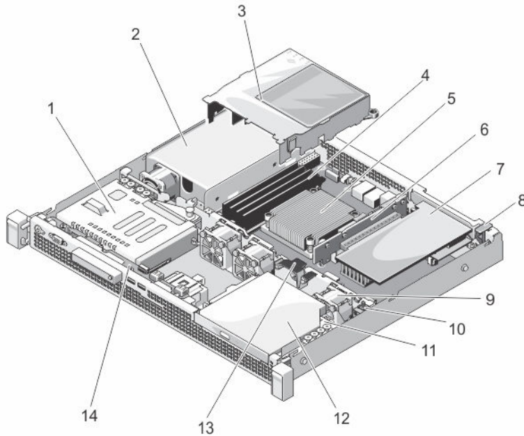
图 6: 系统内部
