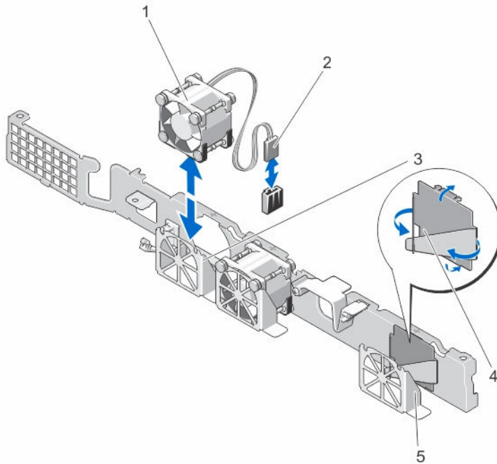
图 15: 卸下和安装冷却风扇
