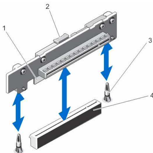
图 22: 卸下和安装扩展卡提升板
