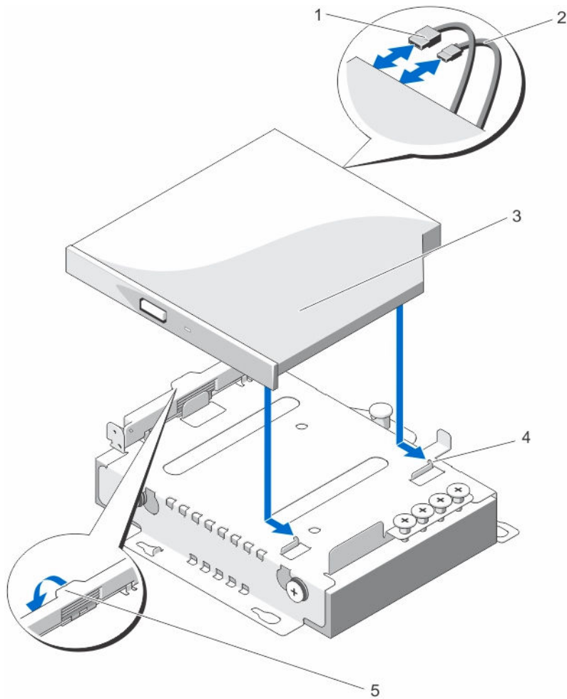
图 8: 卸下和安装光盘驱动器
