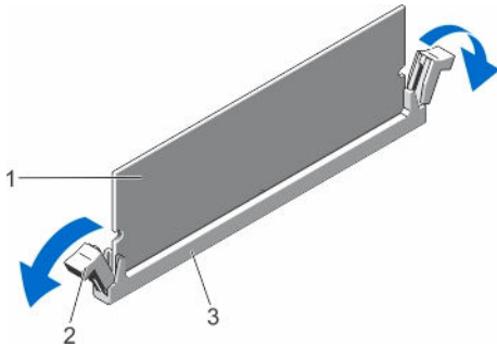
图 18: 卸下内存模块
