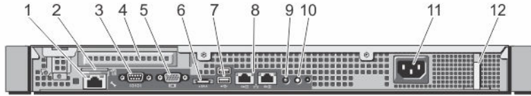
图 2: 背面板功能部件和指示灯
