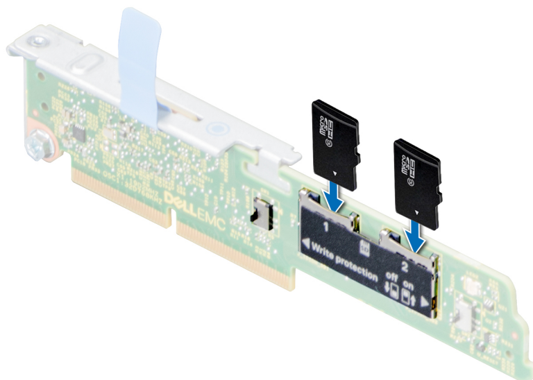
Figure 73. Installation d'une carte MicroSD
