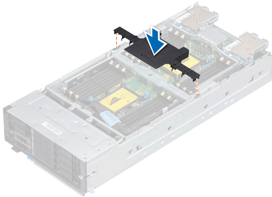
Figure 20. Installation du carénage à air sur le PEM
