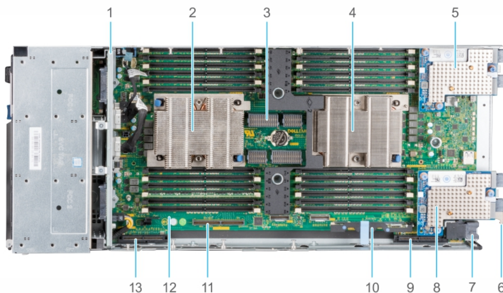
Figure 3. Intérieur du traineau avec carte système
