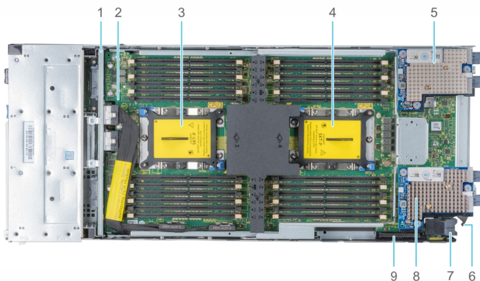
Figure 2. Intérieur du traineau avec PEM
