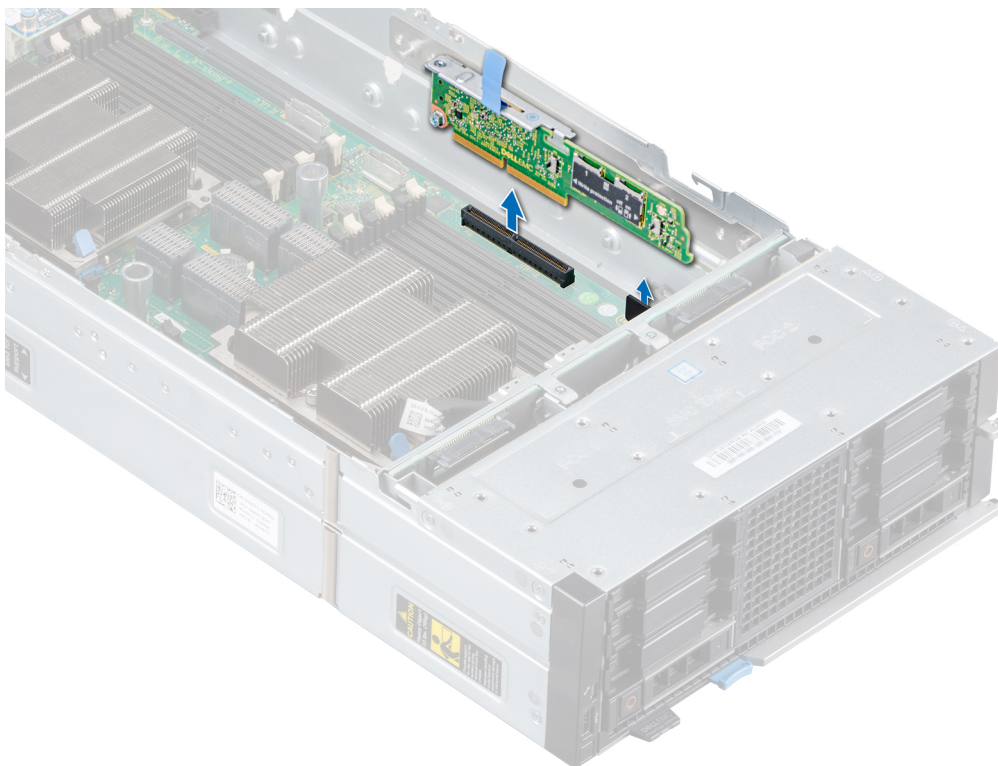
Figure 70. Retrait du module IDSDM
