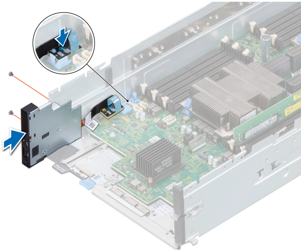
Figure 50. Installation du panneau de commande
