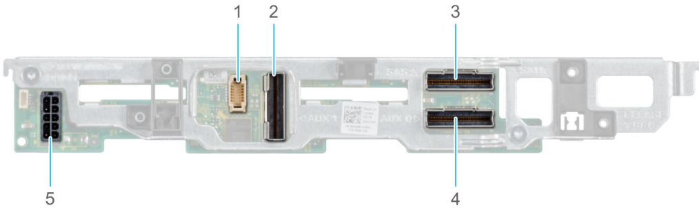
图 28: 4 x 2.5 英寸通用底板
