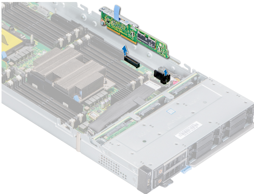
图 66: 卸下 IDSDM 卡
