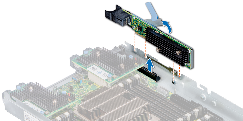
图 76: 卸下小型夹层卡
