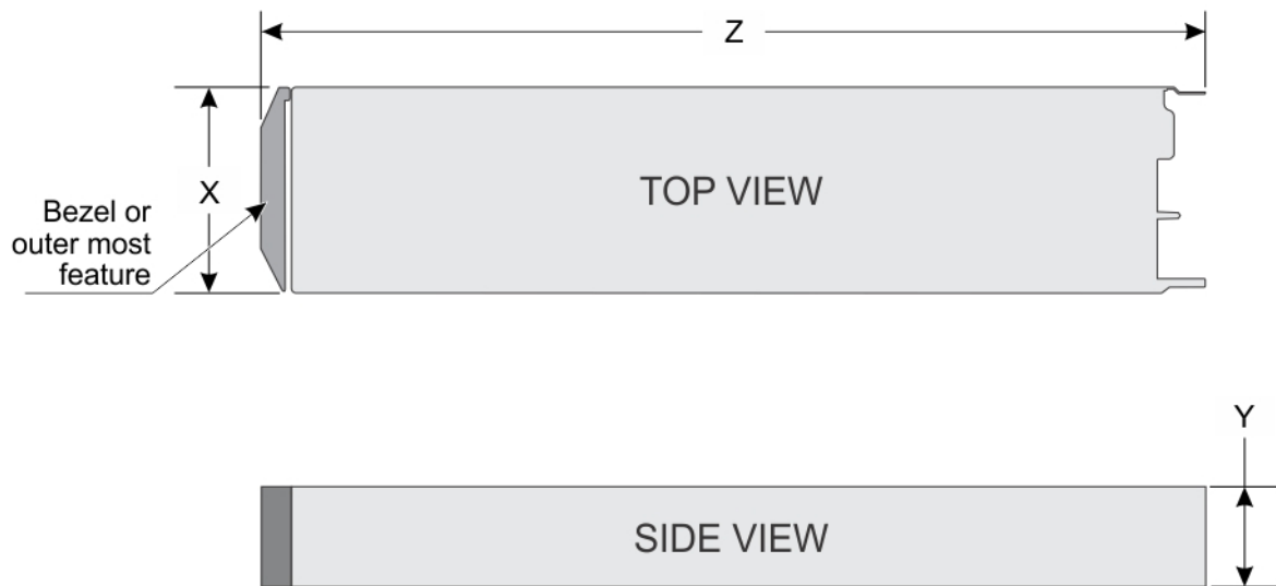
图 88: 系统尺寸
