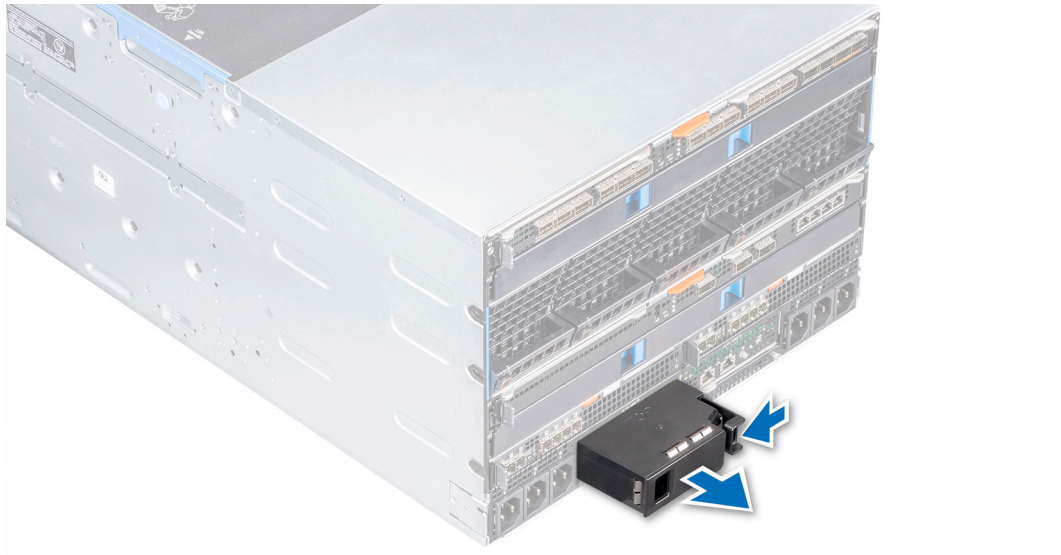
그림 36. 관리 모듈 보호물 제거
