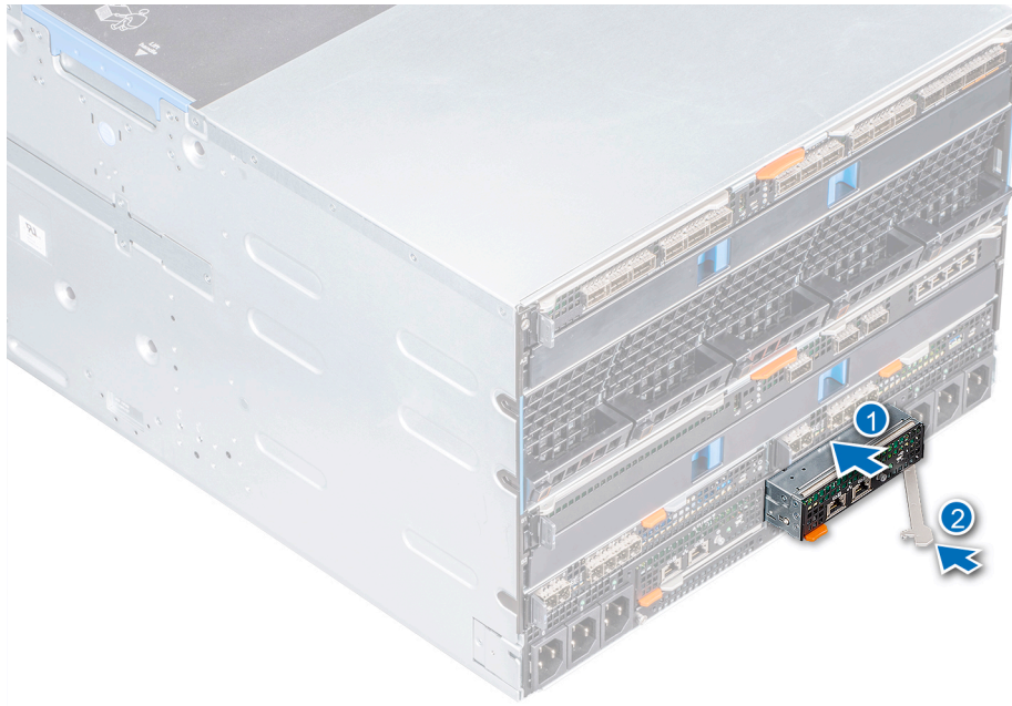
그림 40. 관리 모듈 설치
