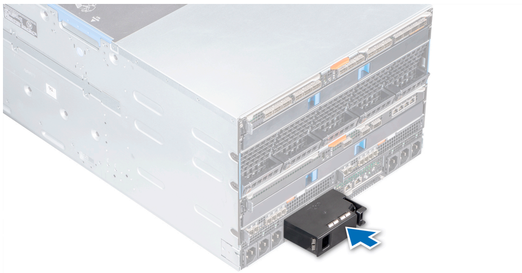
図 37. 管理モジュール ダミーの取り付け
