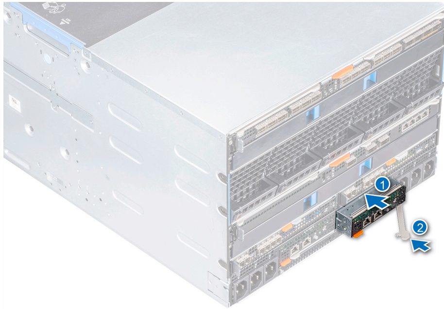
図 40. 管理モジュールの取り付け
