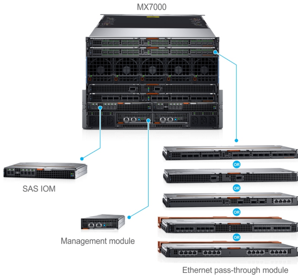
Ilustración 2. Modular de nueva generación: vista posterior
