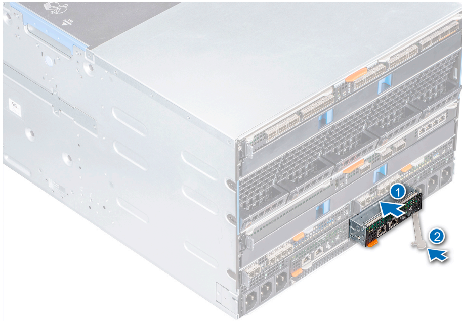
Ilustración 40. Instalación de un módulo de administración
