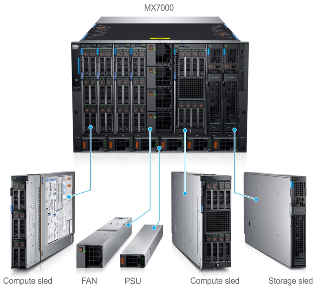
Ilustración 1. Modular de nueva generación: vista frontal
