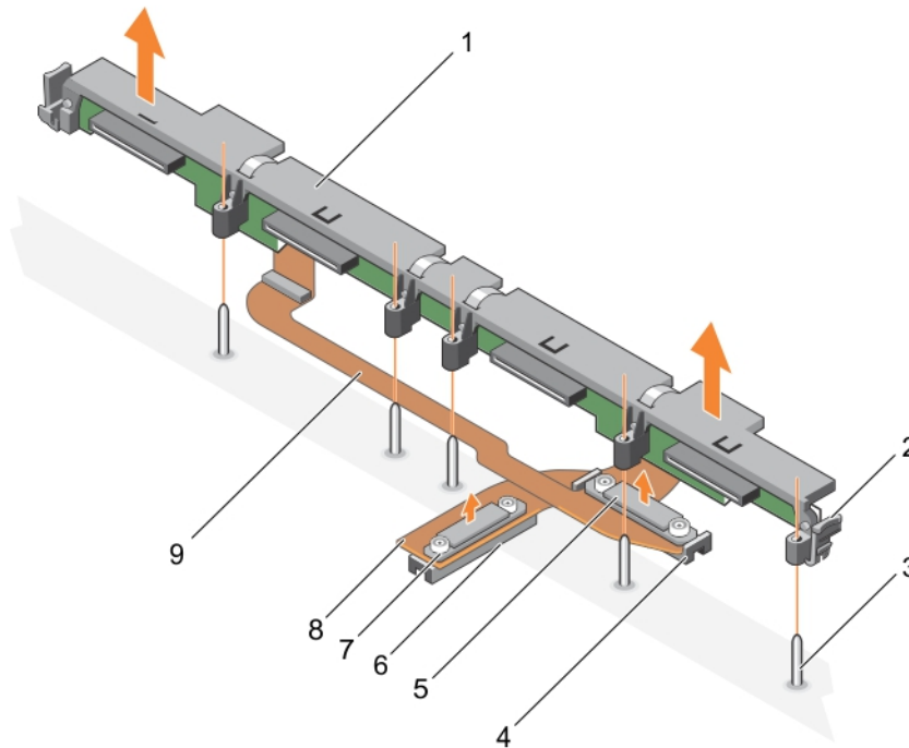
图 58: 卸下 2.5 英寸 (x2) SATA 硬盘驱动器或 SSD 和 2.5 英寸 (x2) PCIe SSD 背板
