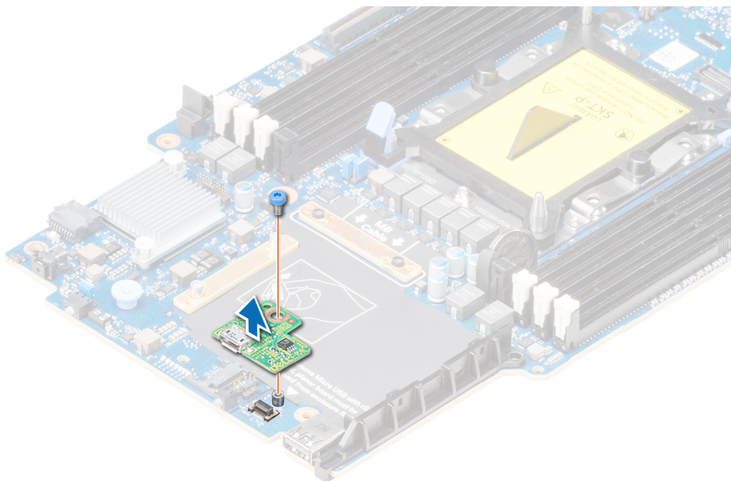
図 58. rSPI カードの取り外し
