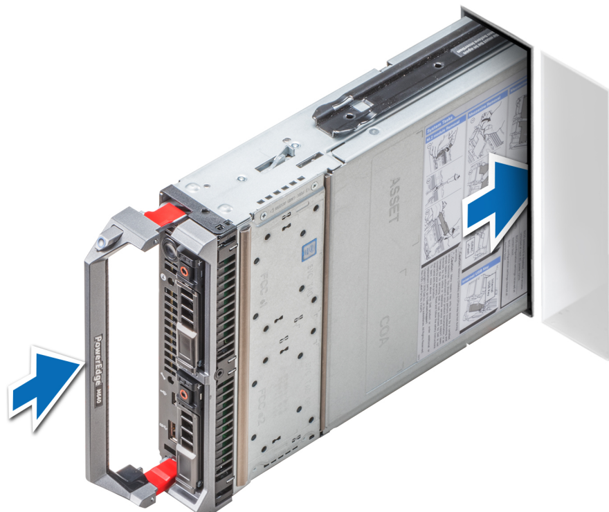
図 10. システムのエンクロージャへの取り付け
