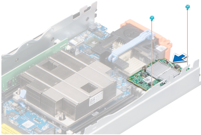
그림 43. 네트워크 도터 카드 설치
