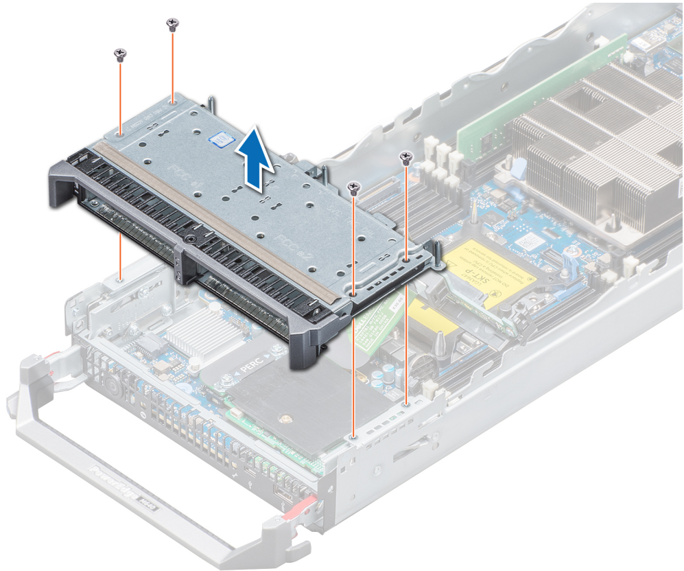
그림 22. 드라이브 케이지 분리
