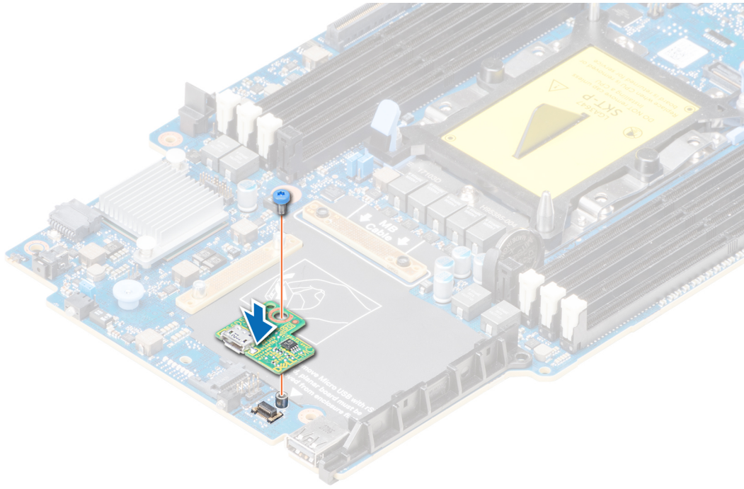
Figure 59. Installation de la carte rSPI
