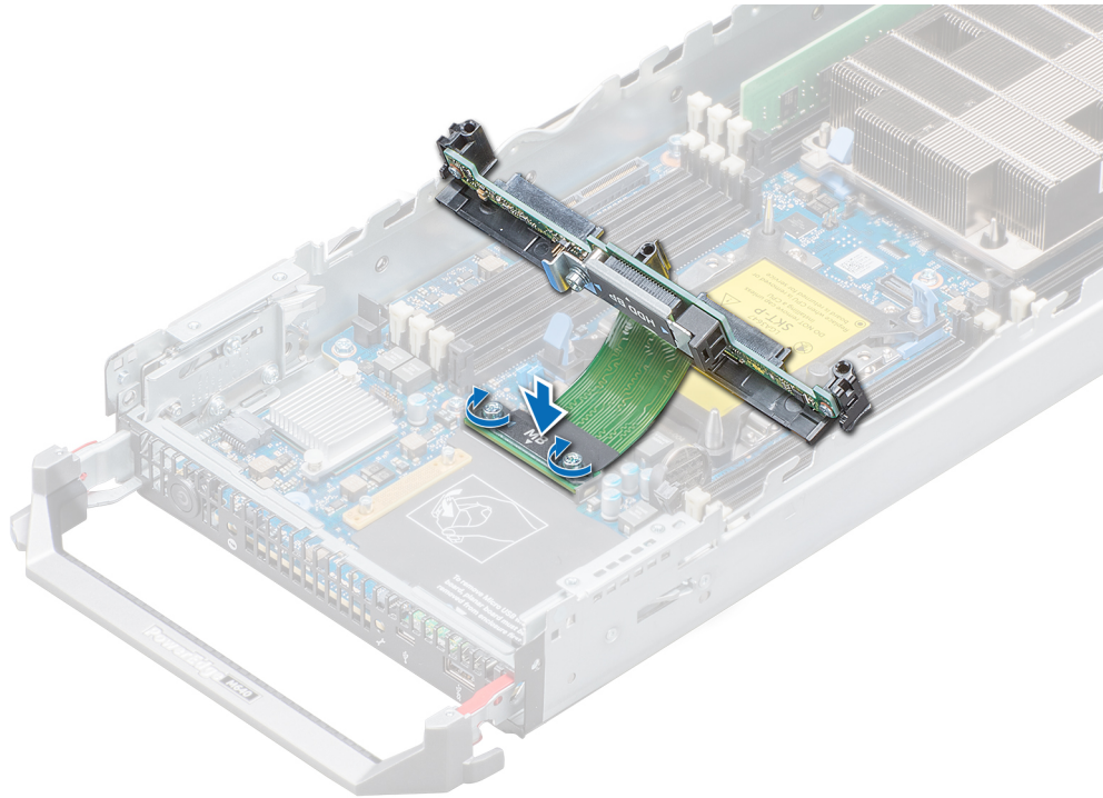
Ilustración 26. Instalación del cable del plano posterior de la unidad de disco duro
