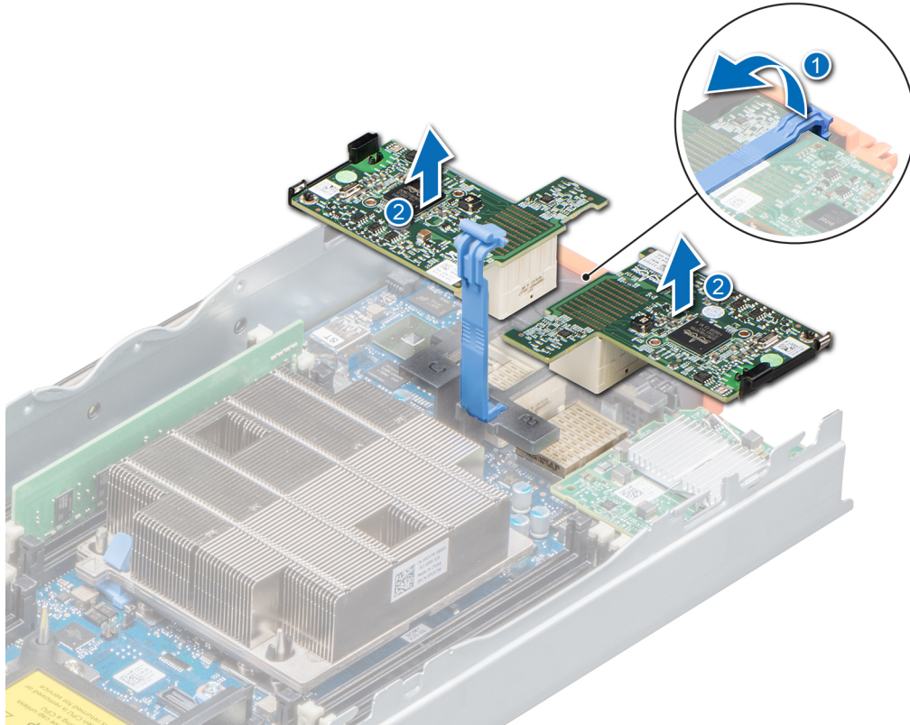
Ilustración 44. Extracción de la Tarjeta intermedia
