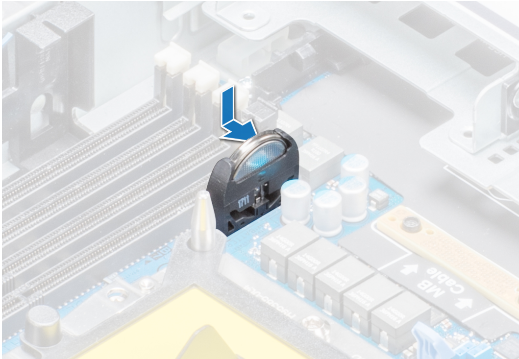
Ilustración 49. Instalación de la batería del sistema
