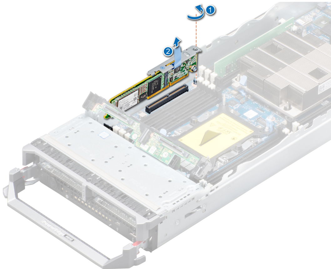
Ilustración 38. Extracción del módulo BOSS M.2
