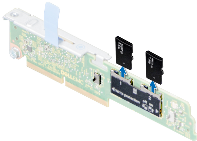
Ilustración 50. Extracción de una tarjeta microSD
