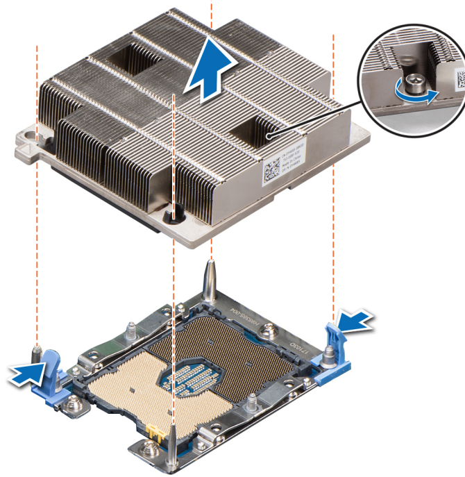
Ilustración 31. Extracción del módulo del procesador y el disipador de calor
