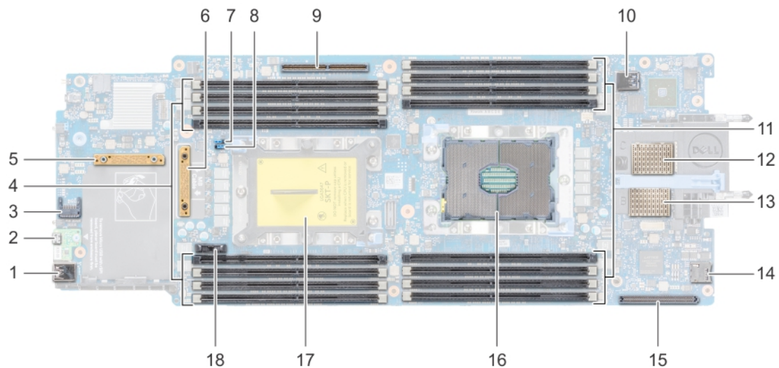
Abbildung 60. Systemplatinenanschlüsse
