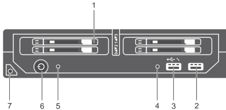
그림 3. 전면 패널 구조 및 표시등 - 1.8인치 SSD시스템
