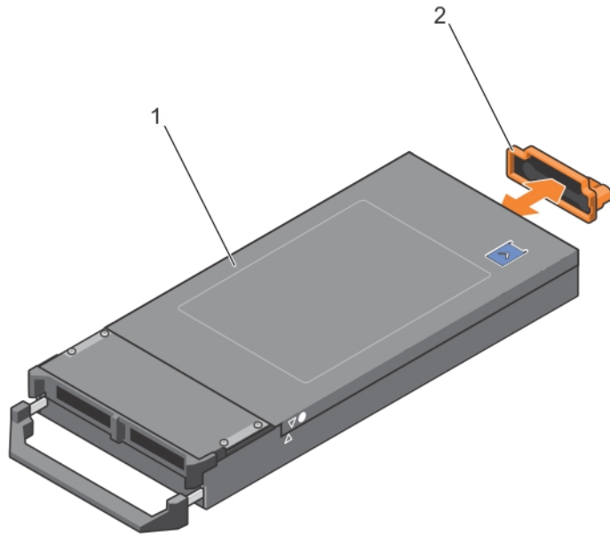
그림 6. I/O 커넥터 덮개 분리 및 설치
