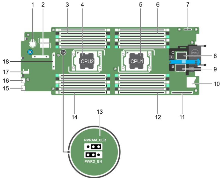
그림 39. 시스템 보드 커넥터
