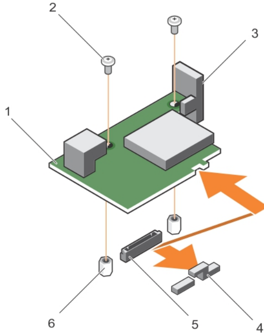
그림 17. IDSDM 카드 분리 및 설치
