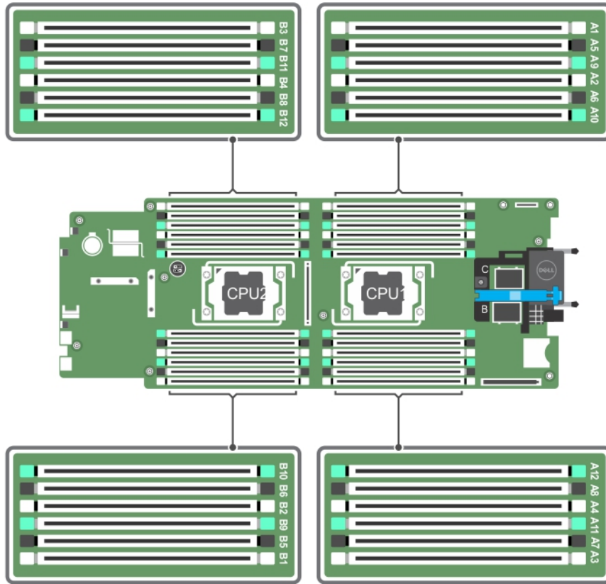
그림 12. 메모리 소켓 위치
