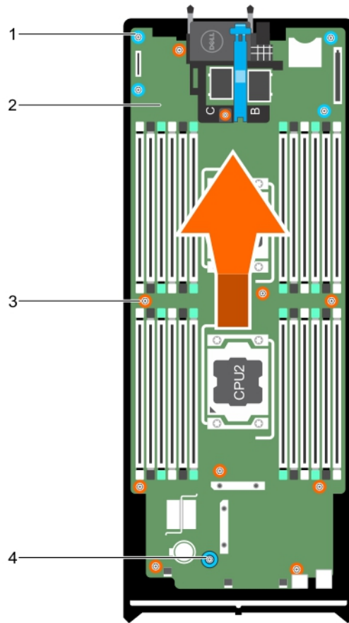
그림 36. 시스템 보드 분리 및 설치
