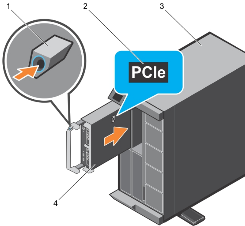
그림 7. 서버 모듈 분리 및 설치
