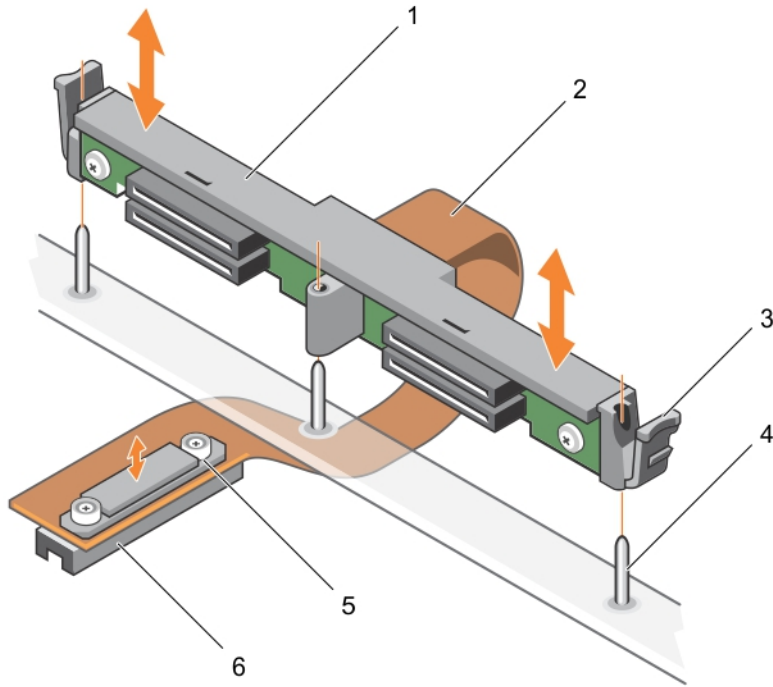
그림 34. 1.8인치(x4) SSD 후면판 분리 및 설치
