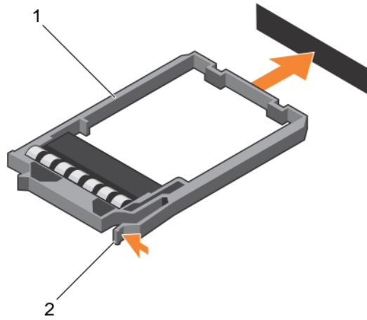
그림 29 . 1.8인치 SSD 보호물 분리 및 설치
