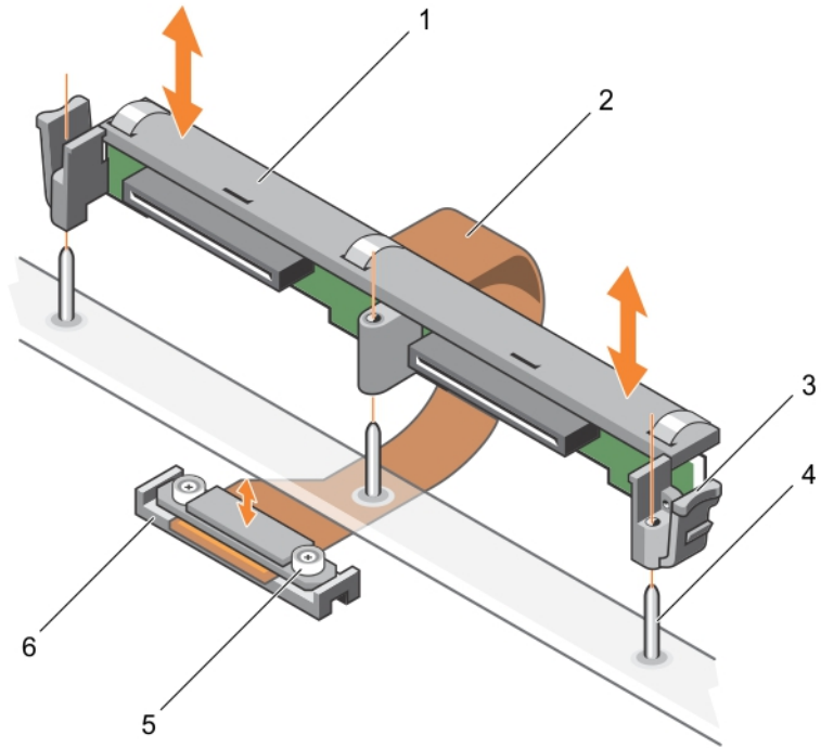
그림 33. 2.5인치(x2) 하드 드라이브/SSD 후면판 분리 및 설치
