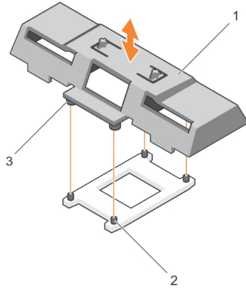
그림 11. 프로세서/DIMM 보호물 분리 및 설치
