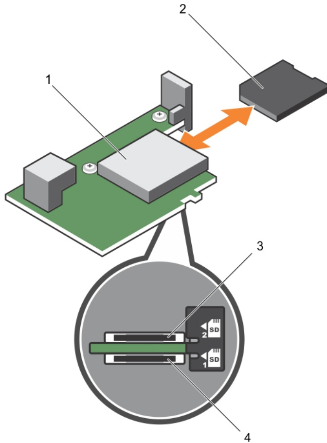
그림 15. SD 카드 교체
