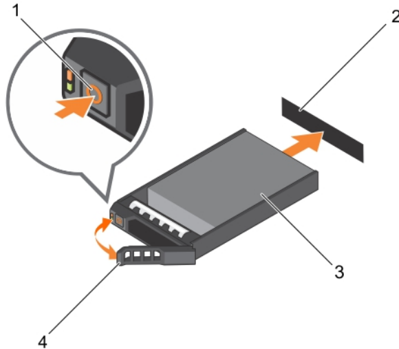
그림 27. 하드 드라이브/SSD 분리 및 설치
