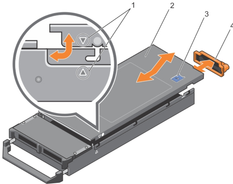
그림 8. 시스템 덮개 분리 및 설치
