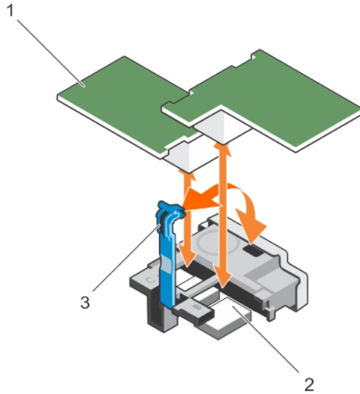
그림 14 . PCIe 메자닌 카드 분리 및 설치
