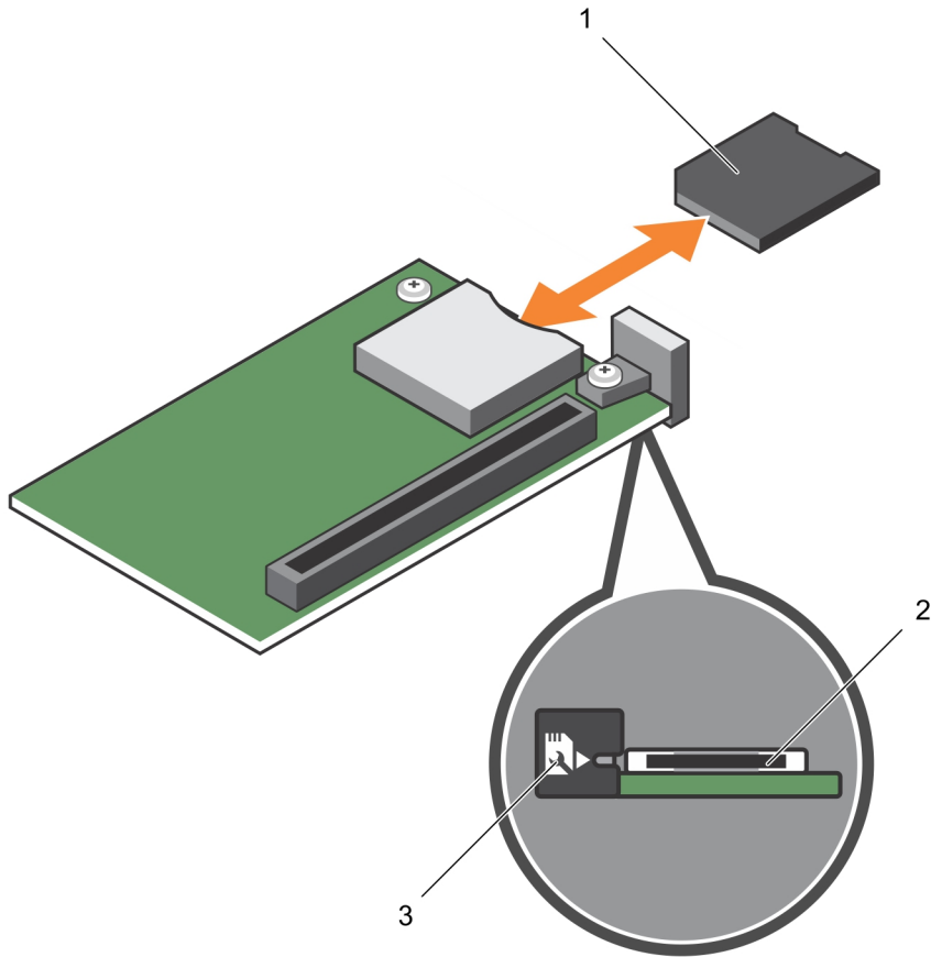
그림 19. SD vFlash 카드 장착
