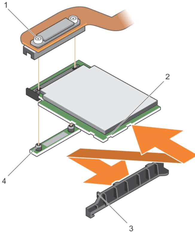
그림 35 . PCIe 확장/저장소 컨트롤러 카드 분리 및 설치
