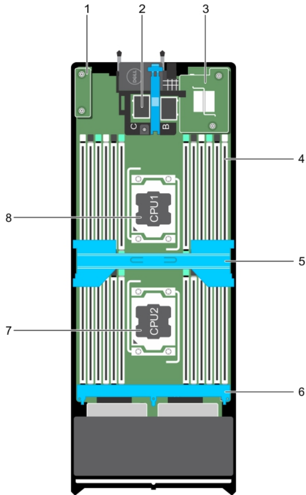
그림 9. 서버 모듈 내부
