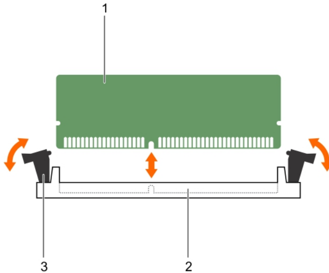
그림 13. 메모리 모듈 분리
