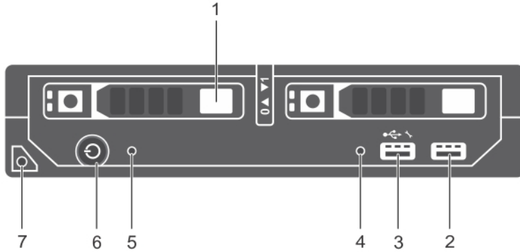
그림 2. 전면 패널 구조 및 표시등 - 2.5인치 하드 드라이브/SSD시스템
