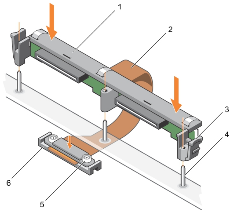
図 56. 2.5 インチ (x2) ハードドライブまたは SSD バックプレーンの取り付け
