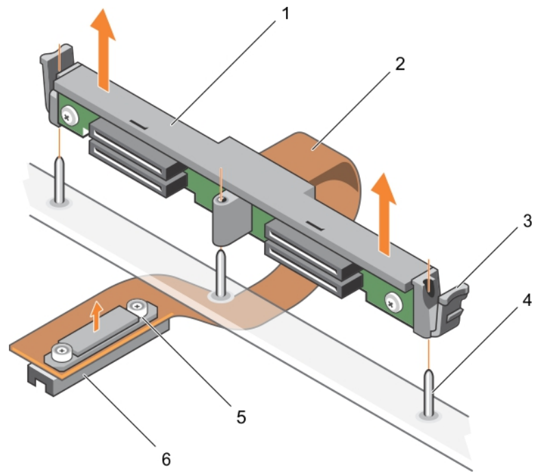
図 55.18 1.8 インチ (x4) SSD バックプレーンの取り外し
