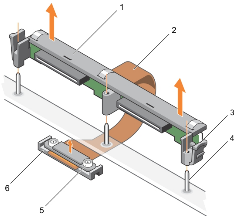
図 54. 2.5 インチ (x2) ハードドライブまたは SSD バックプレーンの取り外し
