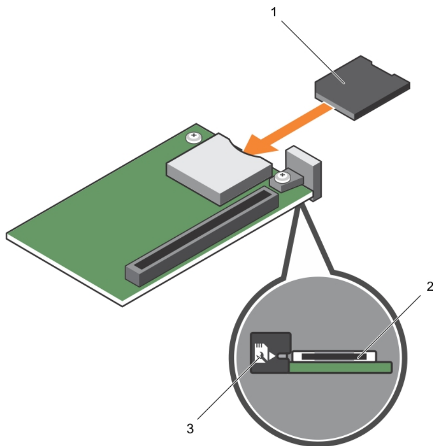
図 30. SD vFlash カードの取り付け
