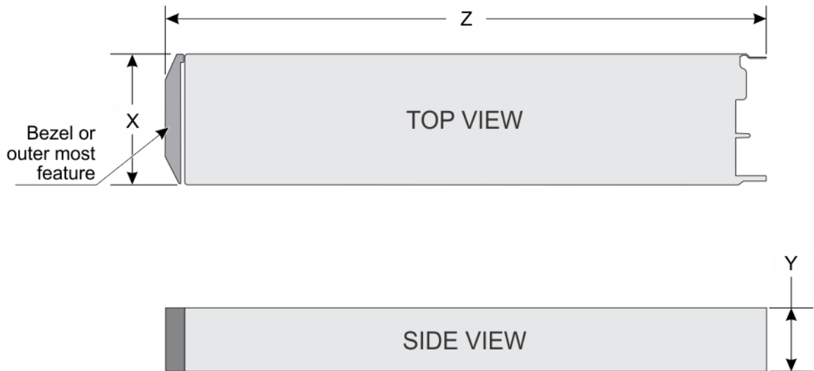
図 6. シャーシ寸法
