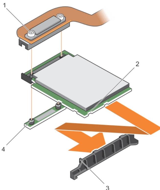
図 64. PCIe エクステンダまたはストレージコントローラカードの取り付け
