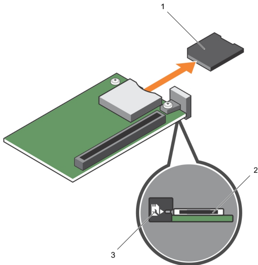
図 29. SD vFlash カードの取り付け
