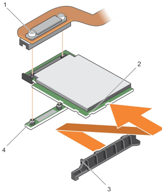
図 63. PCIe エクステンダまたはストレージコントローラカードの取り外し
