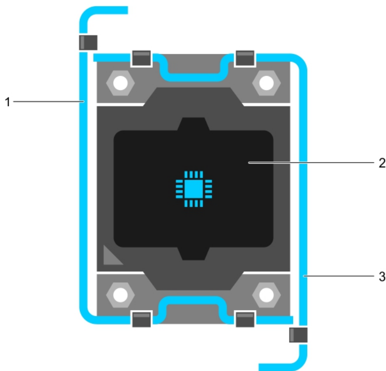
図 34. プロセッサシールドのレバー開閉手順
