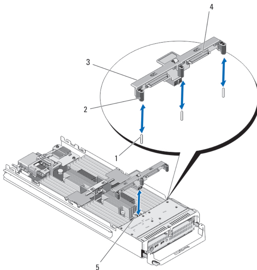
图 19: 卸下和安装硬盘驱动器/SSD 背板
