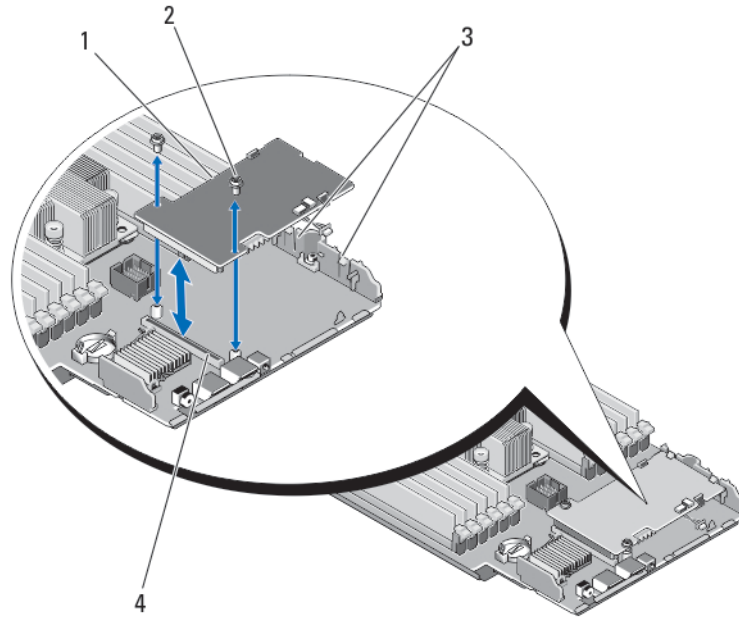
图 22: 卸下和安装 PCIe 扩展卡/存储控制器卡
