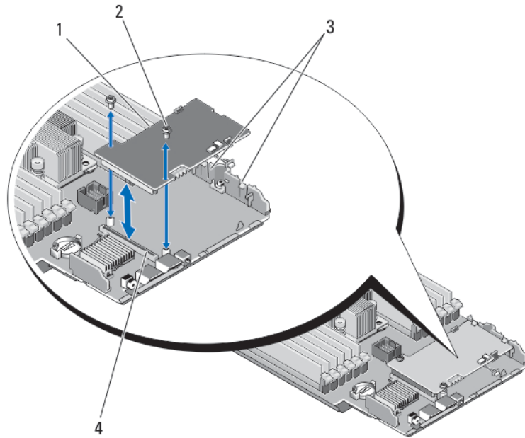
그림 22. PCIe 확장기/저장소 컨트롤러 카드 분리 및 설치
