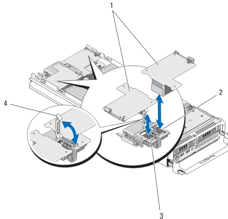
Figure 9. Installation et retrait d'une carte mezzanine
