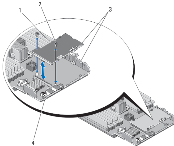
Figure 22. Retrait et installation de la carte PCIe Extender/contrôleur de stockage
