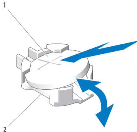
Figure 21. Remplacement de la pile de secours de la NVRAM
