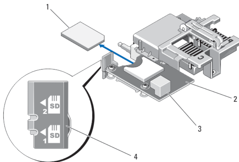
Figure 10. Remplacement de la carte SD
