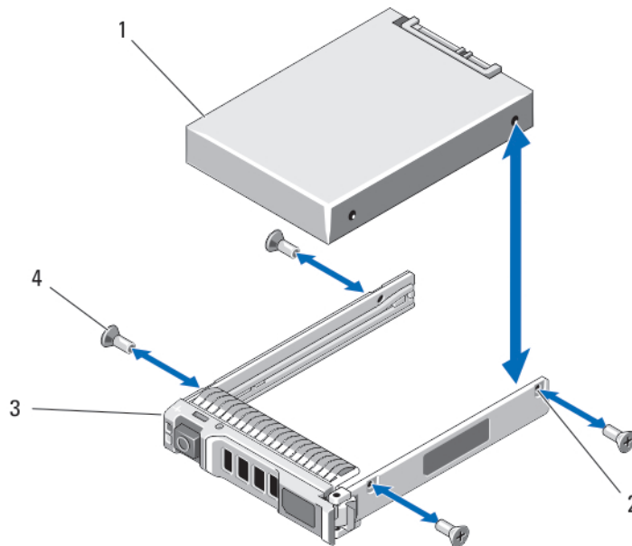
Figure 18. Retrait et installation d'un disque dur/SSD dans un support de disque dur/SSD
