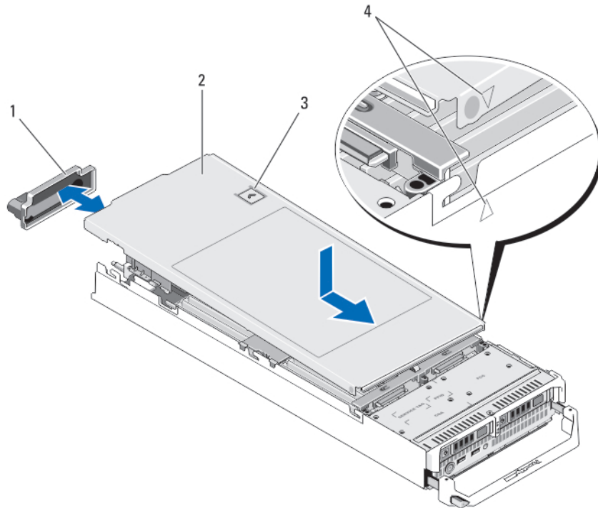
Figure 4. Ouverture et fermeture d'un serveur lame
